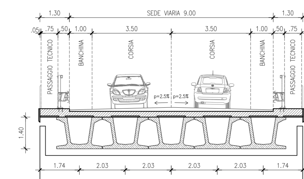
Sezione trasversale - Scala 1:100
