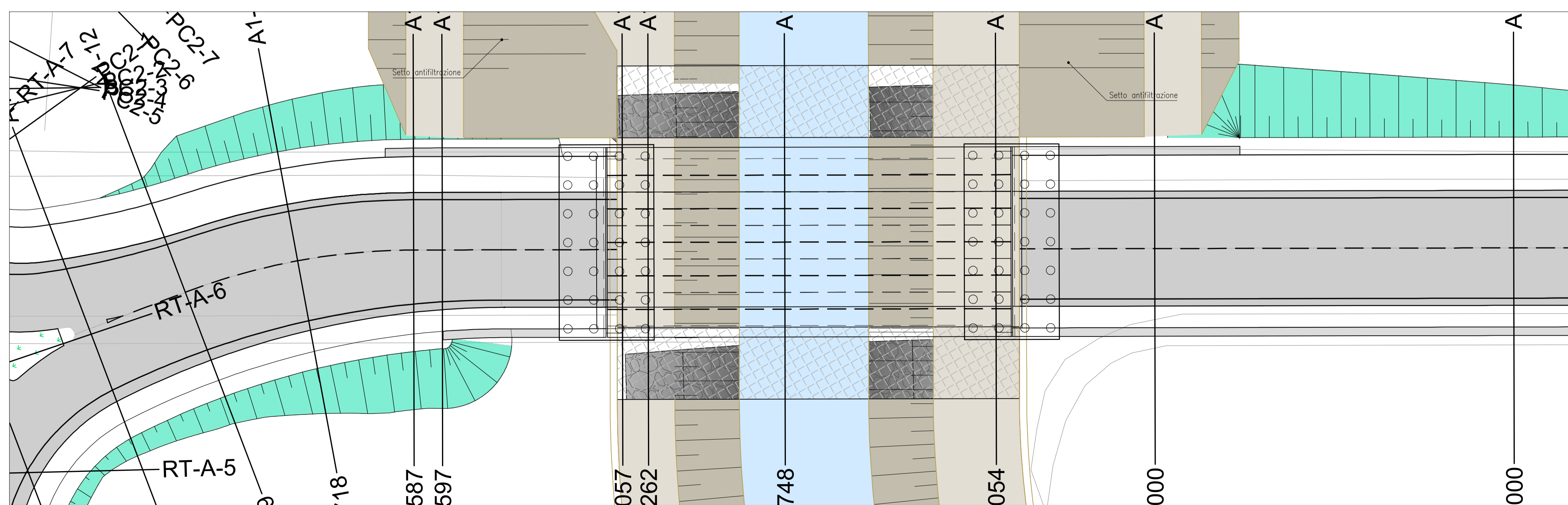
Planimetria di inquadramento - Scala 1:200
