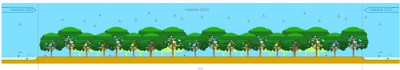
Figura 1. La sezione ambientale della porzione centrale del lago, ove sarà ricreato l'habitat 92A0 – Foreste a galleria di Salix alba e Populus alba , aree starter
