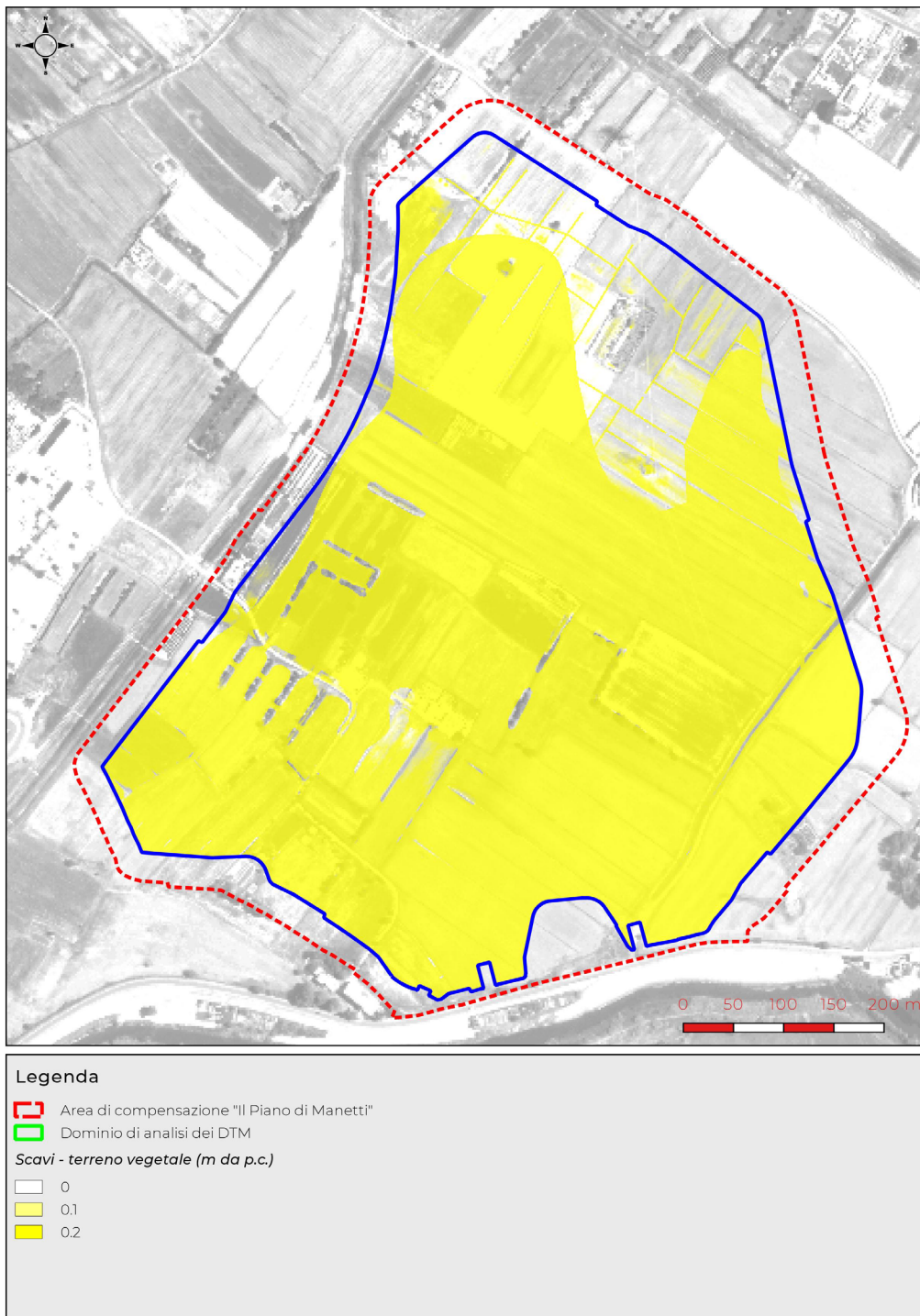
Figura 5. Ricostruzione degli habitat – opere agronomiche e naturalistiche: planimetria di sintesi degli scavi – terreno vegetale
