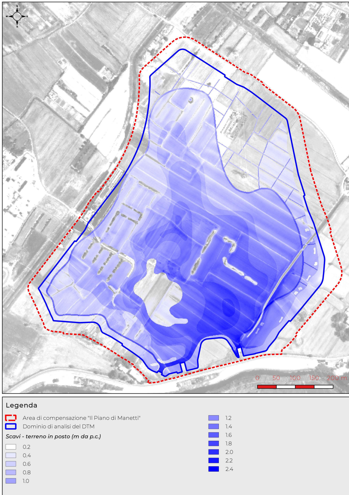
Figura 6. Ricostruzione degli habitat – opere agronomiche e naturalistiche: planimetria di sintesi degli scavi – terreno in posto
