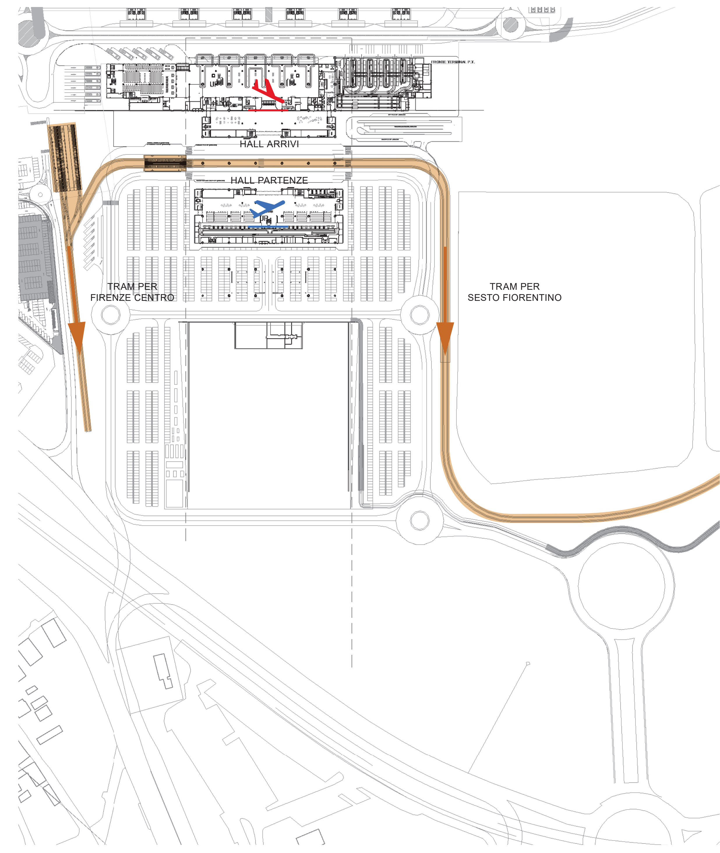
CIRCOLAZIONE TRAMVIARIA 1 : 2,000 2
