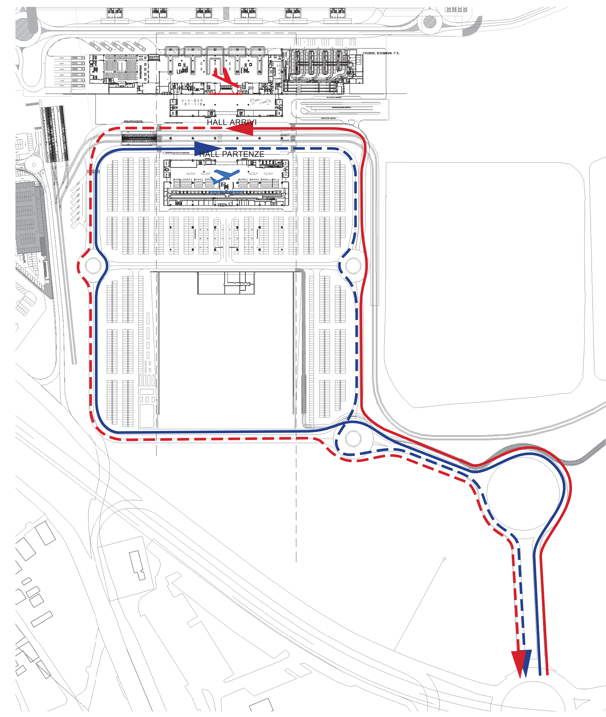
CIRCOLAZIONE AUTOVEICOLI 1 : 2,000 1
