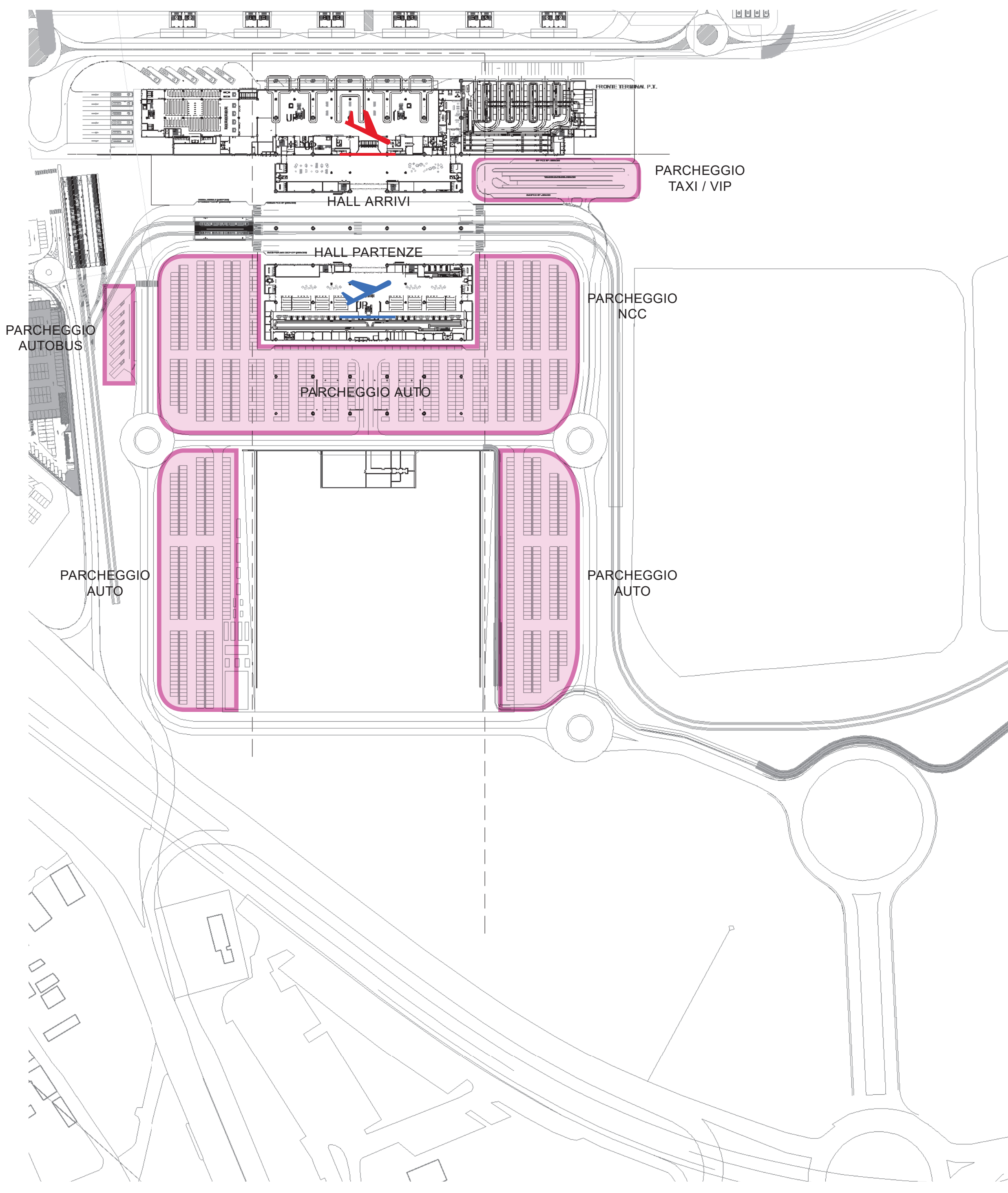
PARCHEGGIO 1 : 2,000 6
