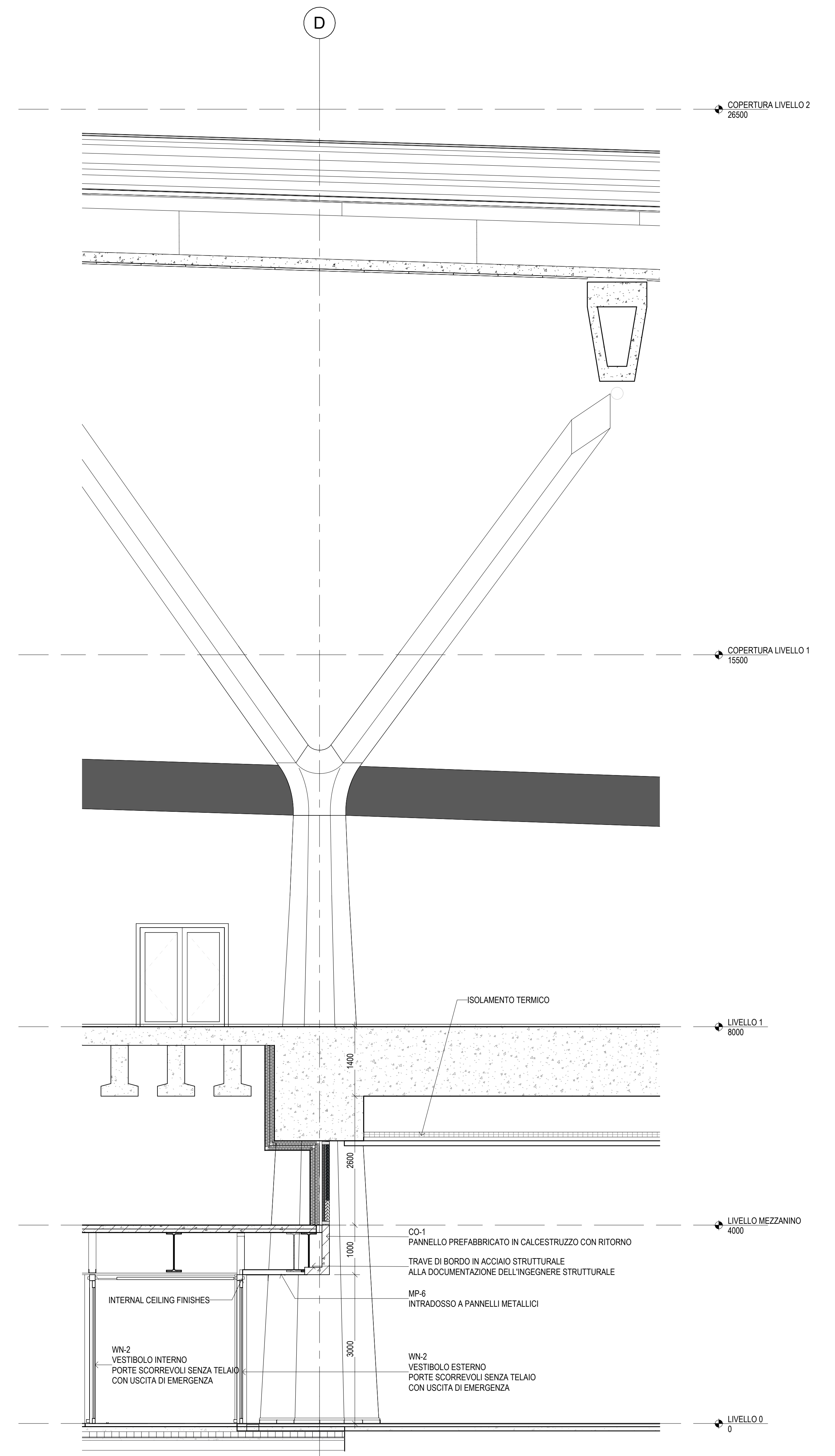
SEZIONE NORD SUD 1 : 50
