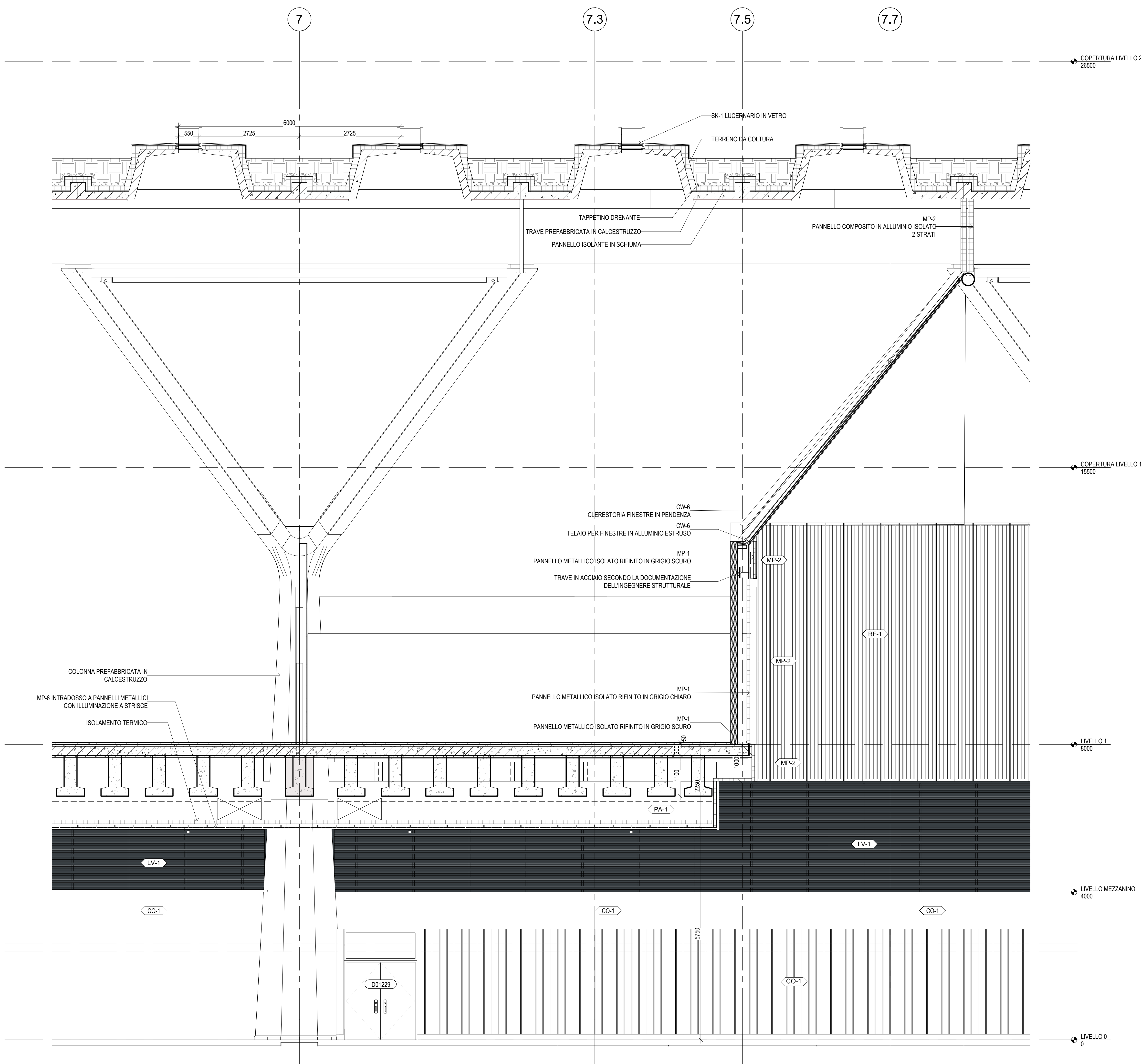
PROSPETTO SUD AIRSIDE 1 : 50
