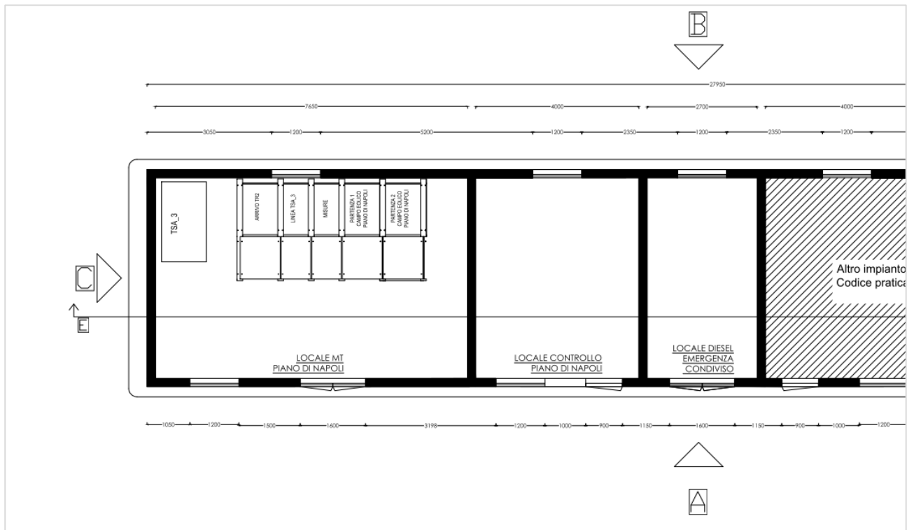
Figura 10 – Planimetria del Locale Controllo e Locale MT (1/2)
