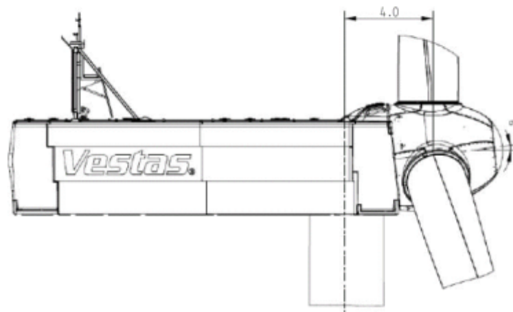
Figura 4 - Rappresentazione navicella Vestas
