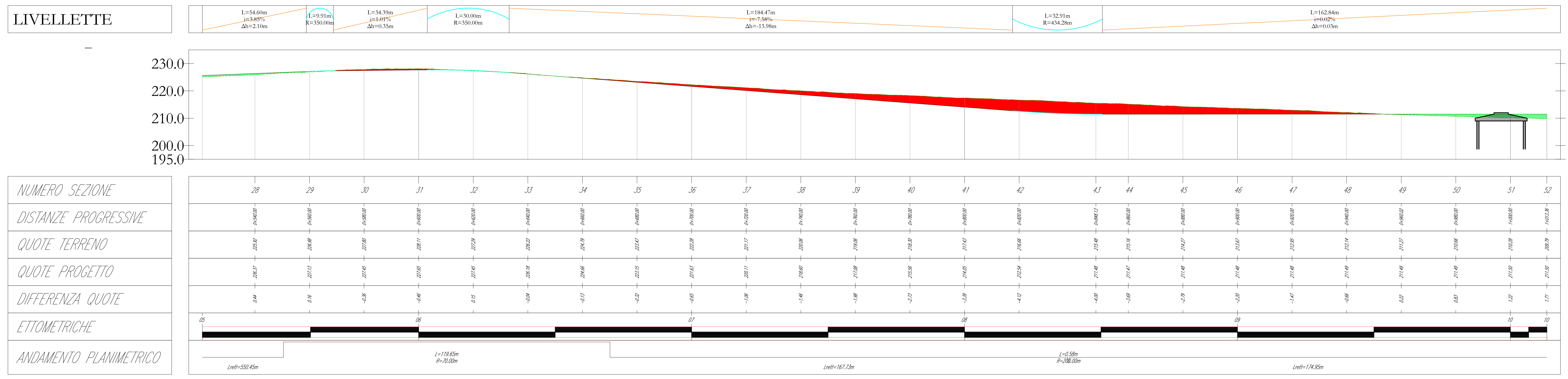
Profilo: Tracciato 2 di 2 Q.Rif. : 195.00
