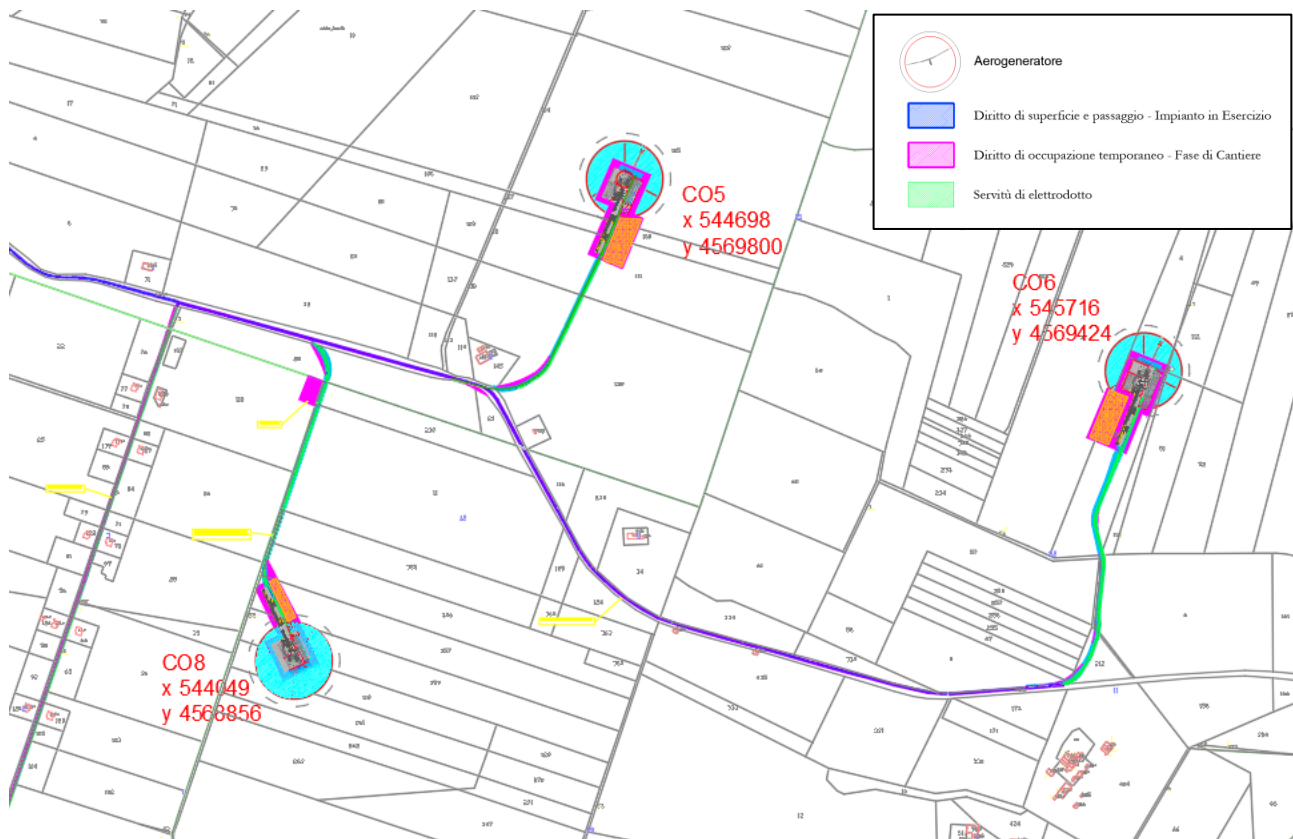
Figura 4 - Rappresentazione grafica generale aree di occupazione e servizi (2/2)
