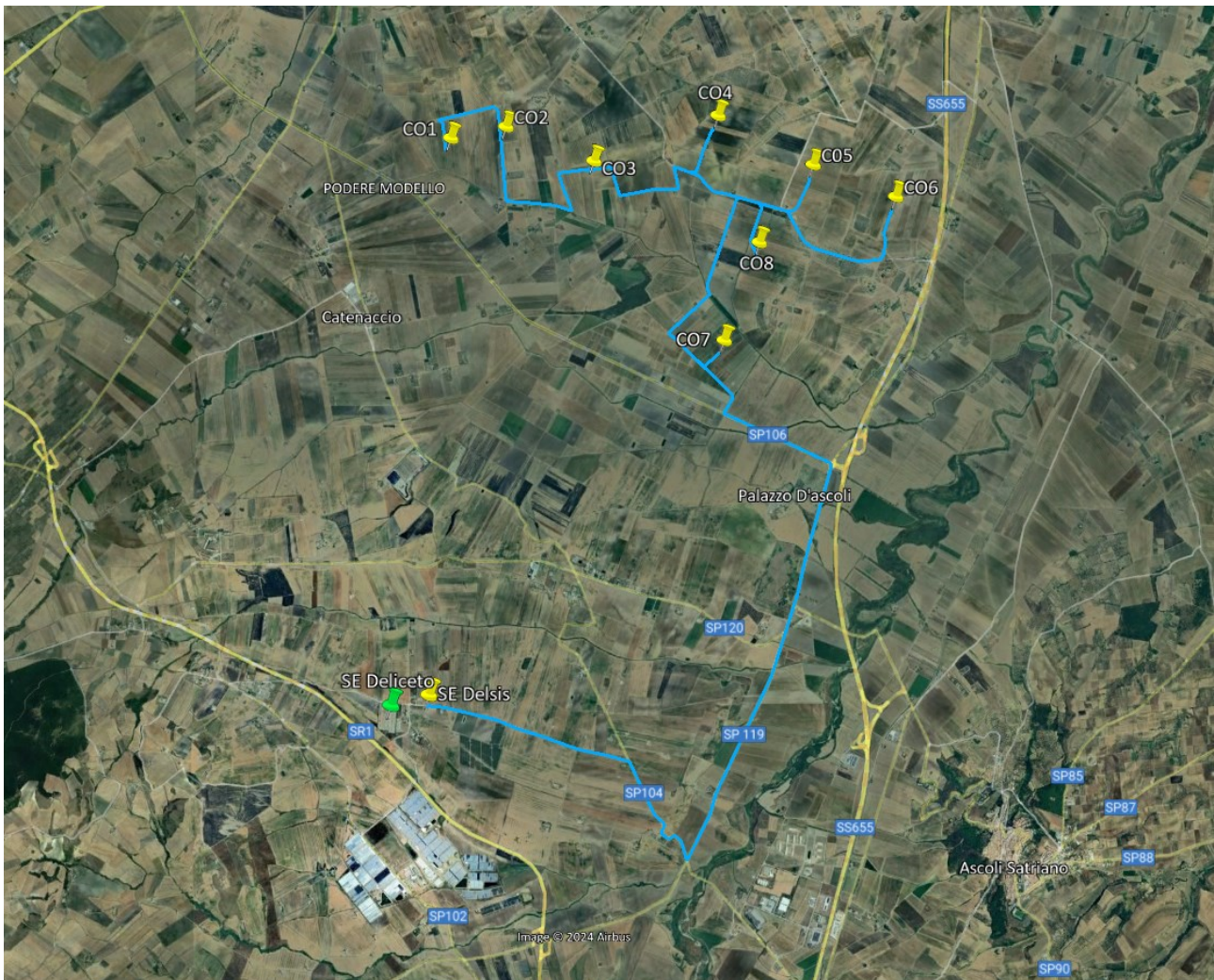
Figura 8 – Rappresentazione grafica generale del cavidotto
