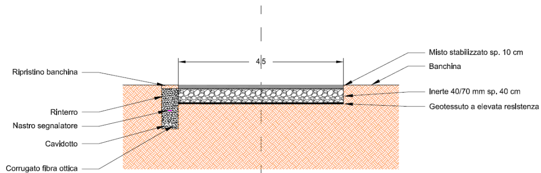
Figura 6 – Sezione tipo strade
