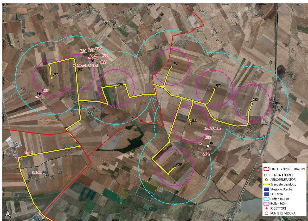
Figura 6: Zona d'impianto con individuazione dei ricettori (R) e dei punti di misura (P) considerati nella stima previsionale di emissione delle turbine di progetto (CO) proposta nella versione ortofotografica satellitare estratta da Google Earth.
