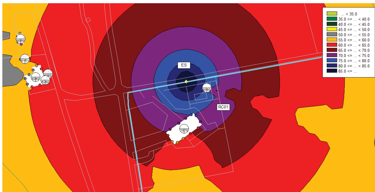
Figura 8 – Stralcio planimetrico della mappa acustica calcolata in corrispondenza del ricettore RC01 nelle fasi di cantiere maggiormente critiche (Fase 16).
