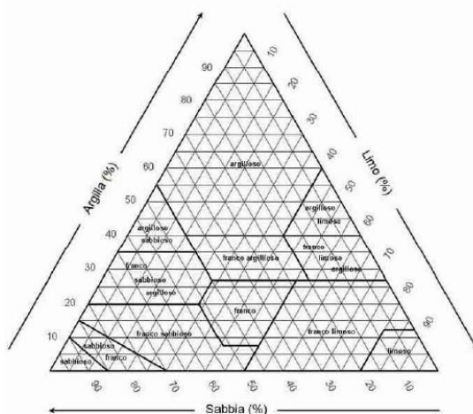
Figura 3.6. – Classificazione Tessitura del terreno USDA.
