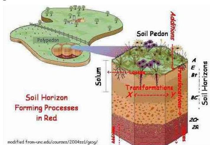
Figura 3.5. – Unità rappresentativa del suolo – PEDON.
