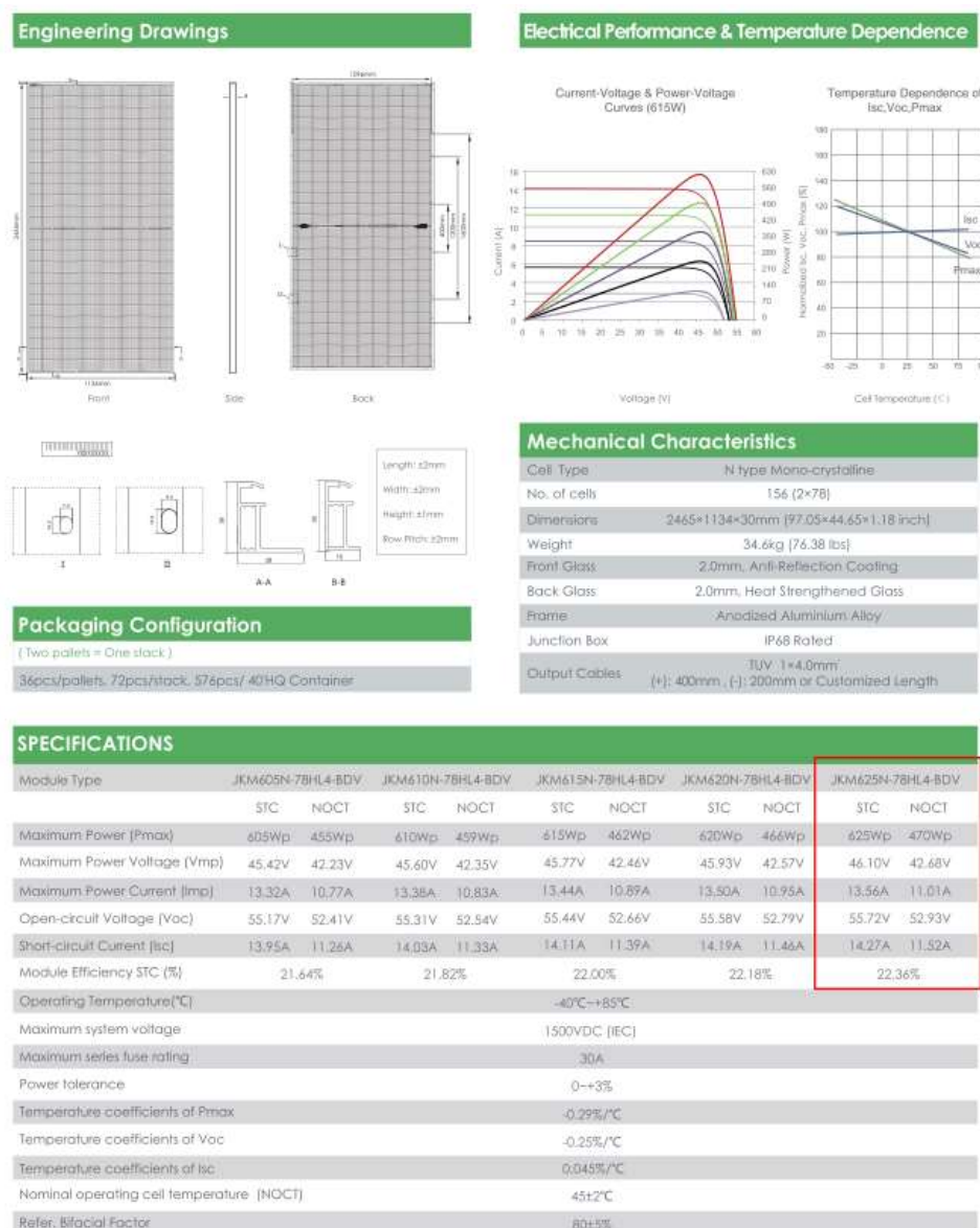
Figura 1 - Dati tecnici pannelli FV
