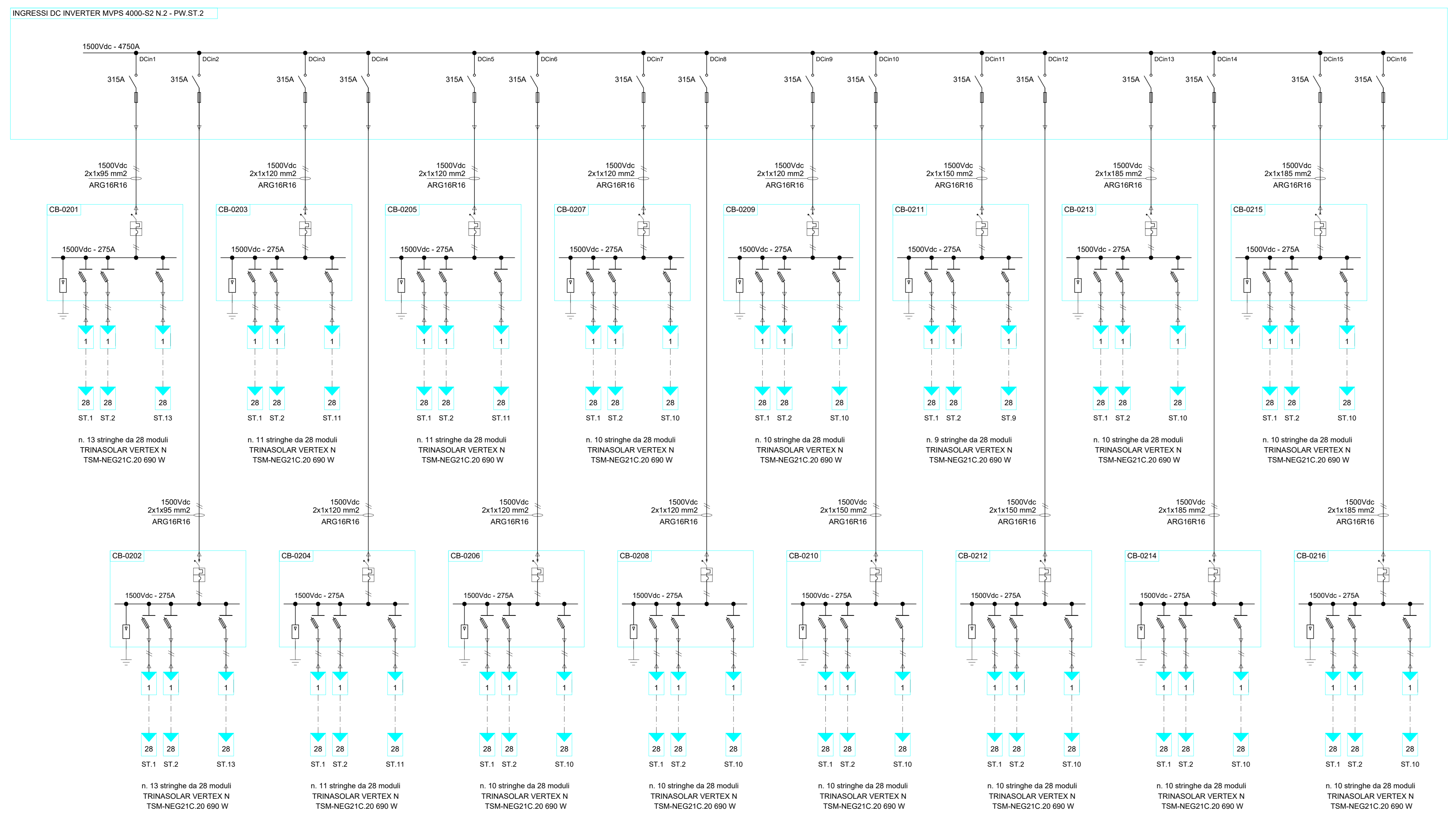
Schema Unifilare BT. StringBox - SOTTOCAMPO 2
