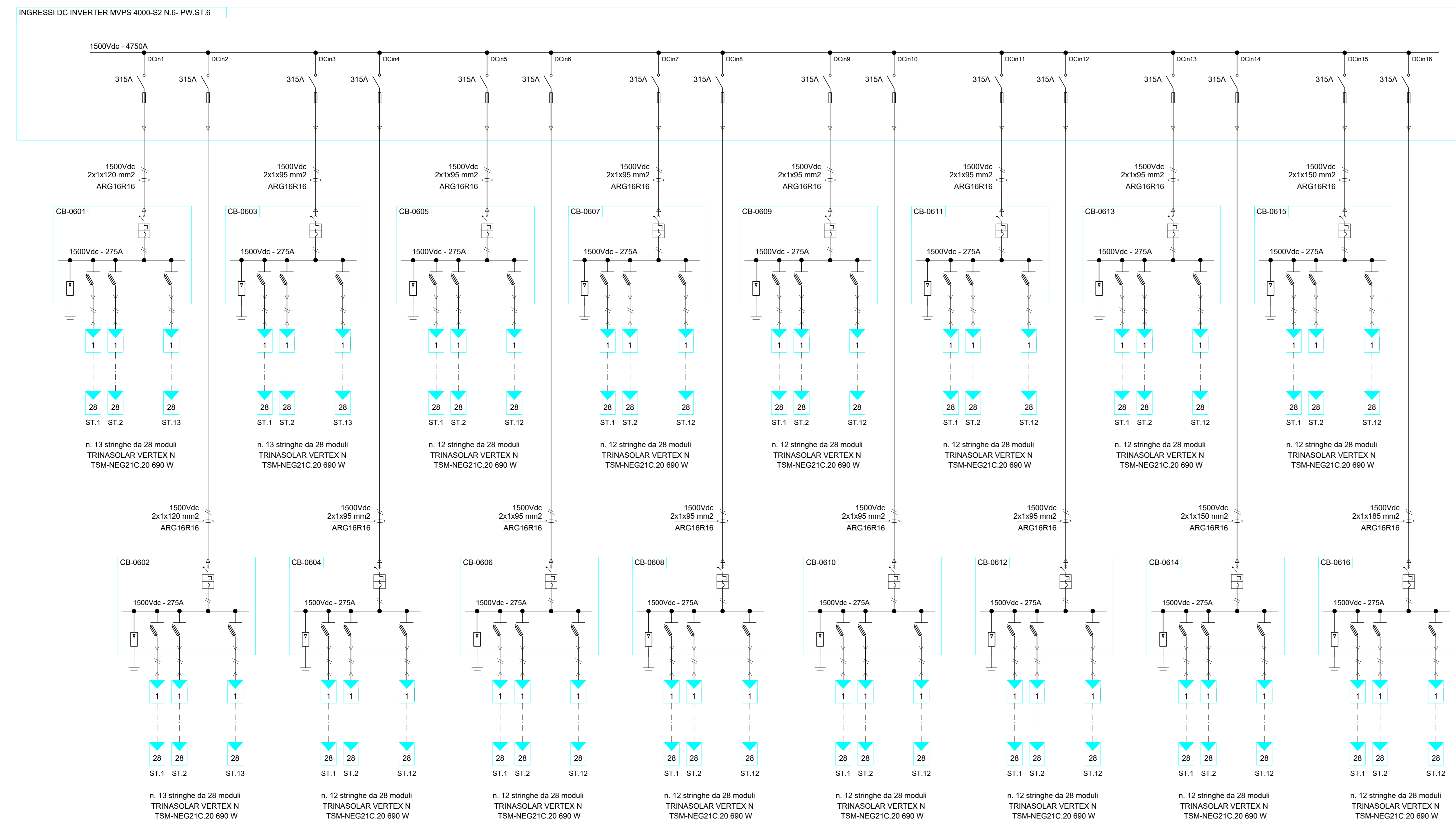
Schema Unifilare BT. StringBox - SOTTOCAMPO 6
