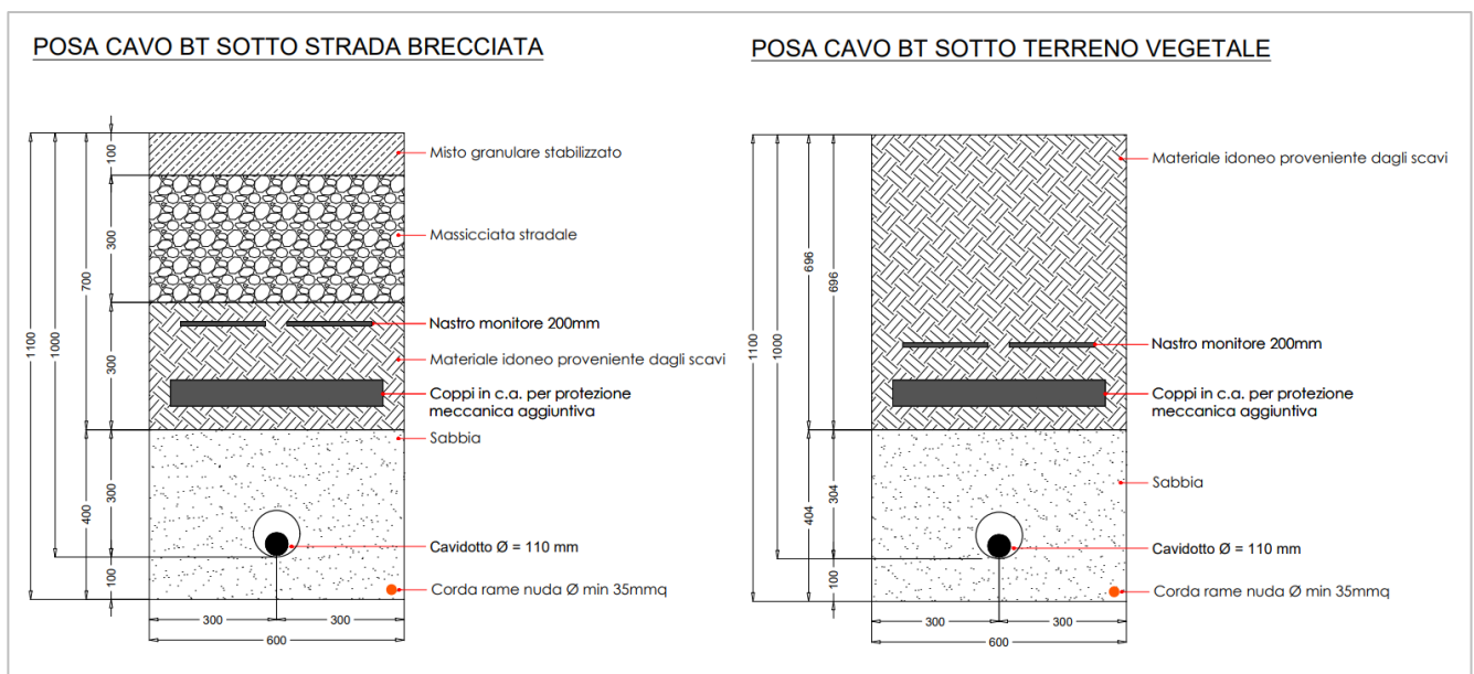
Figura 26 – Tipologico sezioni scavo BT
