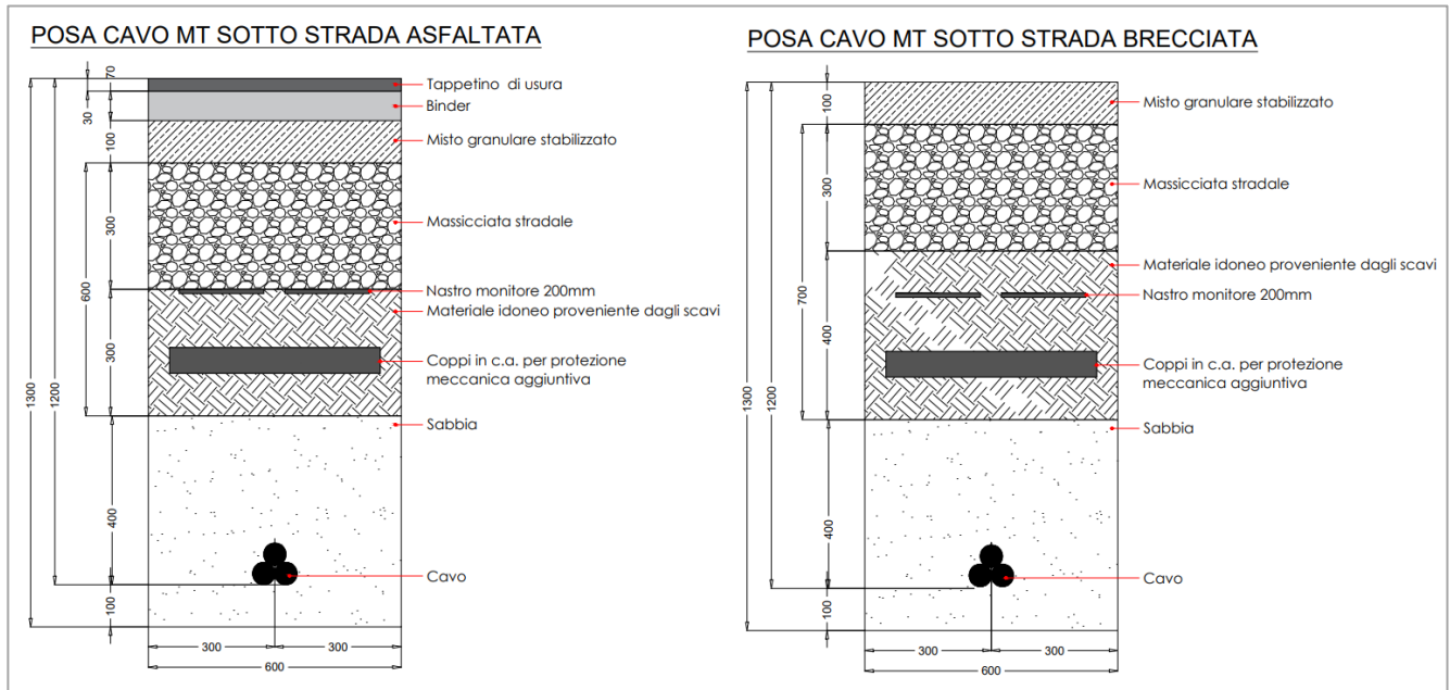
Figura 25 – Tipologico sezioni scavo MT
