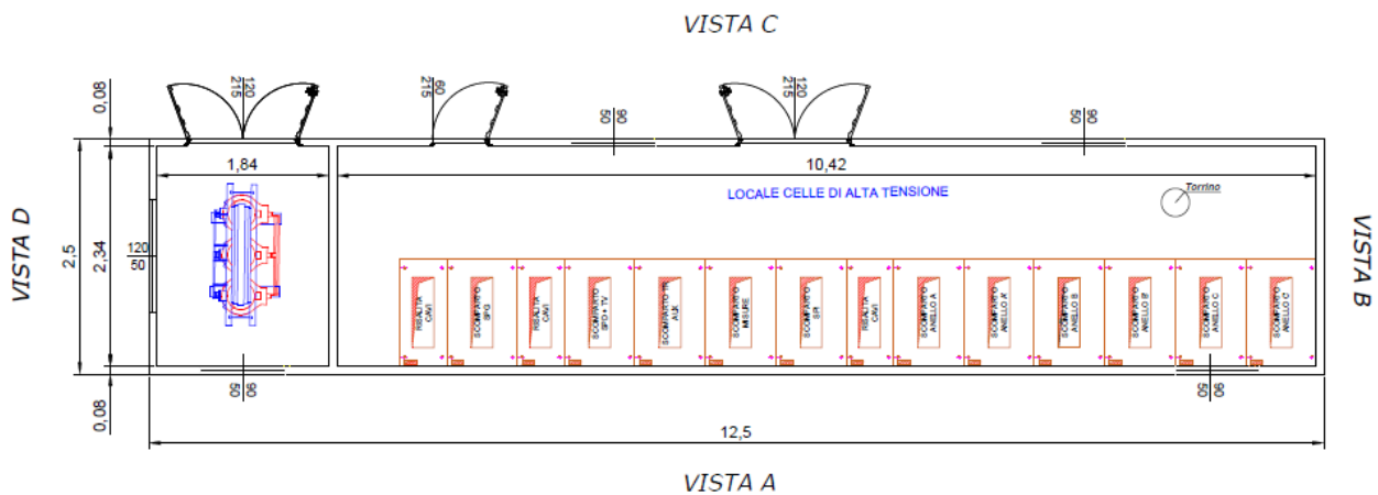
Figura 20 – Dimensioni cabina raccolta utente
