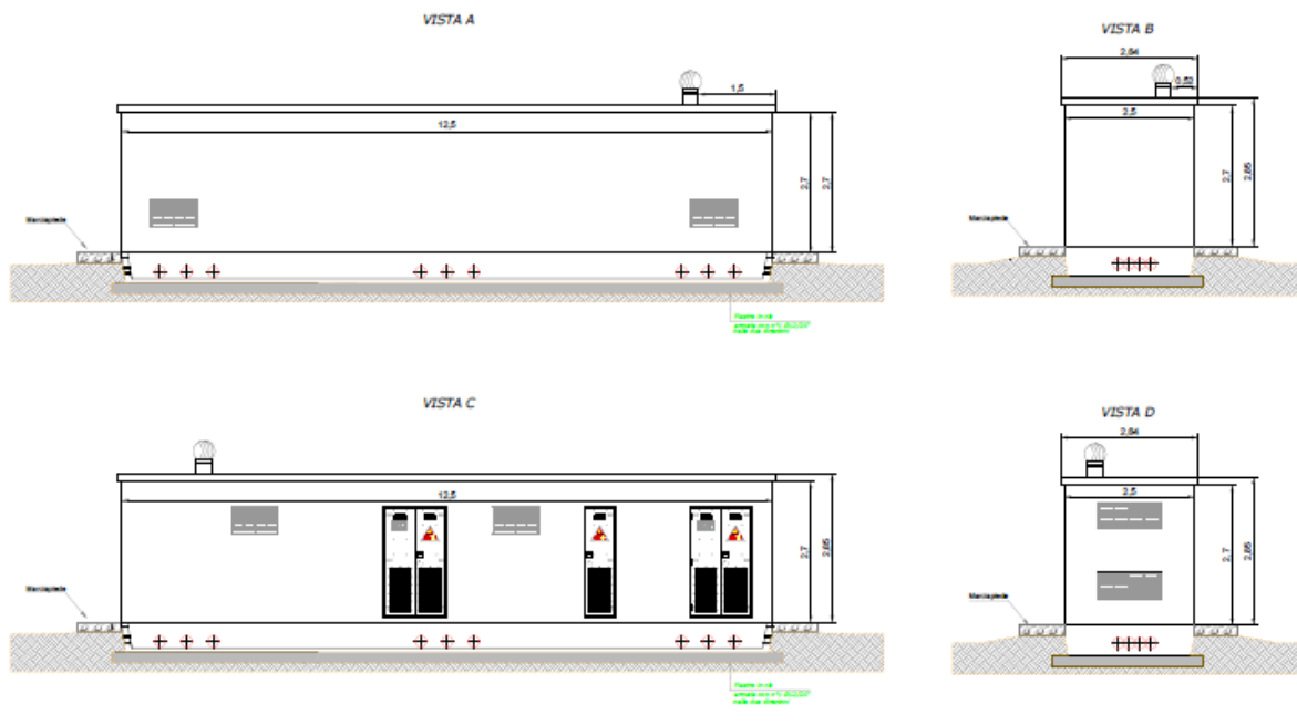
Figura 21 – Vista cabina raccolta utente
