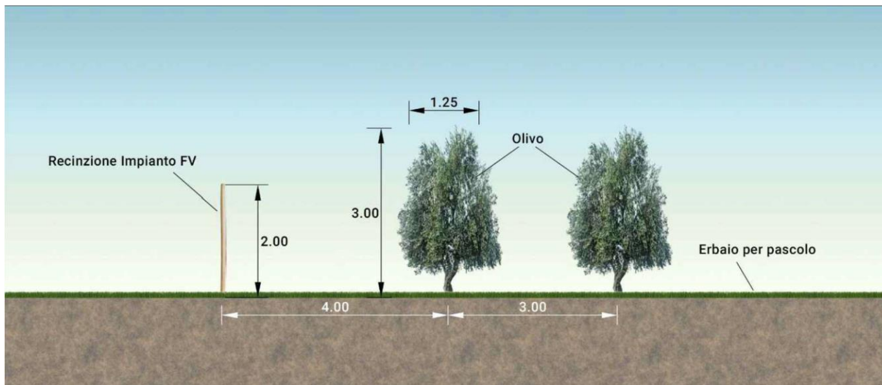
Figura 24 Sezione dell'impianto con l'indicazione della disposizione dell'oliveto e della recinzione.
