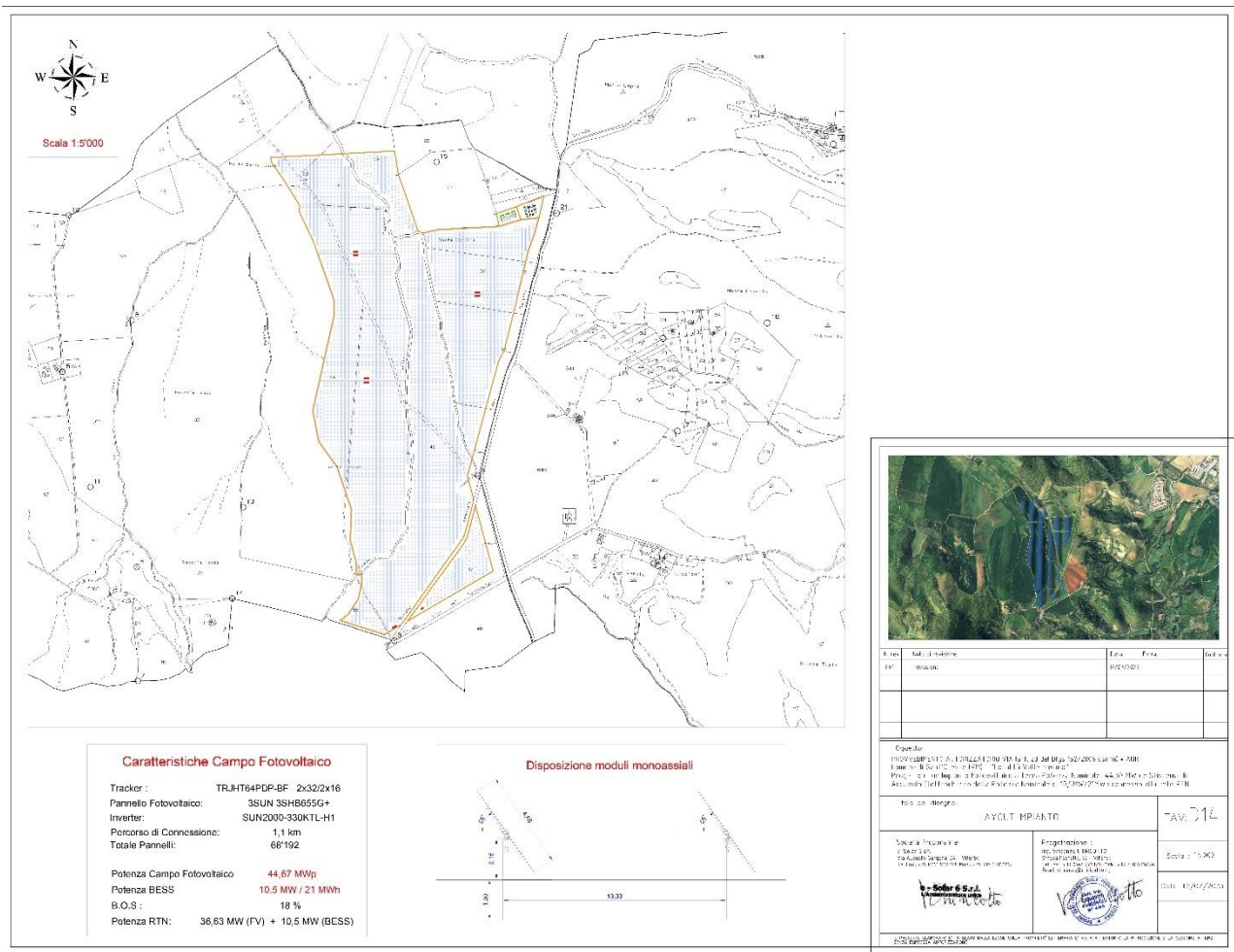
Figura 23 – Layout impianto
