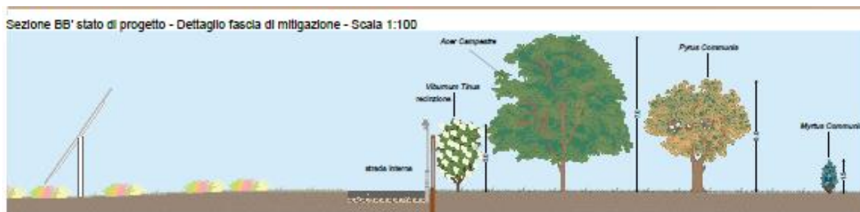
Figura 84 - Sezione area di mitigazione SP
