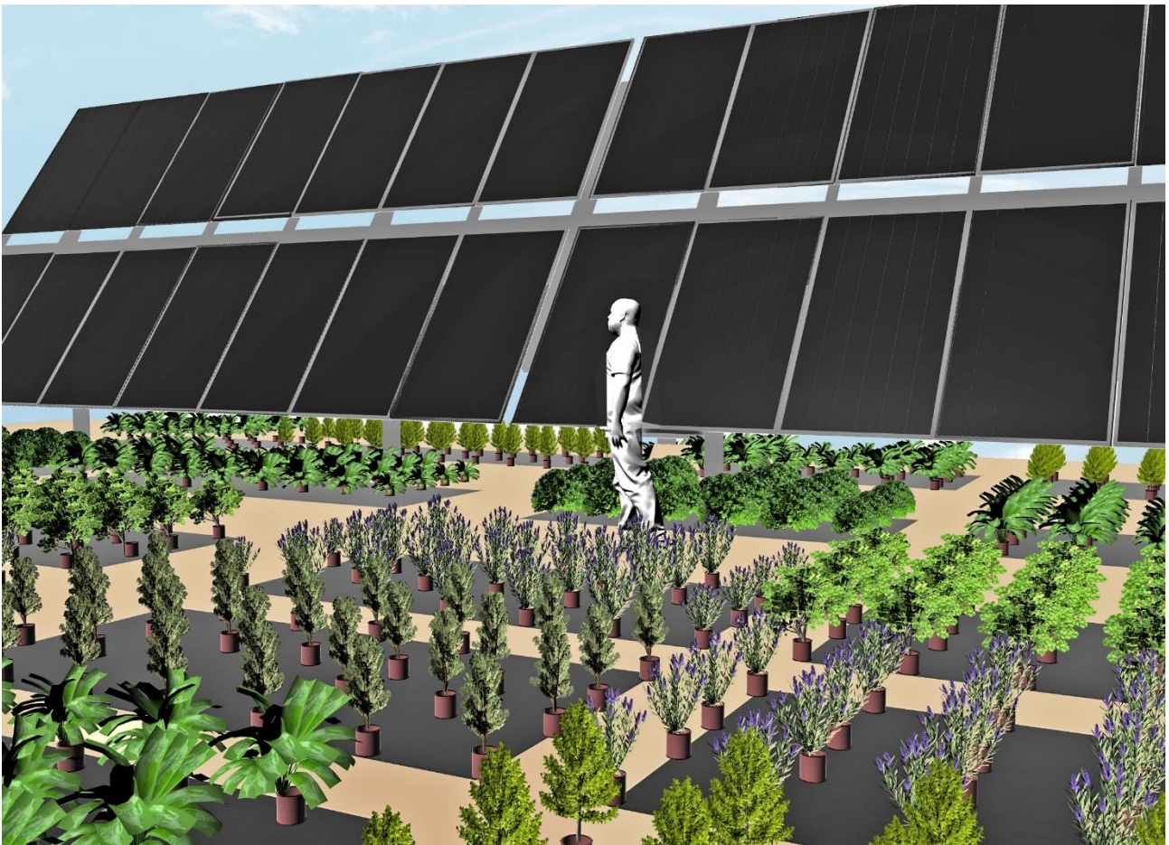
Figura 26 - Veduta del modello tracker alla massima altezza
