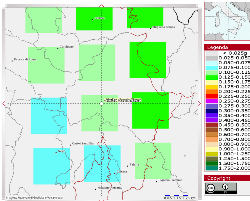
Figura 32 - Mappa interattiva della pericolosità sismica
