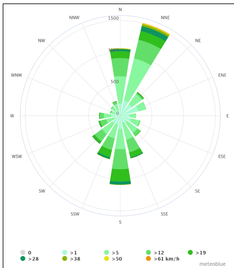
Figura 44 - Rosa dei venti
