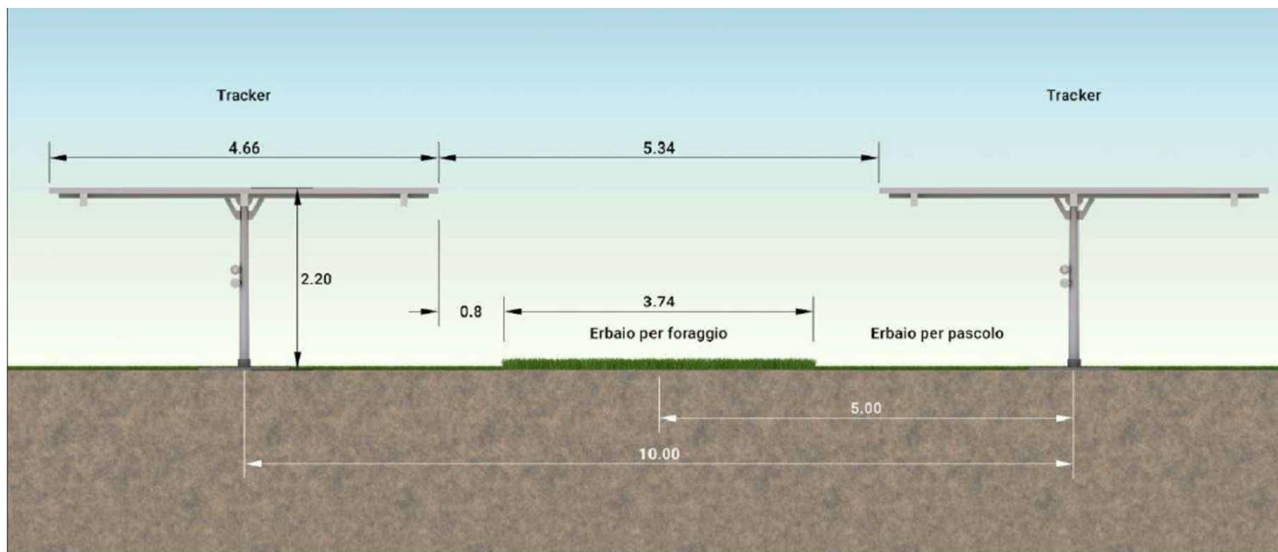
Figura 23 Sezione dell'impianto con l'indicazione della disposizione delle colture agrarie. Area dei tracker.
