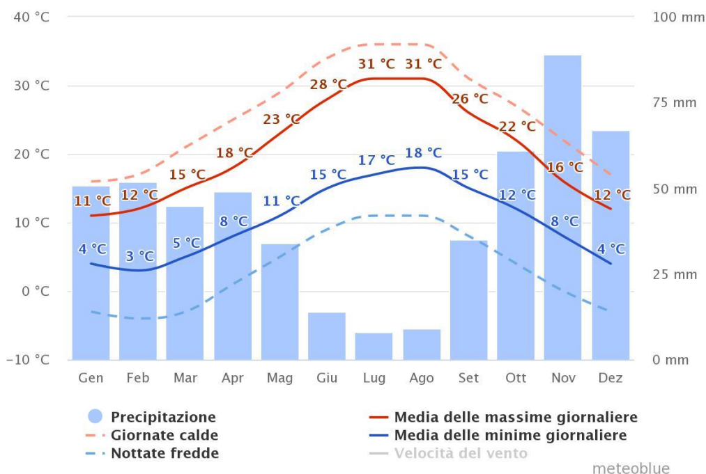
Figura 42 - Dati climatici simulati (previsione)
