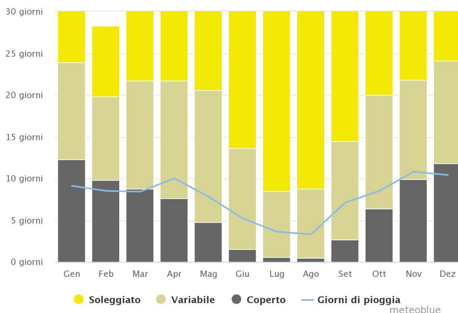
Figura 45- Grafico dei giorni nuvolosi, soleggiati e di pioggia
