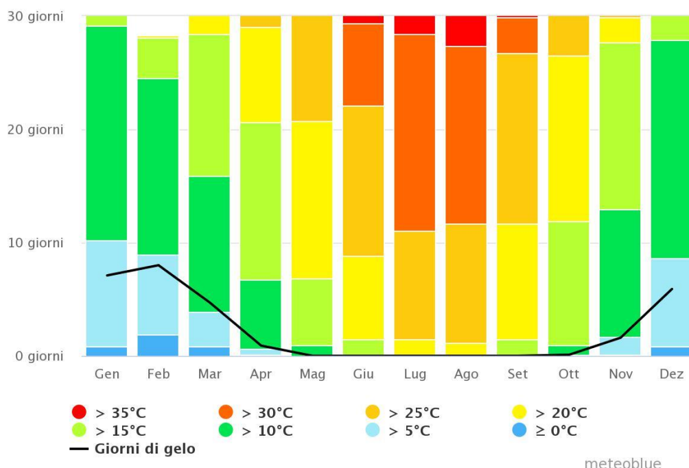
Figura 40 - Andamento delle temperature
