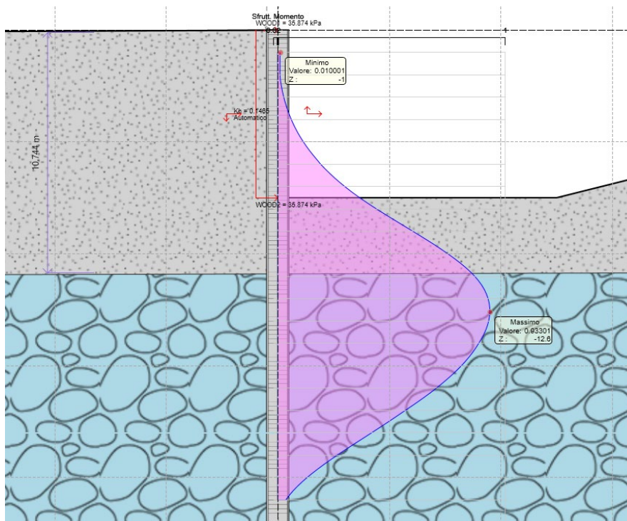
Figura 8.9 Sfruttamento a momento ENV SLU-SISMA
