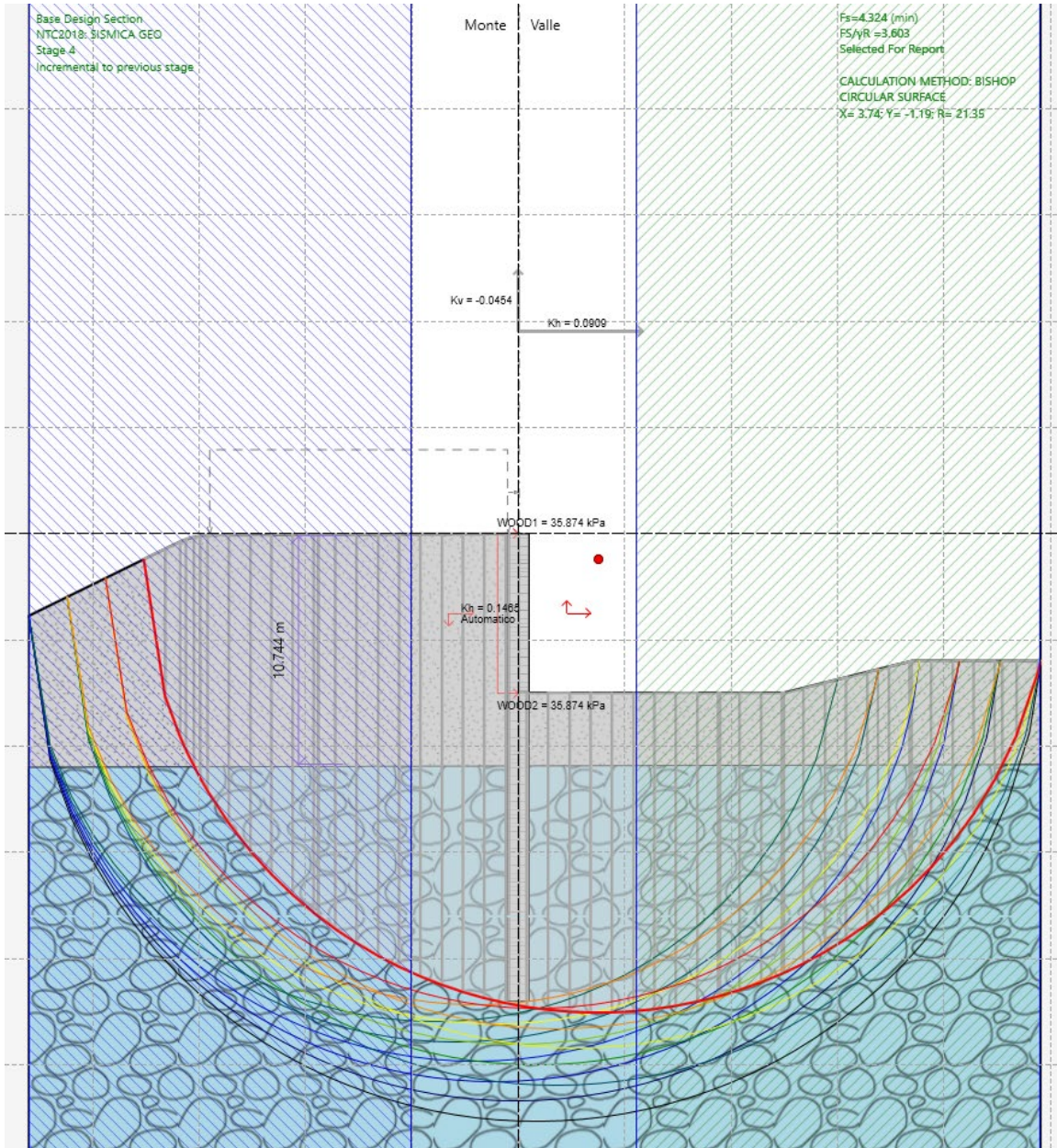
Fig. 14 – Analisi di stabilità SISMICA per il caso A2+M2+SISMA -kv
