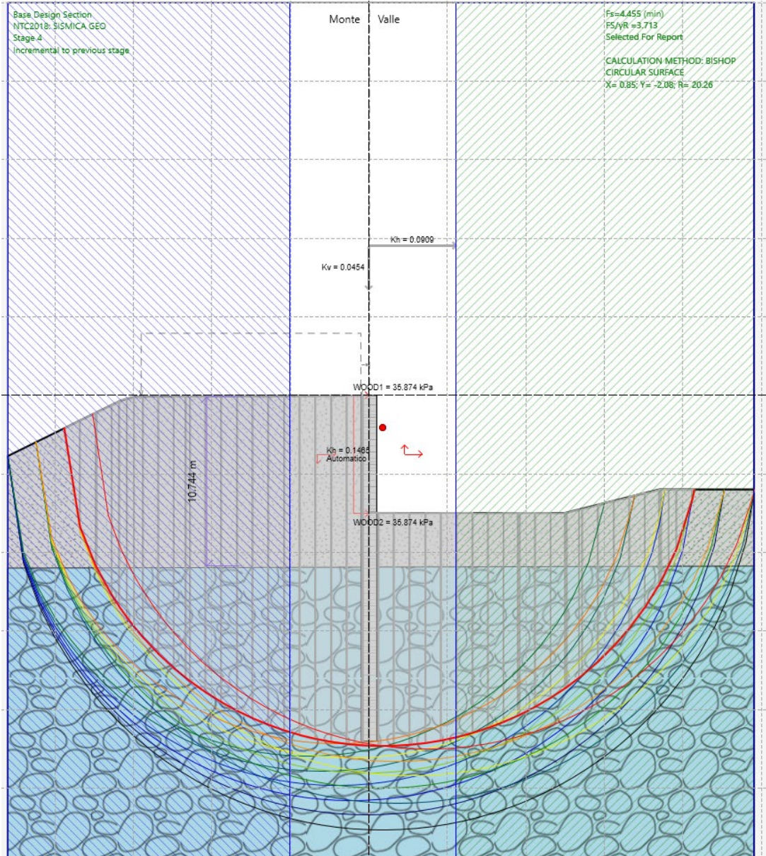
Fig. 13 – Analisi di stabilità SISMICA per il caso A2+M2+SISMA +kv
