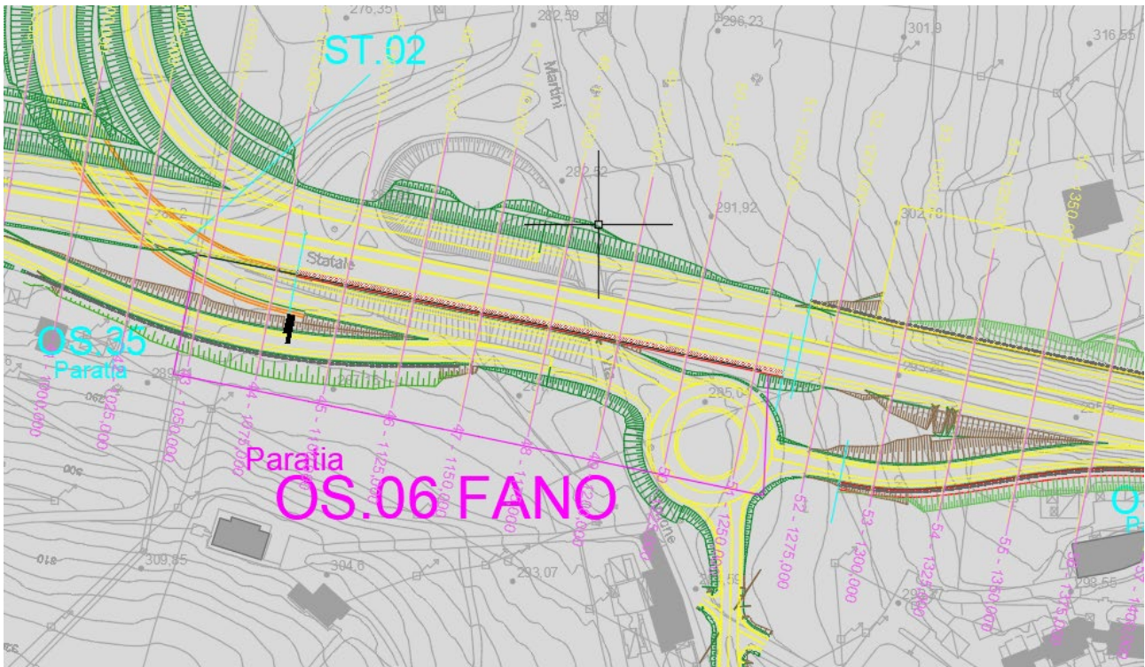
Figura 1.1 KeyPlan dell'opera
