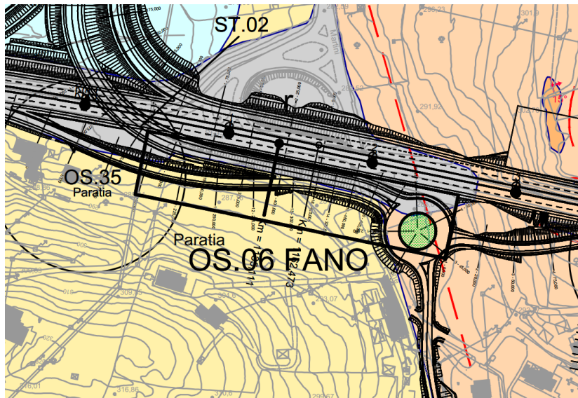
Figura 7.1 Collocazione dell'opera in pianta
