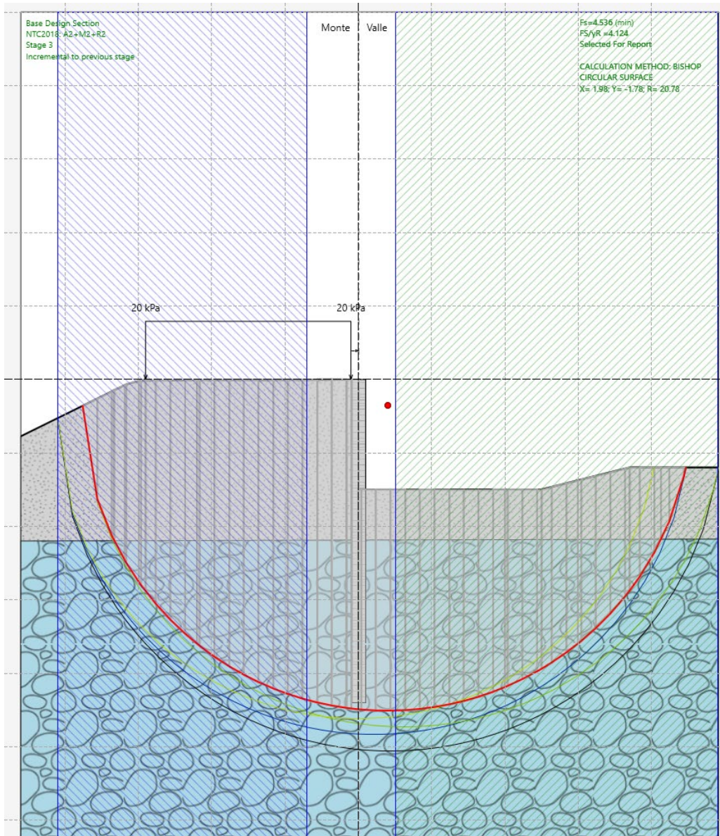
Fig. 12 – Analisi di stabilità STATICA per il caso A2+M2+R2
