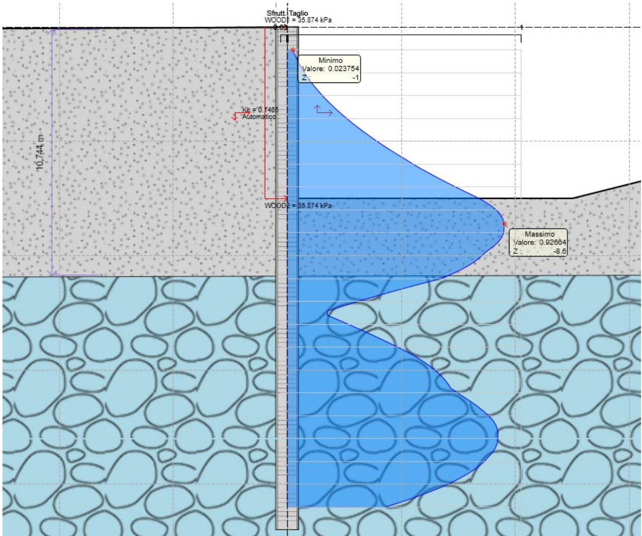
Figura 8.10 Sfruttamento a taglio ENV SLU-SISMA
