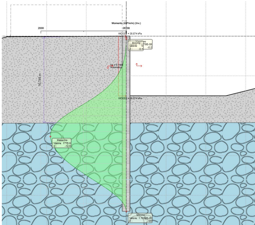
Figura 8.7 Diagramma Momento ENV SLU-SISMA
