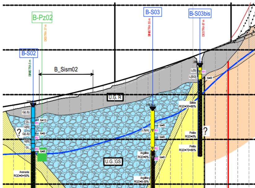
Figura 7.2 Sovrapposizione dell'opera con il profilo in asse
