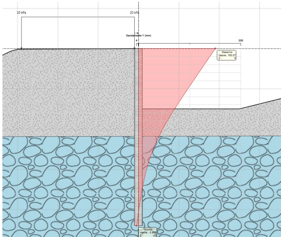
Figura 8.11 Spostamento massimo della paratia
