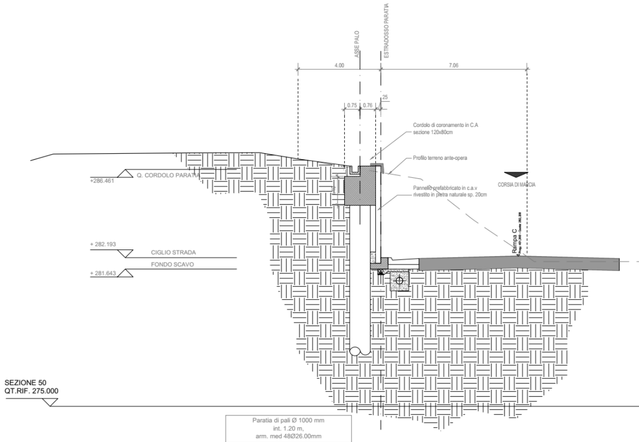
Figura 1.4 Sezioni tipo dell'opera
