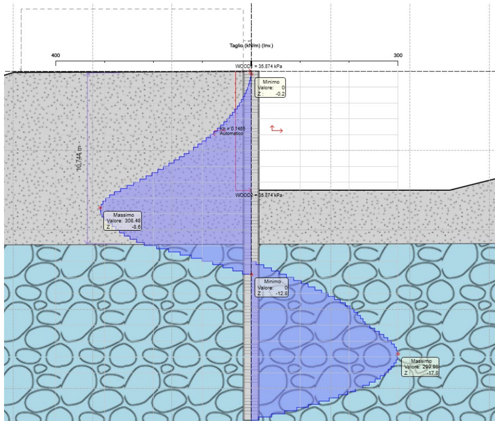
Figura 8.8 Diagramma Taglio ENV SLU-SISMA
