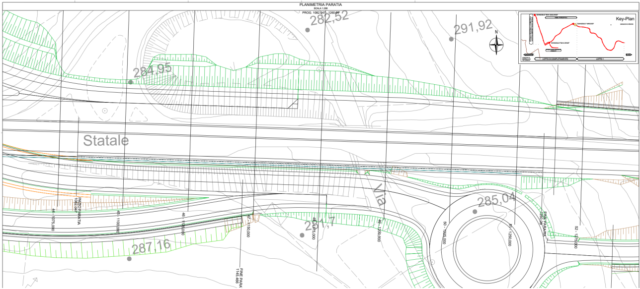
Figura 1.2 Planimetria dell'opera
