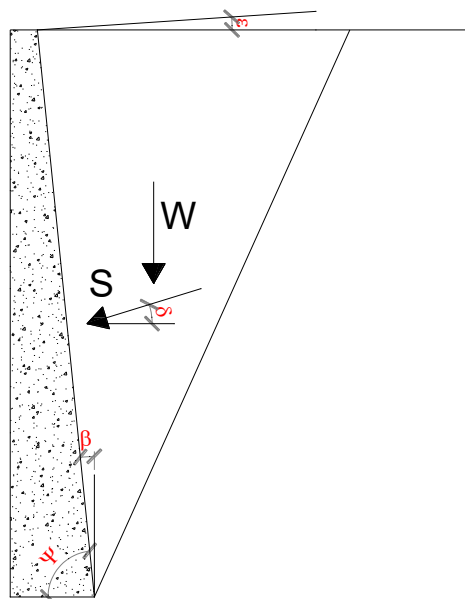
Figura 2-2 Parametri geoemetrici per il calcolo dei coefficienti di spinta attiva e passiva.
