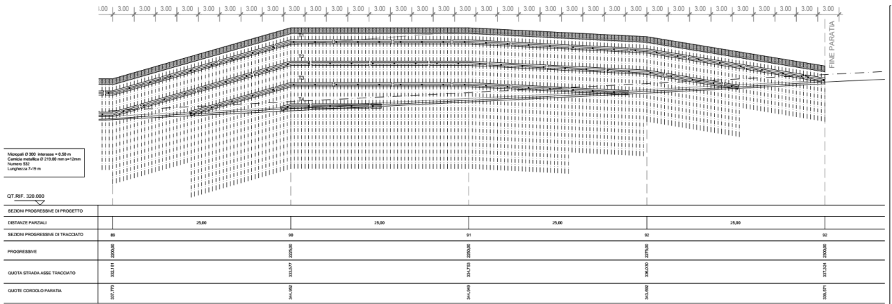
Figura 1.3 Profilo dell'opera
