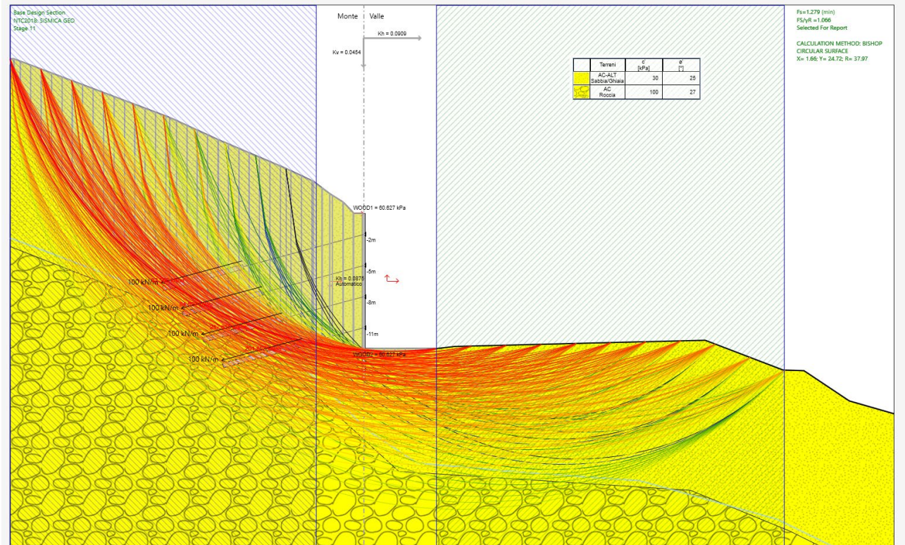
Fig. 16 – Analisi di stabilità SISMICA per il caso A2+M2+SISMA +kv
