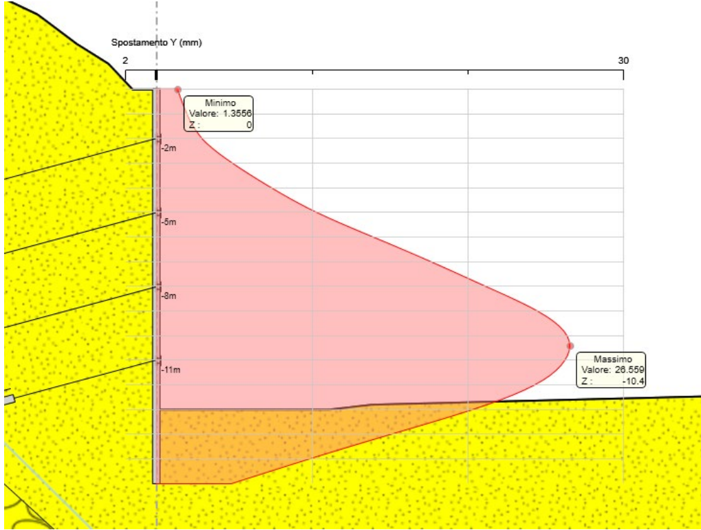
Figura 8.14 Spostamento massimo della paratia
