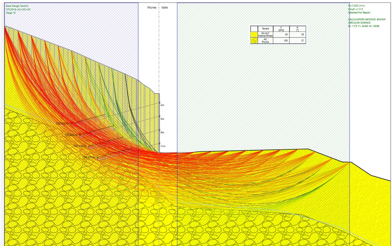
Fig. 15 – Analisi di stabilità STATICA per il caso A2+M2+R2
