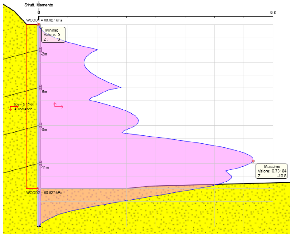
Figura 8.11 Sfruttamento a momento ENV SLU-SISMA
