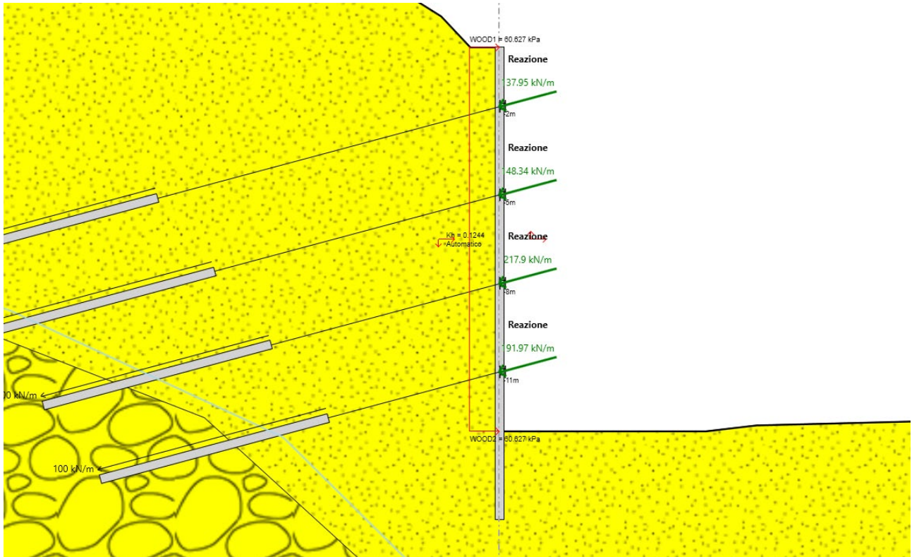
Figura 8.13 Reazioni ai supporti ENV SLU-SISMA
