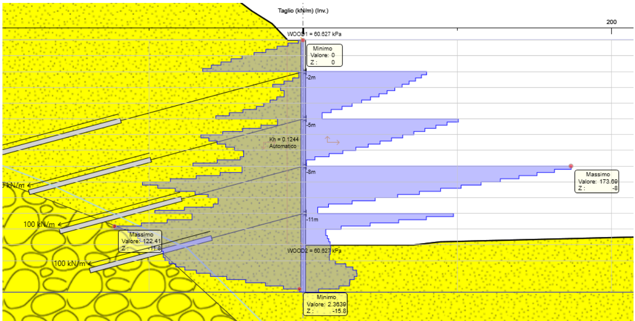
Figura 8.10 Diagramma Taglio ENV SLU-SISMA
