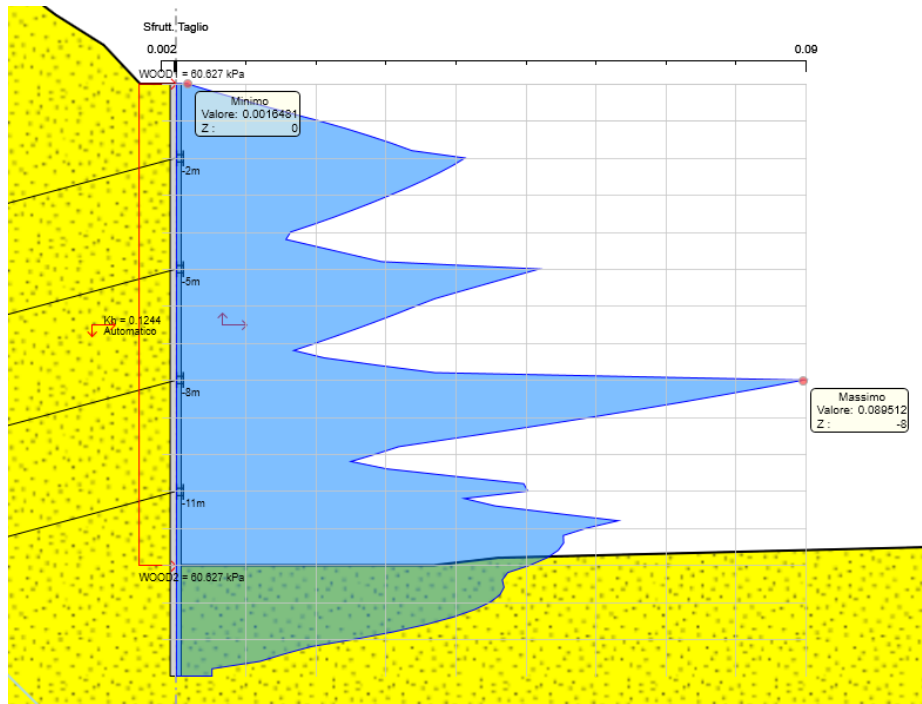
Figura 8.12 Sfruttamento a taglio ENV SLU-SISMA
