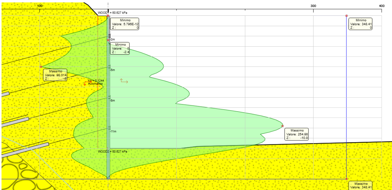
Figura 8.9 Diagramma Momento ENV SLU-SISMA
