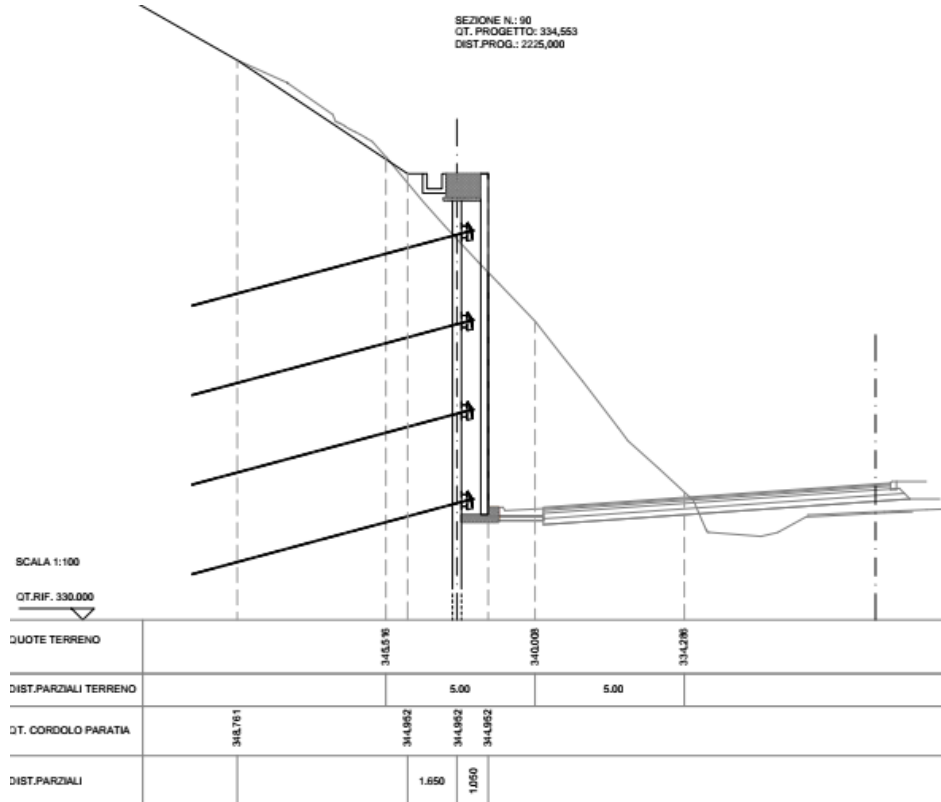
Figura 8.1 Sezione 90 tipo oggetto di verifica
