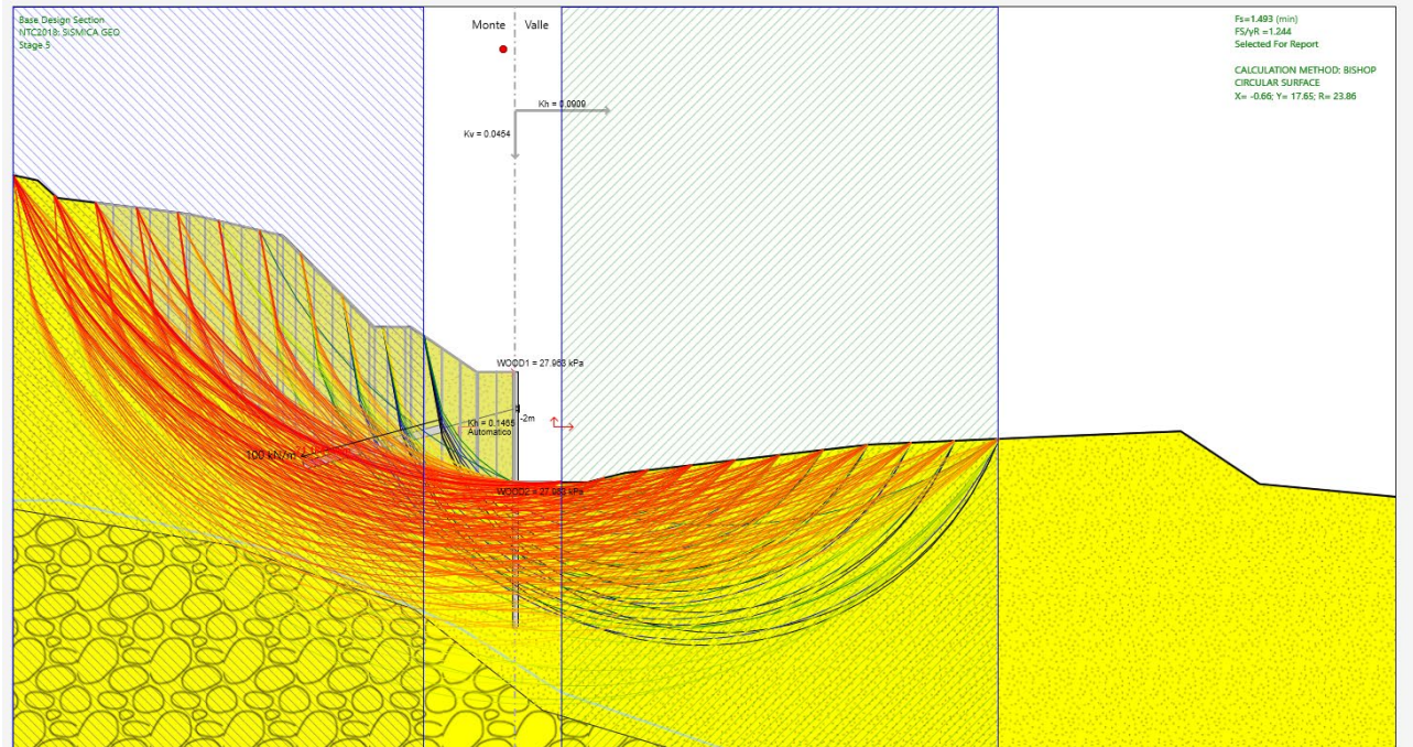
Fig. 13 – Analisi di stabilità SISMICA per il caso A2+M2+SISMA +kv
