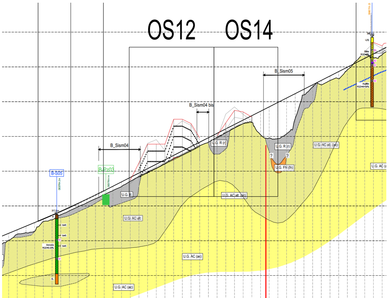
Figura 7.1 Sovrapposizione dell'opera con il profilo in asse
