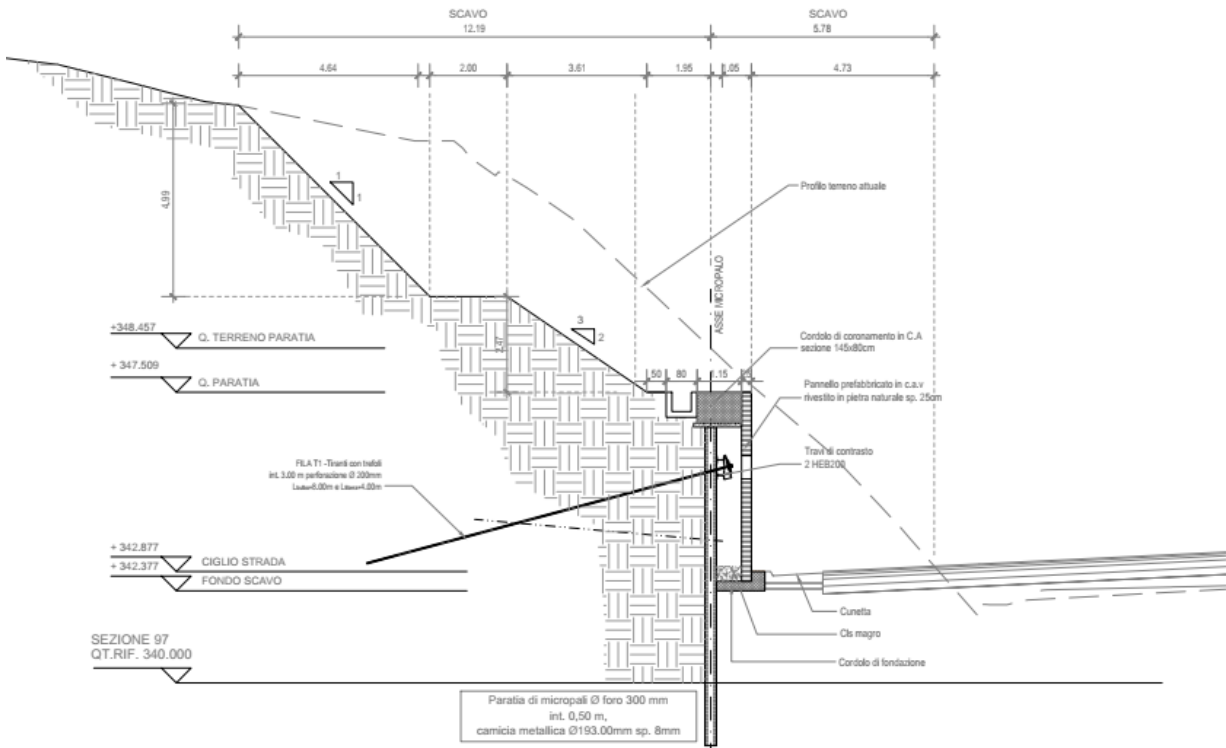
Figura 1.4 Sezioni tipo dell'opera
