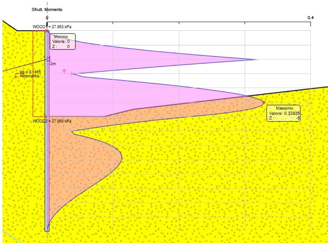
Figura 8.8 Sfruttamento a momento ENV SLU-SISMA
