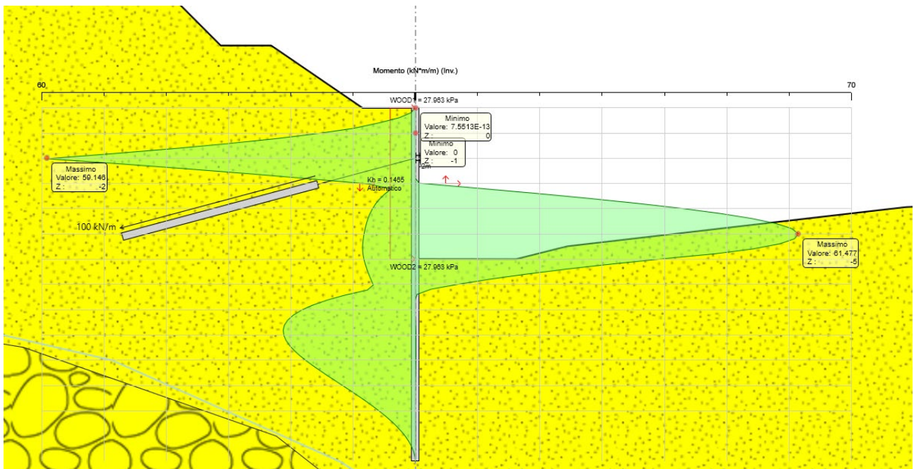
Figura 8.6 Diagramma Momento ENV SLU-SISMA
