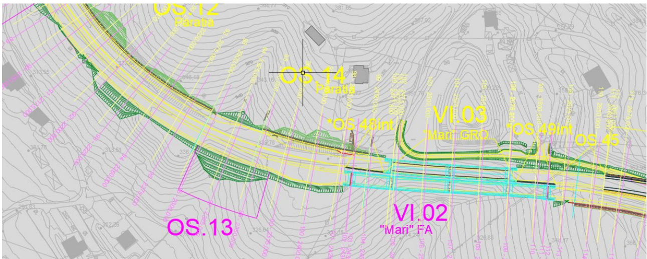
Figura 1.1 KeyPlan dell'opera
