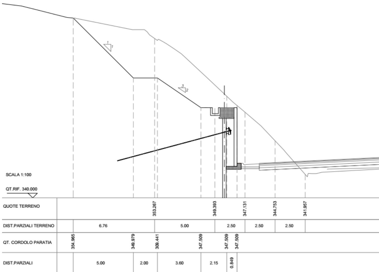
Figura 8.1 Sezione 97 tipo oggetto di verifica
