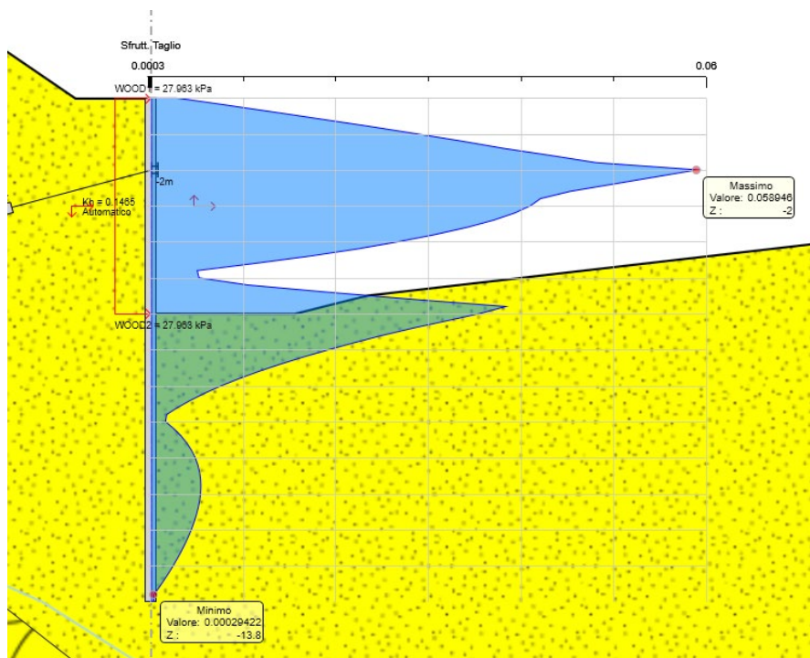
Figura 8.9 Sfruttamento a taglio ENV SLU-SISMA
