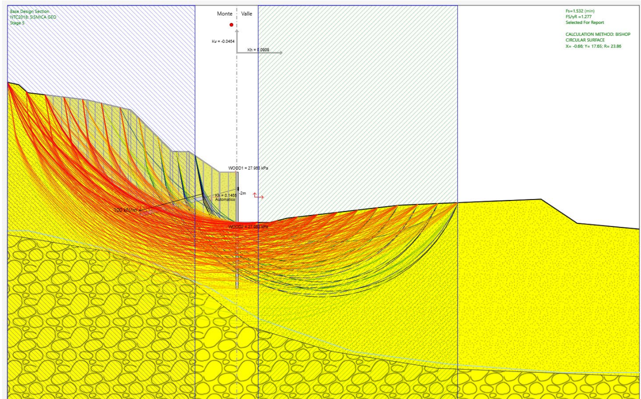
Fig. 14 – Analisi di stabilità SISMICA per il caso A2+M2+SISMA -kv
