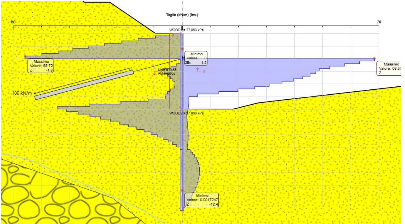
Figura 8.7 Diagramma Taglio ENV SLU-SISMA
