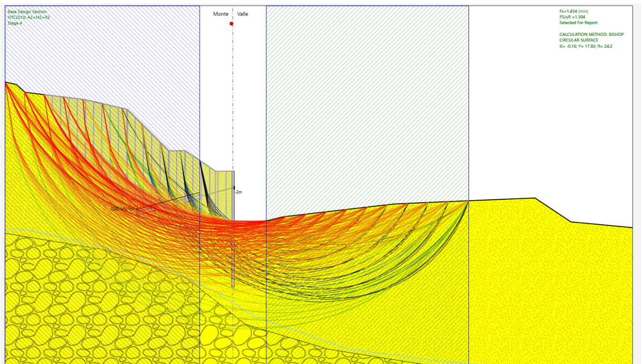
Fig. 12 – Analisi di stabilità STATICA per il caso A2+M2+R2
