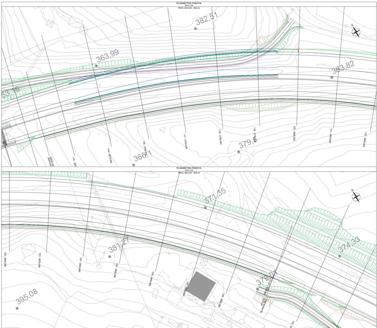
Figura 1.2 Planimetria dell'opera
