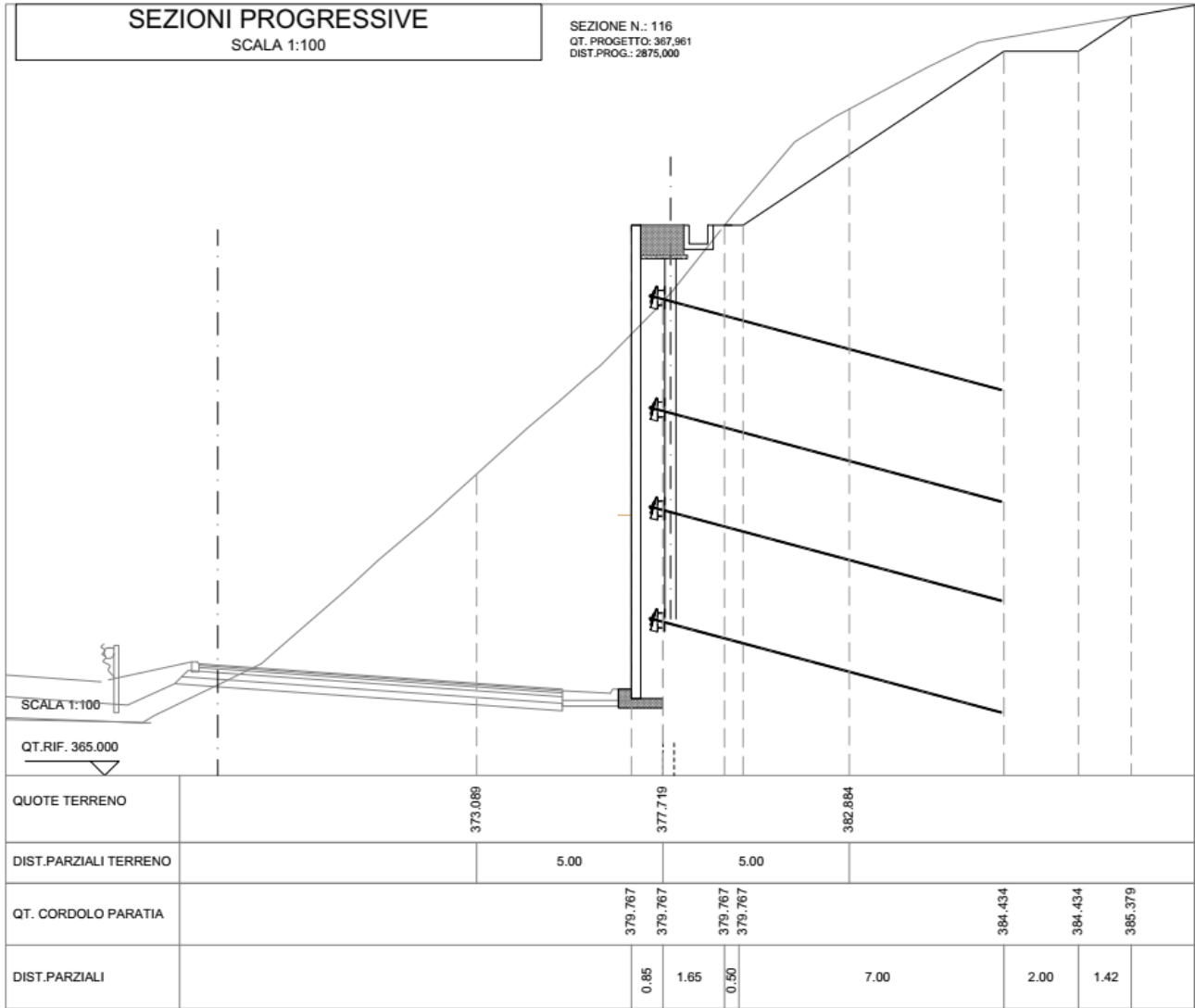
Figura 8.1 Sezione 116 tipo oggetto di verifica
