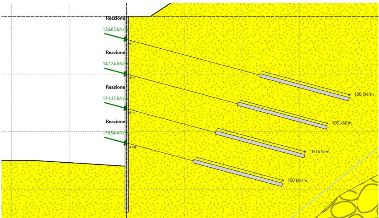
Figura 8.13 Reazioni ai supporti ENV SLU-SISMA
