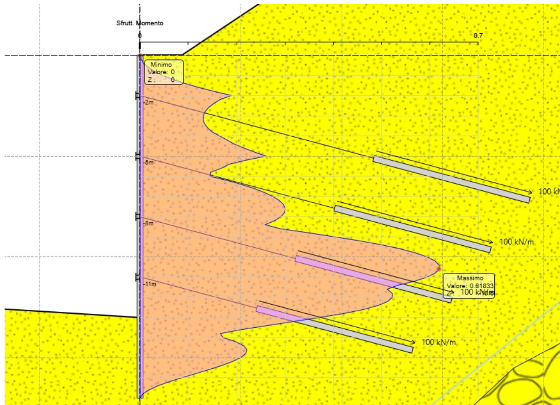
Figura 8.11 Sfruttamento a momento ENV SLU-SISMA
