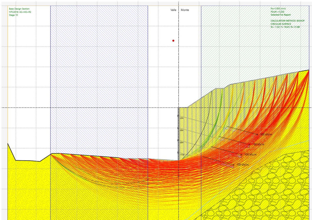
Fig. 15 – Analisi di stabilità STATICA per il caso A2+M2+R2
