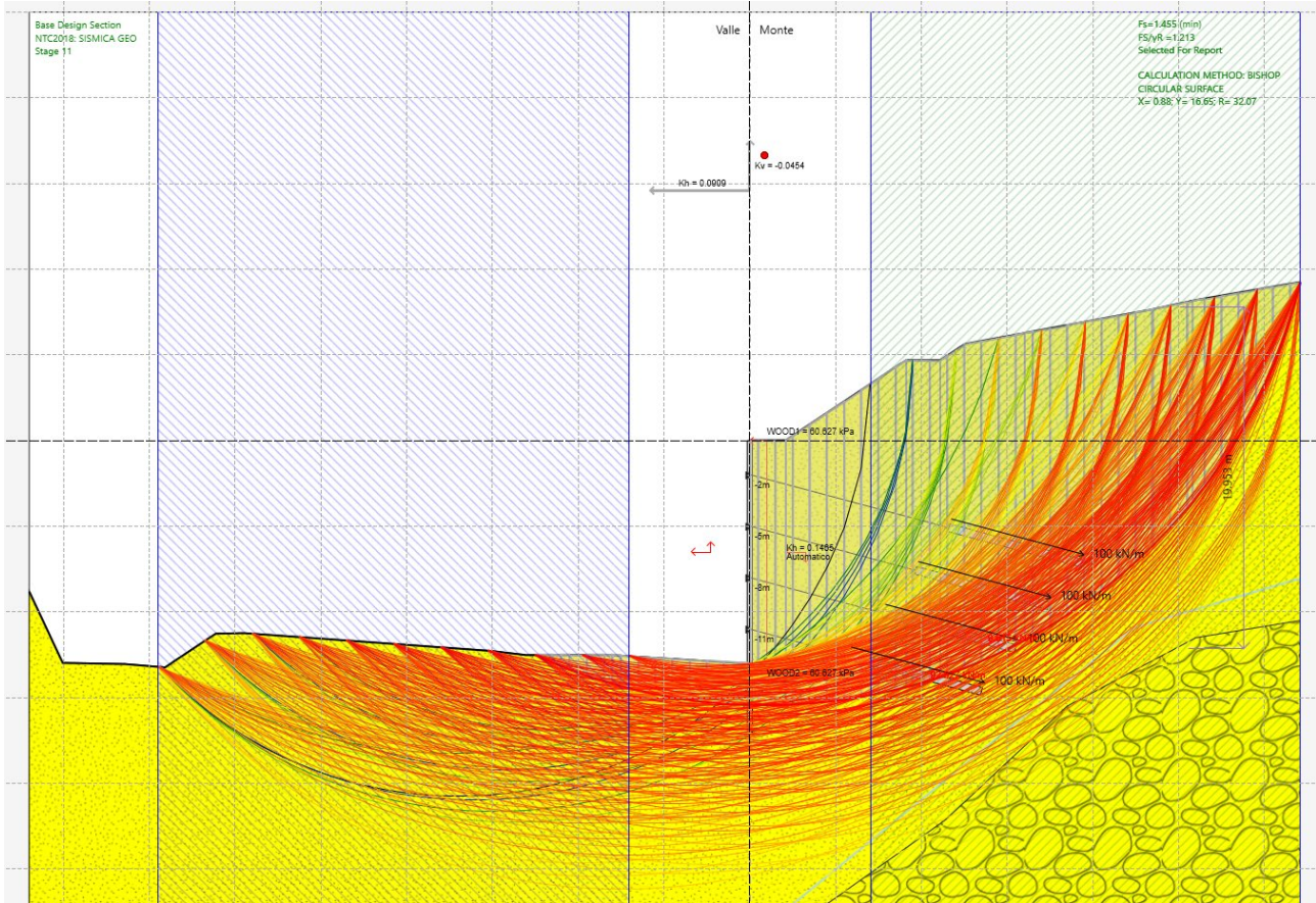
Fig. 17 – Analisi di stabilità SISMICA per il caso A2+M2+SISMA -kv
