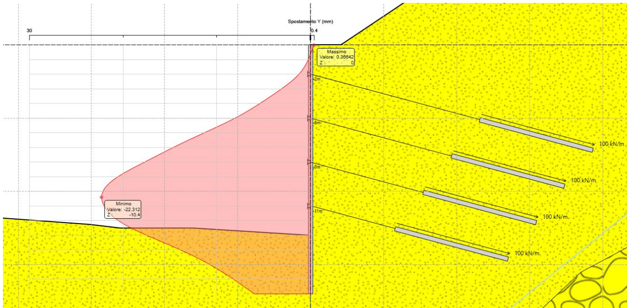
Figura 8.14 Spostamento massimo della paratia
