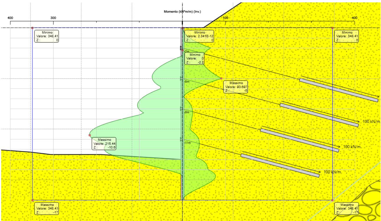
Figura 8.9 Diagramma Momento ENV SLU-SISMA
