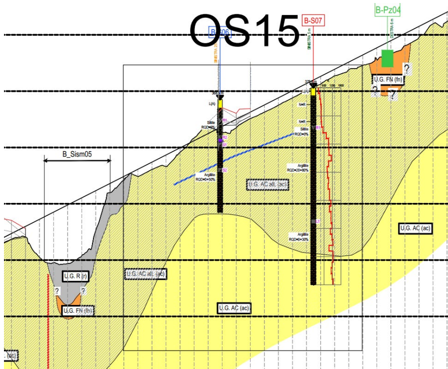
Figura 7.1 Sovrapposizione dell'opera con il profilo in asse
