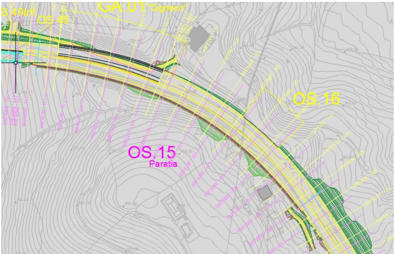
Figura 1.1 KeyPlan dell'opera
