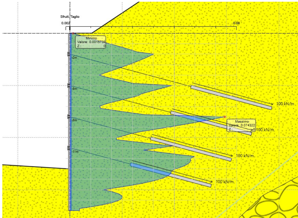
Figura 8.12 Sfruttamento a taglio ENV SLU-SISMA
