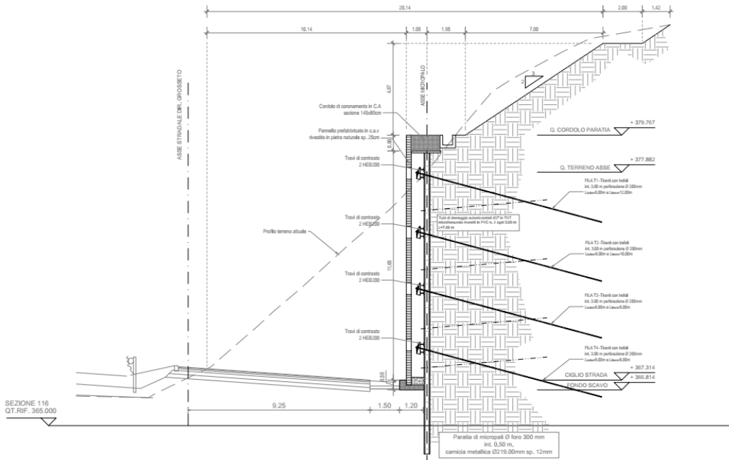
Figura 1.4 Sezioni tipo dell'opera
