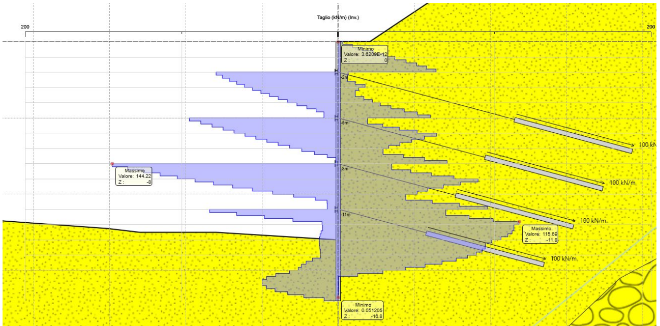
Figura 8.10 Diagramma Taglio ENV SLU-SISMA
