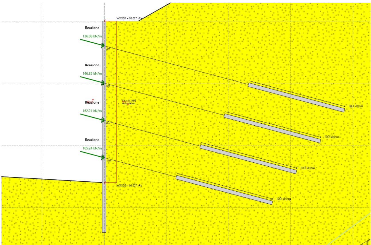
Figura 8.13 Reazioni ai supporti ENV SLU-SISMA
