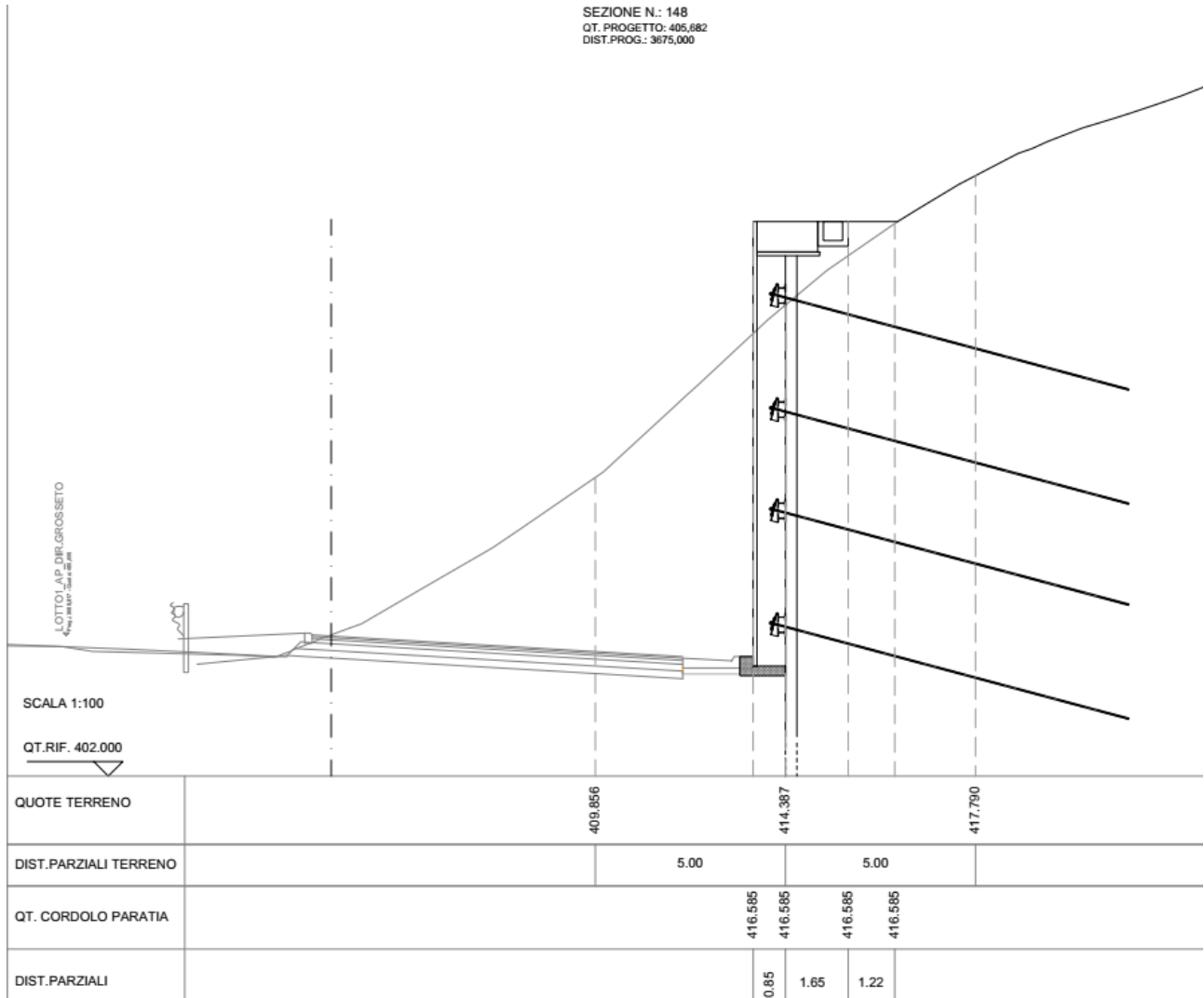
Figura 8.1 Sezione 148 tipo oggetto di verifica
