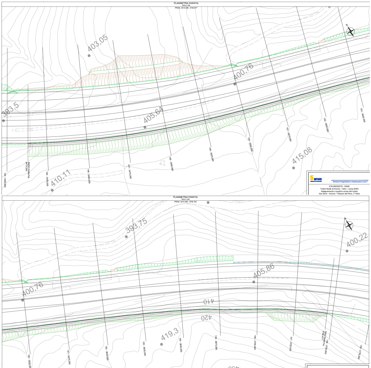
Figura 1.2 Planimetria dell'opera
