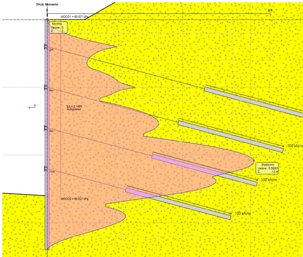
Figura 8.11 Sfruttamento a momento ENV SLU-SISMA
