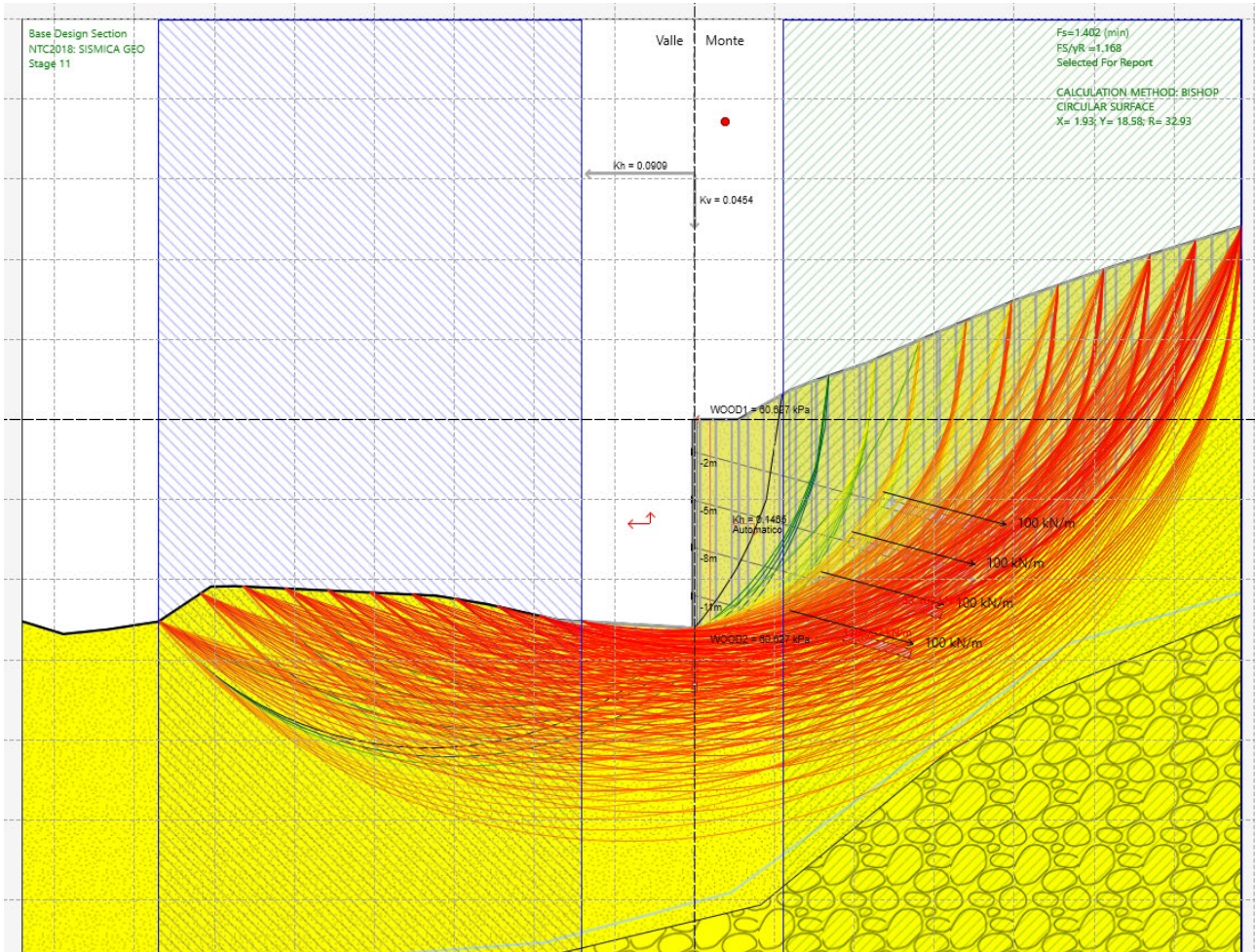
Fig. 16 – Analisi di stabilità SISMICA per il caso A2+M2+SISMA +kv
