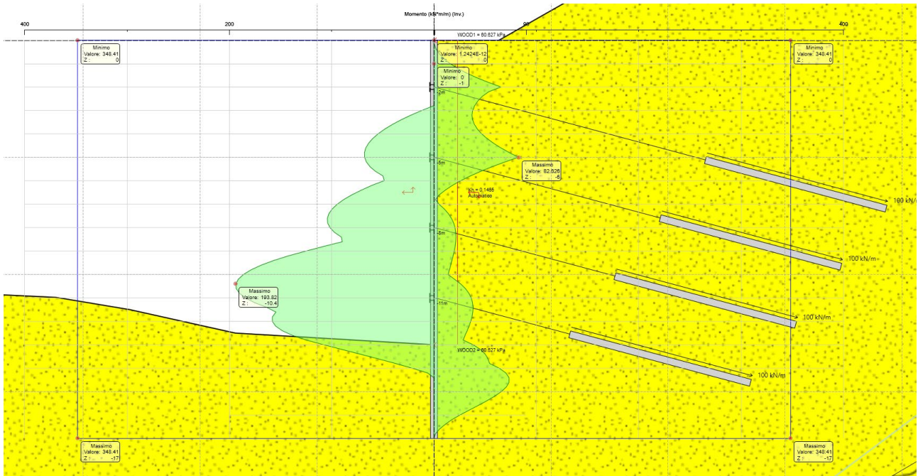
Figura 8.9 Diagramma Momento ENV SLU-SISMA
