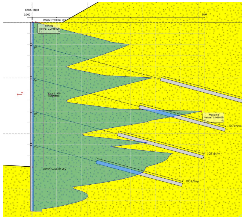
Figura 8.12 Sfruttamento a taglio ENV SLU-SISMA
