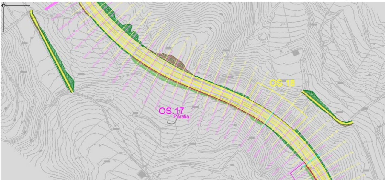
Figura 1.1 KeyPlan dell'opera
