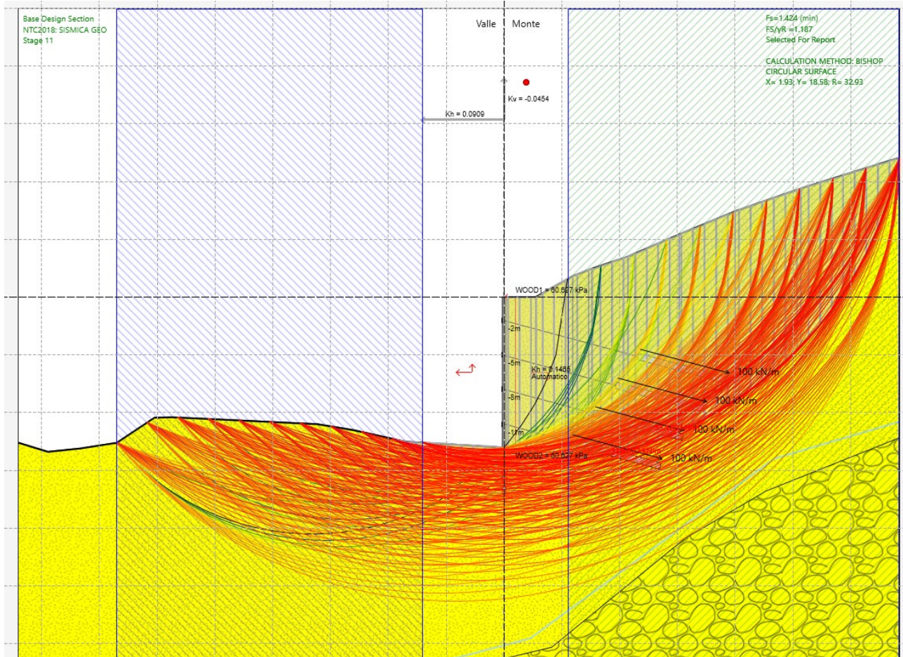
Fig. 17 – Analisi di stabilità SISMICA per il caso A2+M2+SISMA -kv
