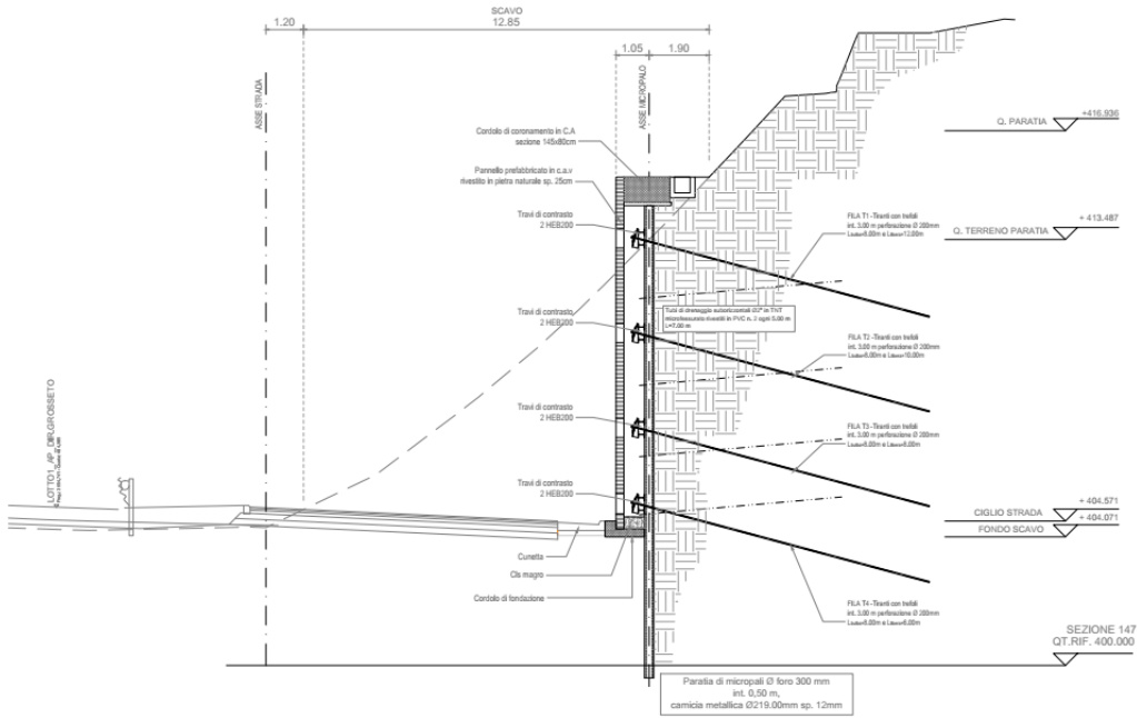
Figura 1.4 Sezioni tipo dell'opera
