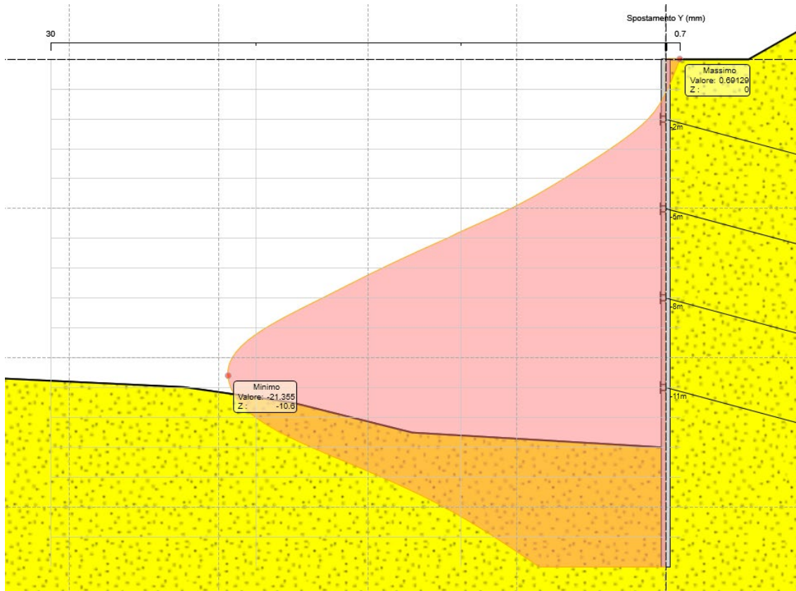
Figura 8.14 Spostamento massimo della paratia
