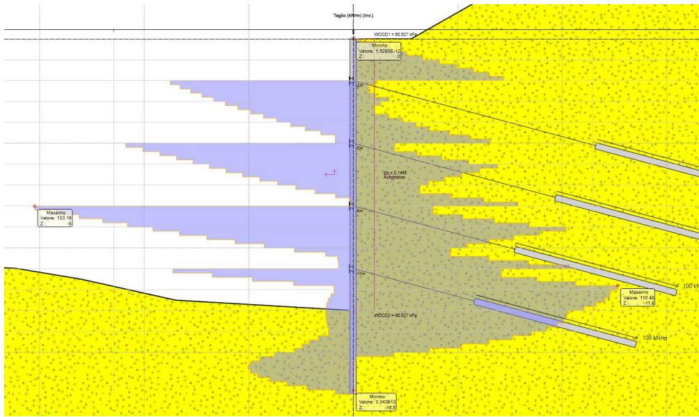
Figura 8.10 Diagramma Taglio ENV SLU-SISMA
