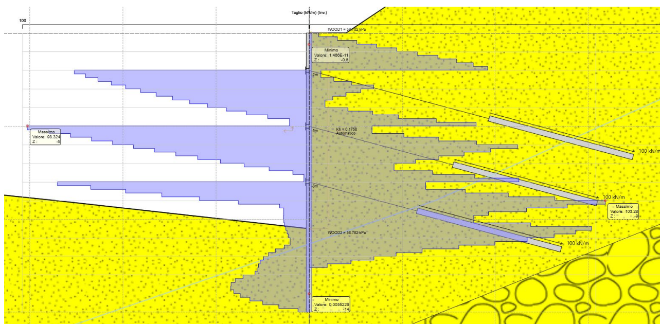
Figura 8.9 Diagramma Taglio ENV SLU-SISMA
