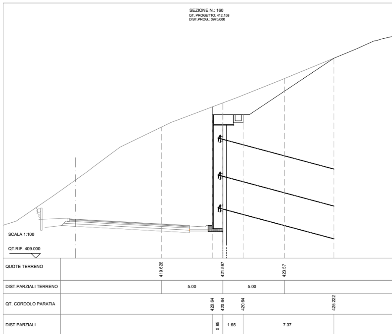
Figura 8.1 Sezione 160 tipo oggetto di verifica
