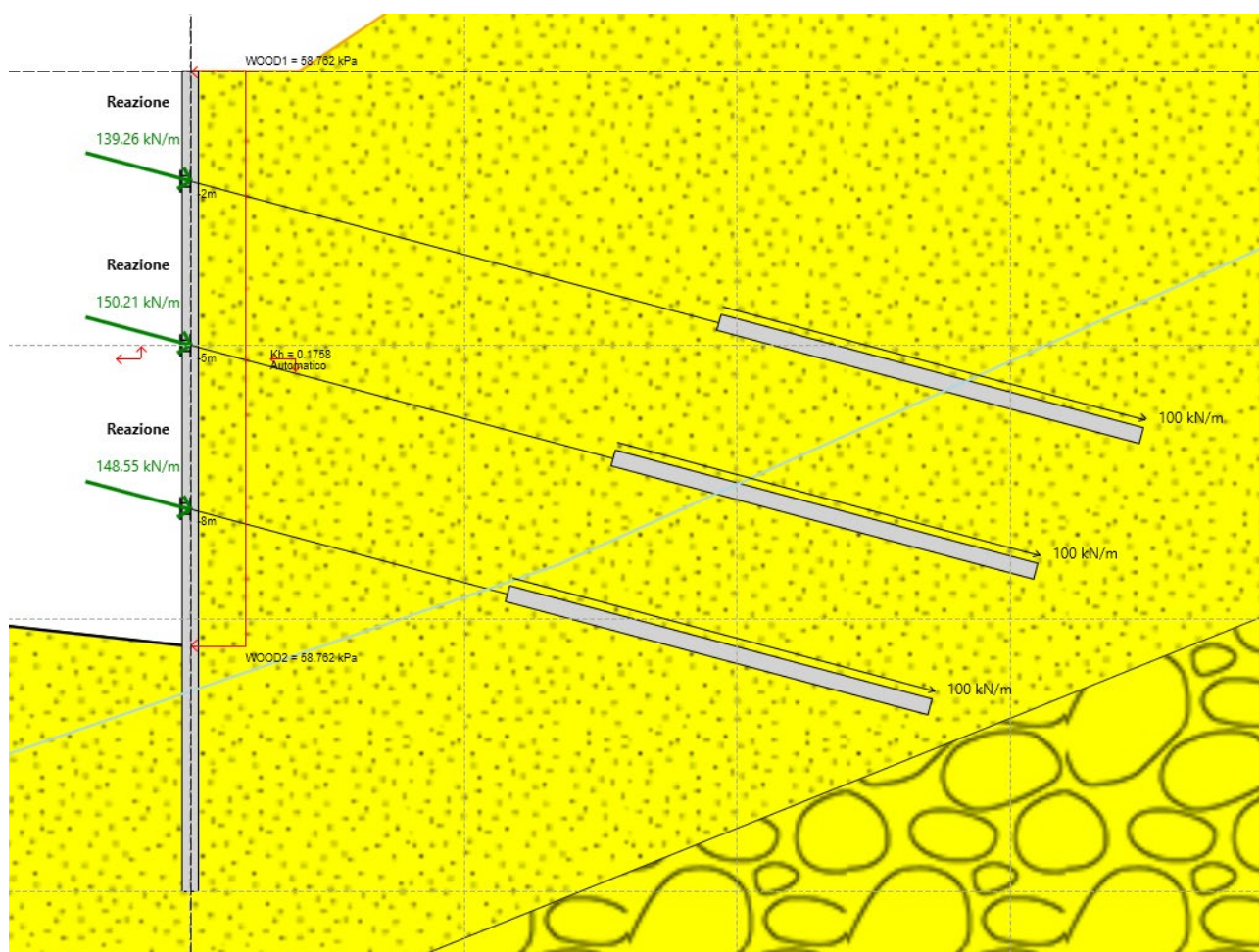
Figura 8.12 Reazioni ai supporti ENV SLU-SISMA
