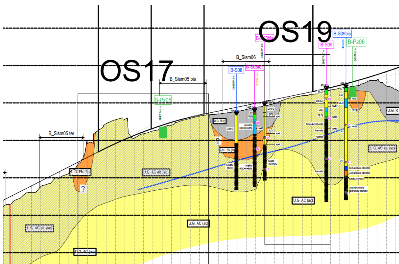
Figura 7.1 Sovrapposizione dell'opera con il profilo in asse
