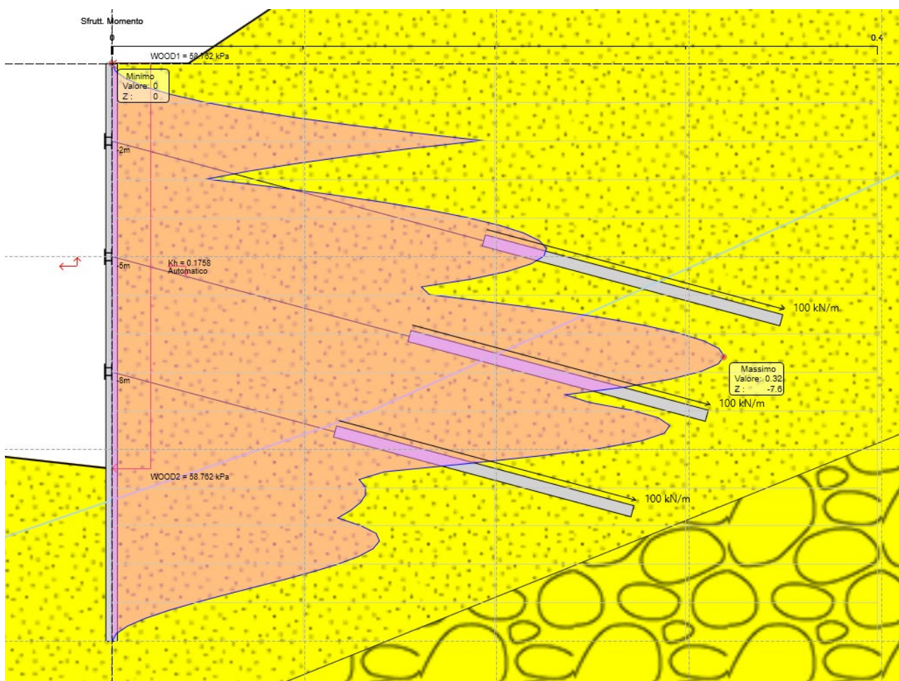
Figura 8.10 Sfruttamento a momento ENV SLU-SISMA
