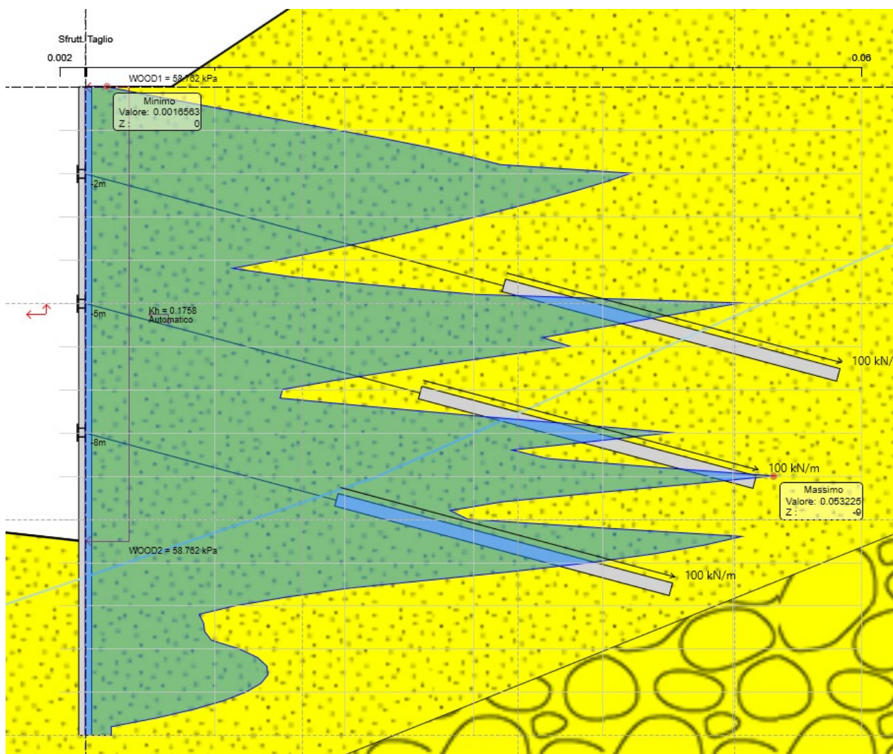
Figura 8.11 Sfruttamento a taglio ENV SLU-SISMA
