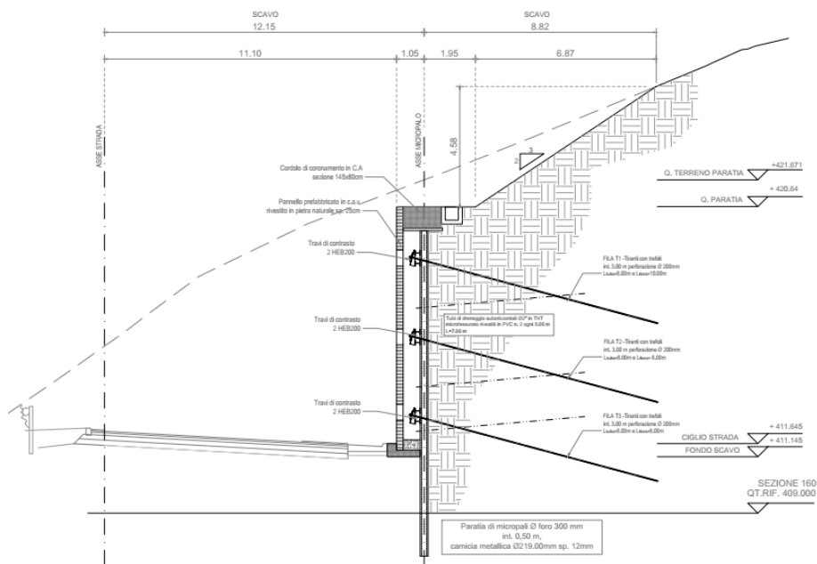
Figura 1.4 Sezioni tipo dell'opera
