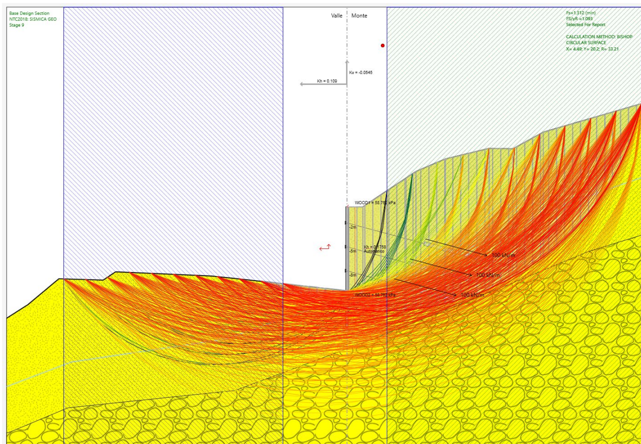
Fig. 16 – Analisi di stabilità SISMICA per il caso A2+M2+SISMA -kv
