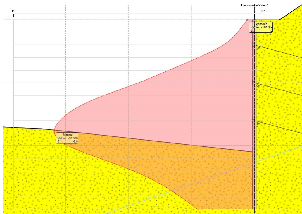
Figura 8.13 Spostamento massimo della paratia
