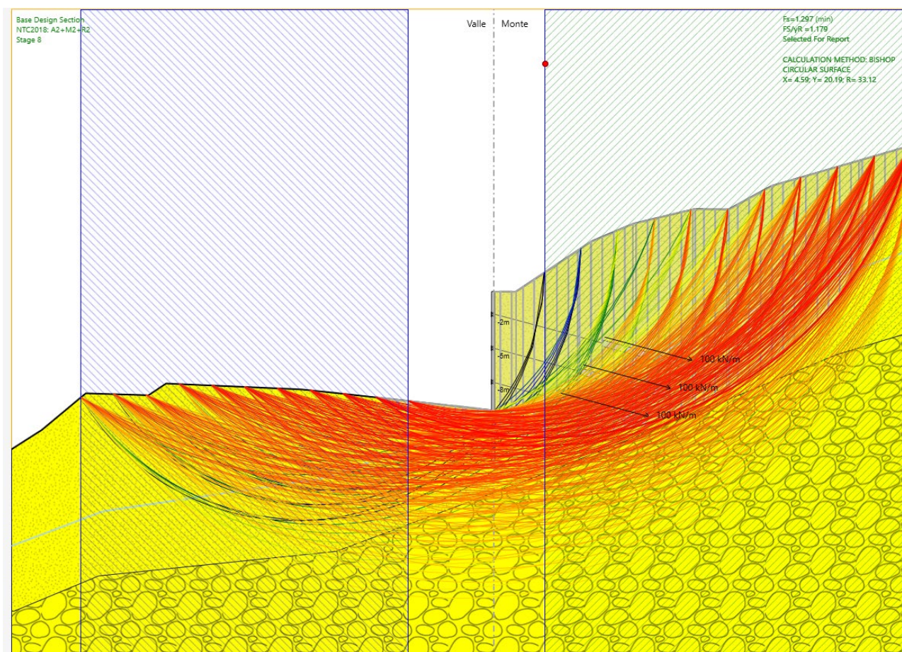
Fig. 14 – Analisi di stabilità STATICA per il caso A2+M2+R2
