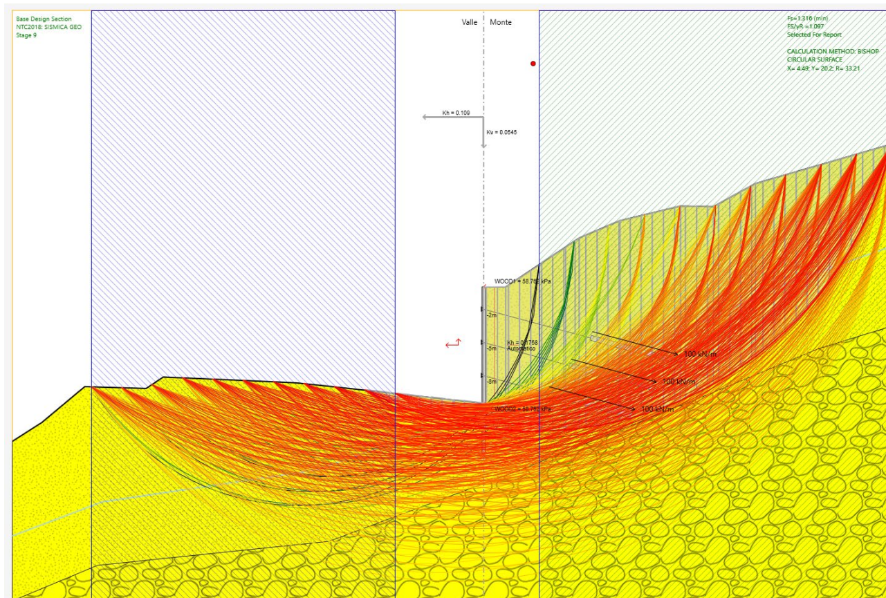
Fig. 15 – Analisi di stabilità SISMICA per il caso A2+M2+SISMA +kv
