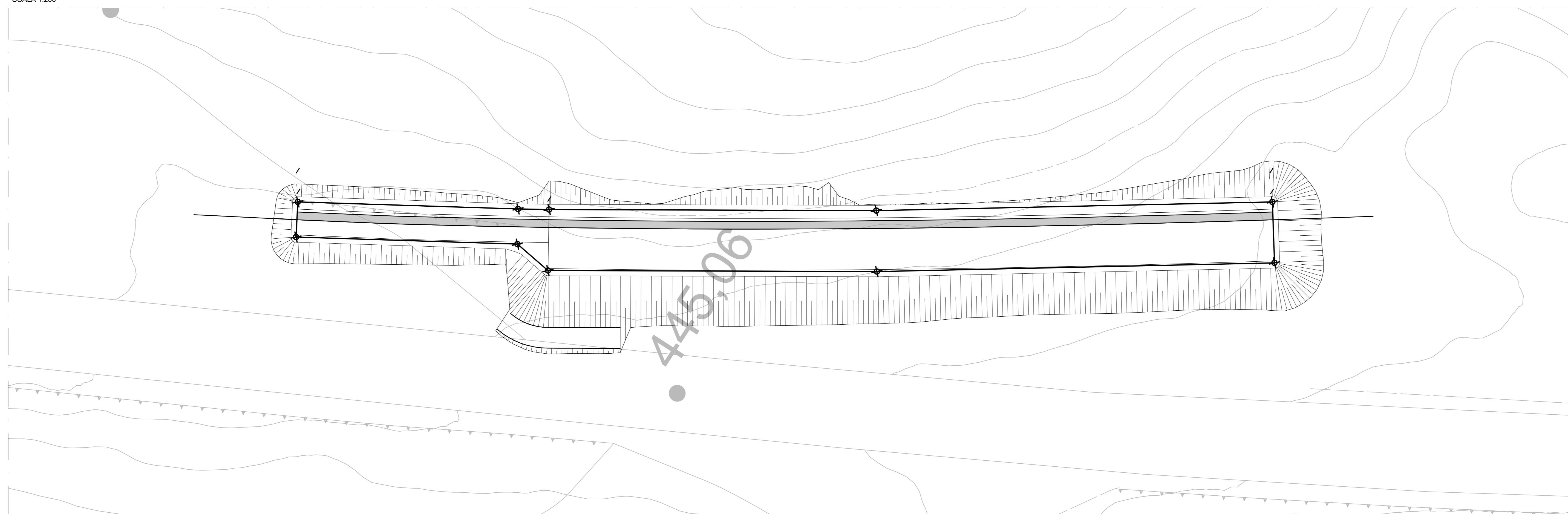
VISTA PLANIMETRICA MURO OS23 SCALA 1:200
