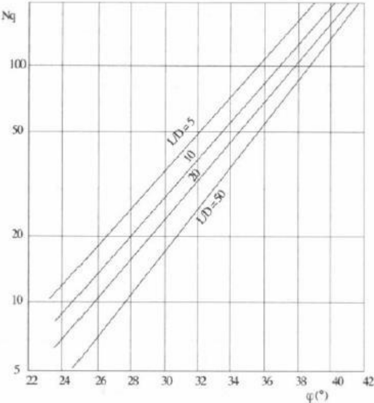
Figura 9 Valori di Nq secondo Berezantzev (1961)
