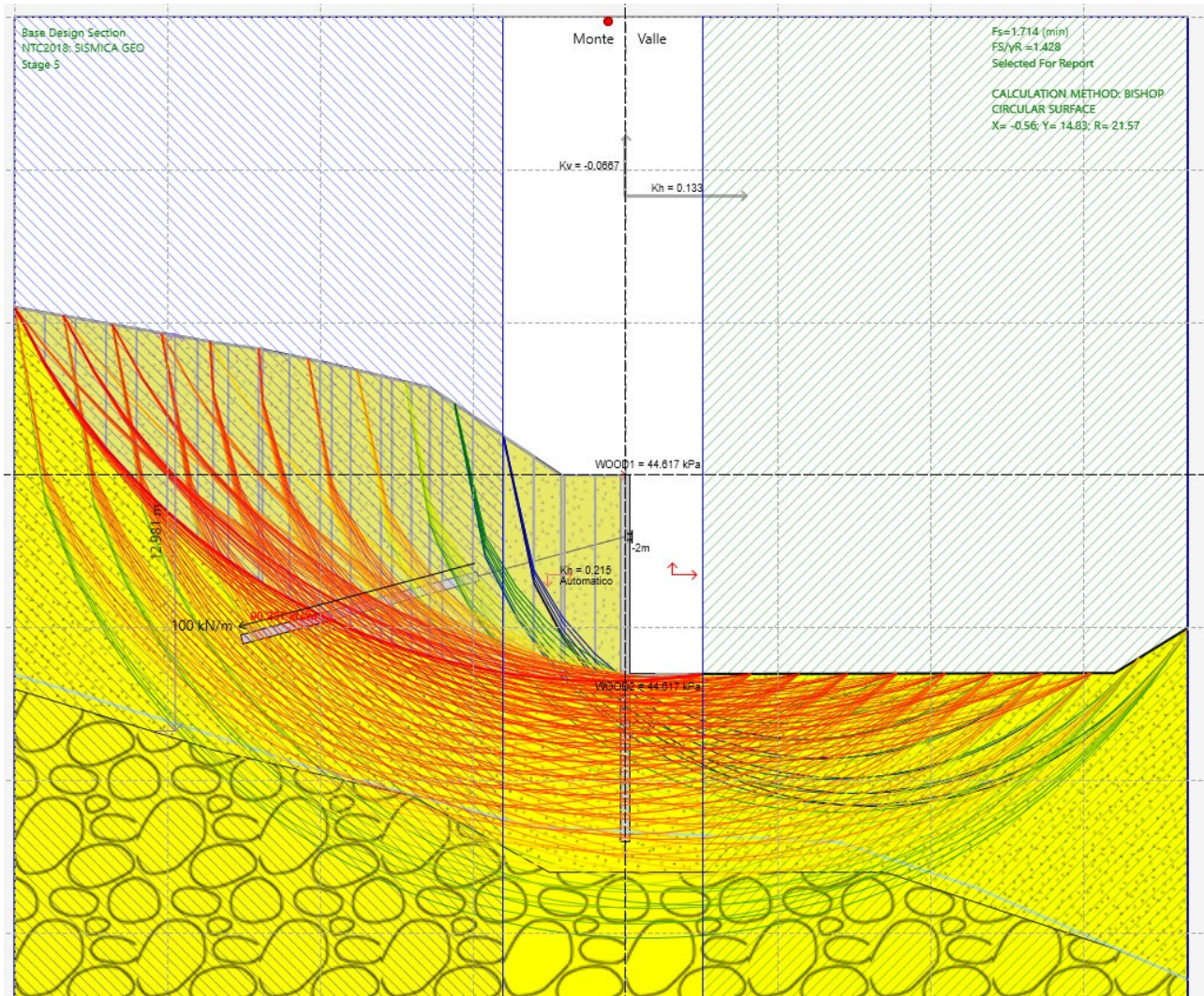
Fig. 14 – Analisi di stabilità SISMICA per il caso A2+M2+SISMA -kv
