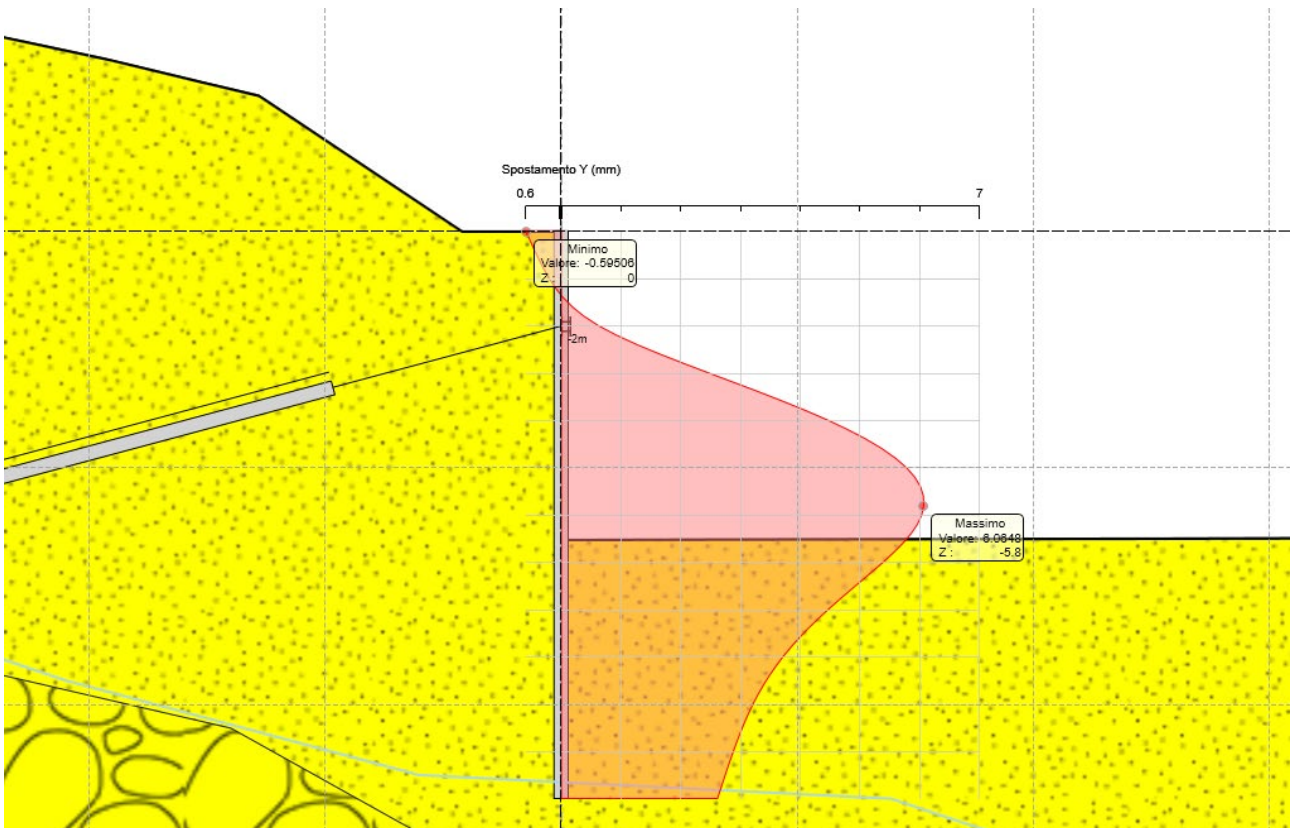
Figura 8.11 Spostamento massimo della paratia
