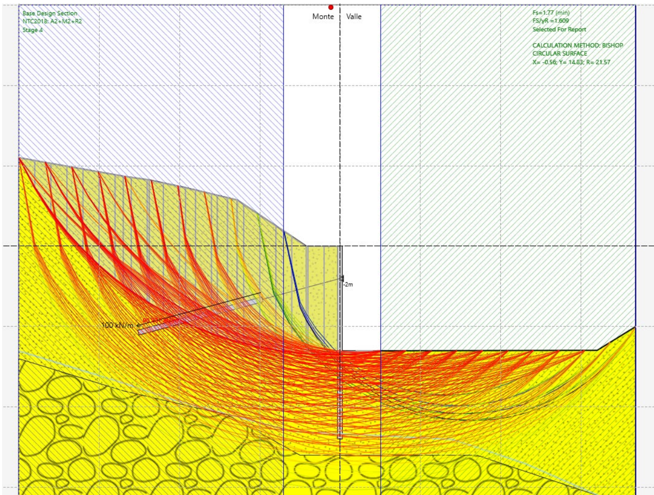
Fig. 12 – Analisi di stabilità STATICA per il caso A2+M2+R2
