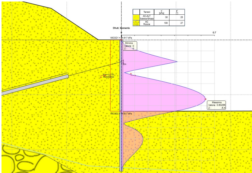
Figura 8.8 Sfruttamento a momento ENV SLU-SISMA
