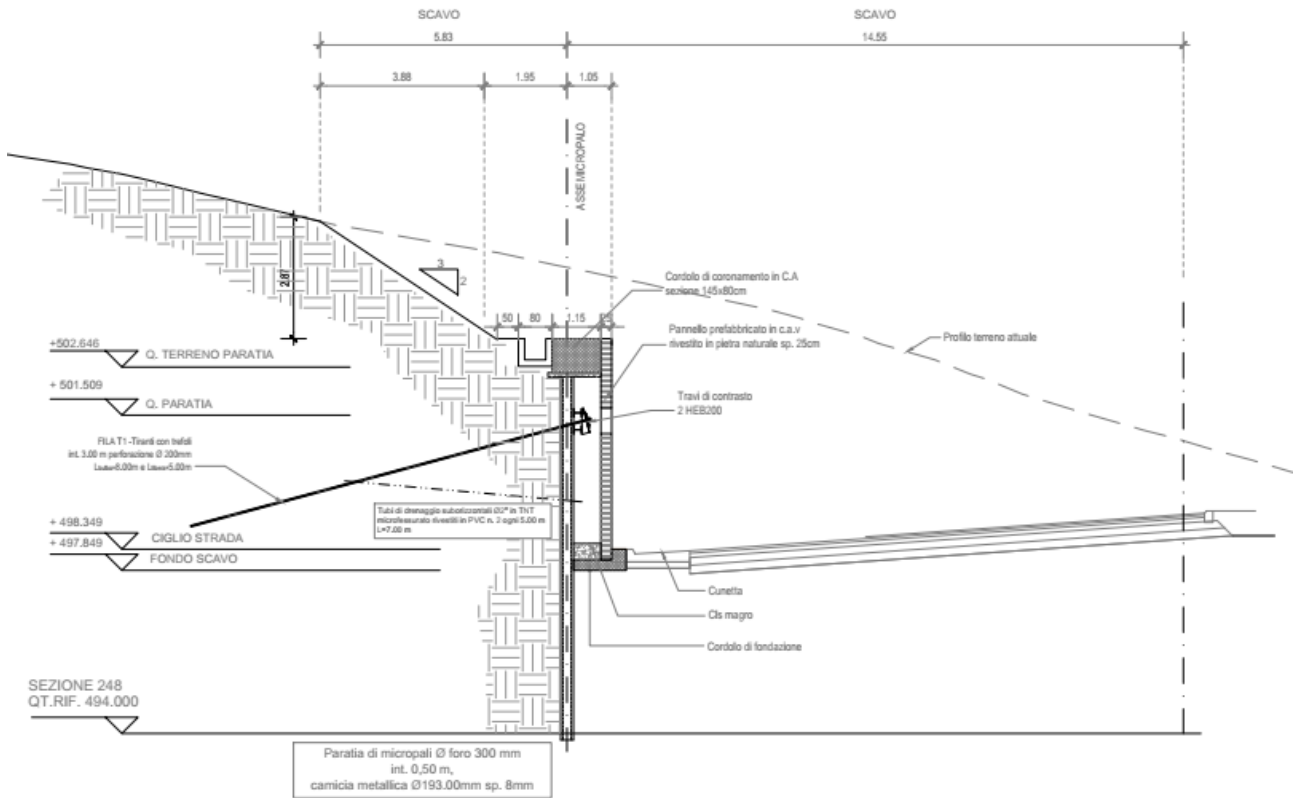
Figura 1.4 Sezioni tipo dell'opera
