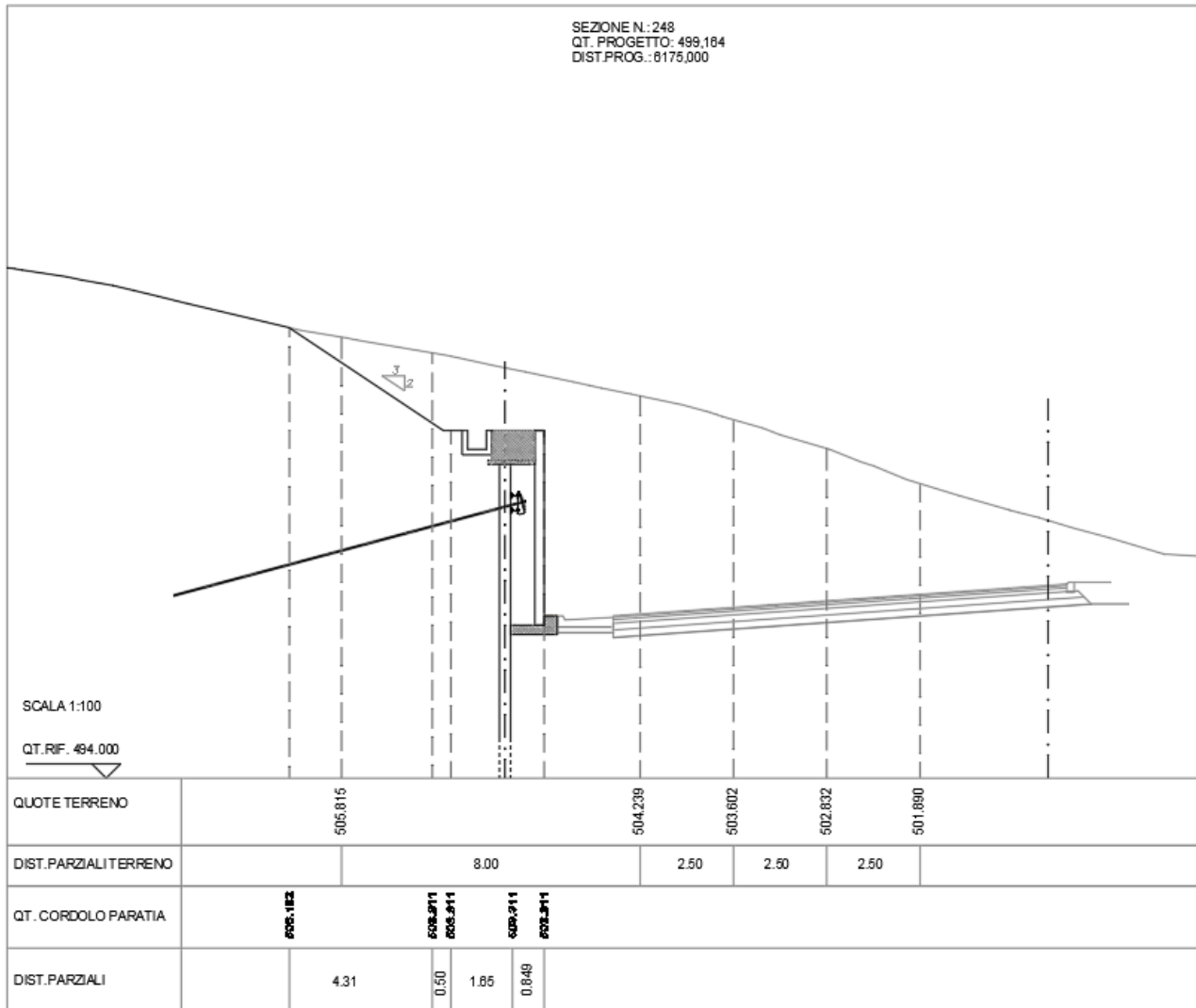
Figura 8.1 Sezione 248 tipo oggetto di verifica
