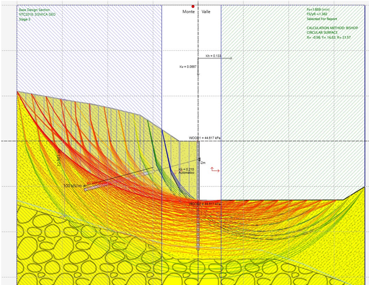
Fig. 13 – Analisi di stabilità SISMICA per il caso A2+M2+SISMA +kv
