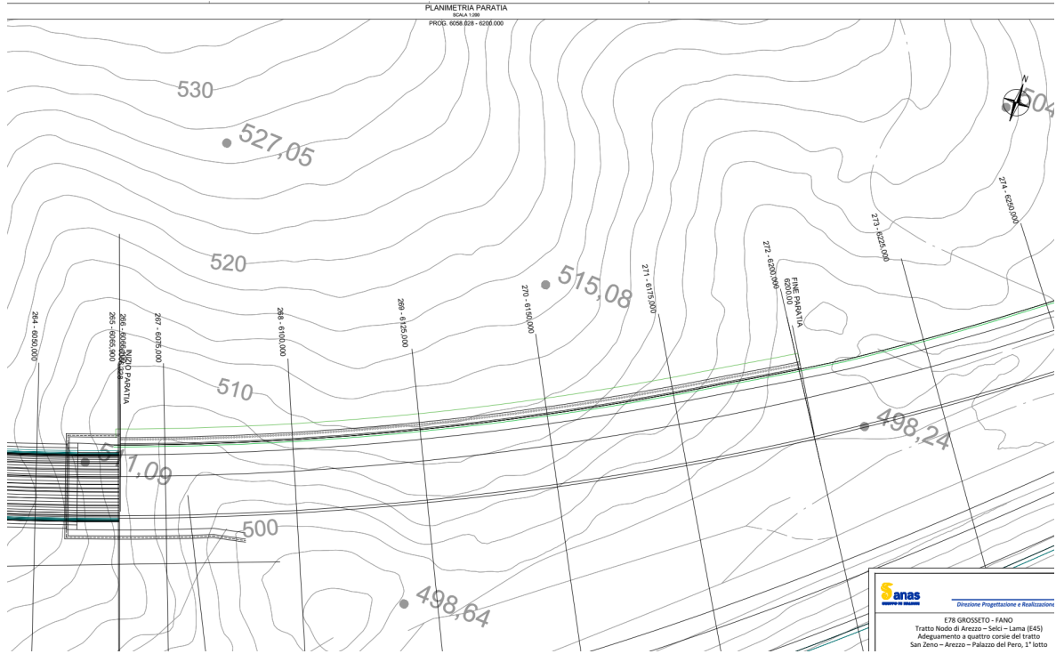
Figura 1.2 Planimetria dell'opera
