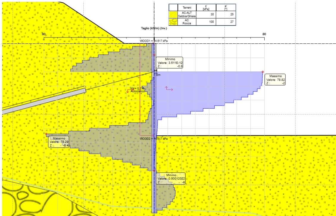
Figura 8.7 Diagramma Taglio ENV SLU-SISMA
