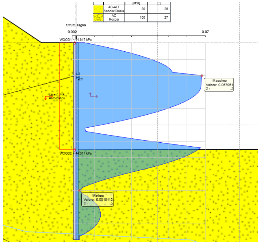
Figura 8.9 Sfruttamento a taglio ENV SLU-SISMA
