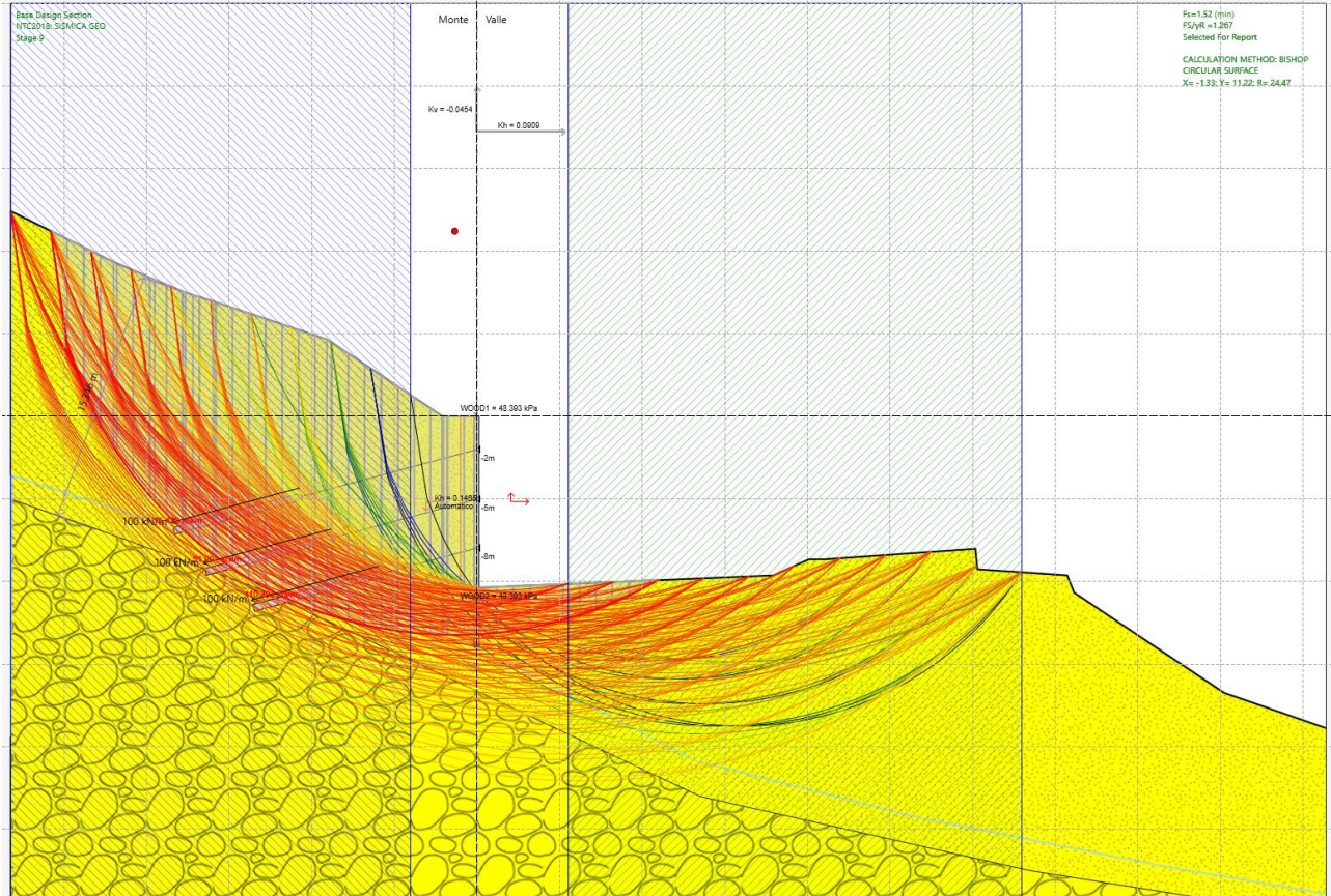
Fig. 16 – Analisi di stabilità SISMICA per il caso A2+M2+SISMA -kv
