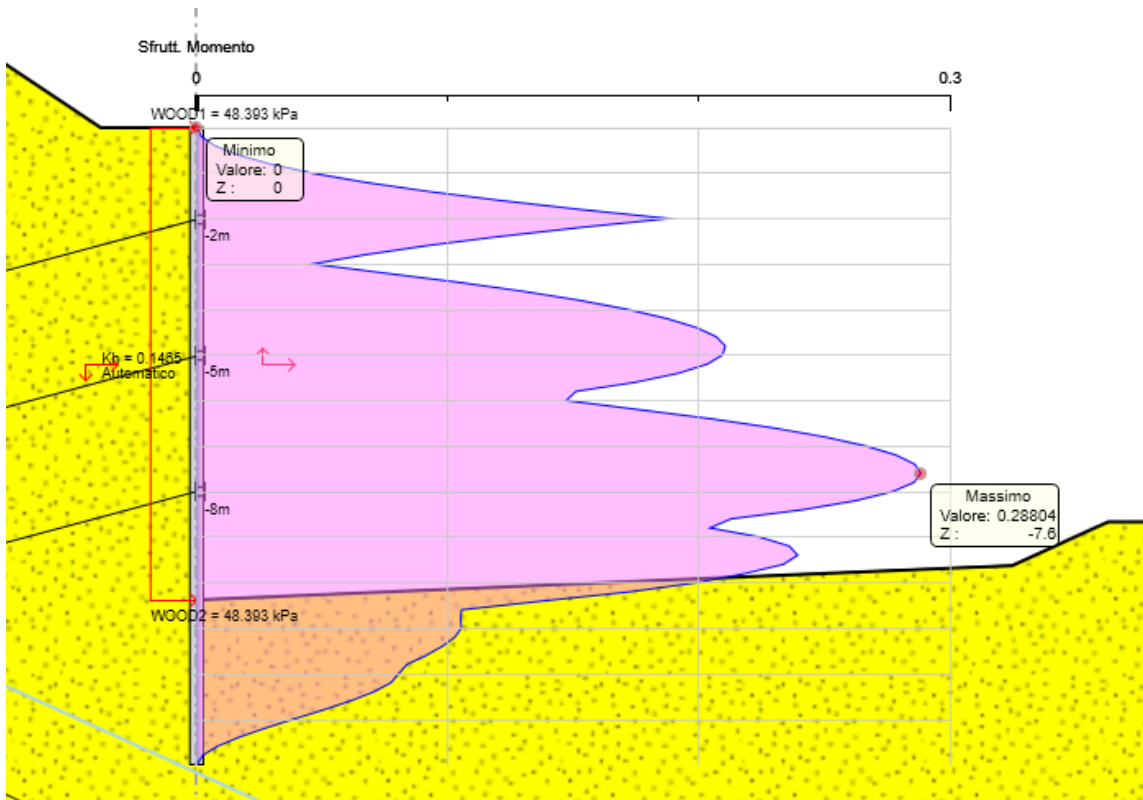
Figura 8.10 Sfruttamento a momento ENV SLU-SISMA
