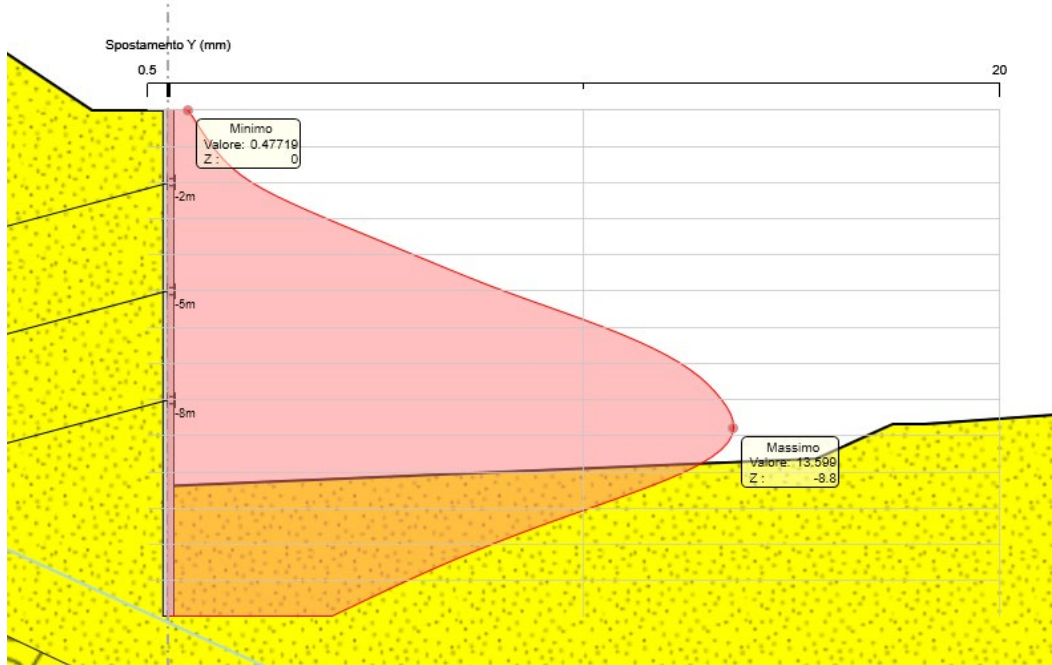
Figura 8.13 Spostamento massimo della paratia
