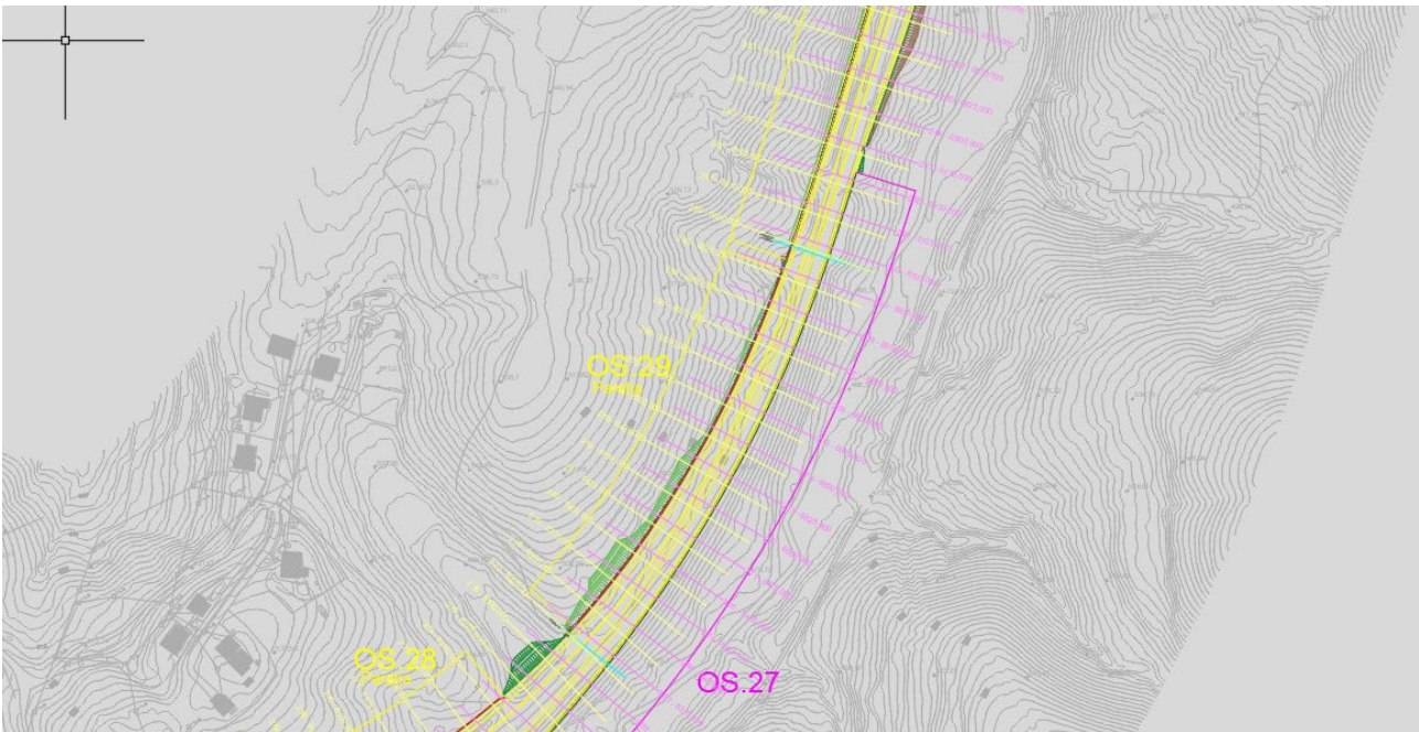
Figura 1.1 KeyPlan dell'opera
