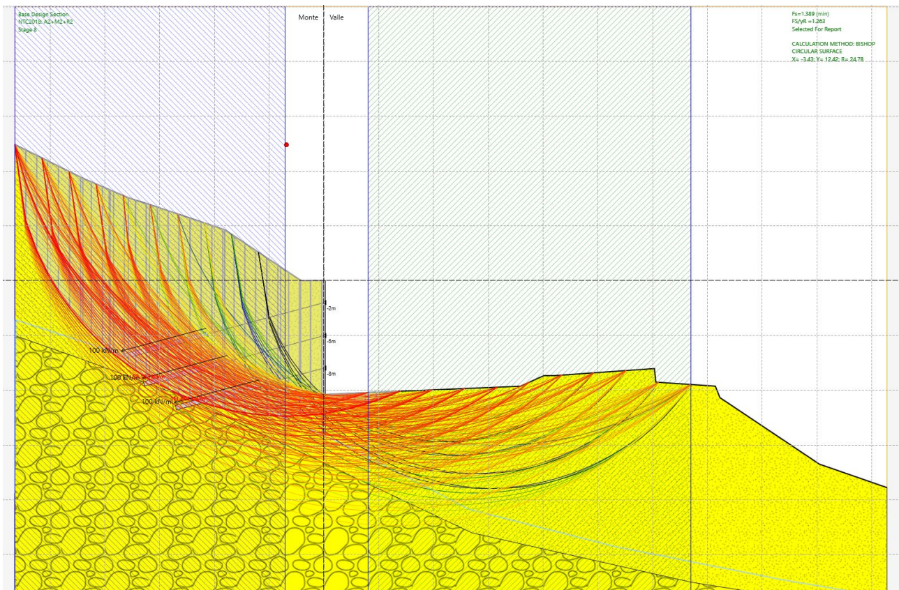
Fig. 14 – Analisi di stabilità STATICA per il caso A2+M2+R2
