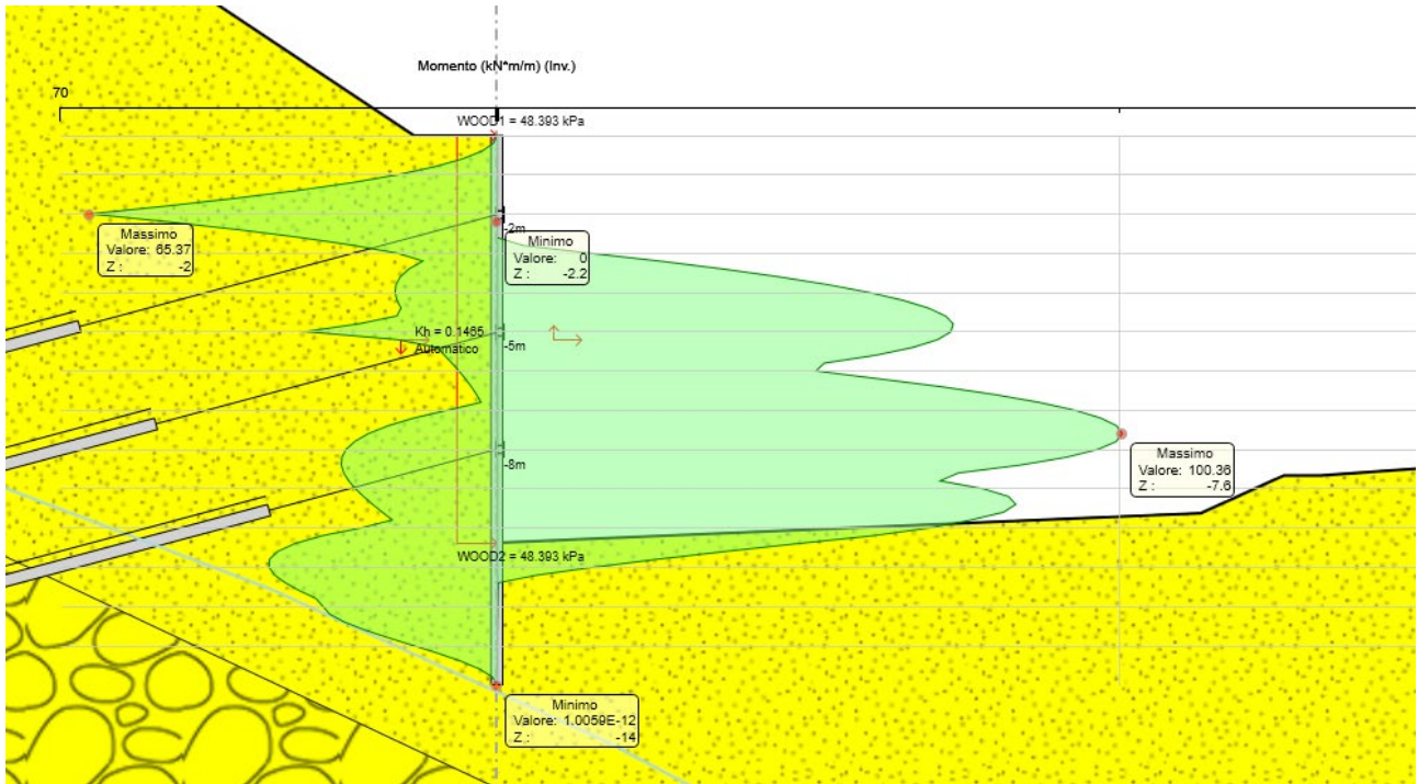
Figura 8.8 Diagramma Momento ENV SLU-SISMA
