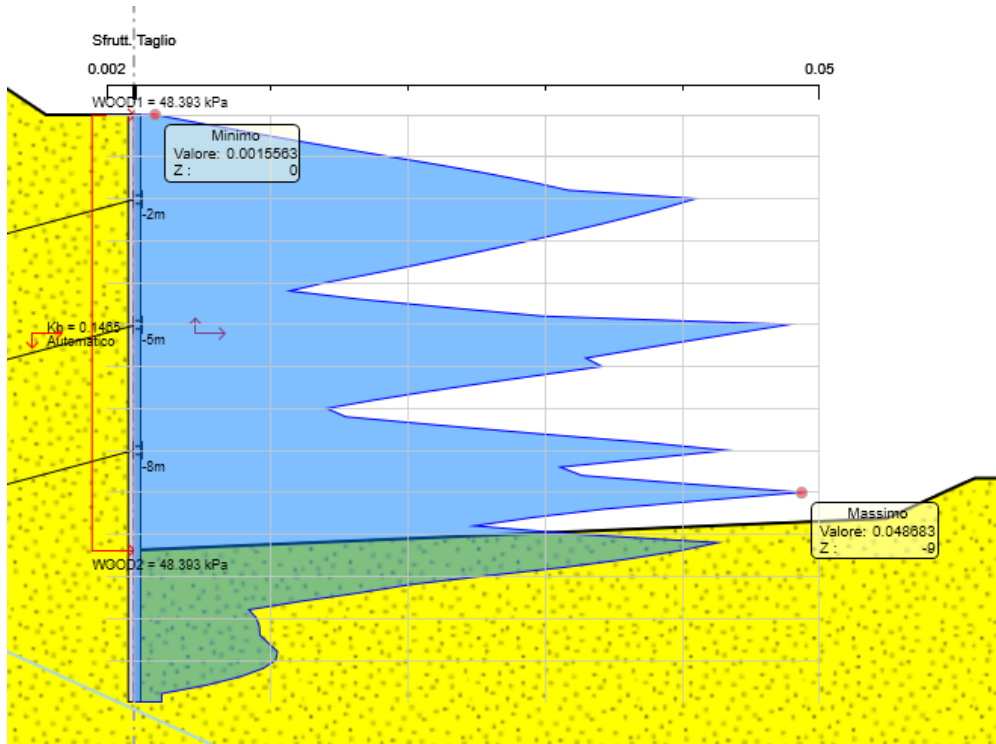
Figura 8.11 Sfruttamento a taglio ENV SLU-SISMA
