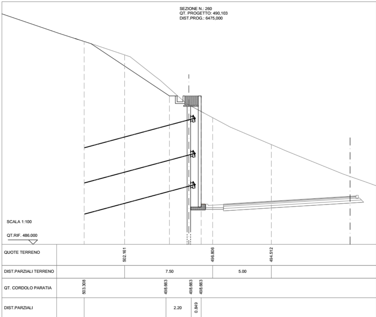
Figura 8.1 Sezione 97 tipo oggetto di verifica
