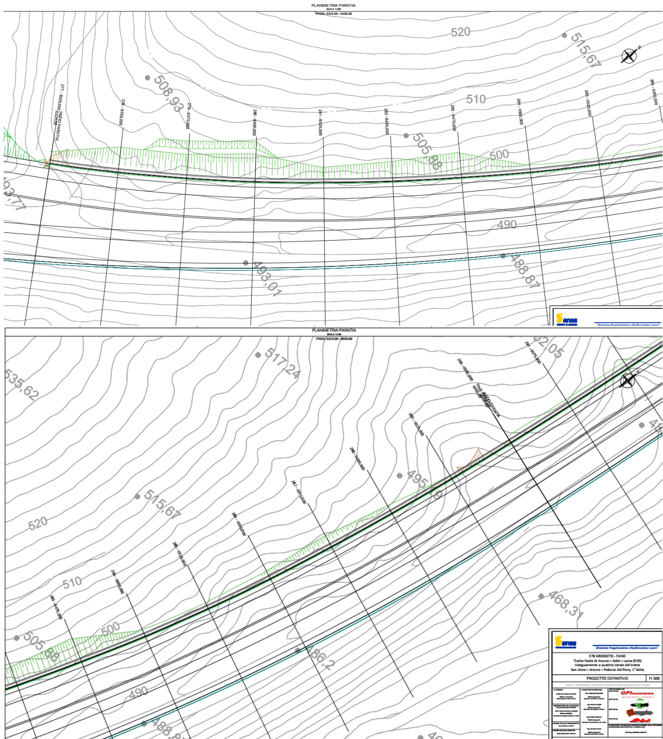
Figura 1.2 Planimetria dell'opera
