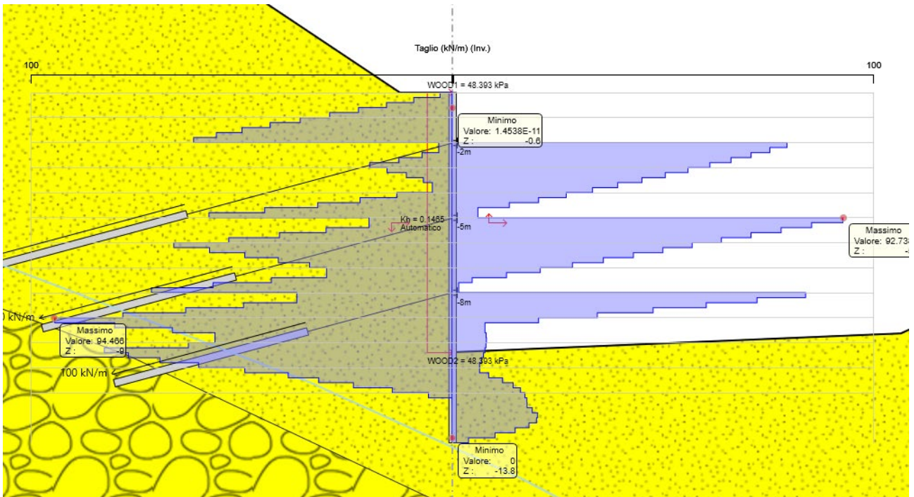
Figura 8.9 Diagramma Taglio ENV SLU-SISMA
