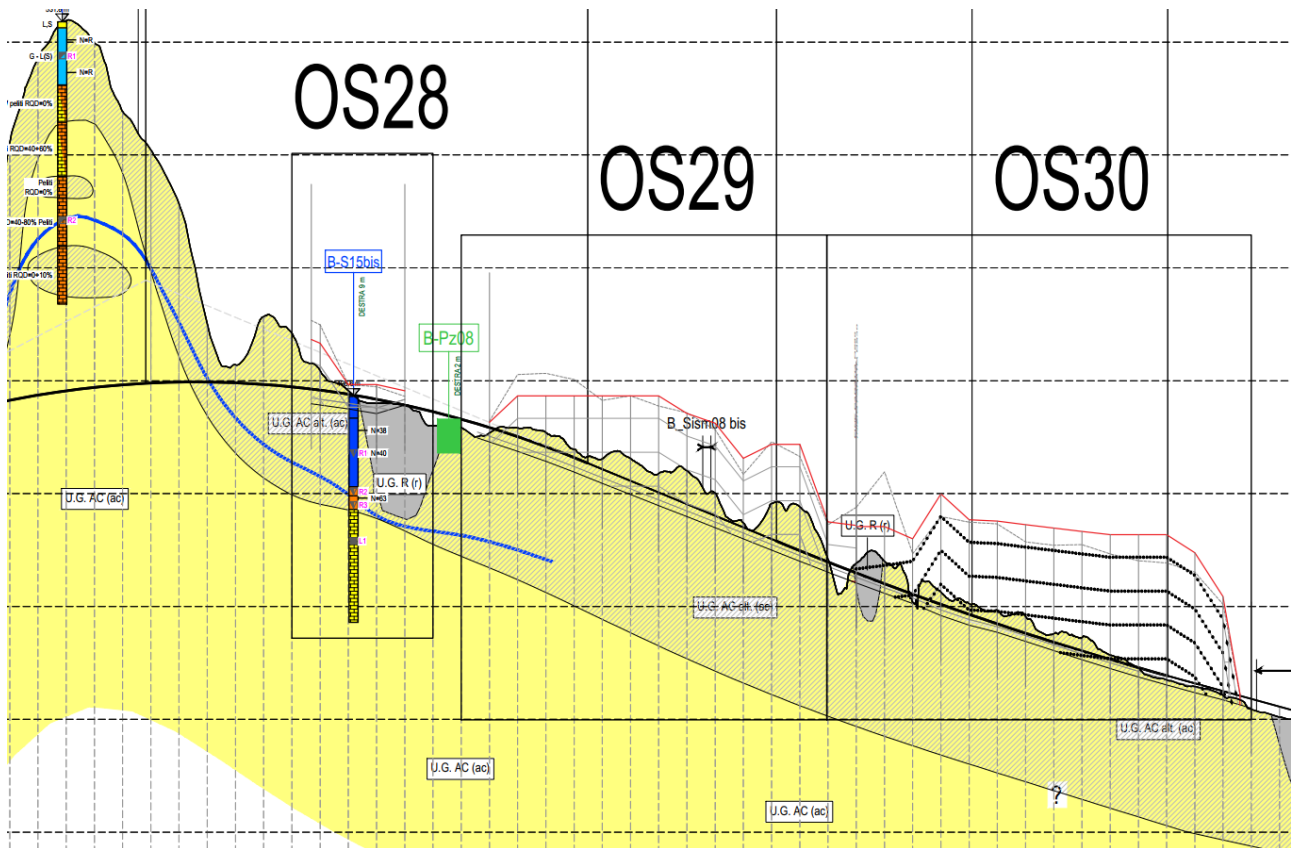
Figura 7.1 Sovrapposizione dell'opera con il profilo in asse
