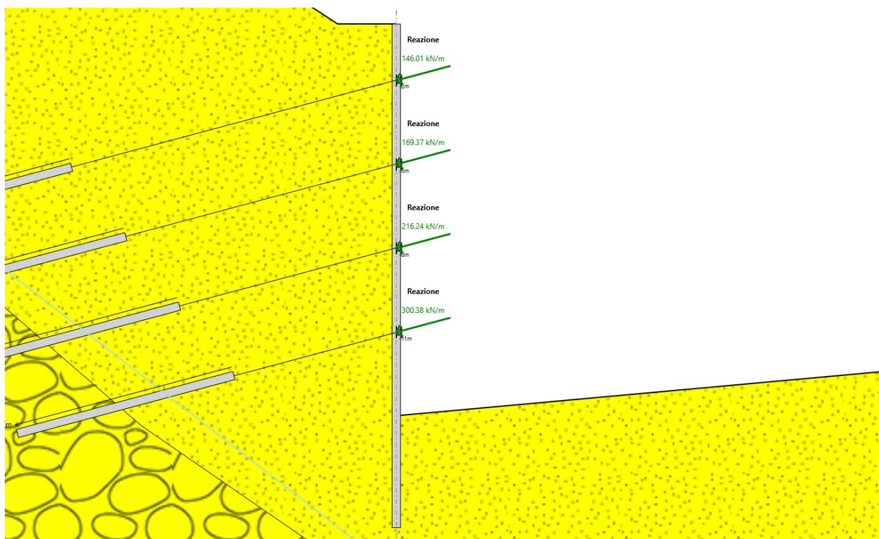
Figura 8.13 Reazioni ai supporti ENV SLU-SISMA
