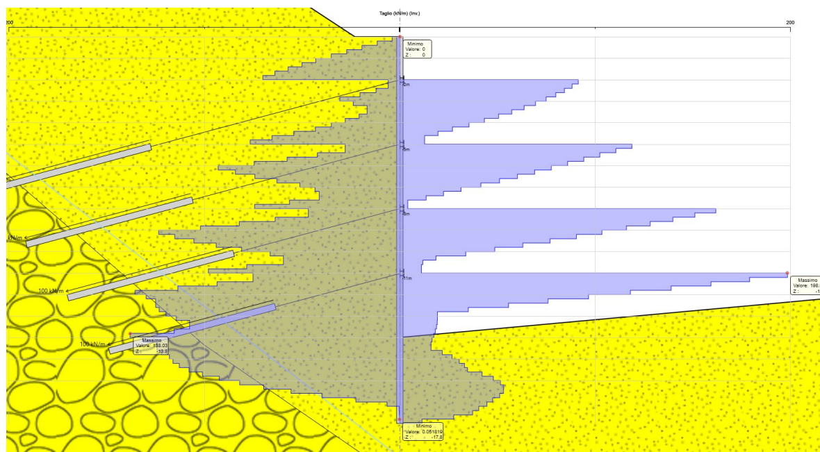
Figura 8.10 Diagramma Taglio ENV SLU-SISMA
