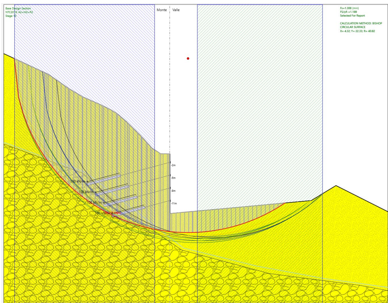
Fig. 15 – Analisi di stabilità STATICA per il caso A2+M2+R2
