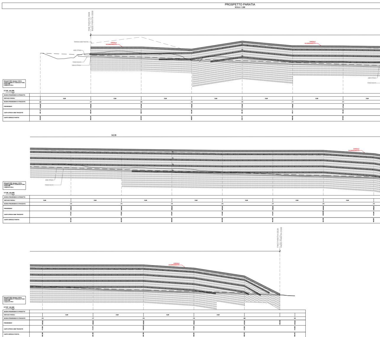
Figura 1.3 Profilo dell'opera
