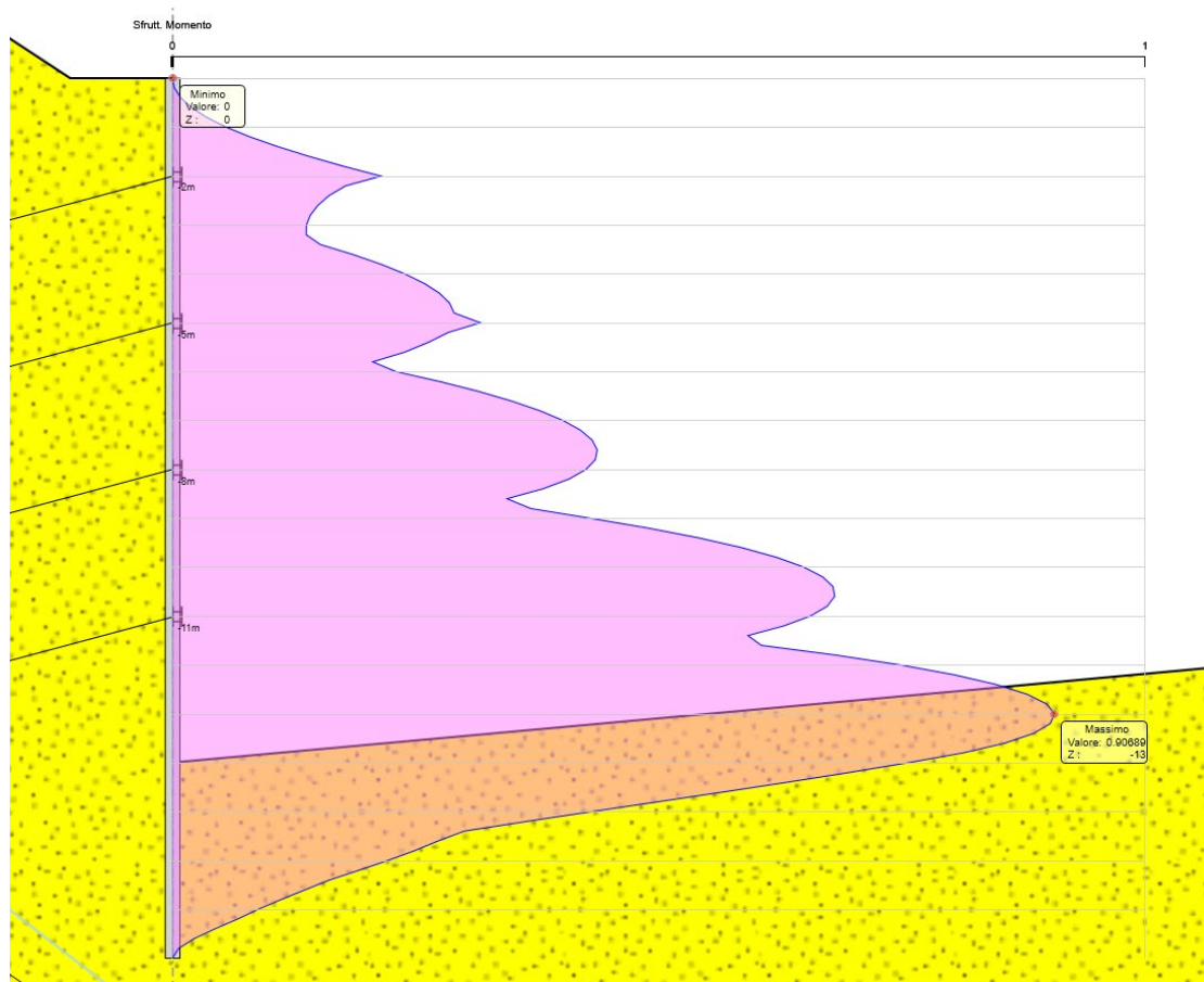
Figura 8.11 Sfruttamento a momento ENV SLU-SISMA
