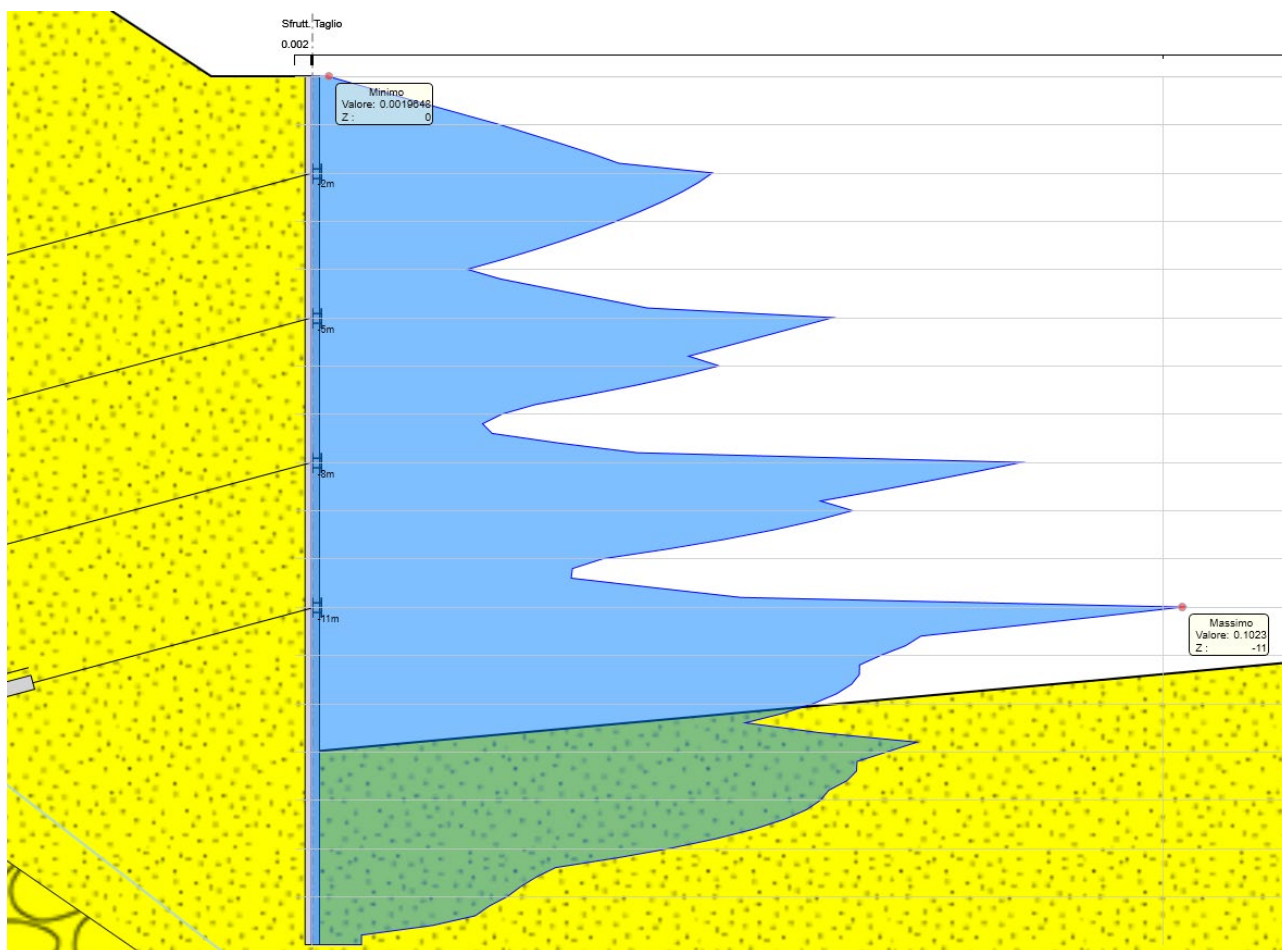
Figura 8.12 Sfruttamento a taglio ENV SLU-SISMA
