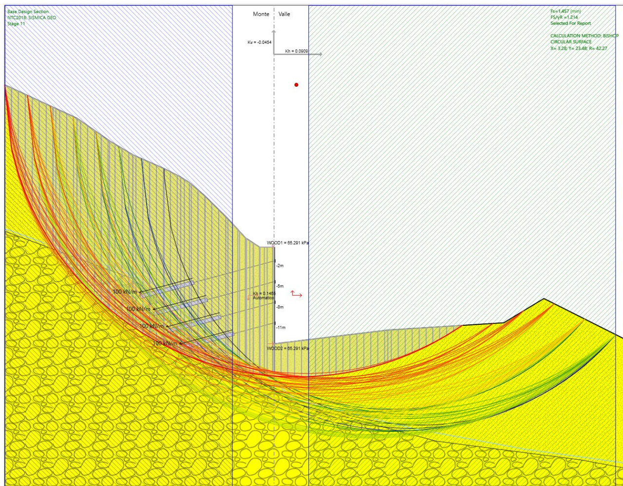
Fig. 17 – Analisi di stabilità SISMICA per il caso A2+M2+SISMA -kv
