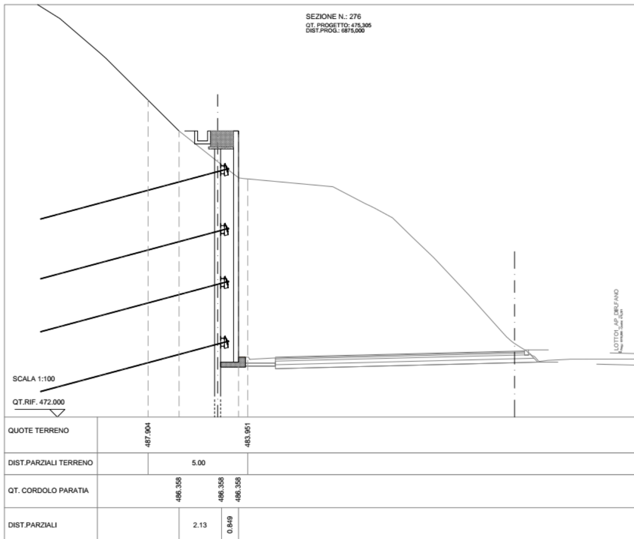
Figura 8.1 Sezione 276 tipo oggetto di verifica
