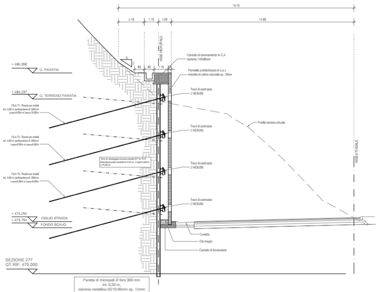
Figura 1.4 Sezioni tipo dell'opera
