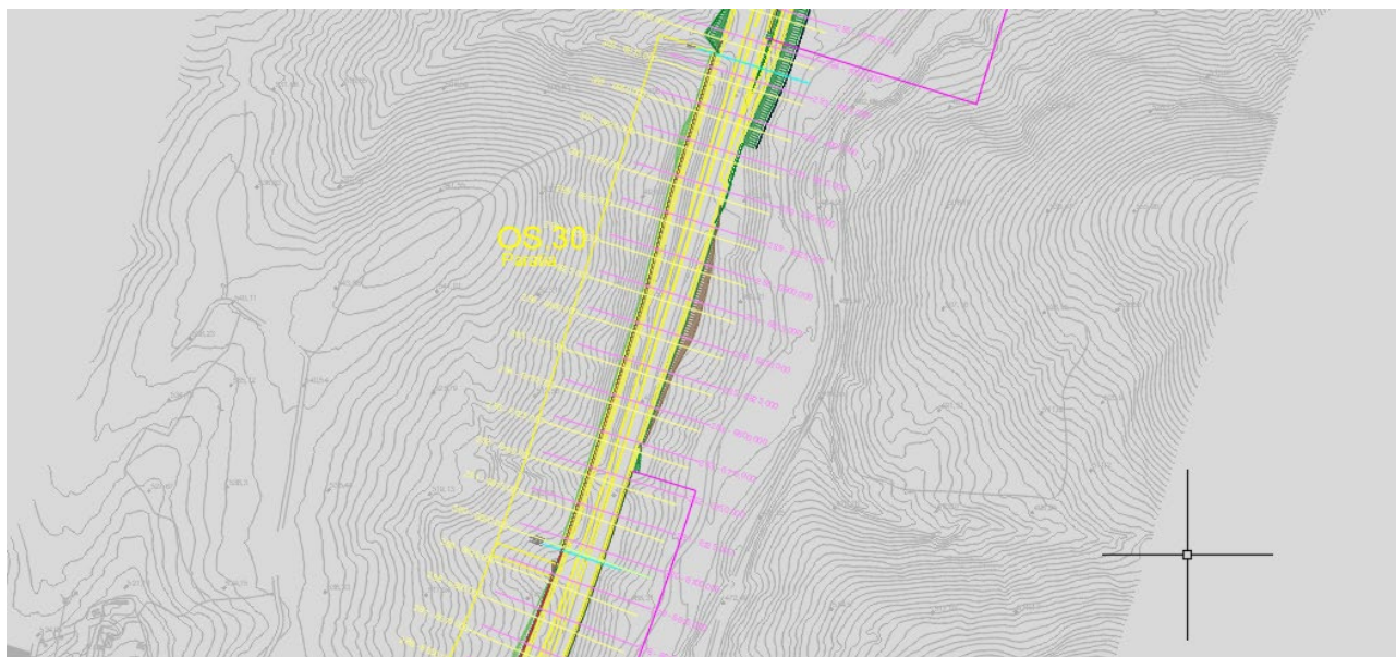
Figura 1.1 KeyPlan dell'opera
