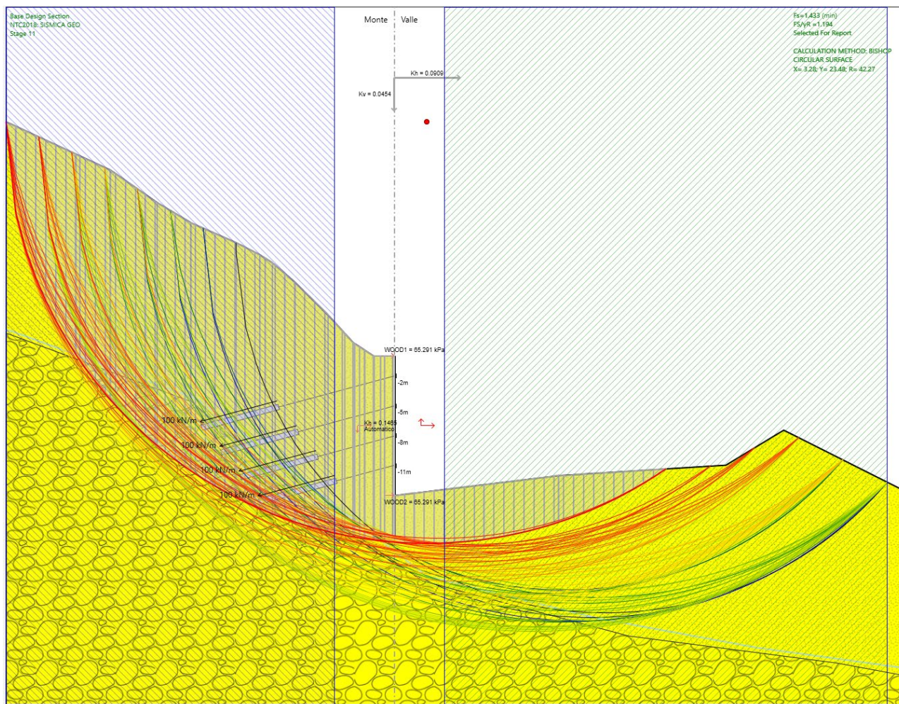
Fig. 16 – Analisi di stabilità SISMICA per il caso A2+M2+SISMA +kv
