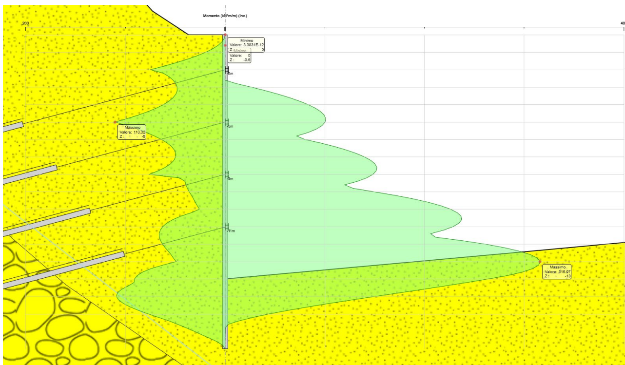
Figura 8.9 Diagramma Momento ENV SLU-SISMA
