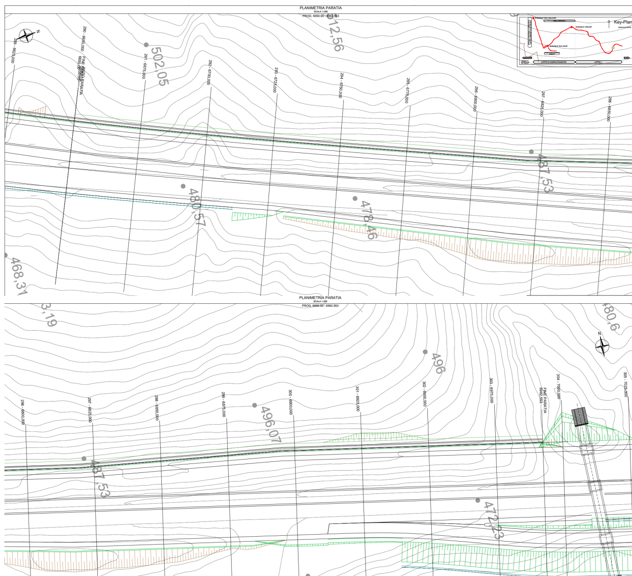
Figura 1.2 Planimetria dell'opera
