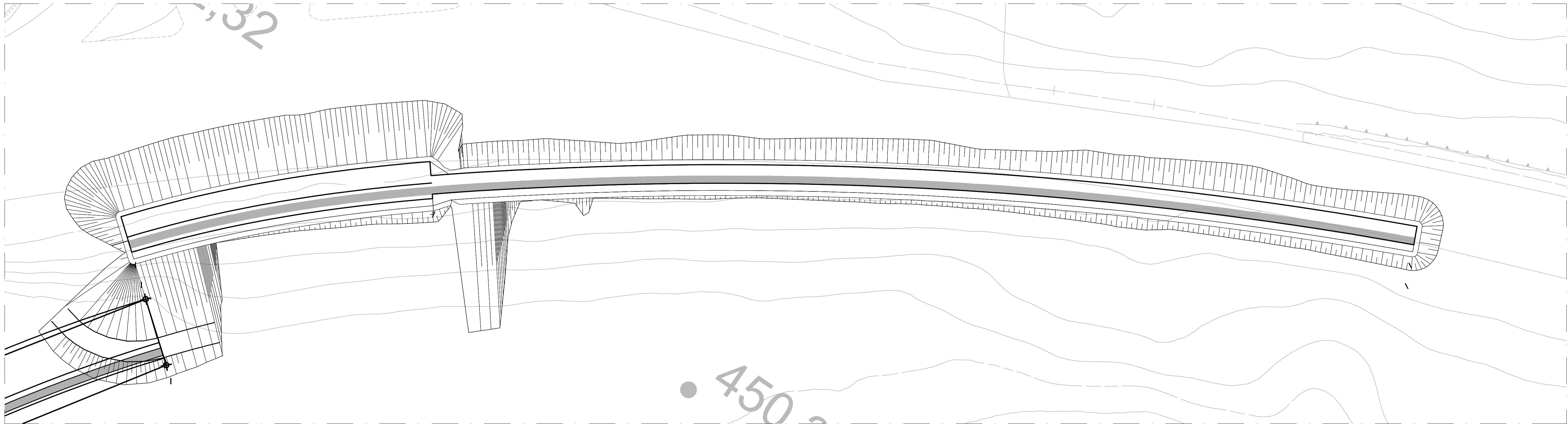
VISTA PLANIMETRICA MURO OS32 SCALA 1:200
