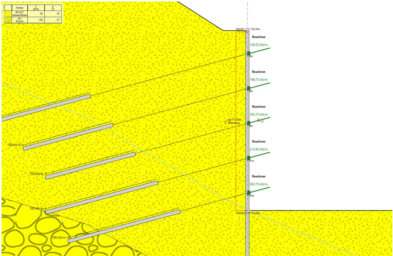
Figura 8.14 Reazioni ai supporti ENV SLU-SISMA
