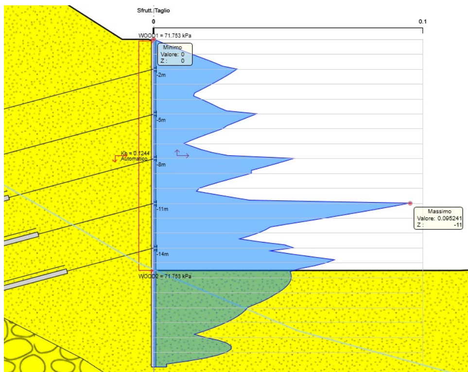
Figura 8.13 Sfruttamento a taglio ENV SLU-SISMA
