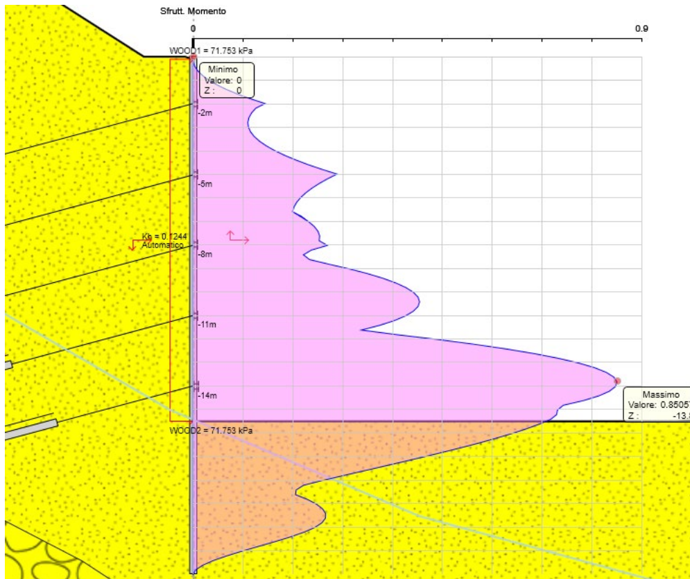
Figura 8.12 Sfruttamento a momento ENV SLU-SISMA
