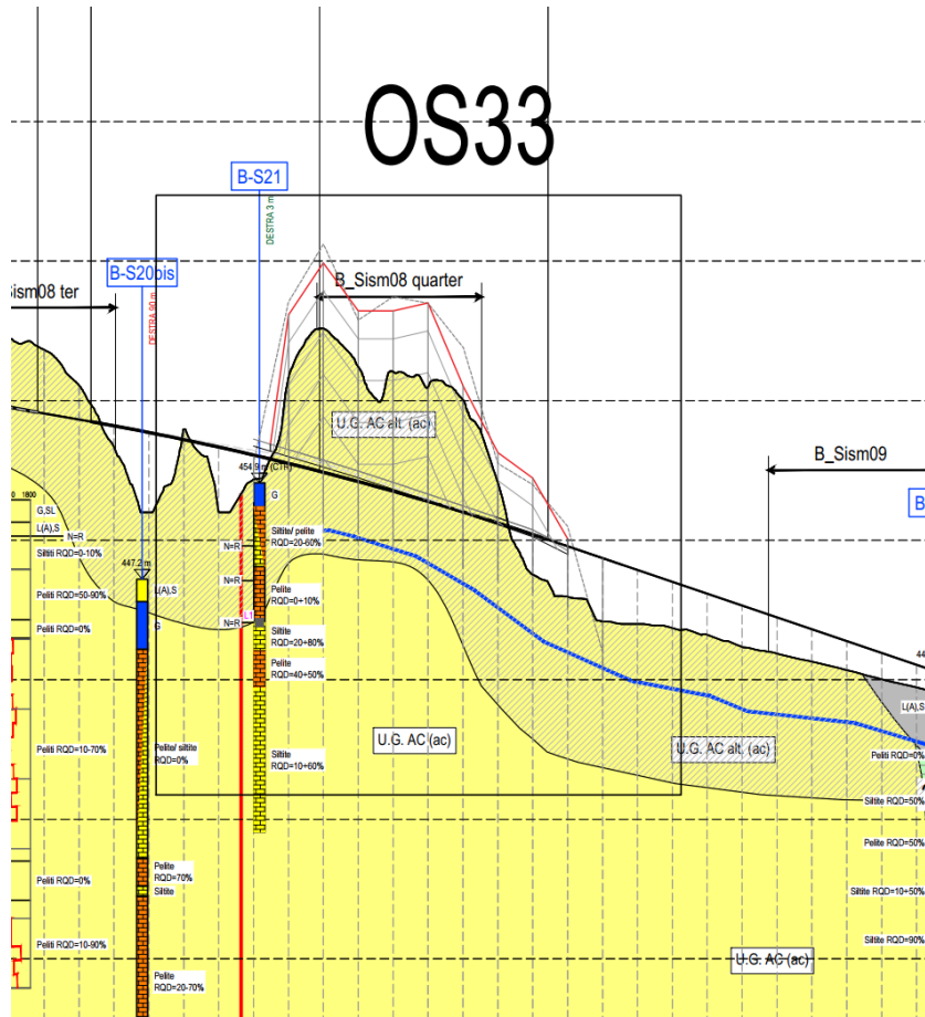
Figura 7.1 Sovrapposizione dell'opera con il profilo in asse
