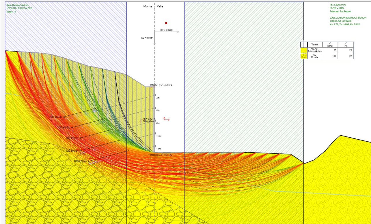
Fig. 17 – Analisi di stabilità SISMICA per il caso A2+M2+SISMA +kv
