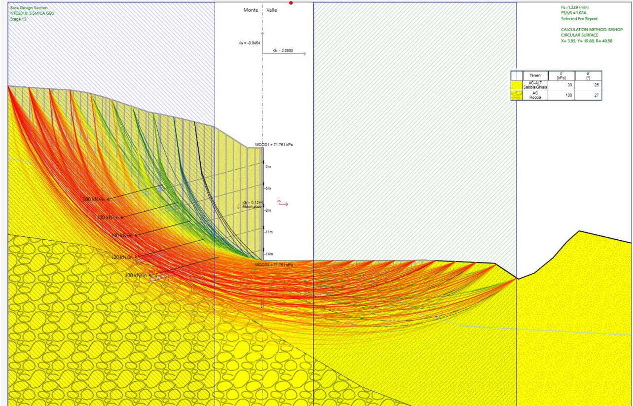
Fig. 18 – Analisi di stabilità SISMICA per il caso A2+M2+SISMA -kv
