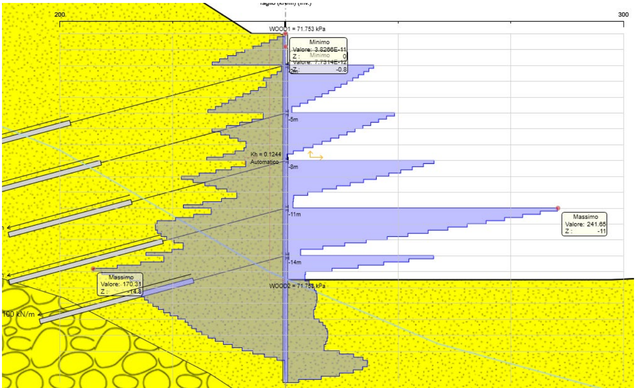
Figura 8.11 Diagramma Taglio ENV SLU-SISMA
