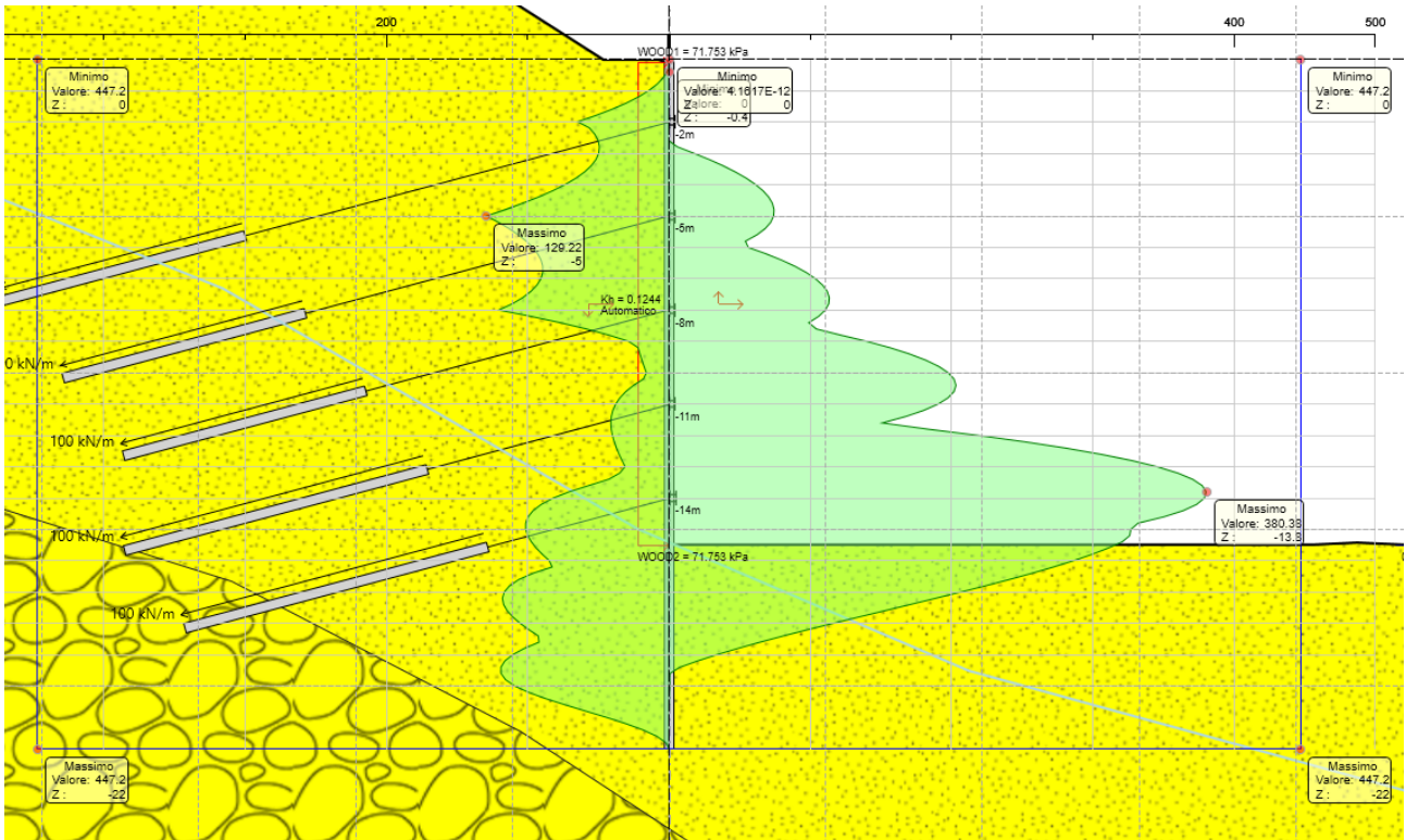
Figura 8.10 Diagramma Momento ENV SLU-SISMA
