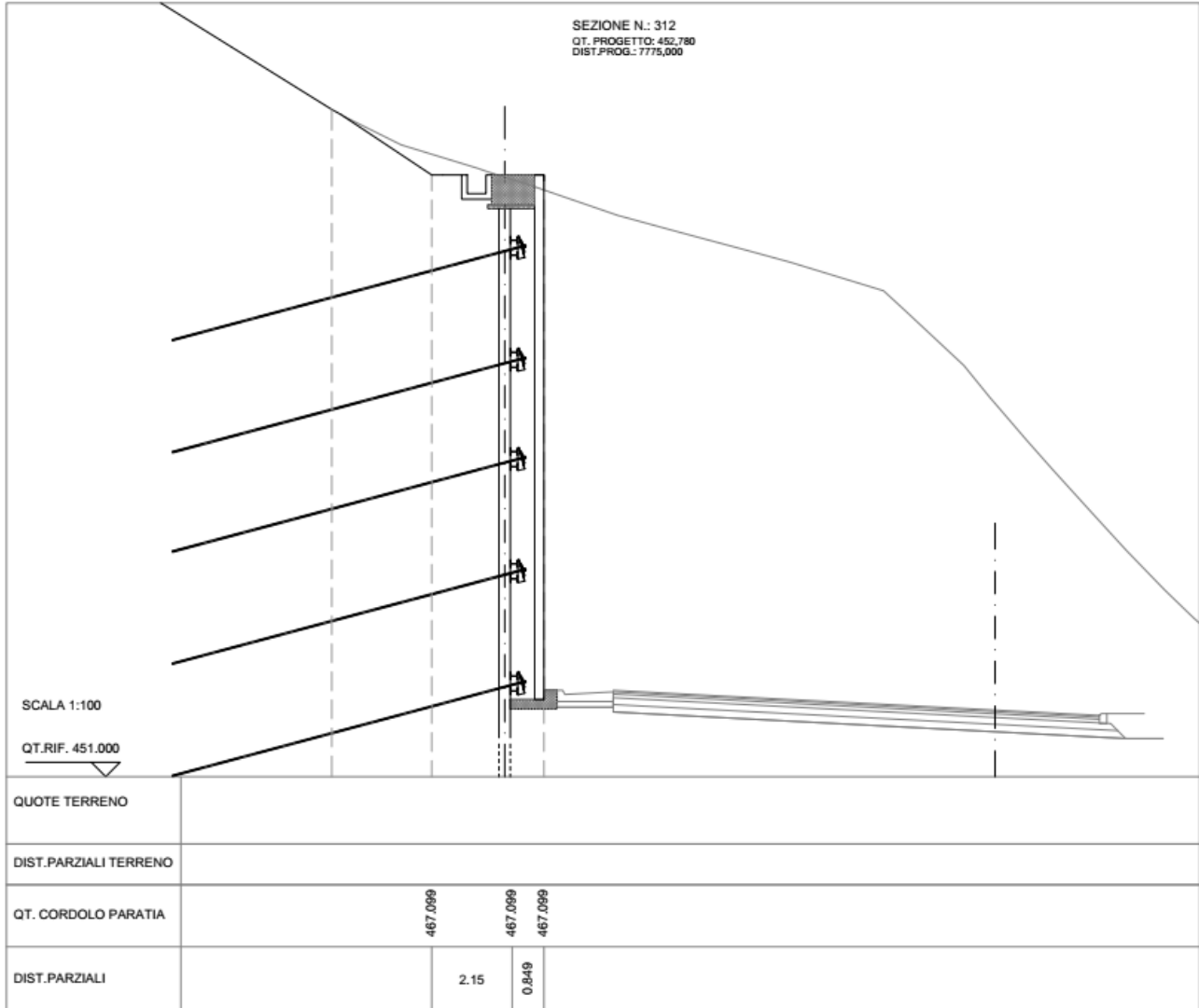
Figura 8.1 Sezione 312 tipo oggetto di verifica
