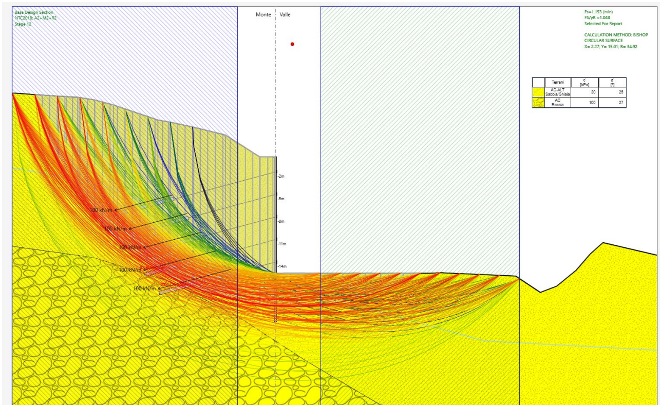
Fig. 16 – Analisi di stabilità STATICA per il caso A2+M2+R2
