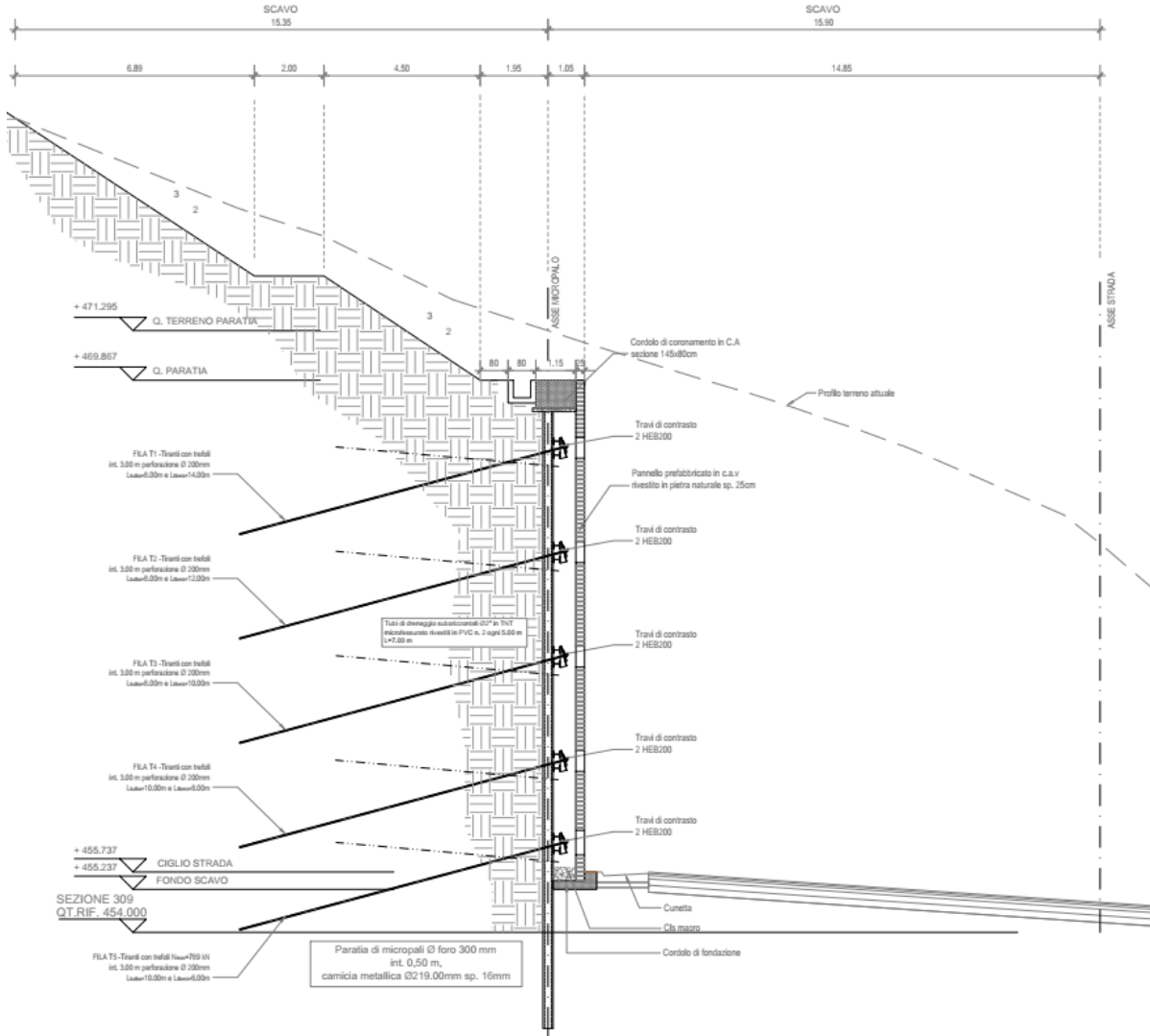
Figura 1.4 Sezioni tipo dell'opera
