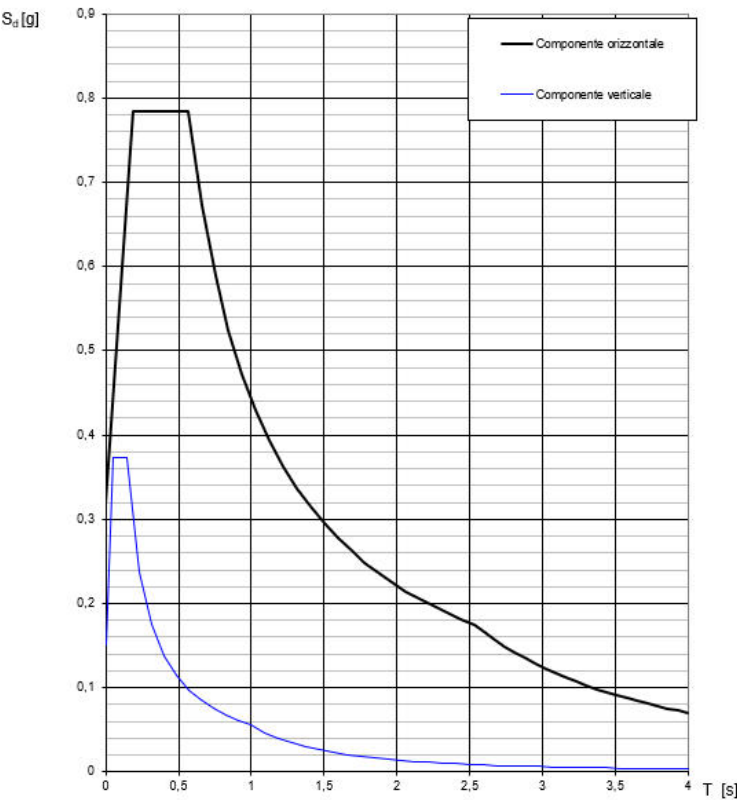
Figura 1-1 Spettro di risposta per lo stato limite SLV
