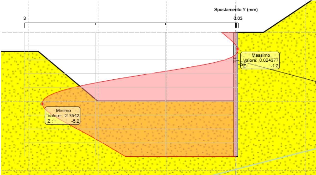
Figura 8.11 Spostamento massimo della paratia
