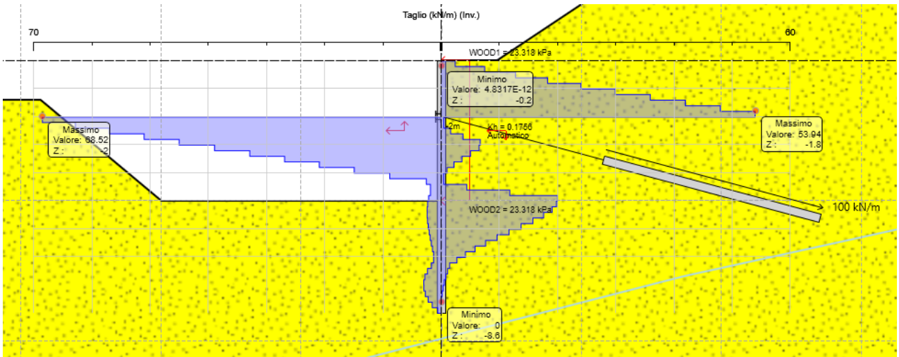
Figura 8.7 Diagramma Taglio ENV SLU-SISMA
