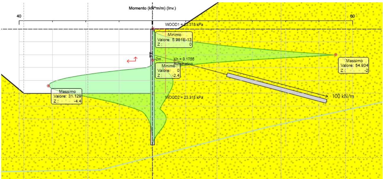
Figura 8.6 Diagramma Momento ENV SLU-SISMA
