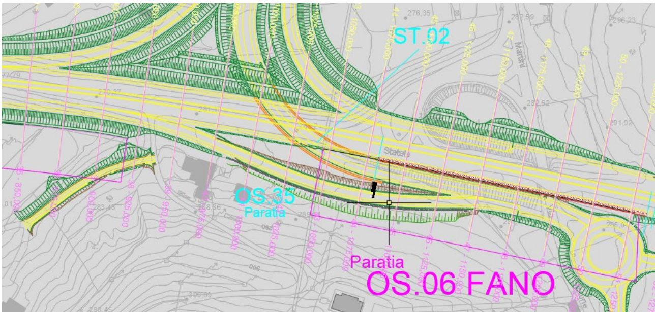
Figura 1.1 KeyPlan dell'opera
