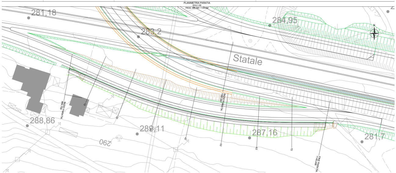
Figura 1.2 Planimetria dell'opera
