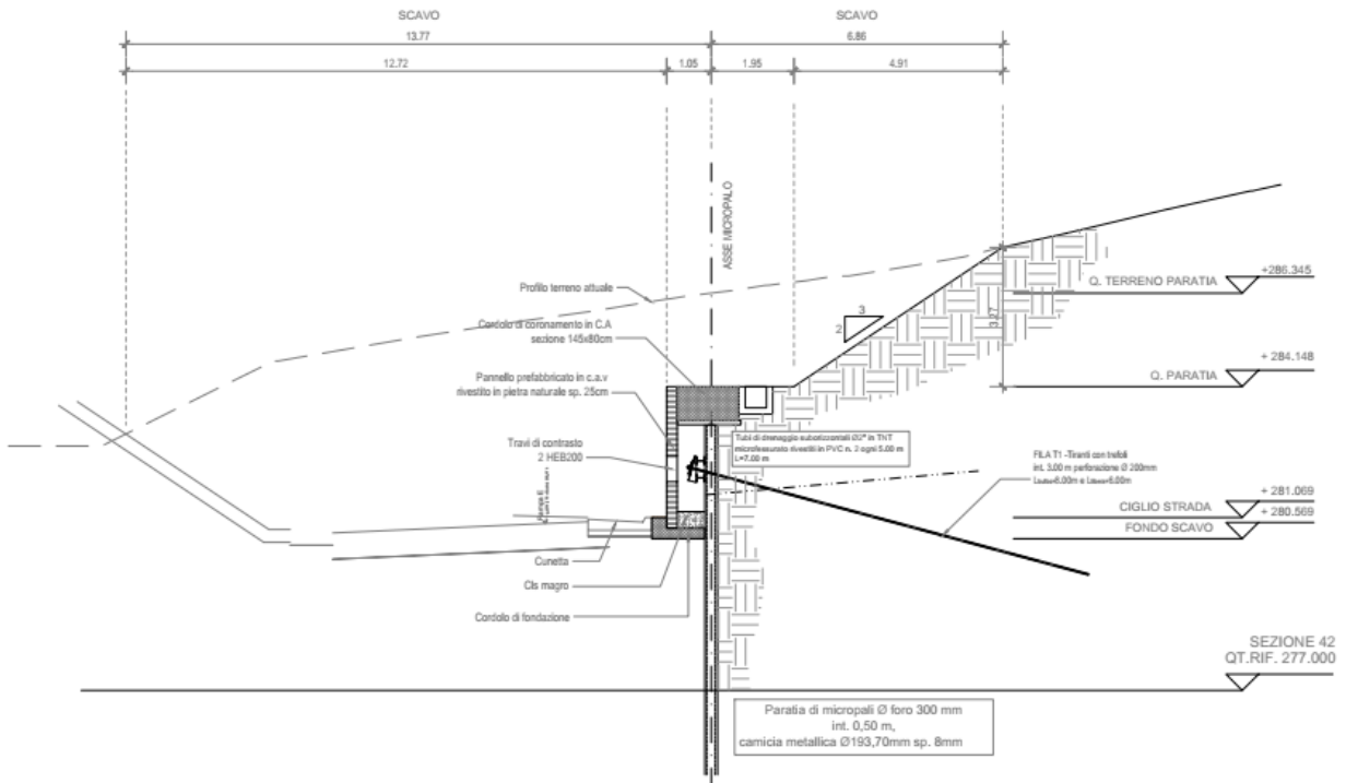
Figura 1.4 Sezioni tipo dell'opera
