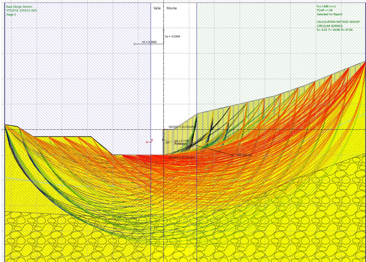
Fig. 14 – Analisi di stabilità SISMICA per il caso A2+M2+SISMA -kv
