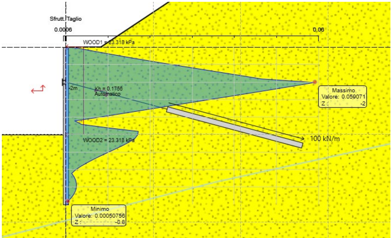
Figura 8.9 Sfruttamento a taglio ENV SLU-SISMA
