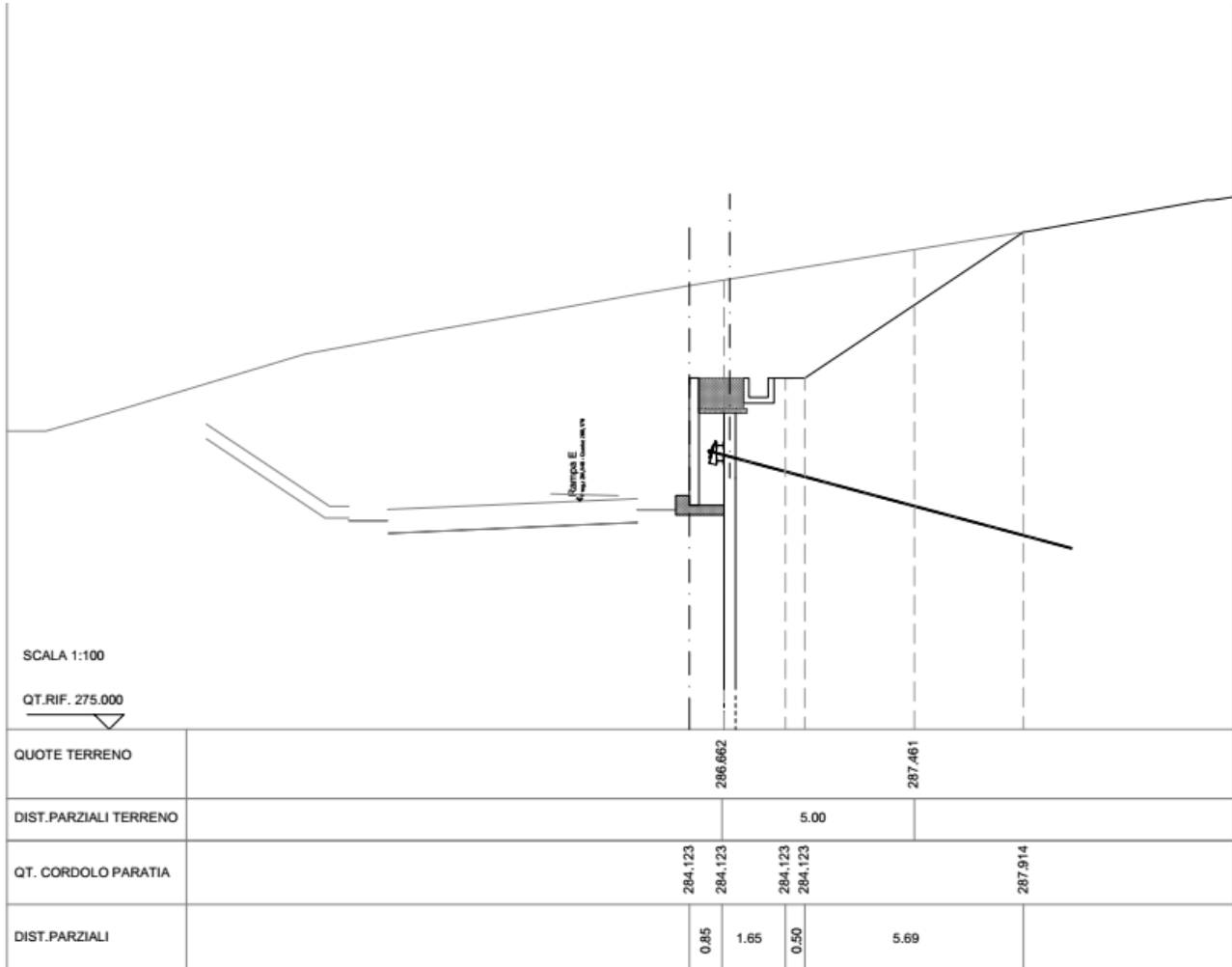
Figura 8.1 Sezione 75 tipo oggetto di verifica
