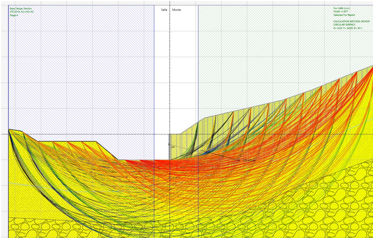
Fig. 12 – Analisi di stabilità STATICA per il caso A2+M2+R2
