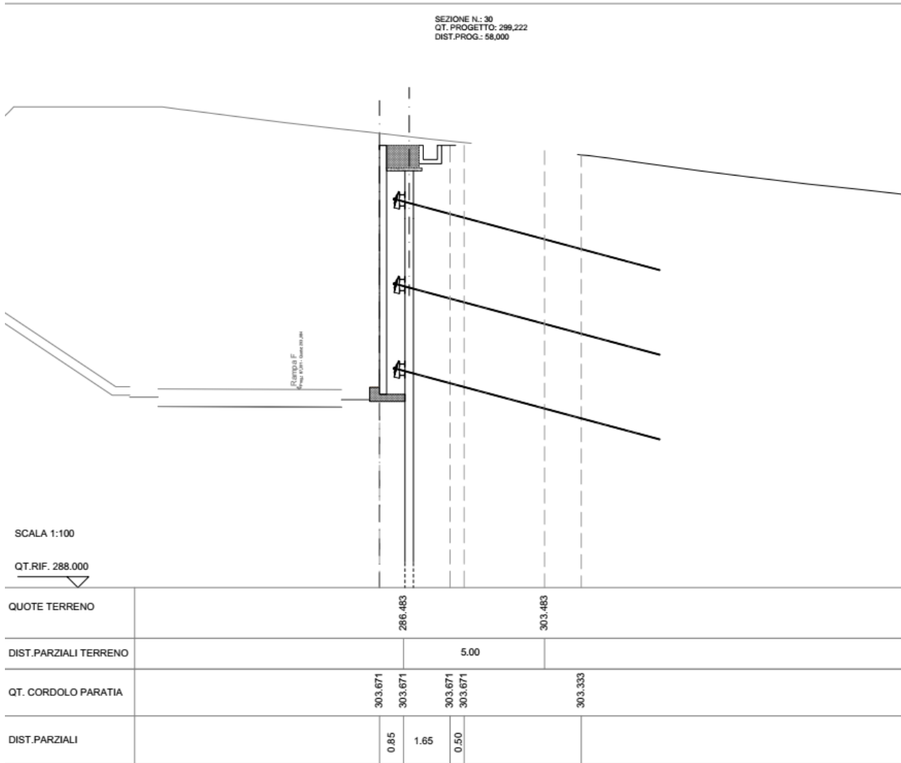
Figura 8.1 Sezione 30 tipo oggetto di verifica
