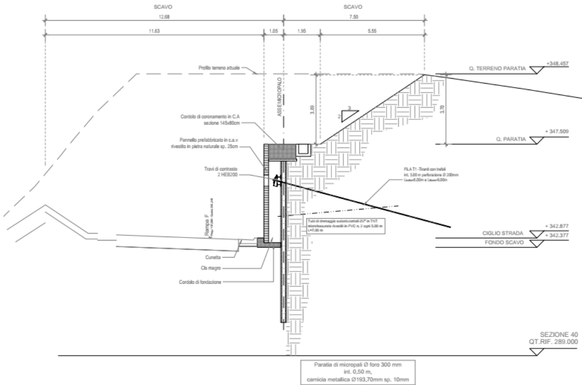
Figura 1.4 Sezioni tipo dell'opera
