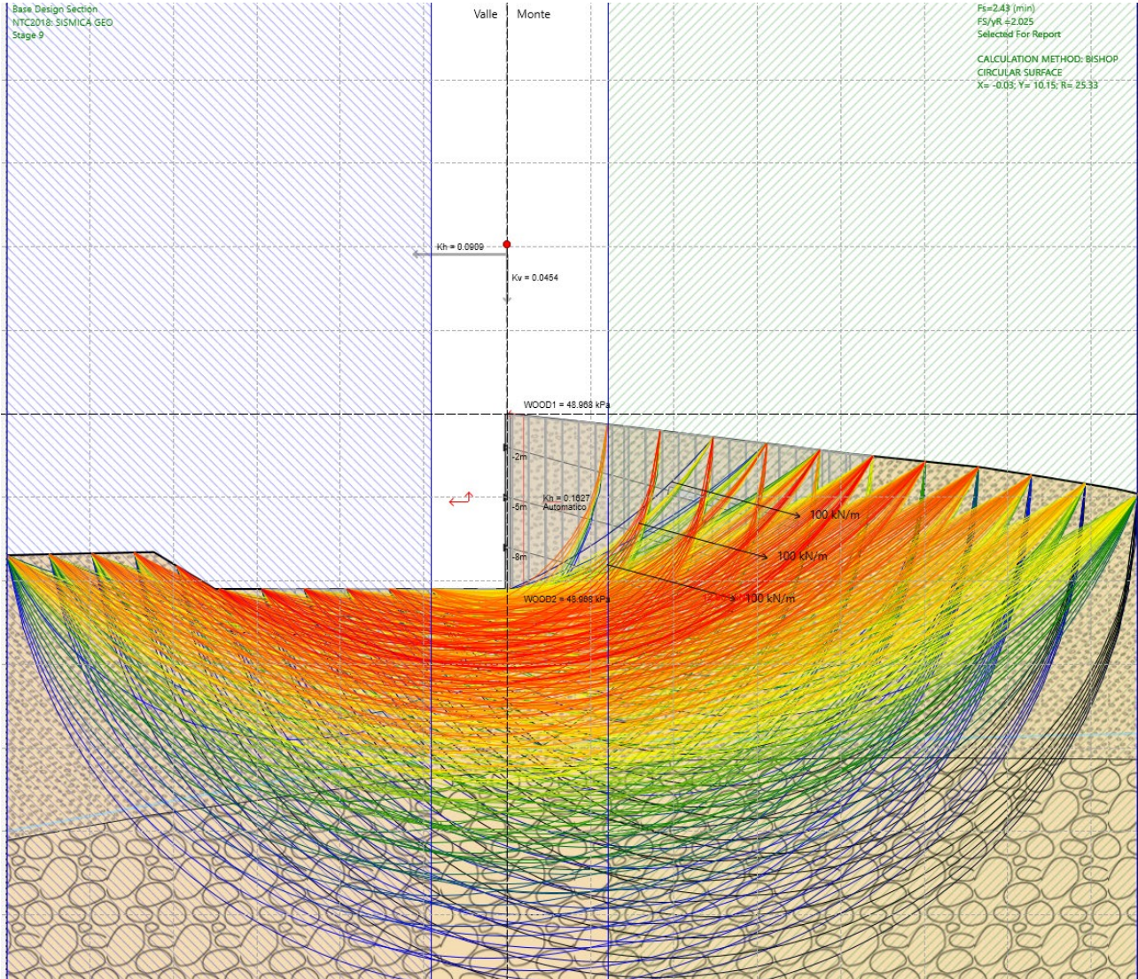
Fig. 15 – Analisi di stabilità SISMICA per il caso A2+M2+SISMA +kv
