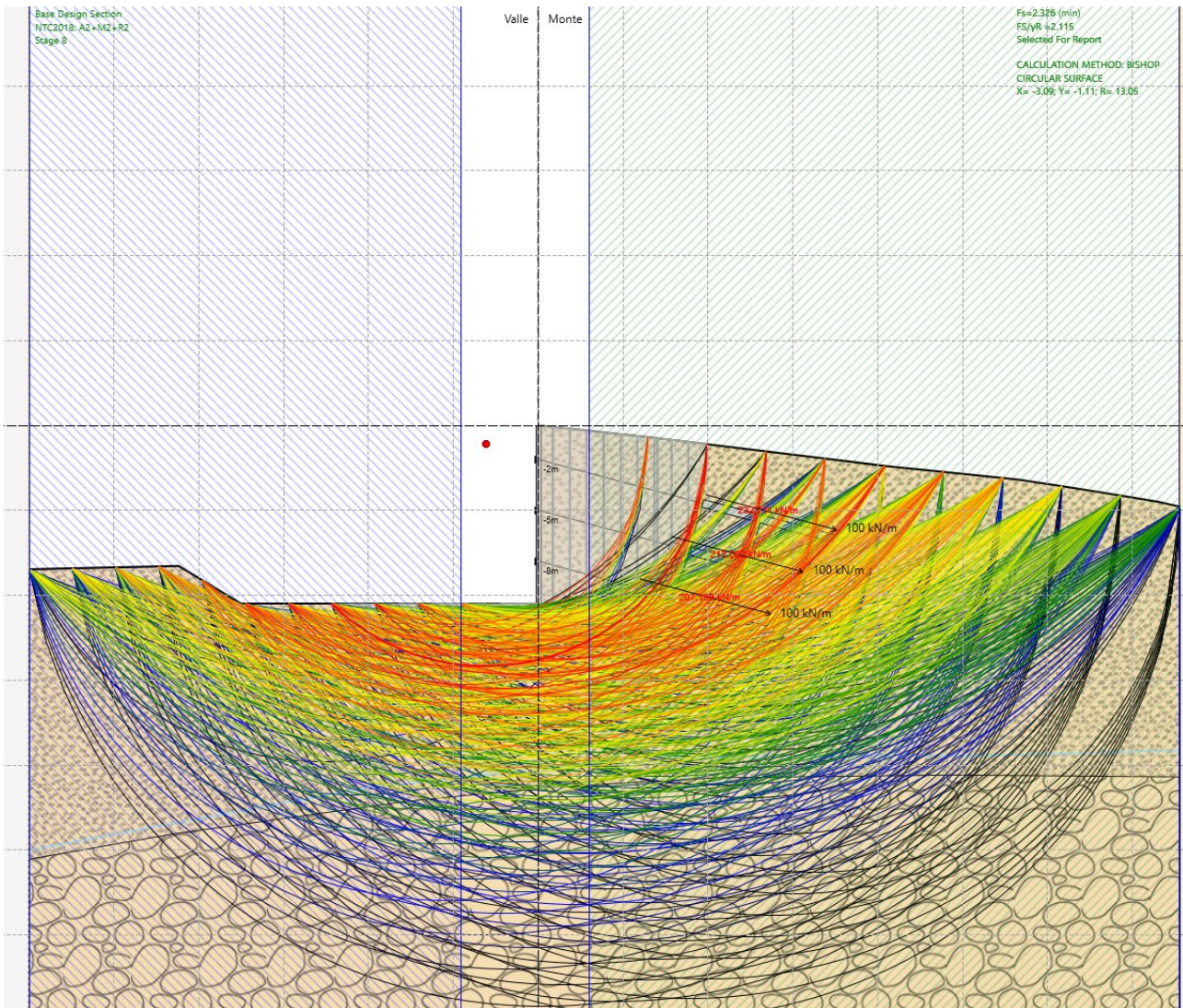
Fig. 14 – Analisi di stabilità STATICA per il caso A2+M2+R2
