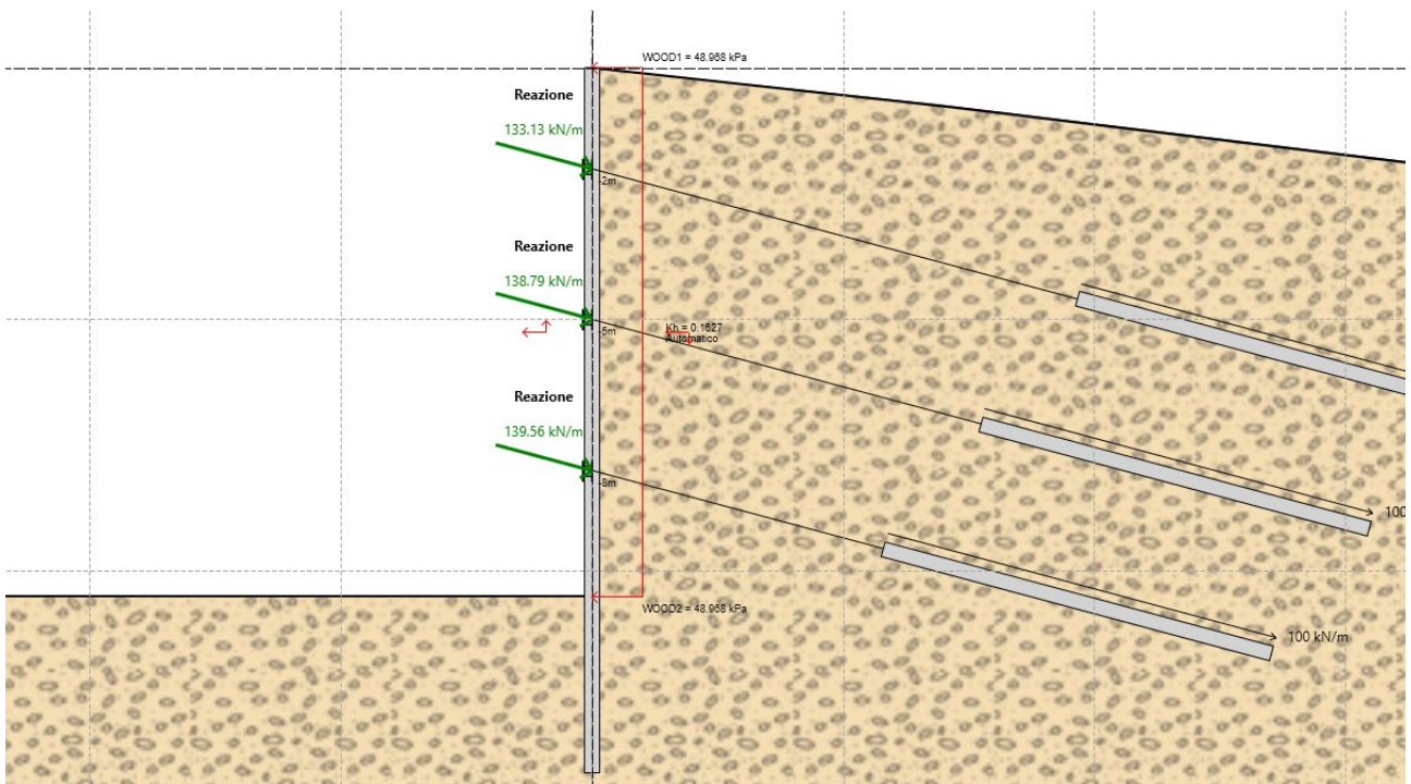
Figura 8.12 Reazioni ai supporti ENV SLU-SISMA
