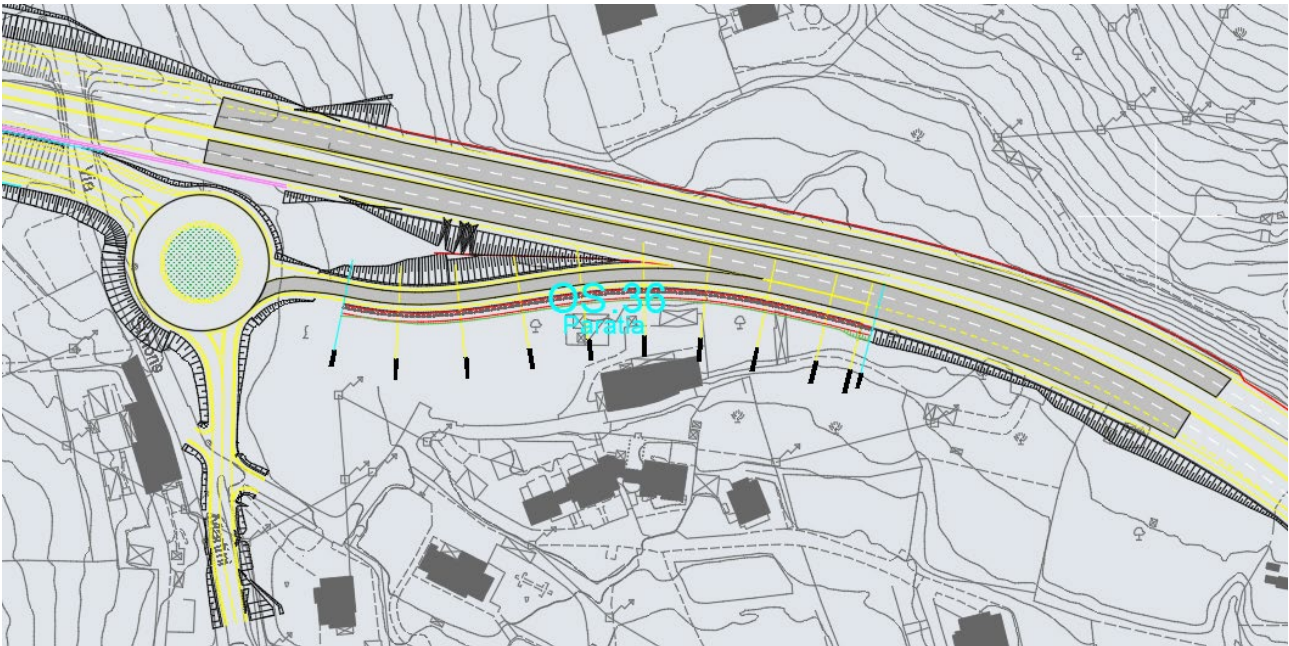
Figura 1.1 KeyPlan dell'opera
