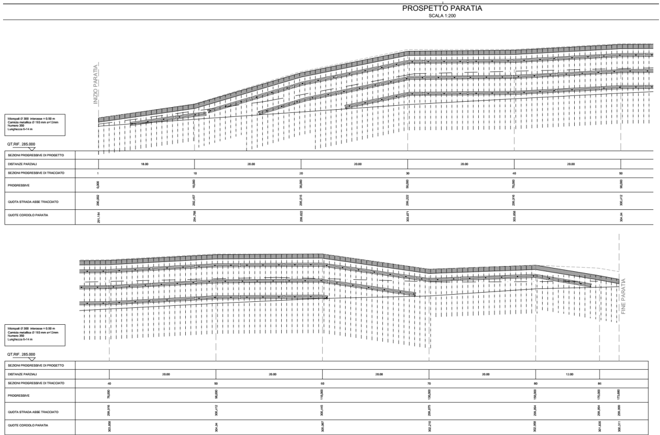
Figura 1.3 Profilo dell'opera
