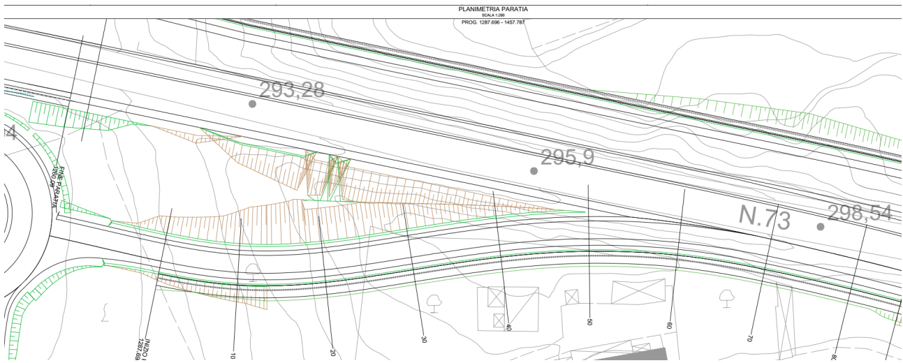
Figura 1.2 Planimetria dell'opera
