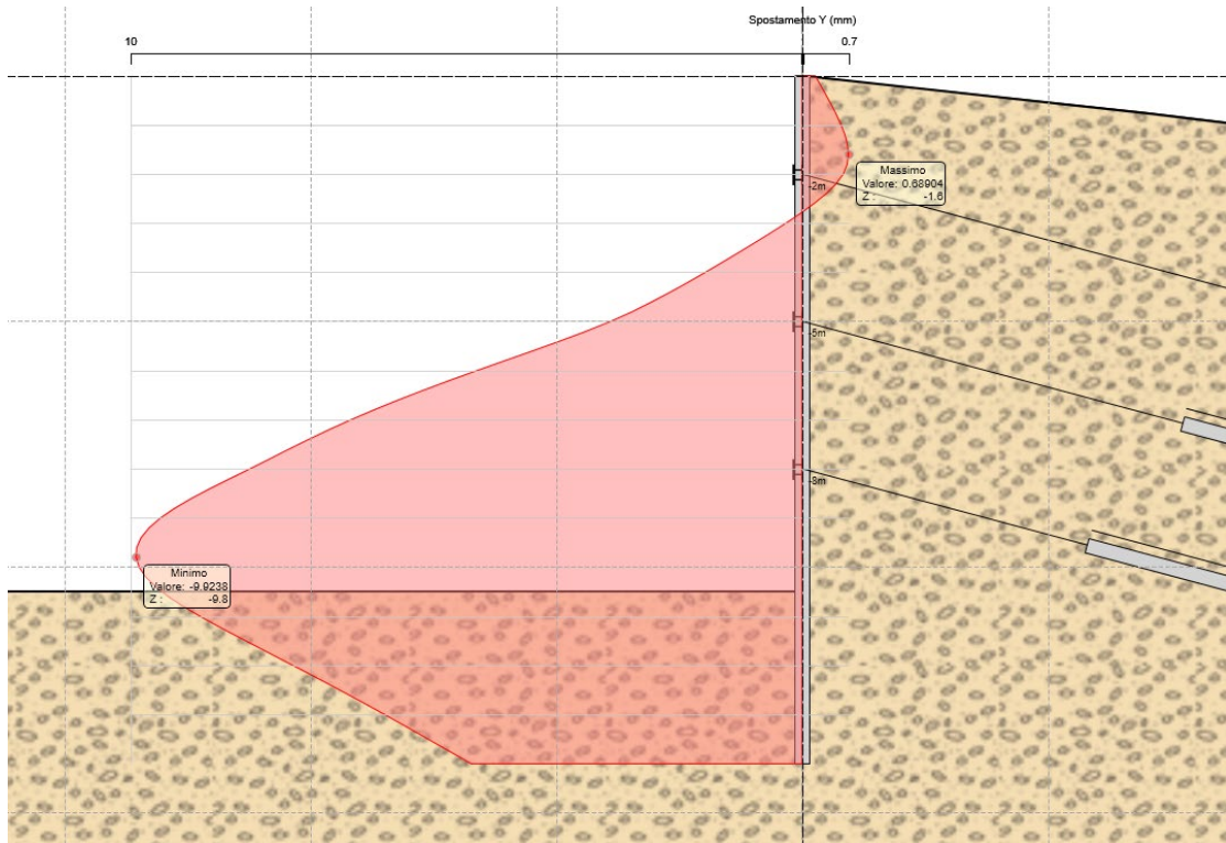
Figura 8.13 Spostamento massimo della paratia
