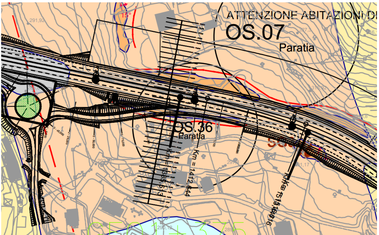
Figura 7.1 Vista in pianta dell'opera sulla carta geologica
