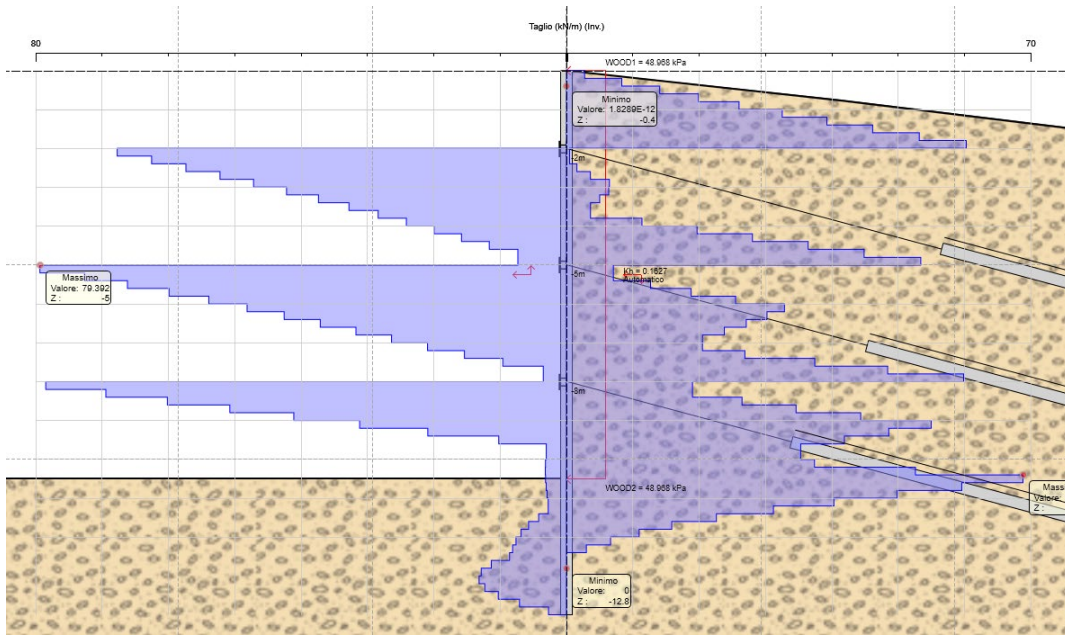
Figura 8.9 Diagramma Taglio ENV SLU-SISMA
