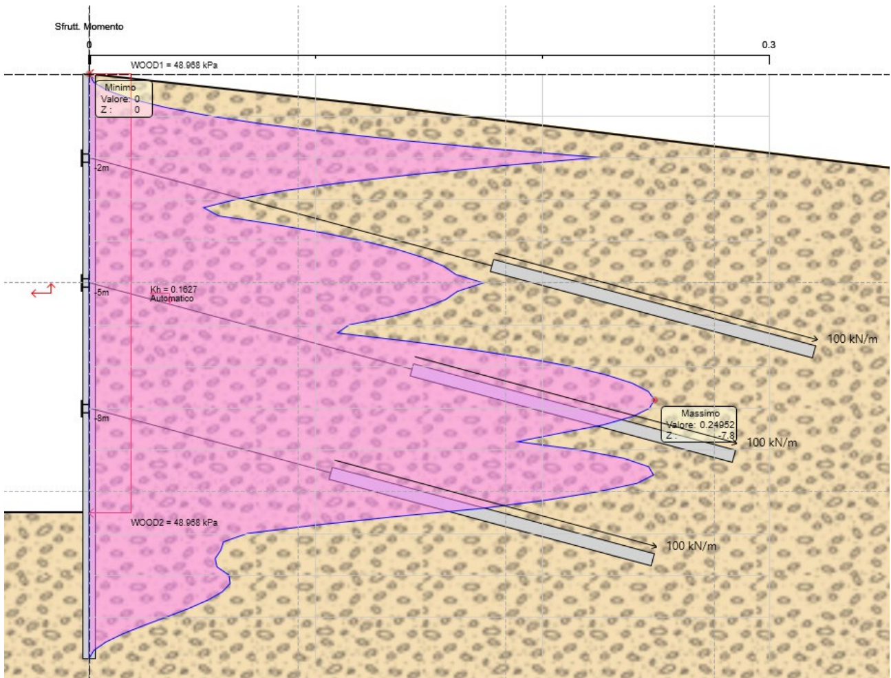
Figura 8.10 Sfruttamento a momento ENV SLU-SISMA
