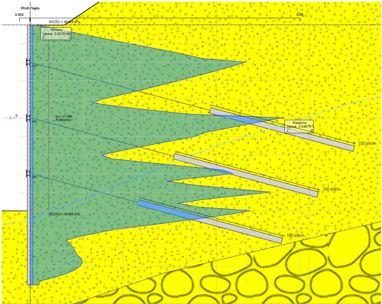
Figura 8.11 Sfruttamento a taglio ENV SLU-SISMA
