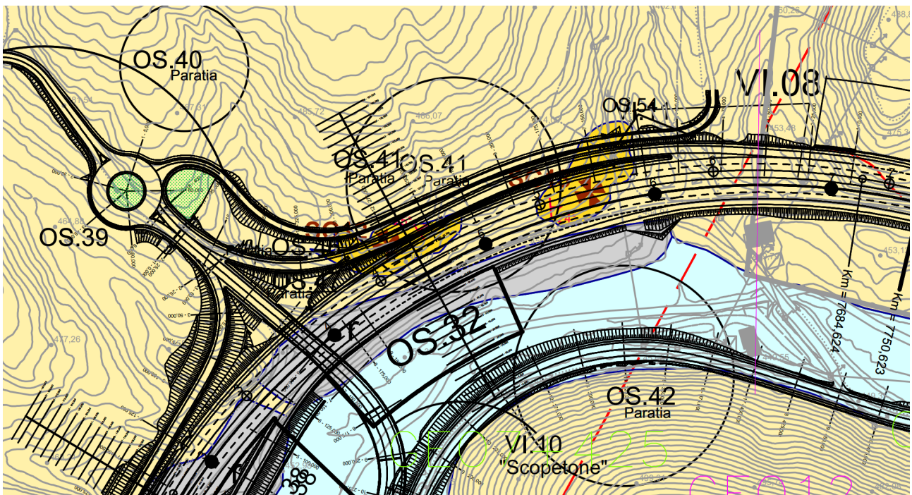
Figura 7.1 Sovrapposizione dell'opera con il profilo in asse
