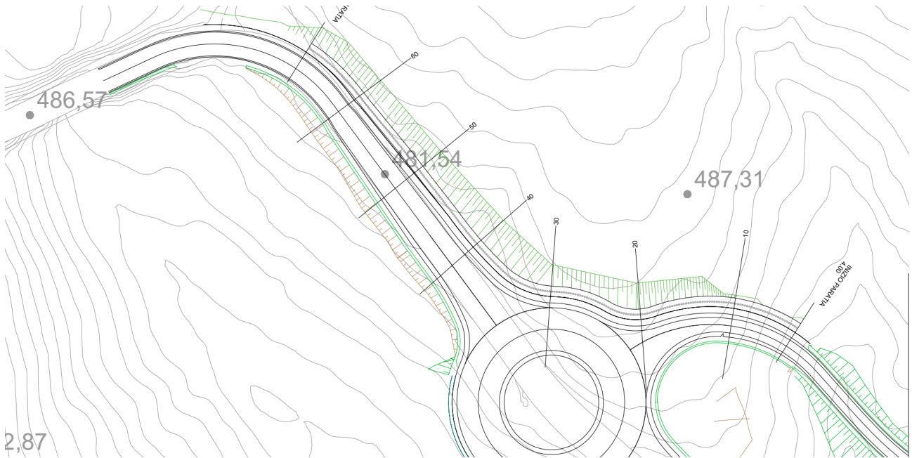
Figura 1.2 Planimetria dell'opera
