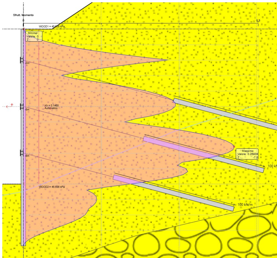
Figura 8.10 Sfruttamento a momento ENV SLU-SISMA
