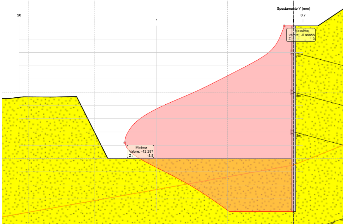
Figura 8.13 Spostamento massimo della paratia
