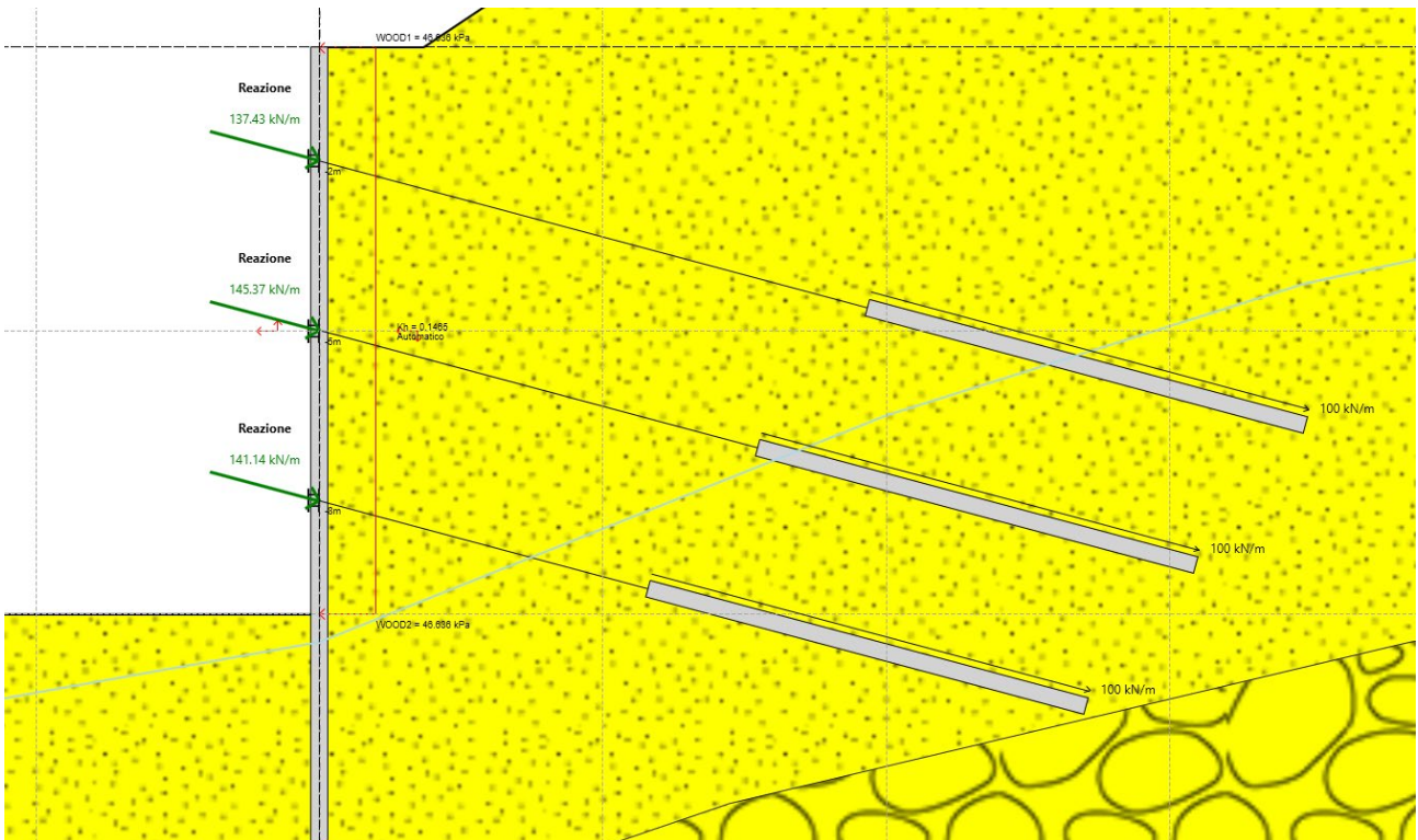
Figura 8.12 Reazioni ai supporti ENV SLU-SISMA
