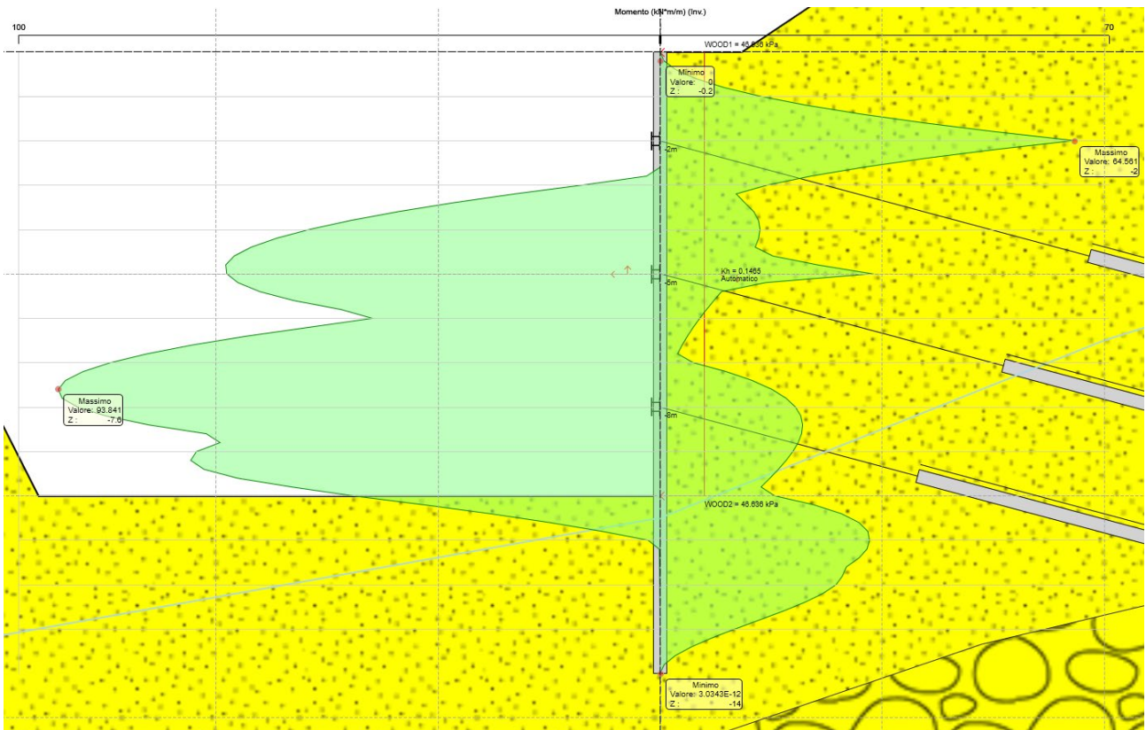
Figura 8.8 Diagramma Momento ENV SLU-SISMA
