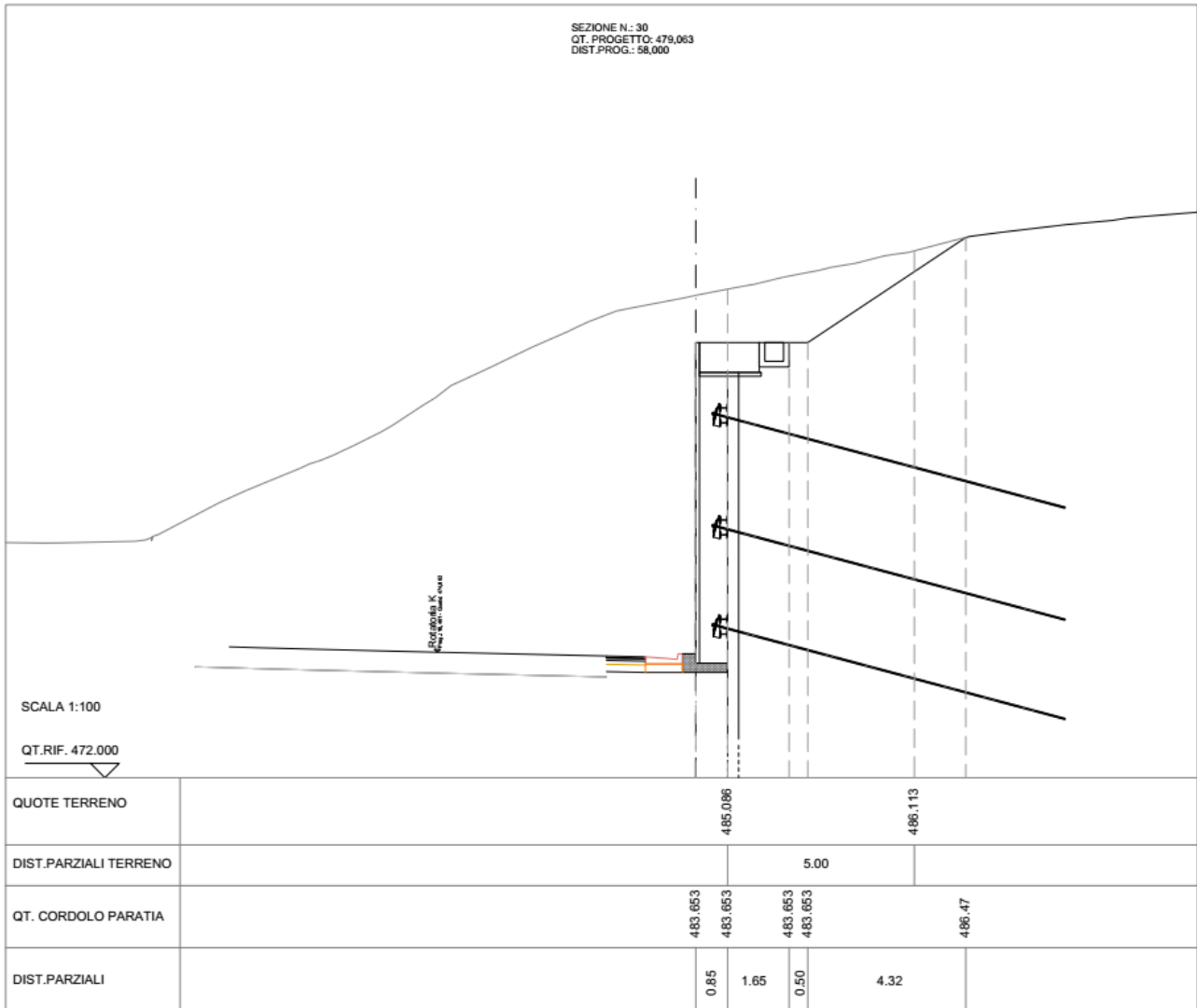
Figura 8.1 Sezione 30 tipo oggetto di verifica
