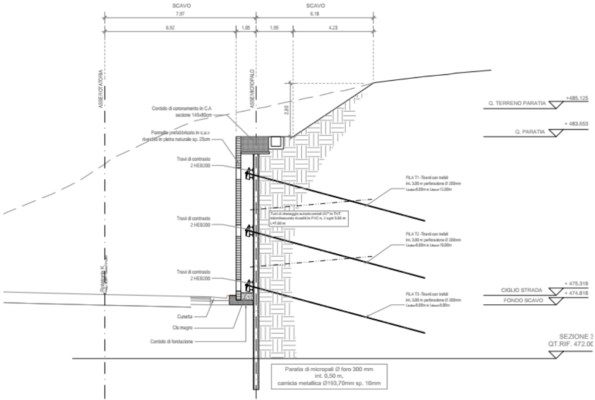
Figura 1.4 Sezioni tipo dell'opera
