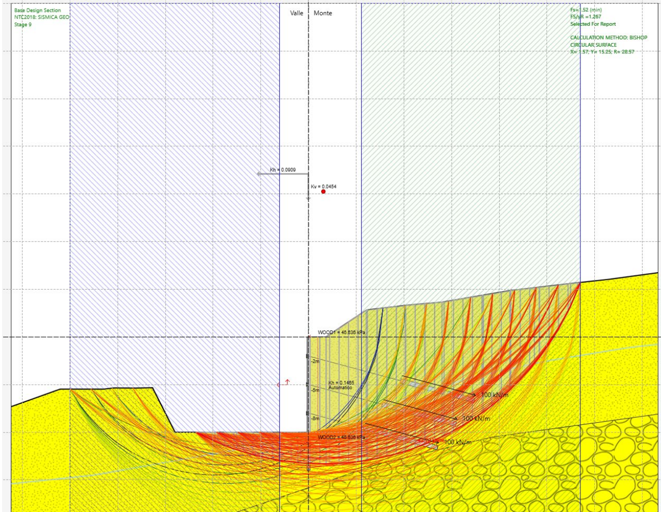
Fig. 15 – Analisi di stabilità SISMICA per il caso A2+M2+SISMA +kv
