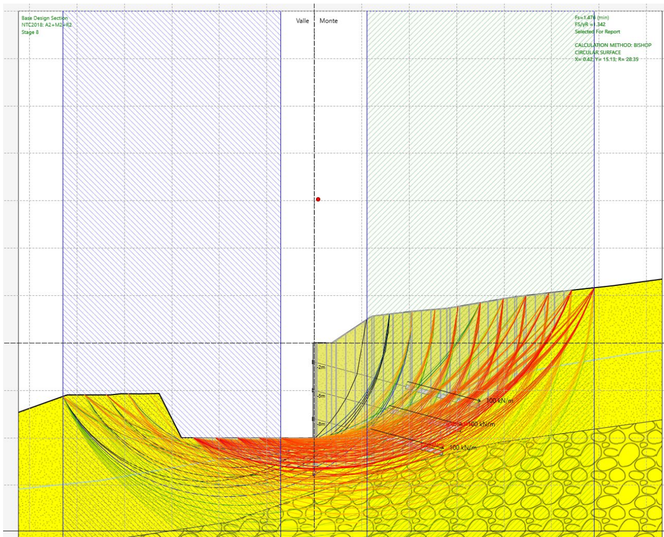
Fig. 14 – Analisi di stabilità STATICA per il caso A2+M2+R2
