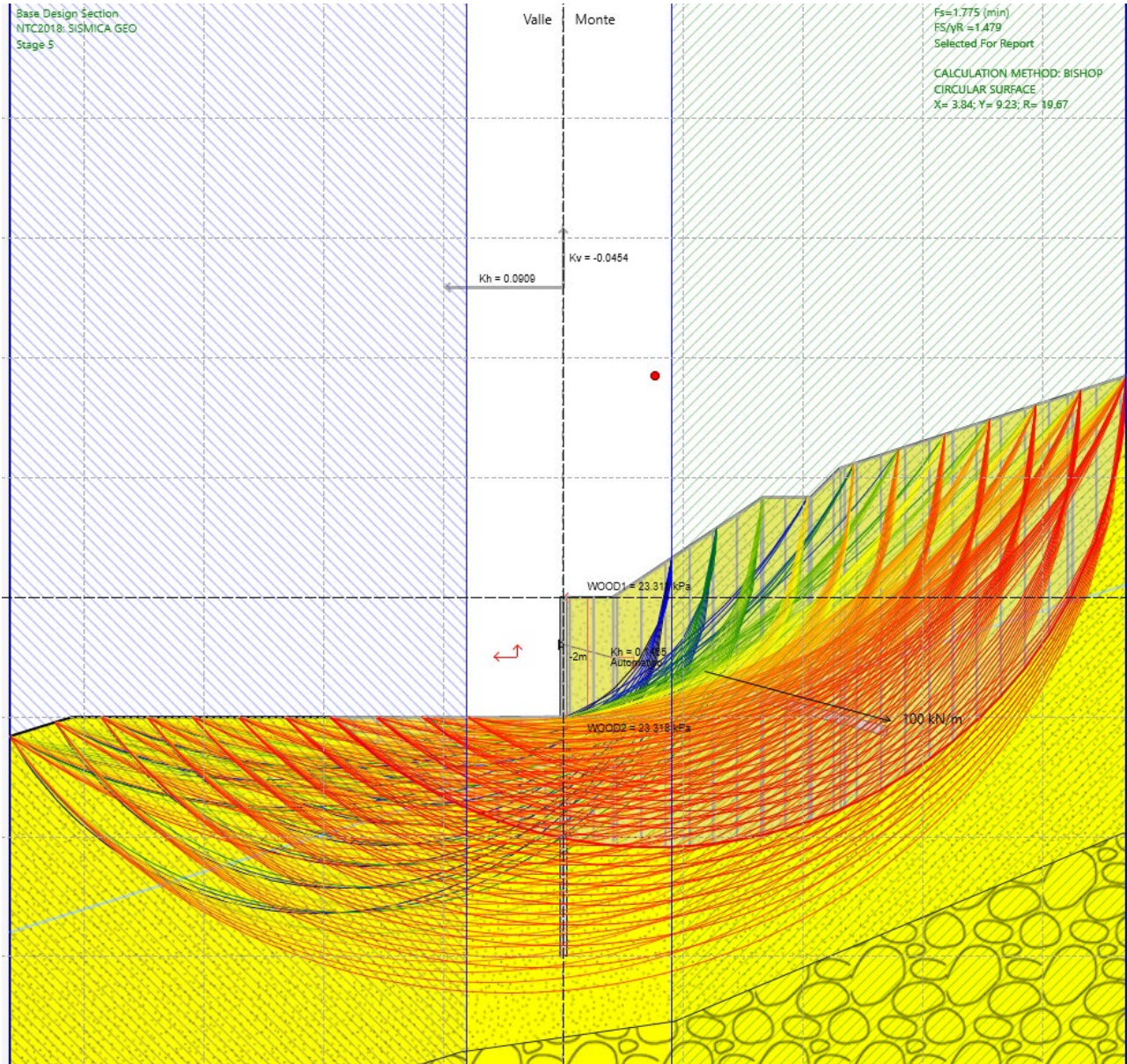
Fig. 14 – Analisi di stabilità SISMICA per il caso A2+M2+SISMA -kv
