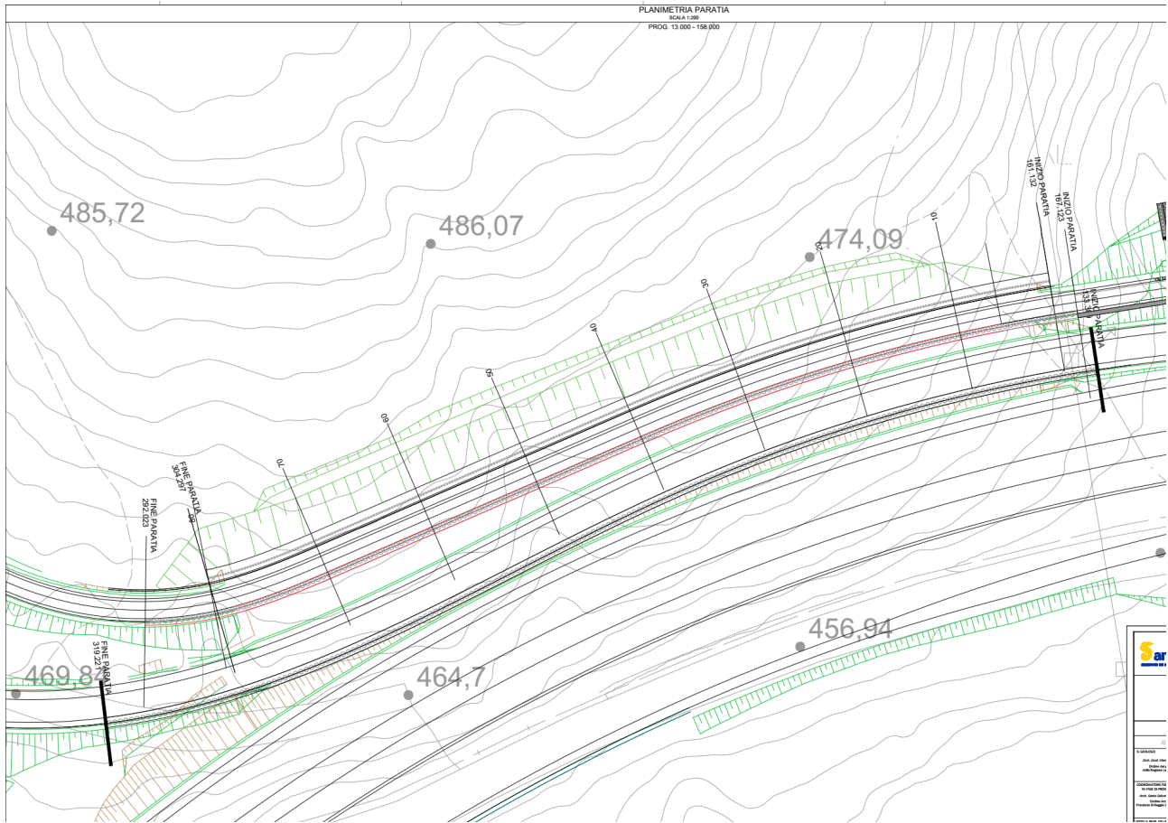
Figura 1.2 Planimetria dell'opera
