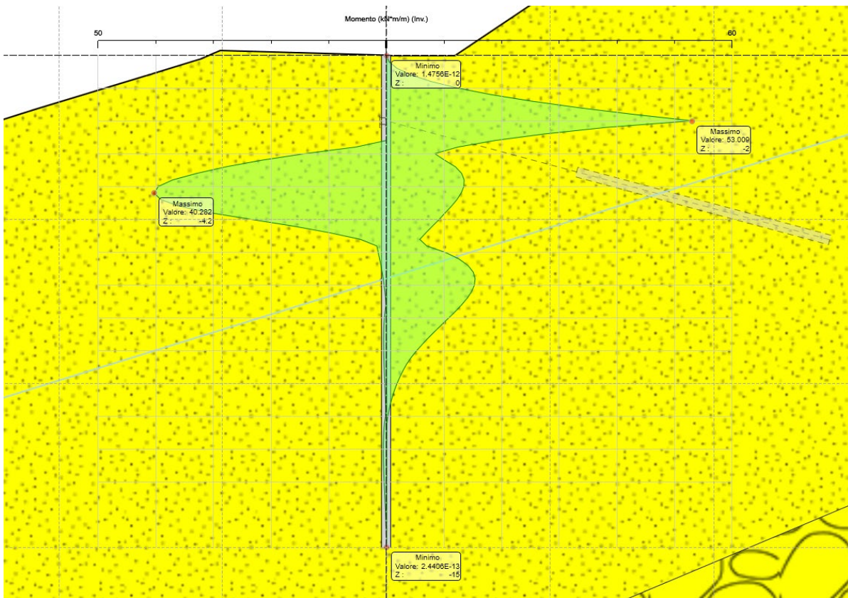
Figura 8.6 Diagramma Momento ENV SLU-SISMA
