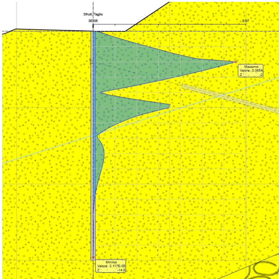
Figura 8.9 Sfruttamento a taglio ENV SLU-SISMA
