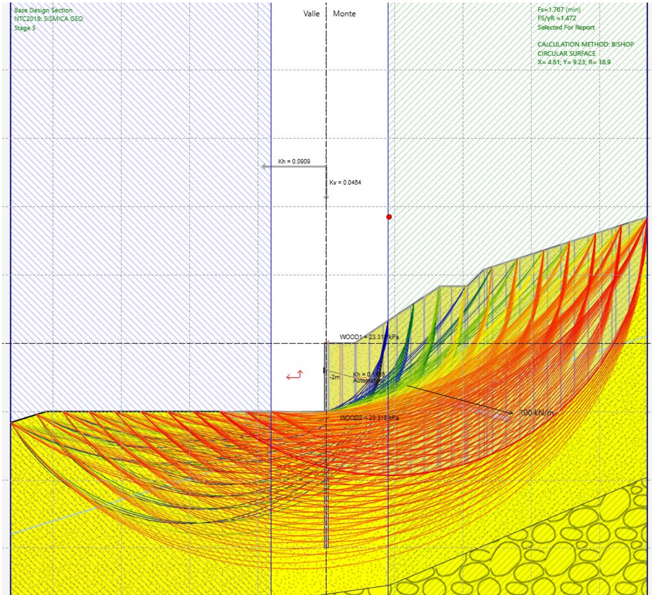
Fig. 13 – Analisi di stabilità SISMICA per il caso A2+M2+SISMA +kv
