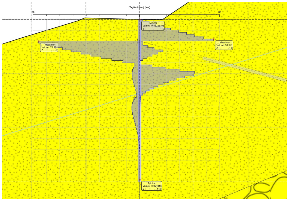
Figura 8.7 Diagramma Taglio ENV SLU-SISMA
