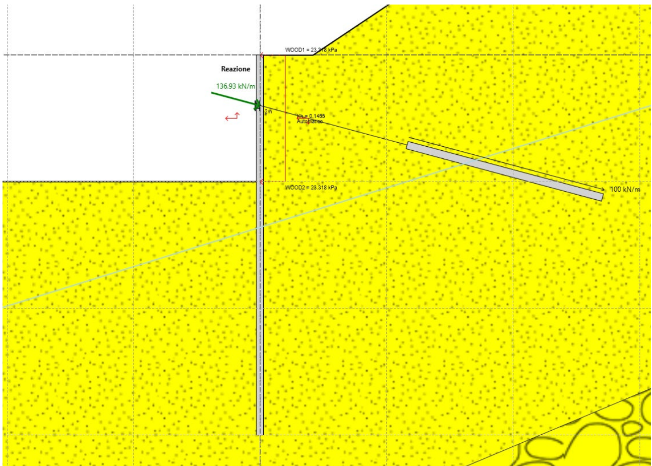
Figura 8.10 Reazioni ai supporti ENV SLU-SISMA
