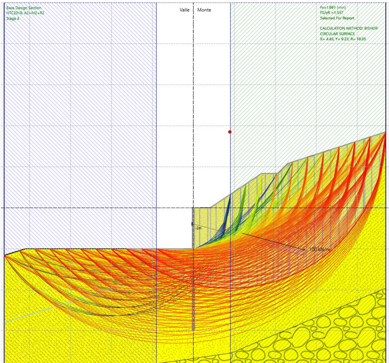
Fig. 12 – Analisi di stabilità STATICA per il caso A2+M2+R2
