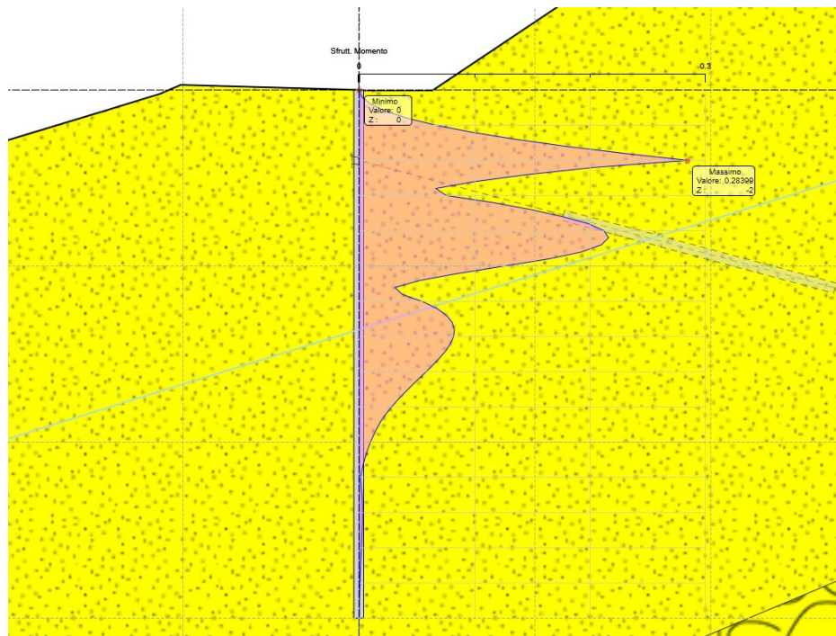
Figura 8.8 Sfruttamento a momento ENV SLU-SISMA
