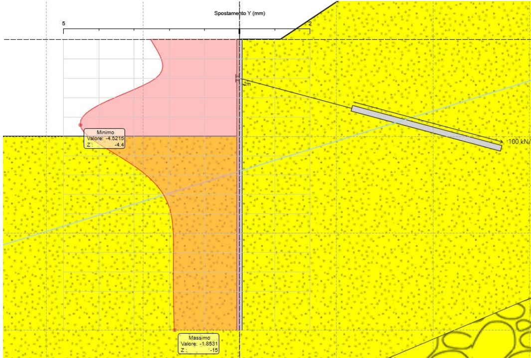
Figura 8.11 Spostamento massimo della paratia
