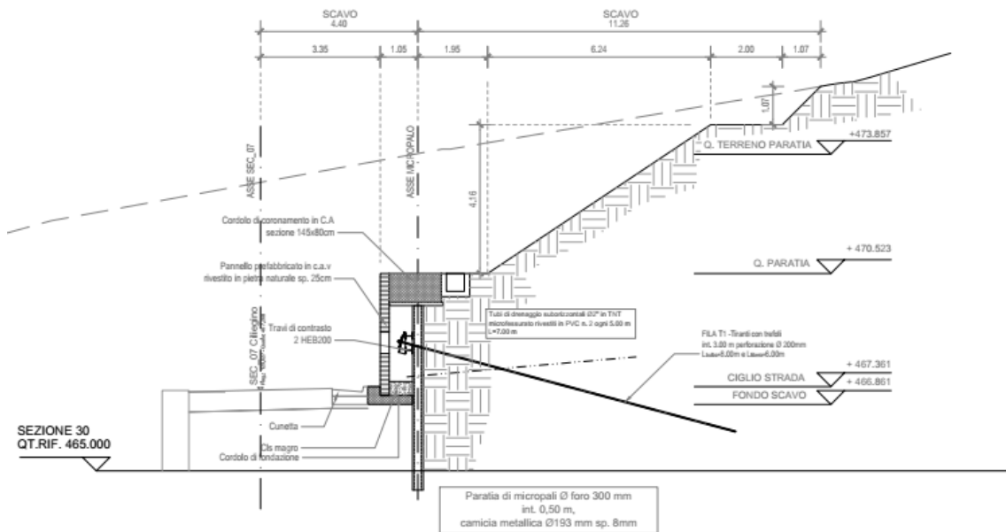
Figura 1.4 Sezioni tipo dell'opera
