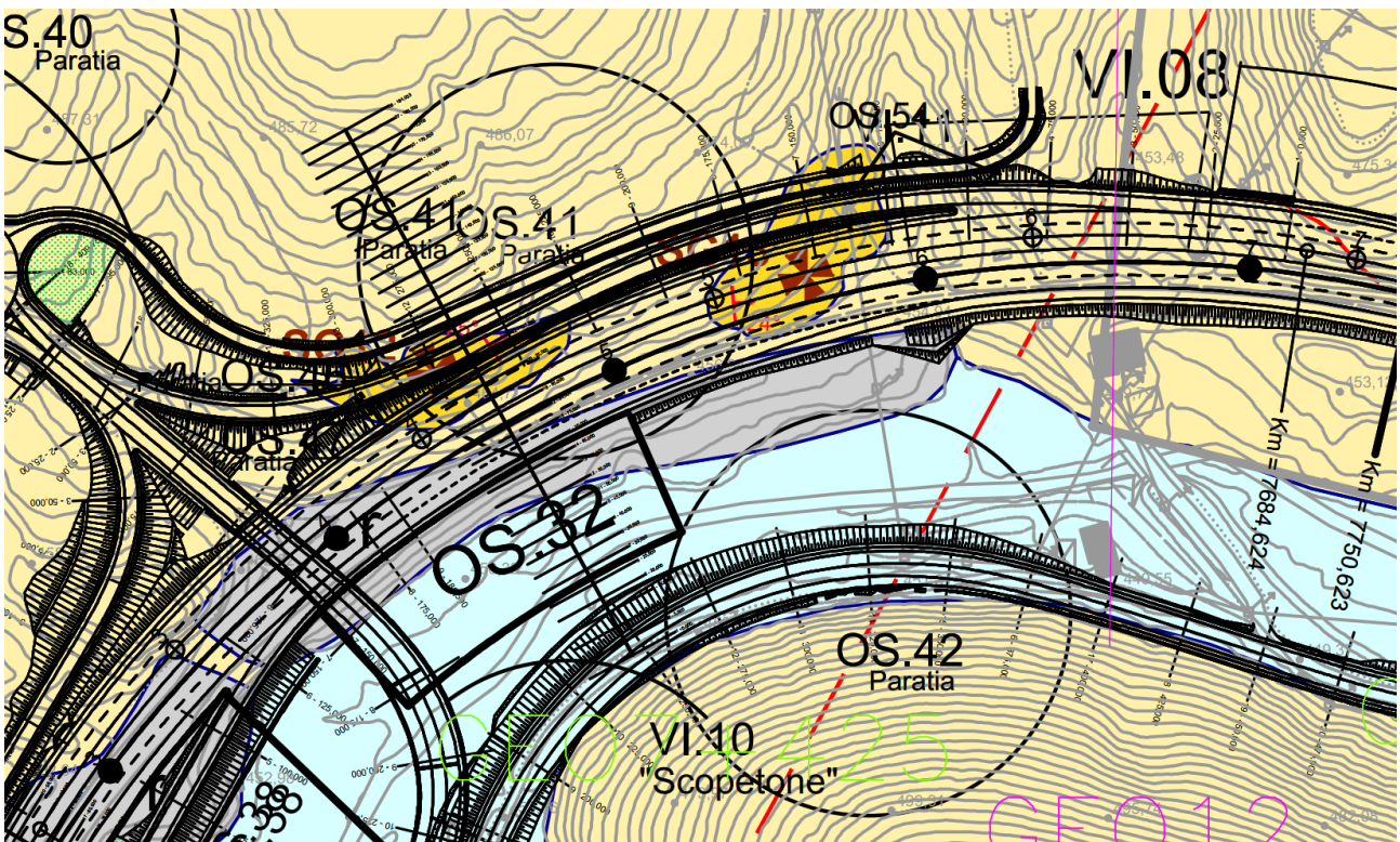
Figura 7.1 Sovrapposizione dell'opera con il profilo in asse
