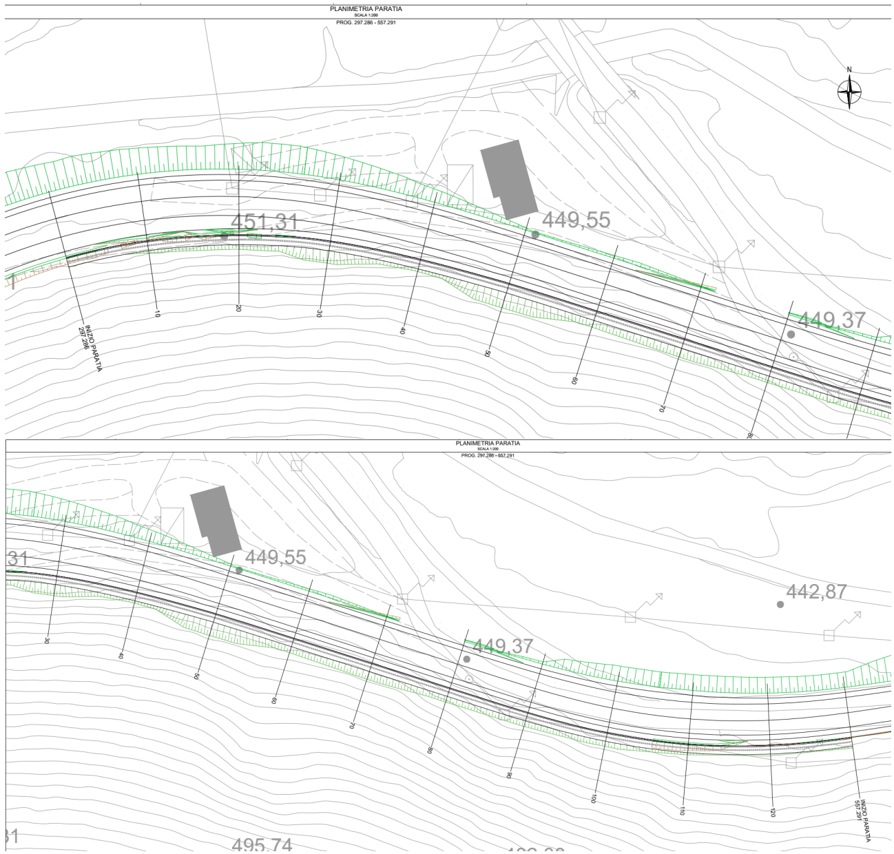
Figura 1.2 Planimetria dell'opera
