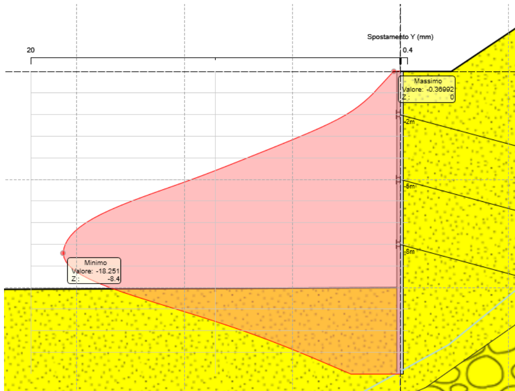
Figura 8.13 Spostamento massimo della paratia
