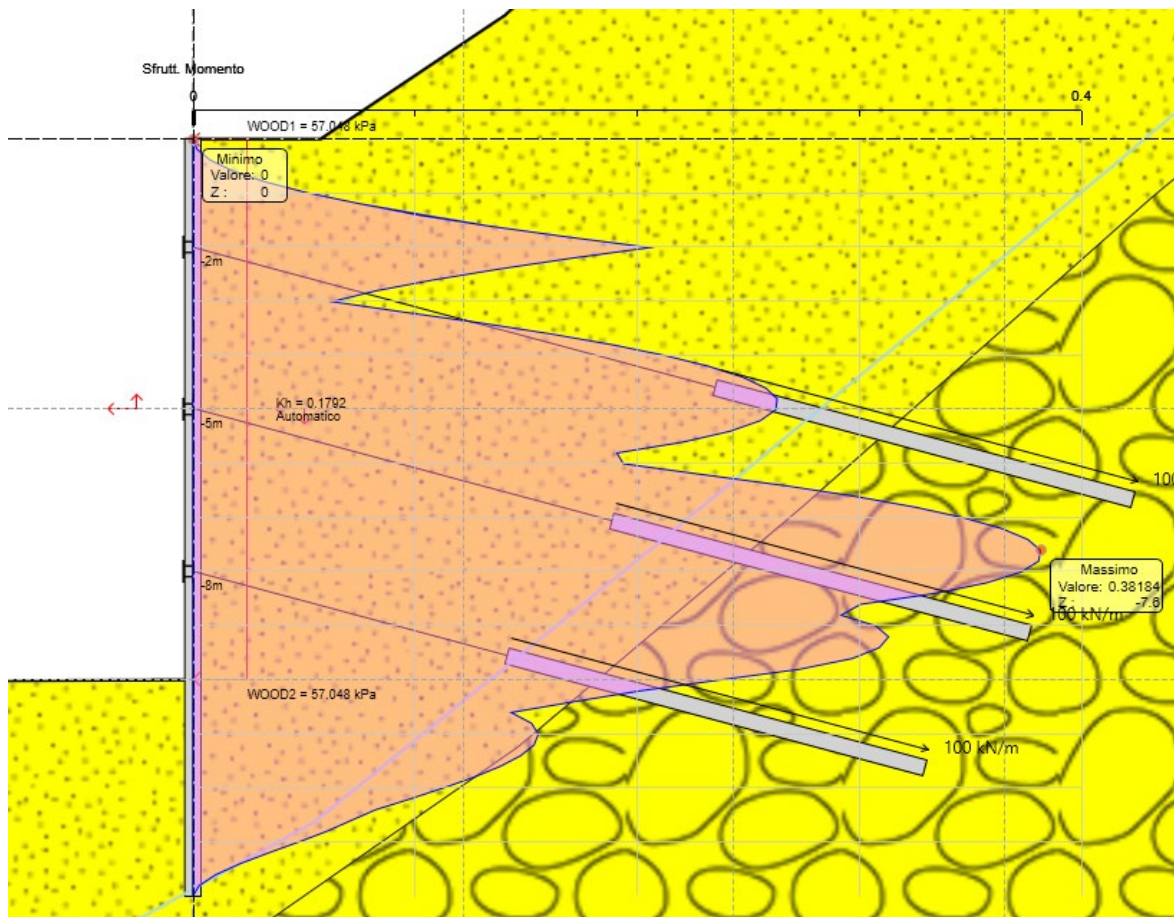
Figura 8.10 Sfruttamento a momento ENV SLU-SISMA
