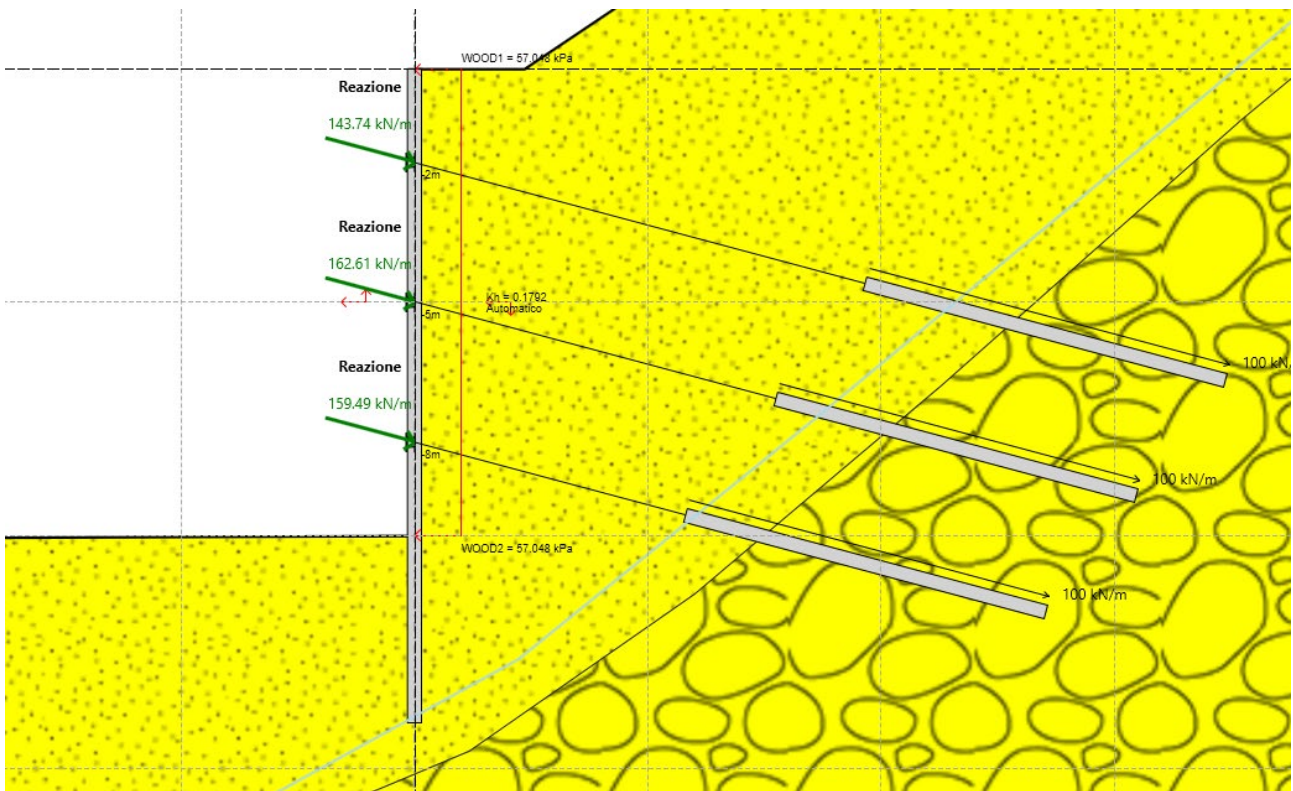
Figura 8.12 Reazioni ai supporti ENV SLU-SISMA
