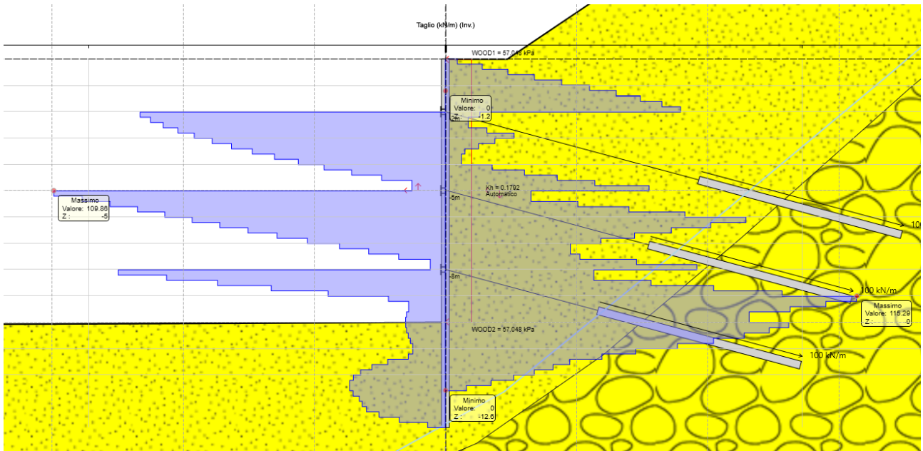
Figura 8.9 Diagramma Taglio ENV SLU-SISMA
