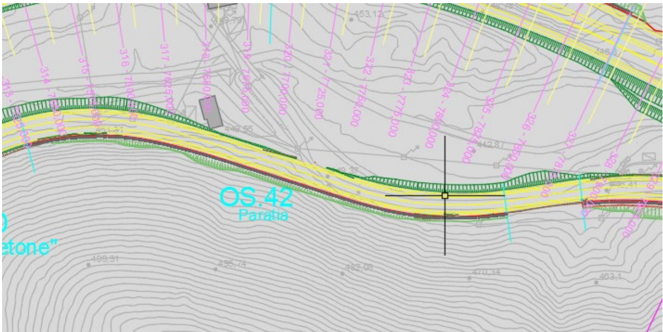
Figura 1.1 KeyPlan dell'opera
