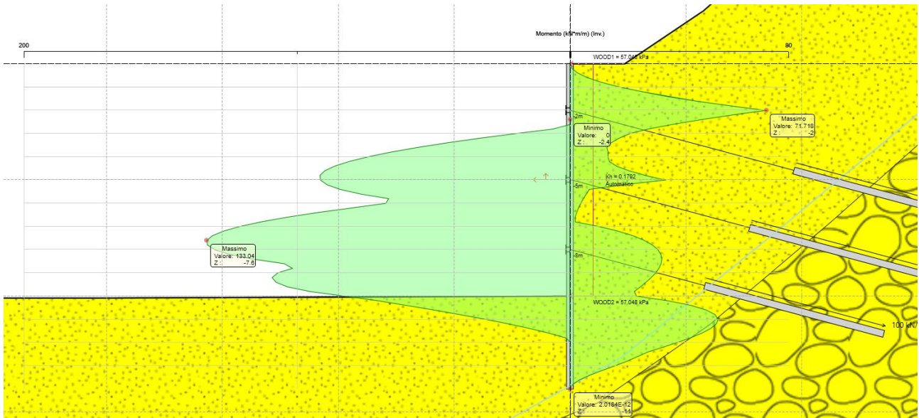
Figura 8.8 Diagramma Momento ENV SLU-SISMA
