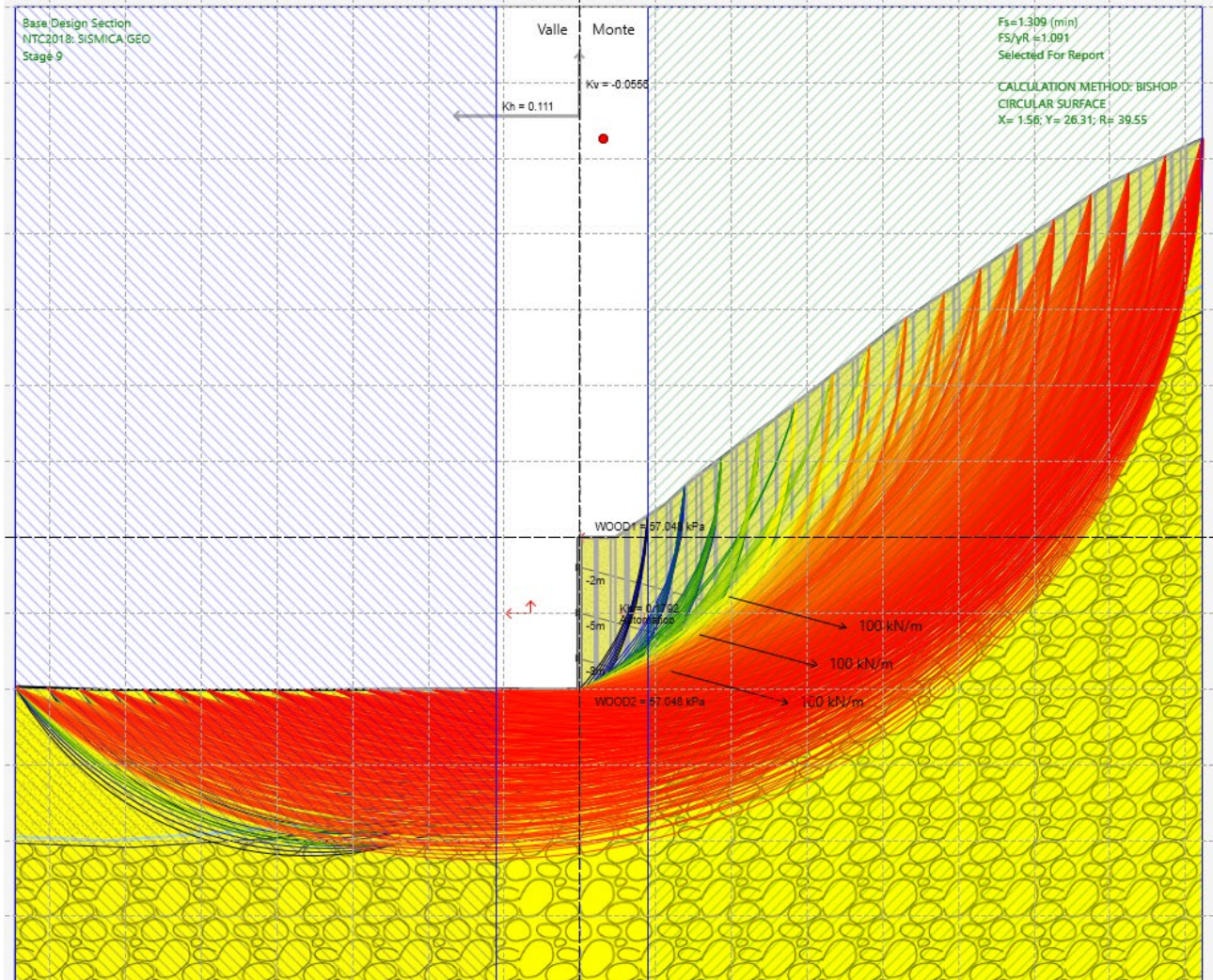
Fig. 16 – Analisi di stabilità SISMICA per il caso A2+M2+SISMA -kv
