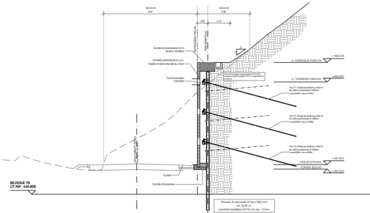
Figura 8.1 Sezione 50 tipo oggetto di verifica
