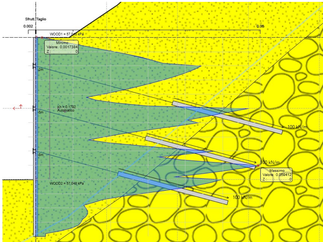
Figura 8.11 Sfruttamento a taglio ENV SLU-SISMA
