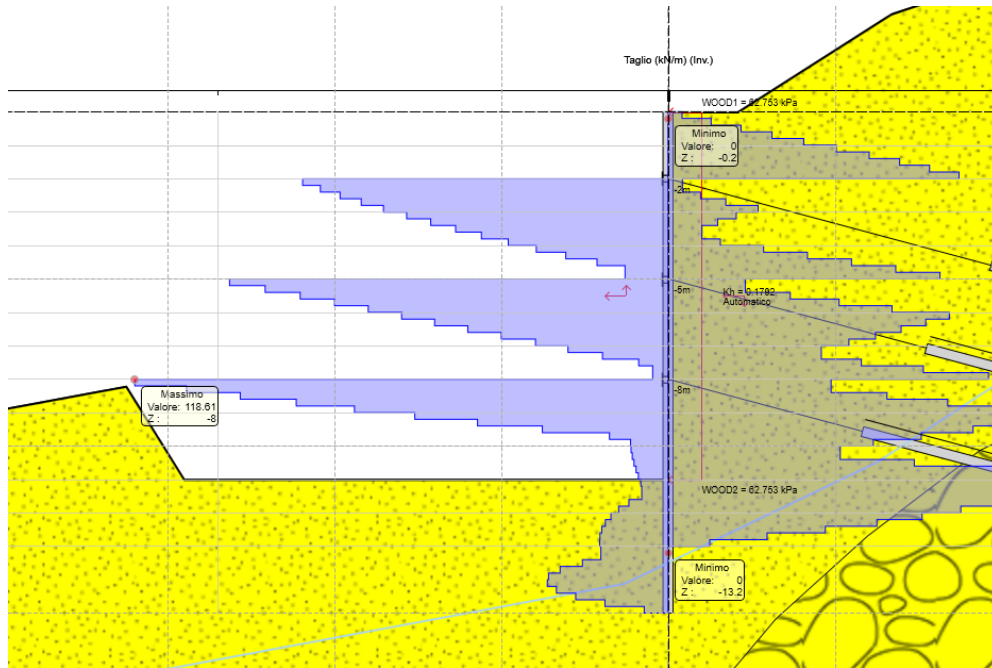
Figura 8.9 Diagramma Taglio ENV SLU-SISMA
