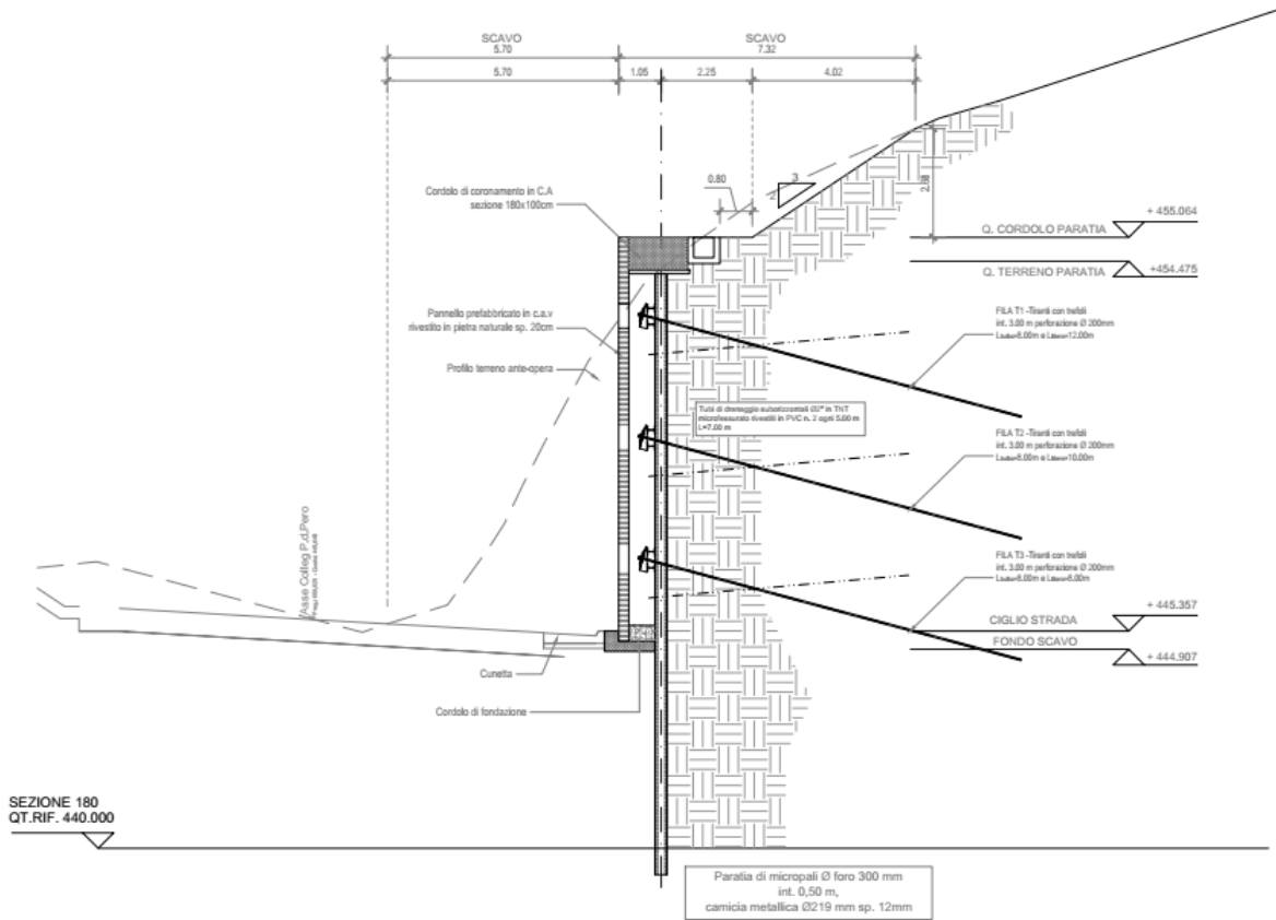
Figura 1.4 Sezioni tipo dell'opera
