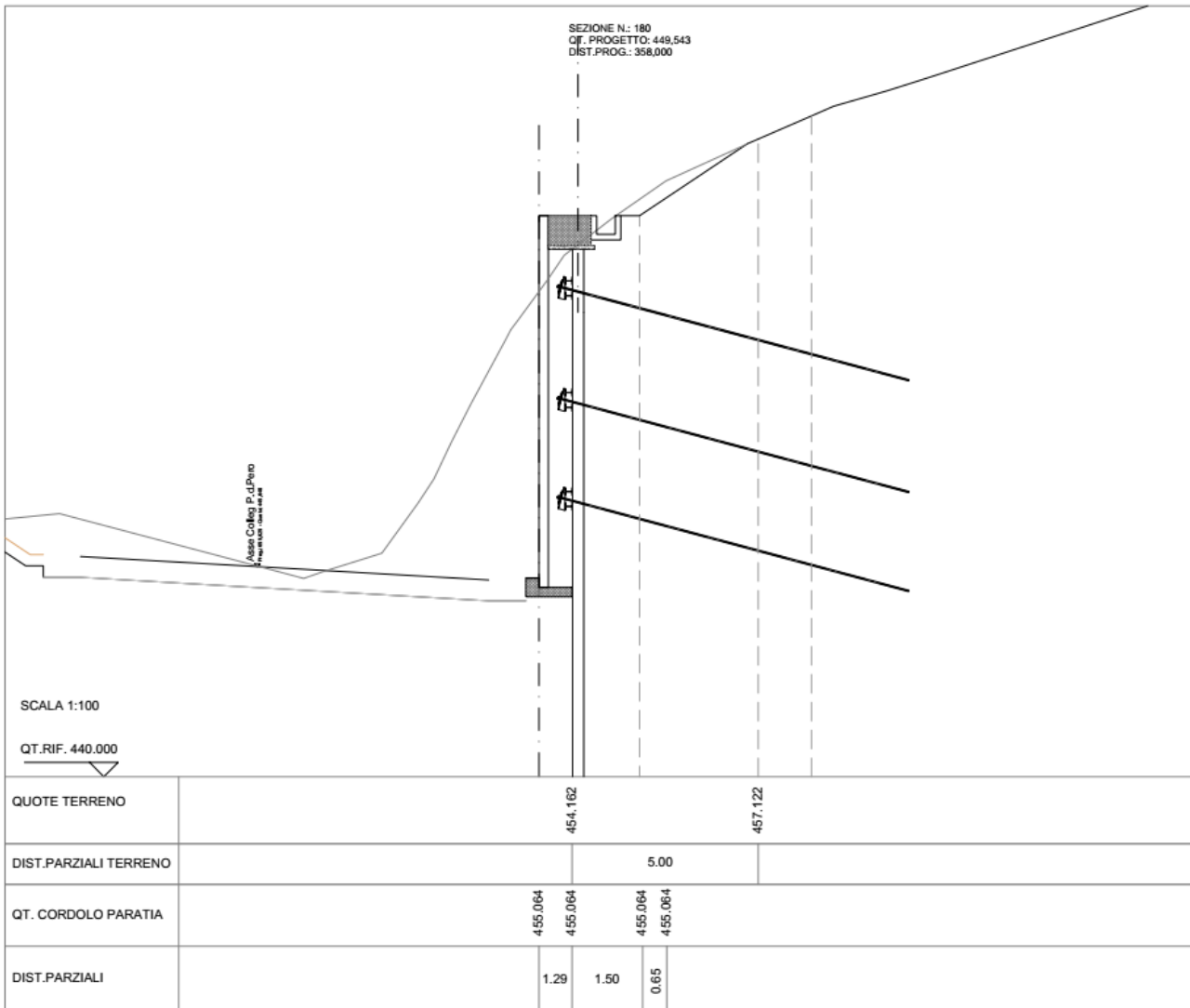
Figura 8.1 Sezione 180 tipo oggetto di verifica
