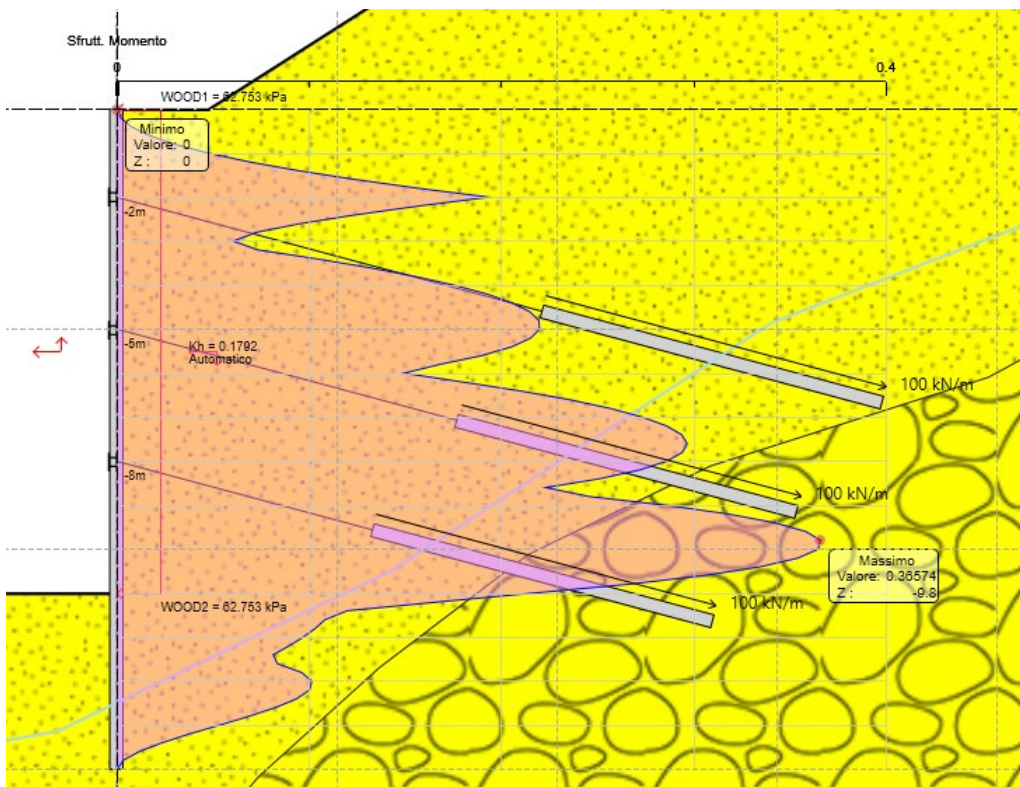
Figura 8.10 Sfruttamento a momento ENV SLU-SISMA
