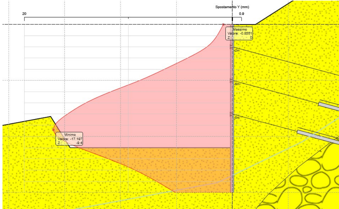
Figura 8.13 Spostamento massimo della paratia
