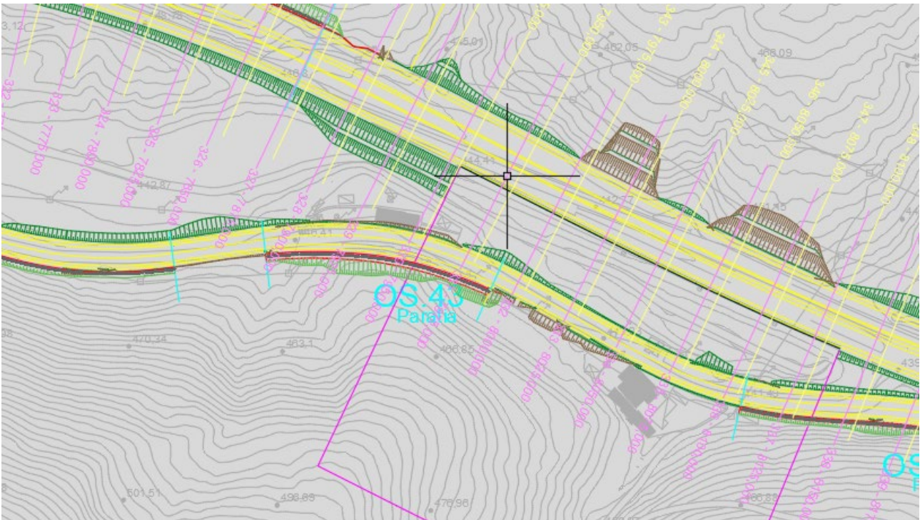
Figura 1.1 KeyPlan dell'opera
