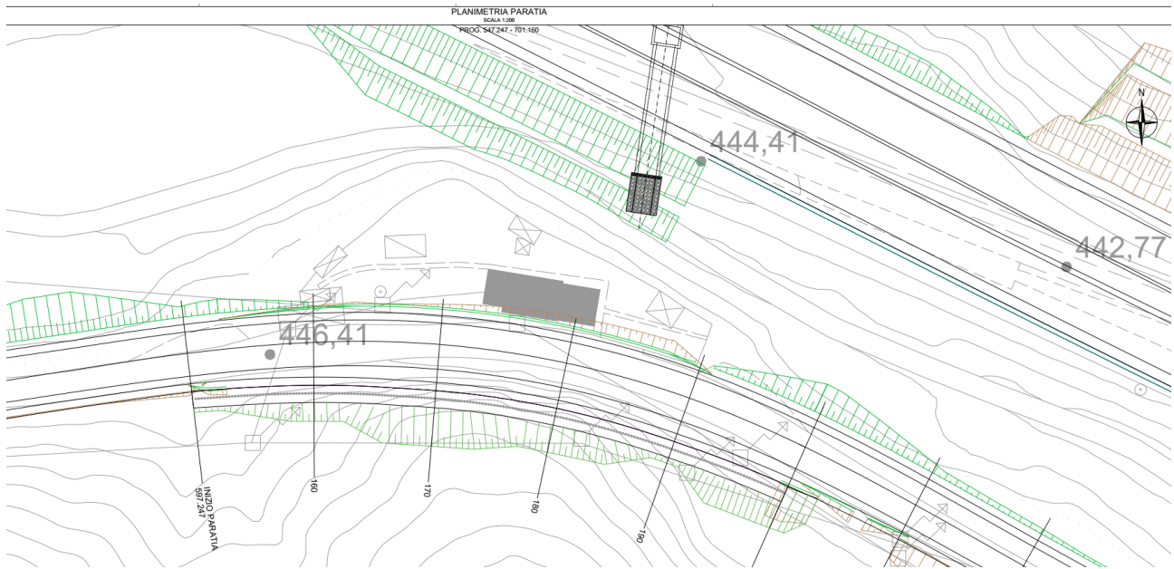
Figura 1.2 Planimetria dell'opera
