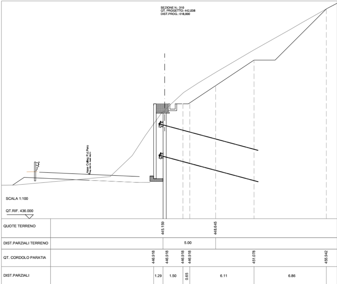
Figura 8.1 Sezione 310 tipo oggetto di verifica
