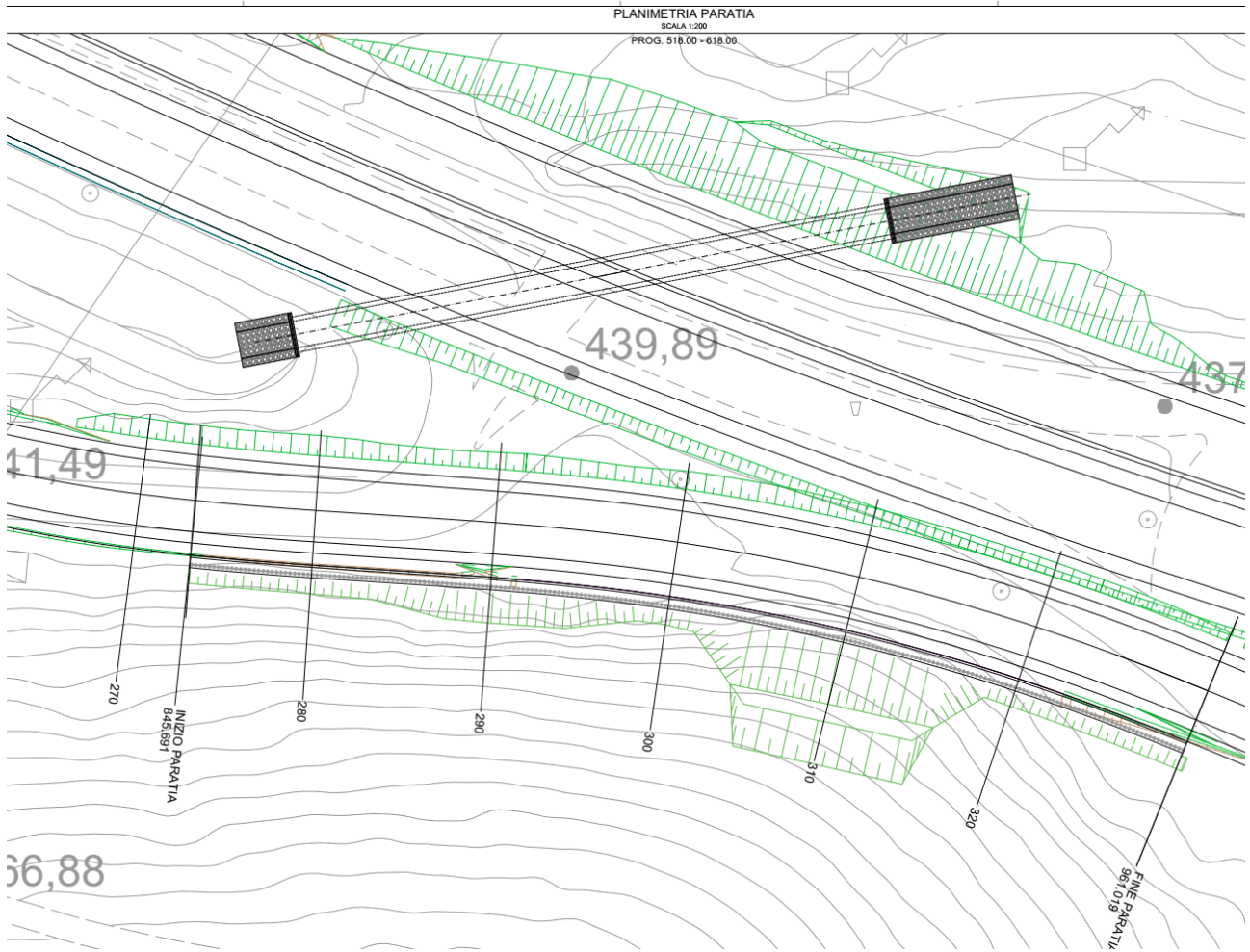
Figura 1.2 Planimetria dell'opera
