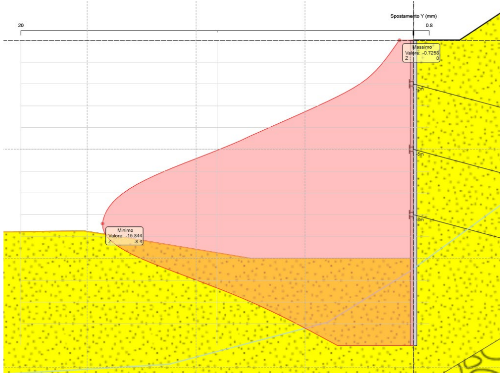
Figura 8.13 Spostamento massimo della paratia
