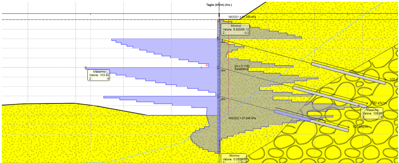
Figura 8.9 Diagramma Taglio ENV SLU-SISMA
