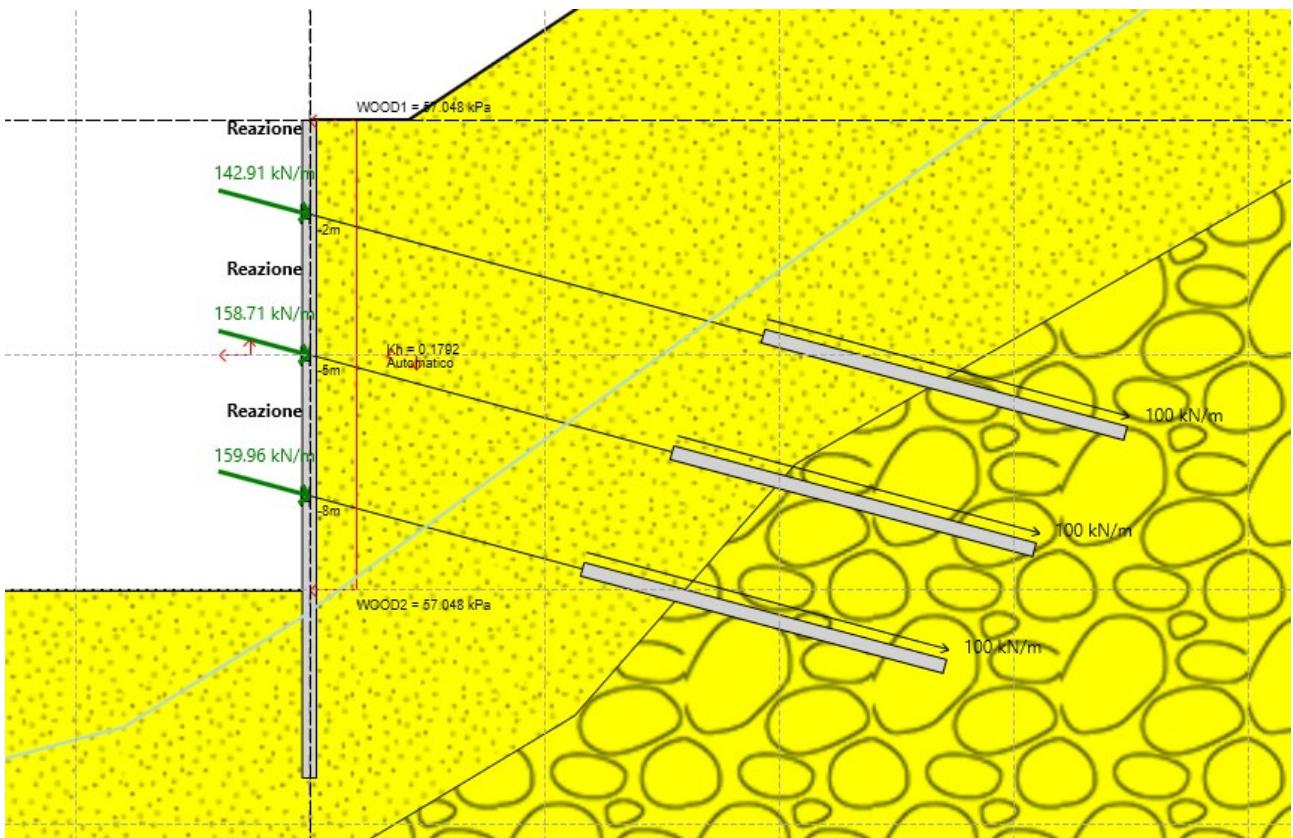
Figura 8.12 Reazioni ai supporti ENV SLU-SISMA
