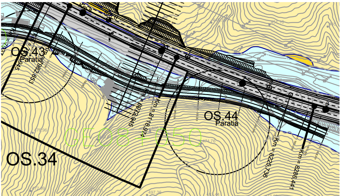
Figura 7.1 Sovrapposizione dell'opera con il profilo in asse
