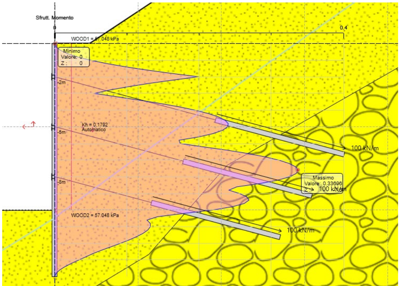
Figura 8.10 Sfruttamento a momento ENV SLU-SISMA
