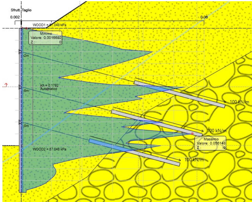
Figura 8.11 Sfruttamento a taglio ENV SLU-SISMA
