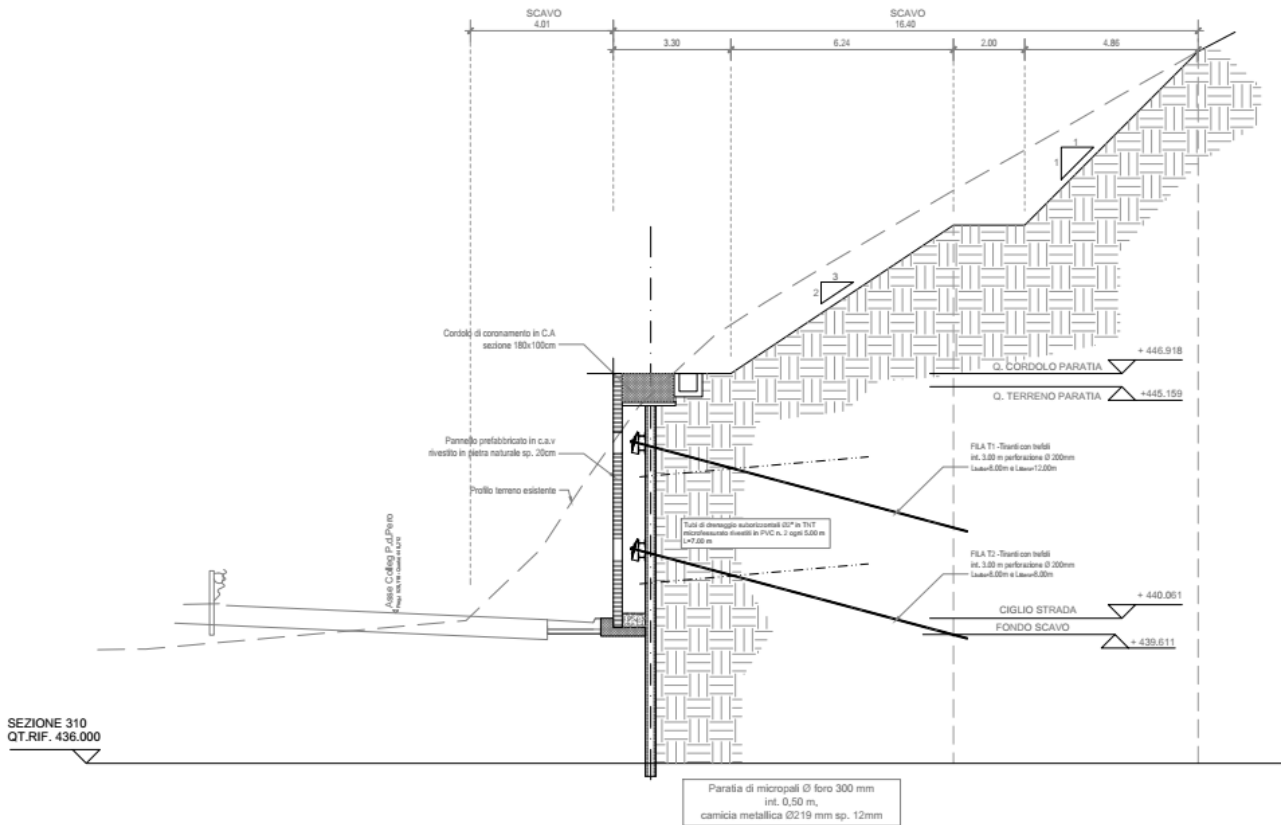
Figura 1.4 Sezioni tipo dell'opera
