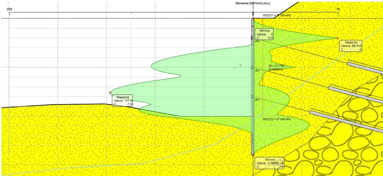
Figura 8.8 Diagramma Momento ENV SLU-SISMA
