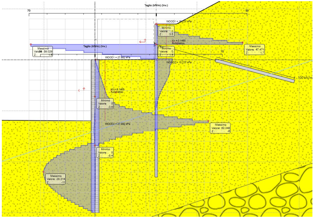
Figura 8.8 Diagramma Taglio ENV SLU-SISMA
