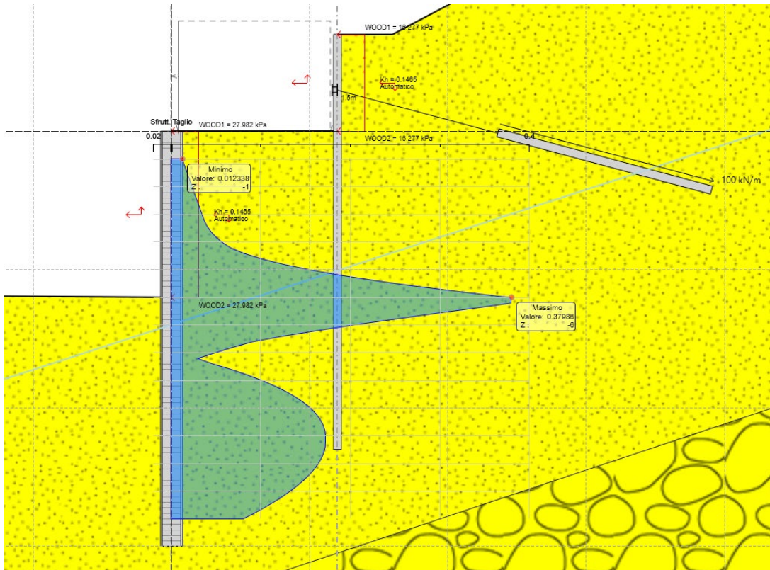
Figura 8.11 Sfruttamento a taglio ENV SLU-SISMA
