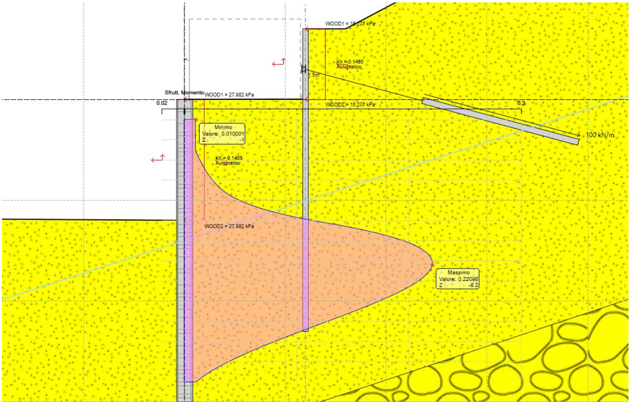
Figura 8.9 Sfruttamento a momento ENV SLU-SISMA
