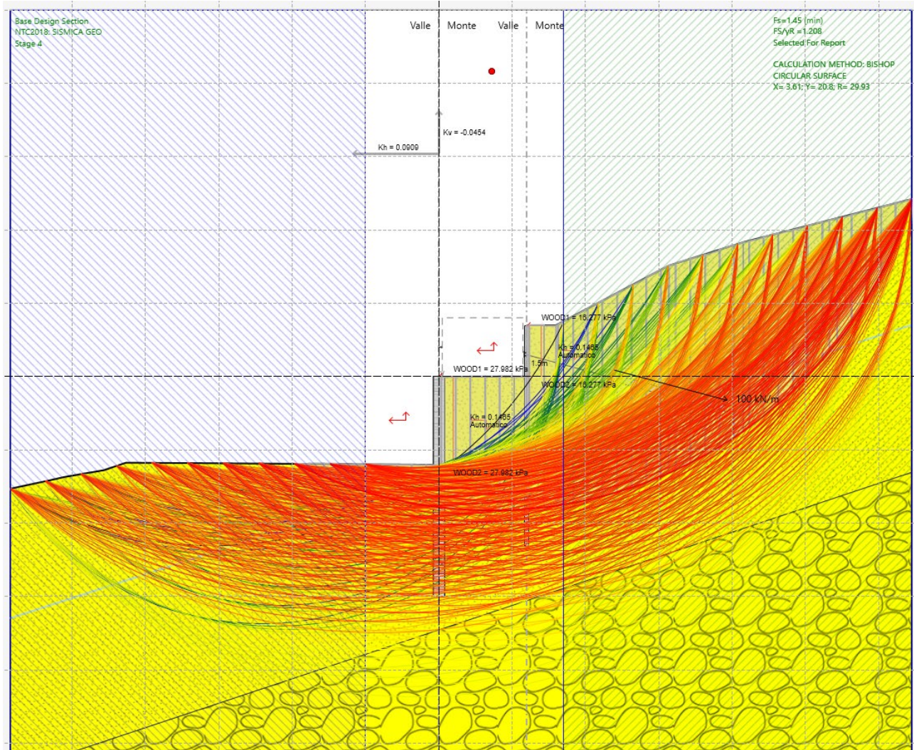
Fig. 17 – Analisi di stabilità SISMICA per il caso A2+M2+SISMA -kv
