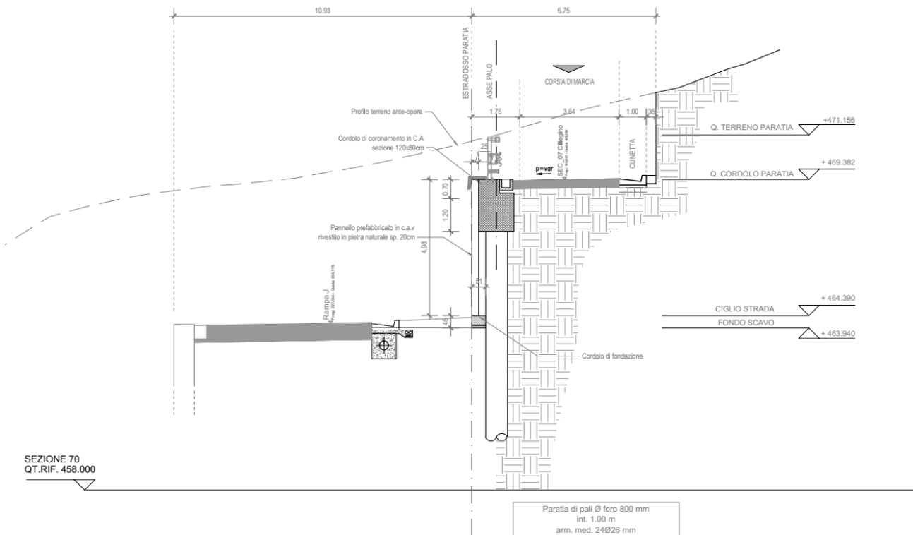
Figura 1.4 Sezioni tipo dell'opera
