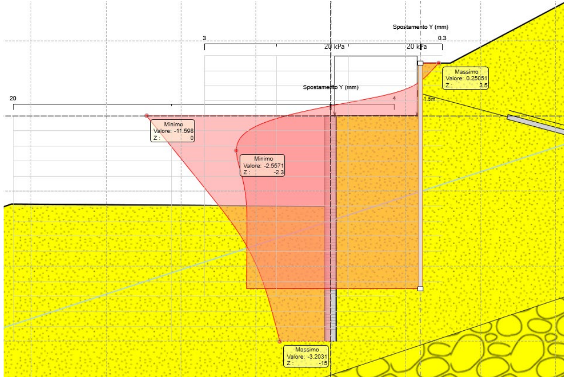
Figura 8.14 Spostamento massimo della paratia
