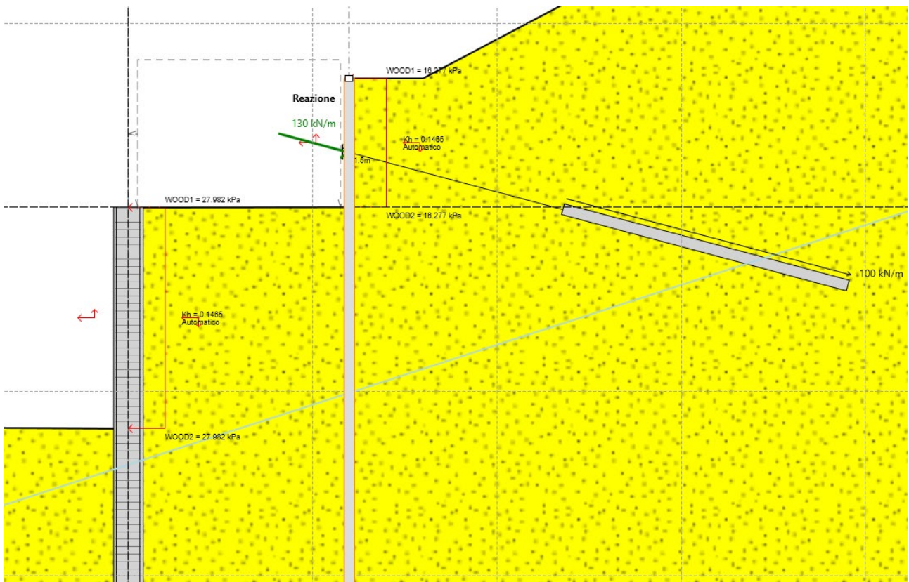
Figura 8.13 Reazioni ai supporti ENV SLU-SISMA
