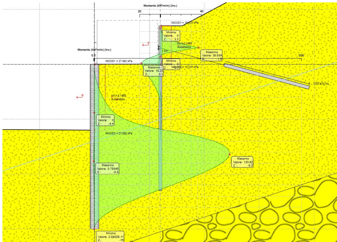
Figura 8.7 Diagramma Momento ENV SLU-SISMA
