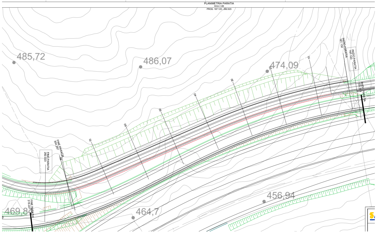
Figura 1.2 Planimetria dell'opera
