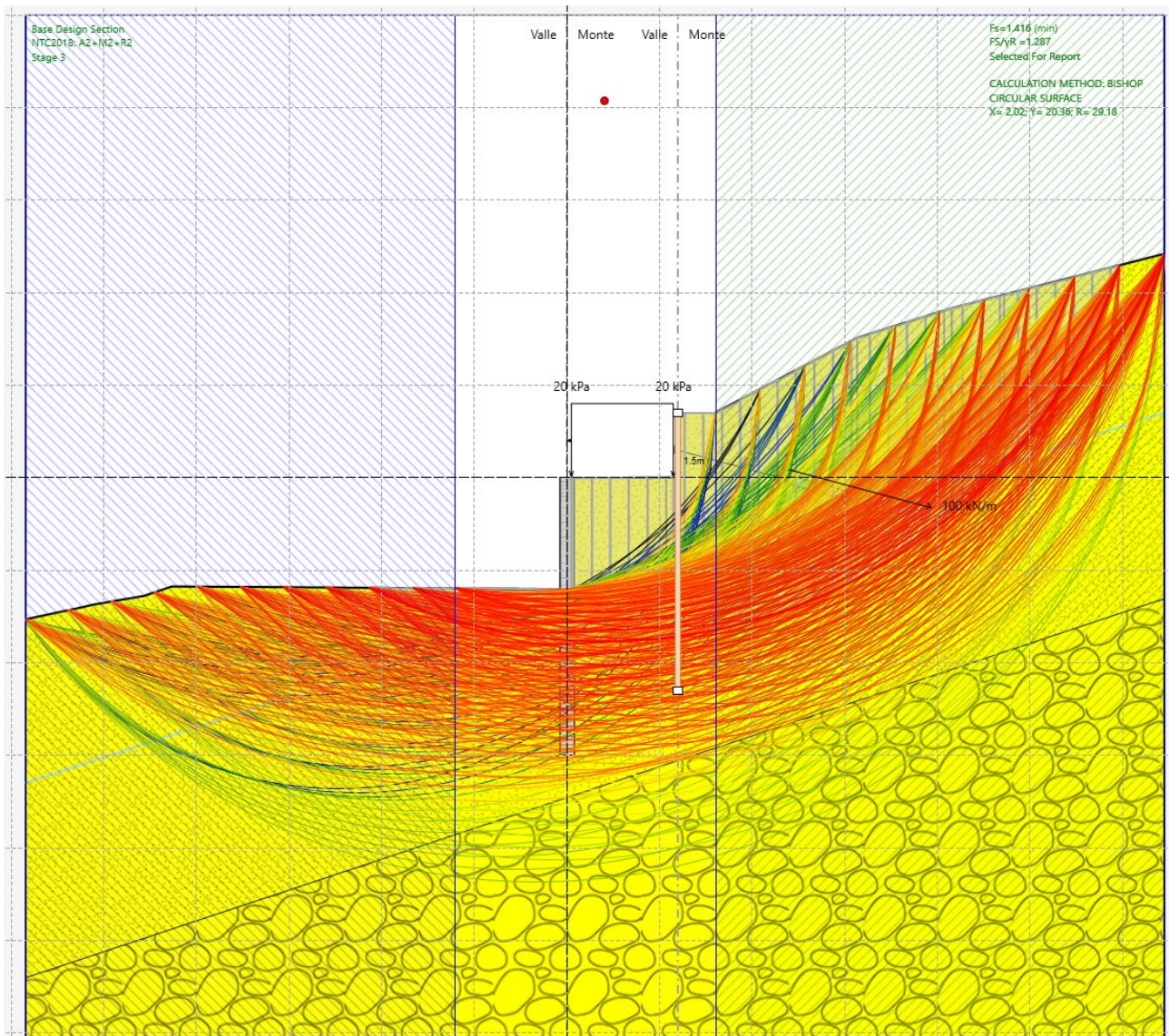
Fig. 15 – Analisi di stabilità STATICA per il caso A2+M2+R2
