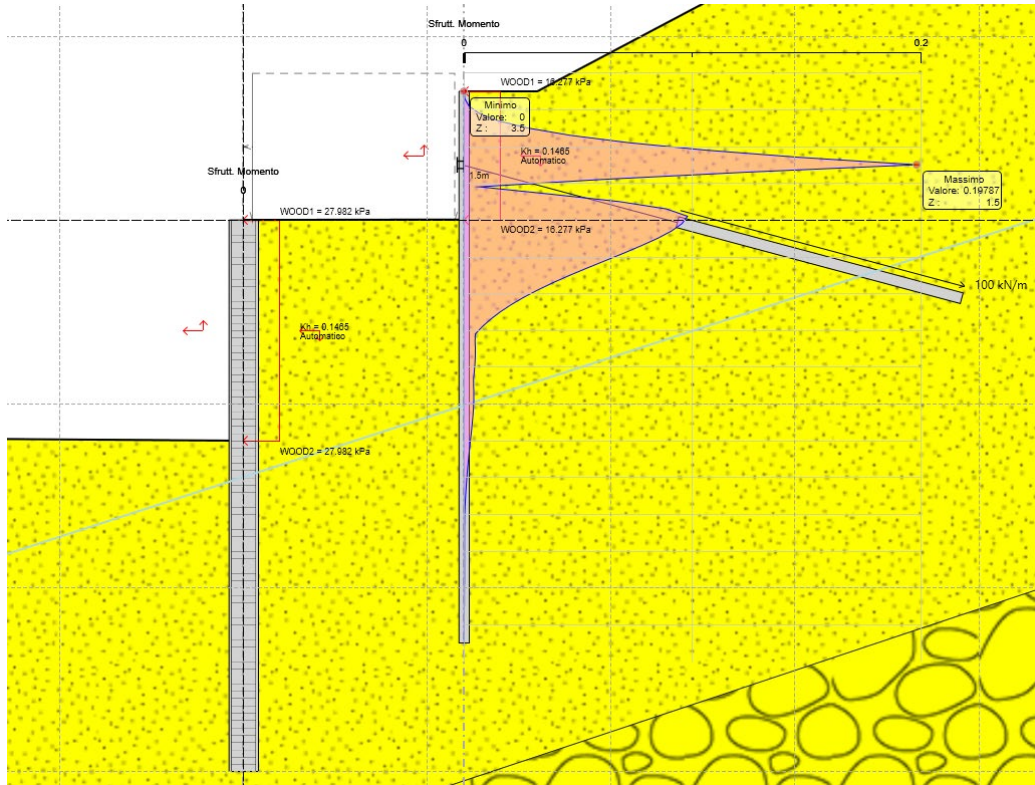
Figura 8.10 Sfruttamento a momento ENV SLU-SISMA
