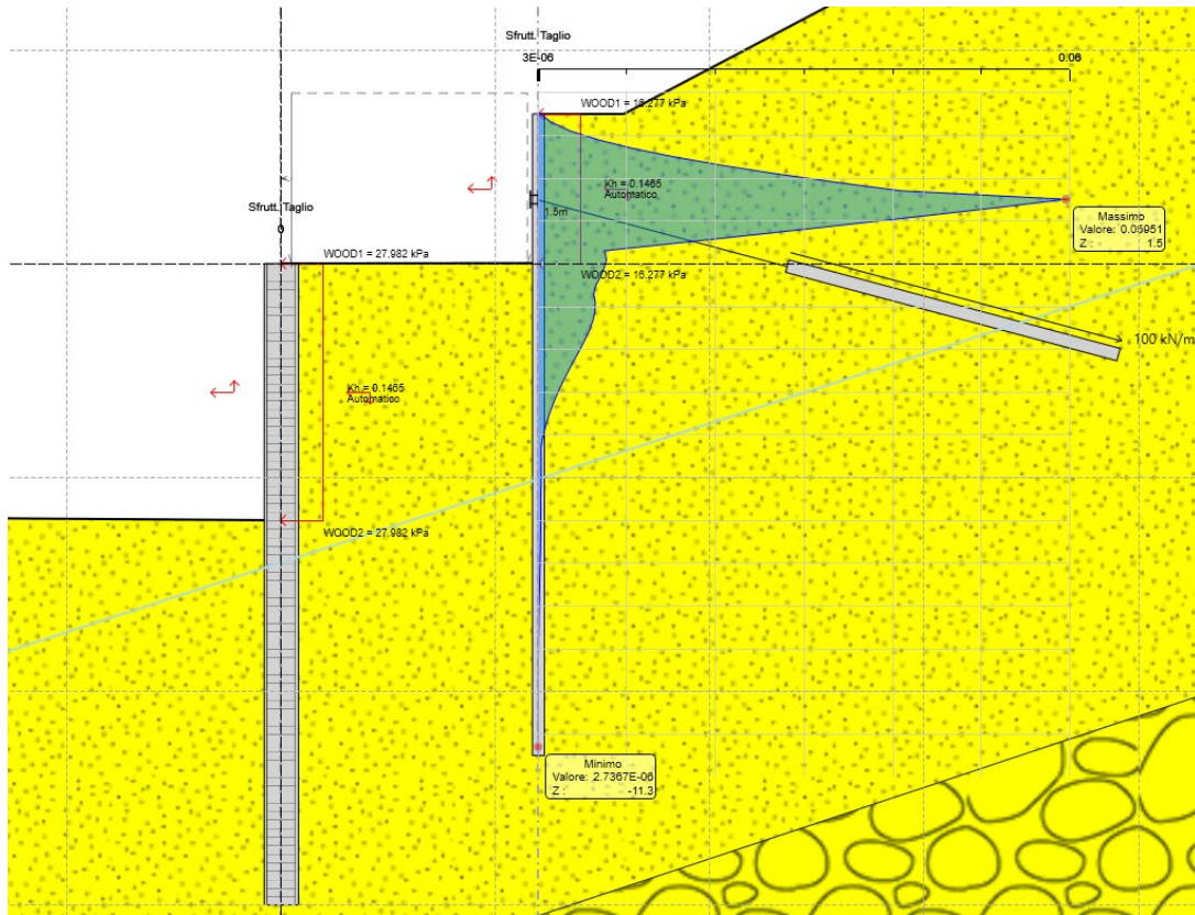
Figura 8.12 Sfruttamento a taglio ENV SLU-SISMA
