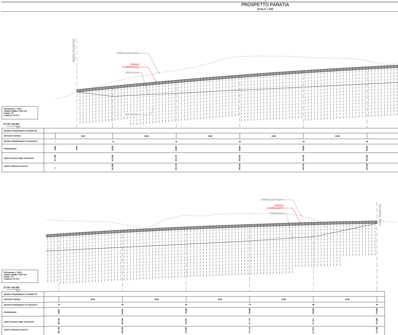
Figura 1.3 Profilo dell'opera
