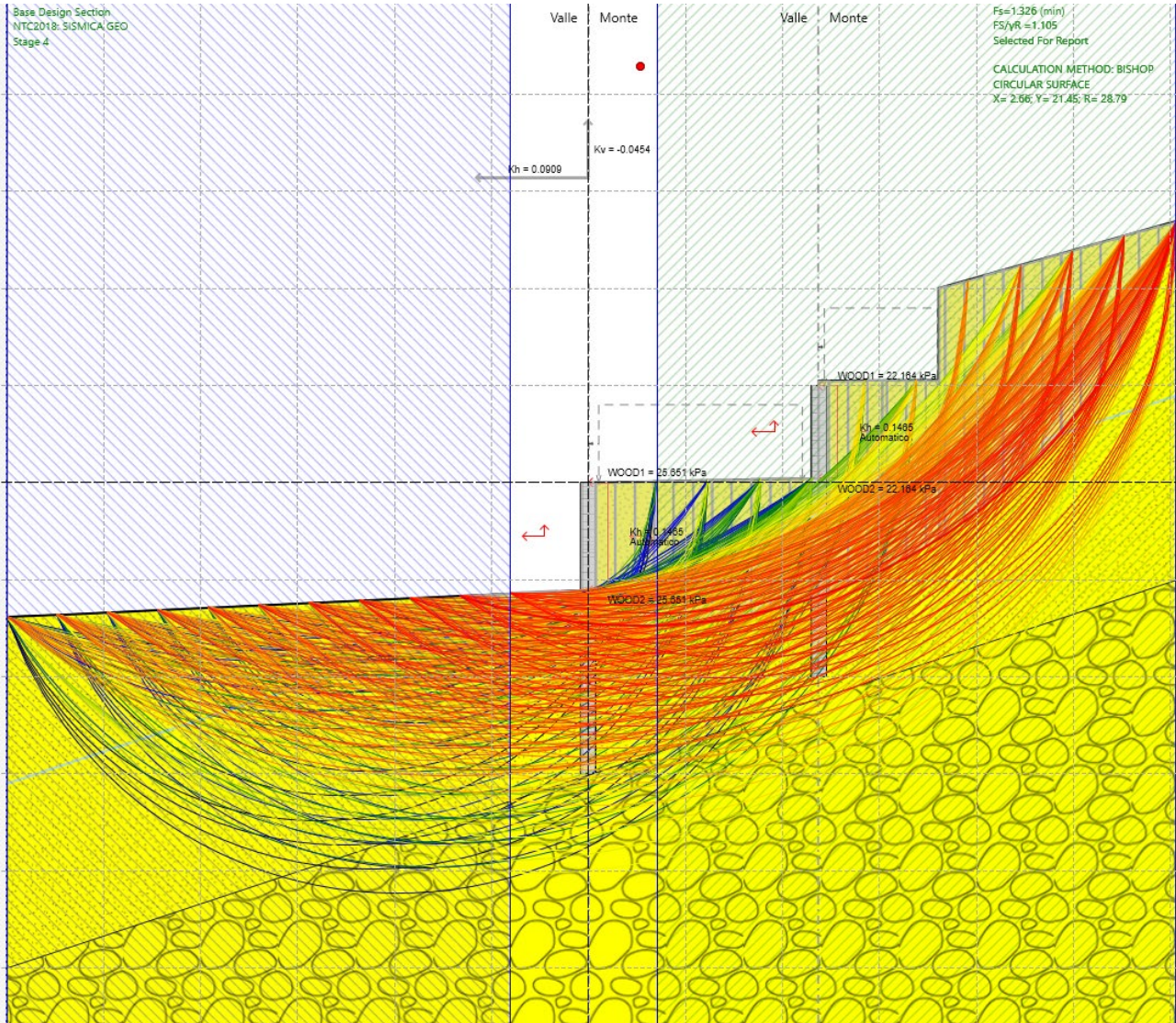
Fig. 14 – Analisi di stabilità SISMICA per il caso A2+M2+SISMA -kv
