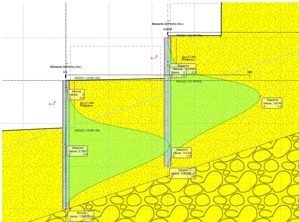
Figura 8.7 Diagramma Momento ENV SLU-SISMA
