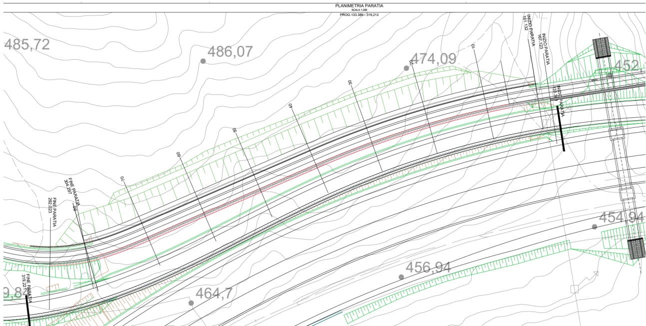
Figura 1.2 Planimetria dell'opera
