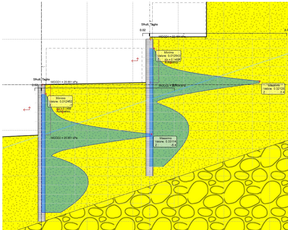
Figura 8.10 Sfruttamento a taglio ENV SLU-SISMA
