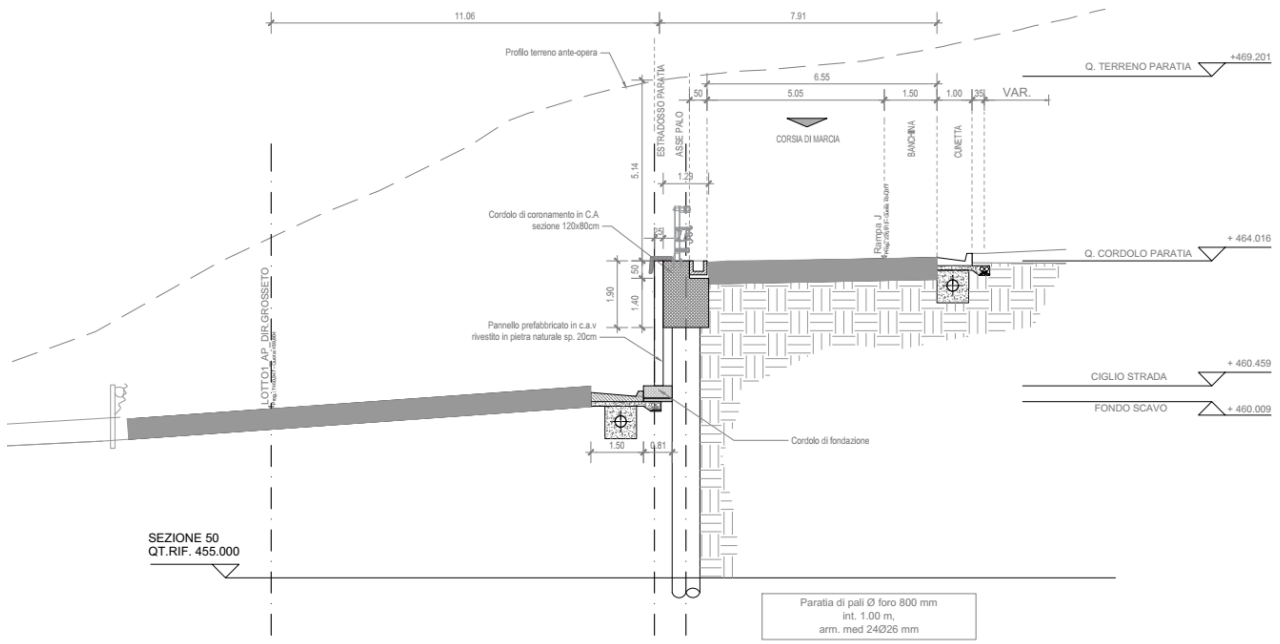
Figura 1.4 Sezioni tipo dell'opera
