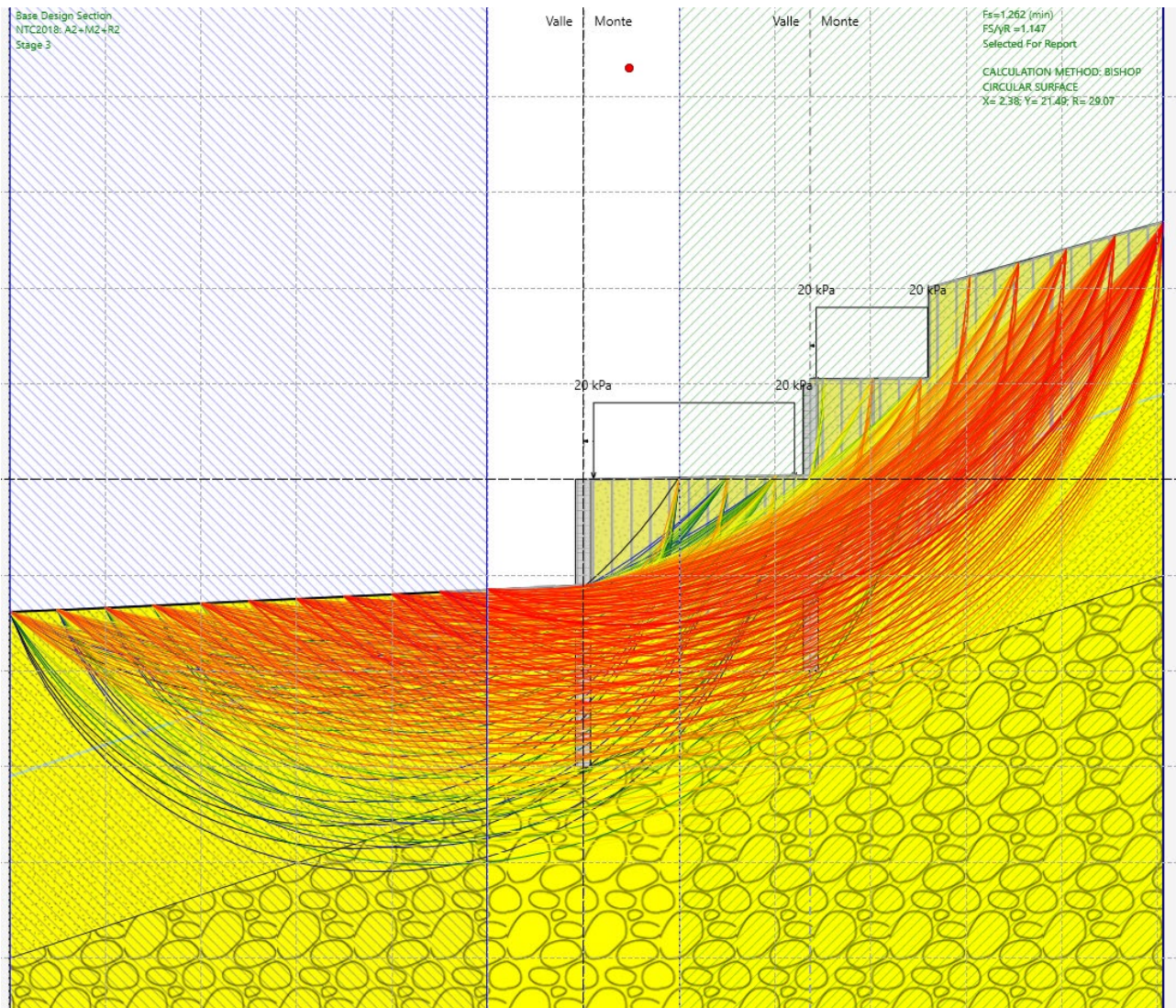
Fig. 12 – Analisi di stabilità STATICA per il caso A2+M2+R2
