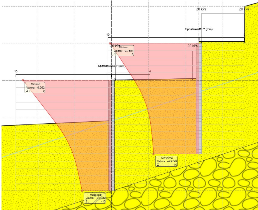
Figura 8.11 Spostamento massimo della paratia
