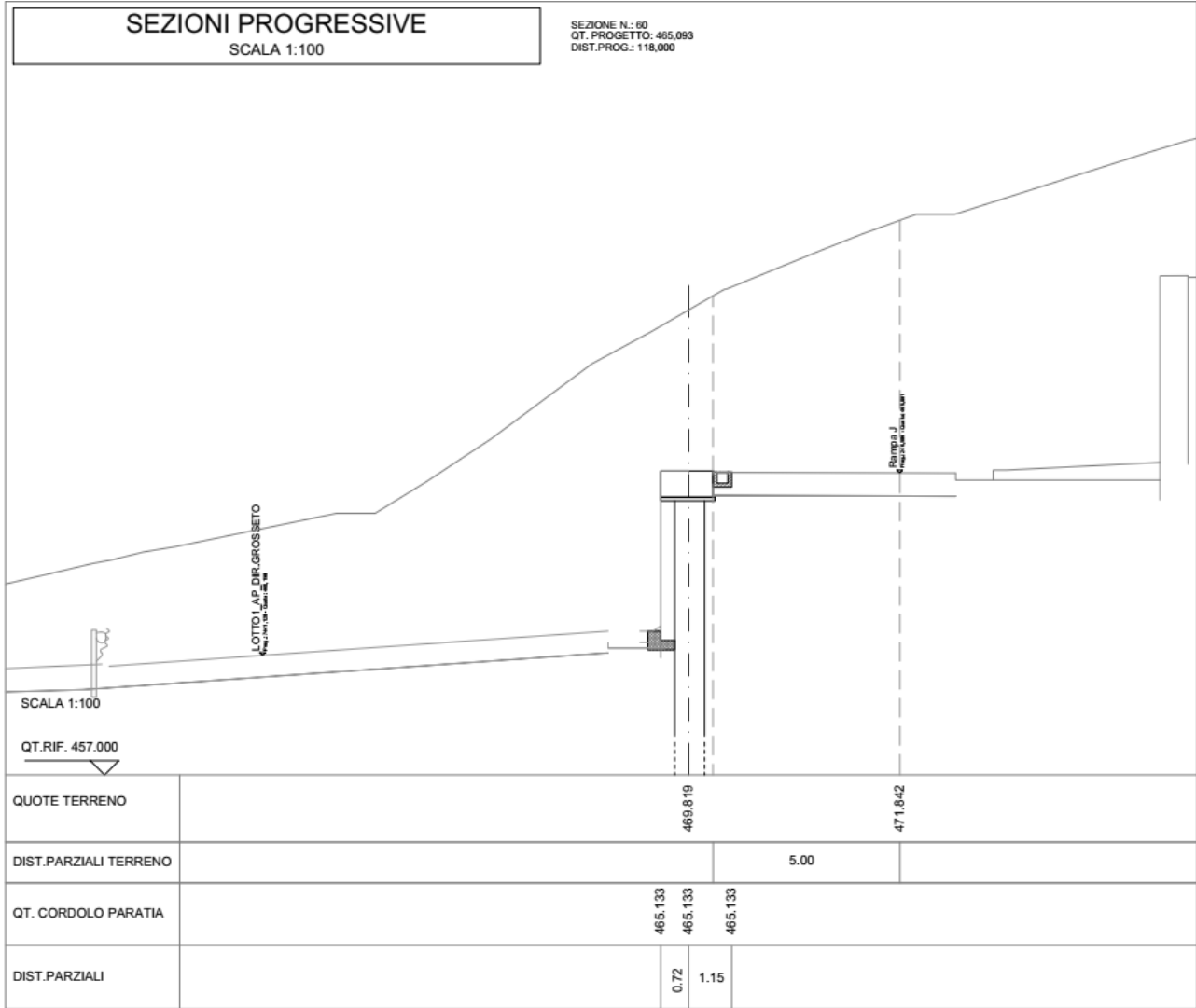
Figura 8.1 Sezione 60 tipo oggetto di verifica
