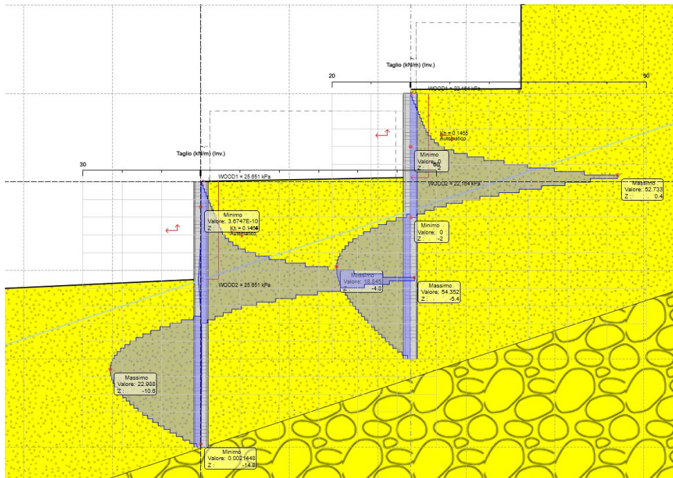
Figura 8.8 Diagramma Taglio ENV SLU-SISMA
