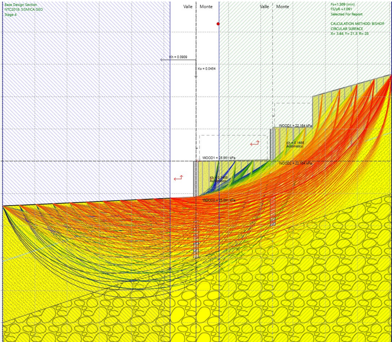
Fig. 13 – Analisi di stabilità SISMICA per il caso A2+M2+SISMA +kv
