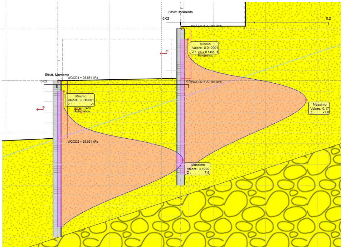
Figura 8.9 Sfruttamento a momento ENV SLU-SISMA
