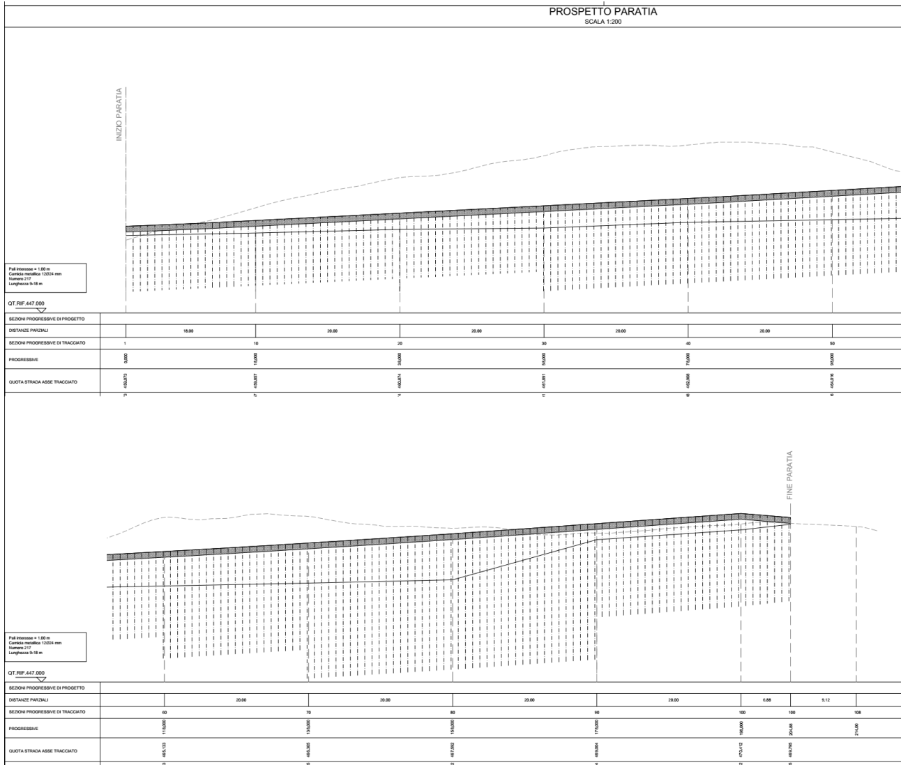
Figura 1.3 Profilo dell'opera
