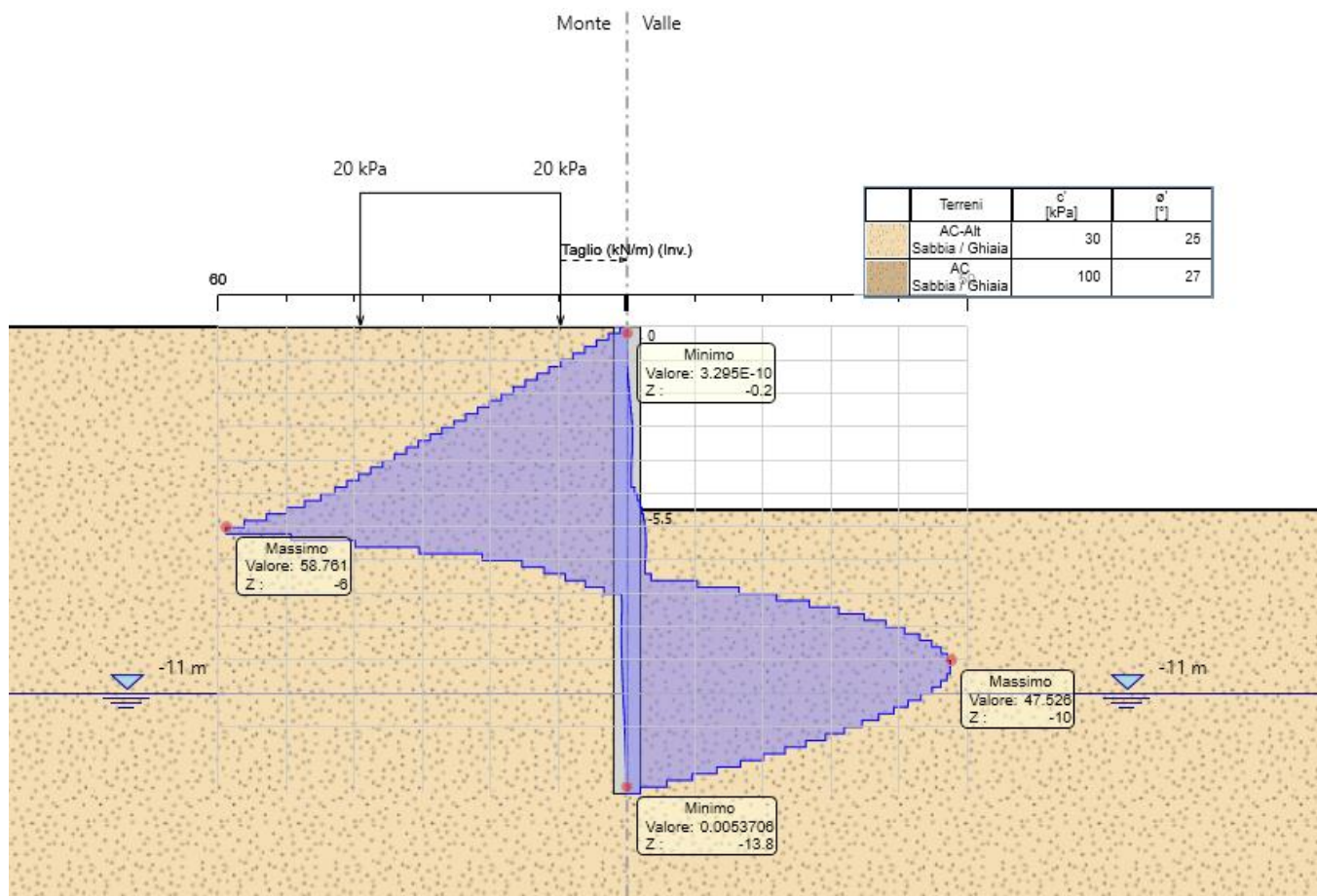
Figura 8.10 Diagramma Taglio ENV SLU-SISMA
