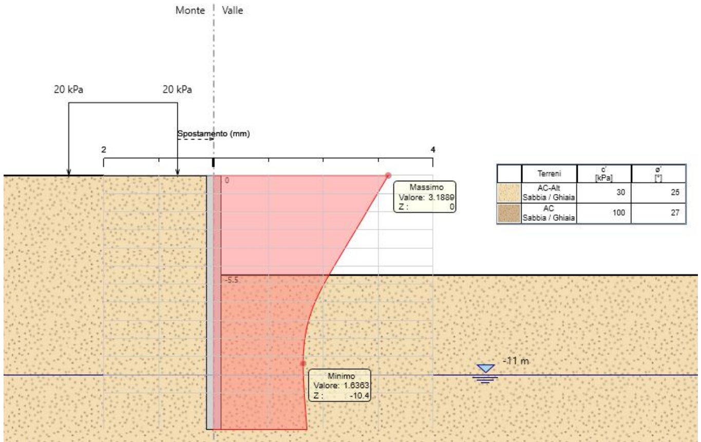
Figura 8.14 Spostamento massimo della paratia
