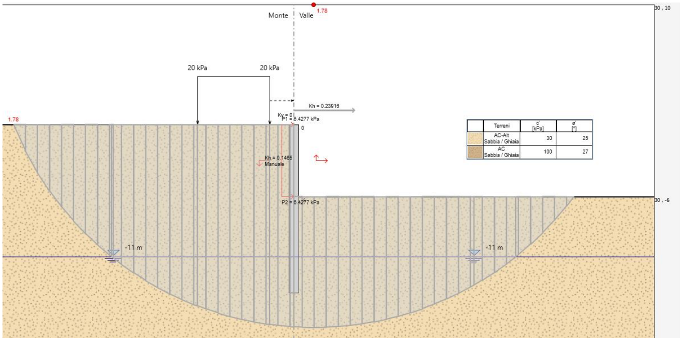
Fig. 16 – Analisi di stabilità SISMICA per il caso A2+M2+SISMA +kv
