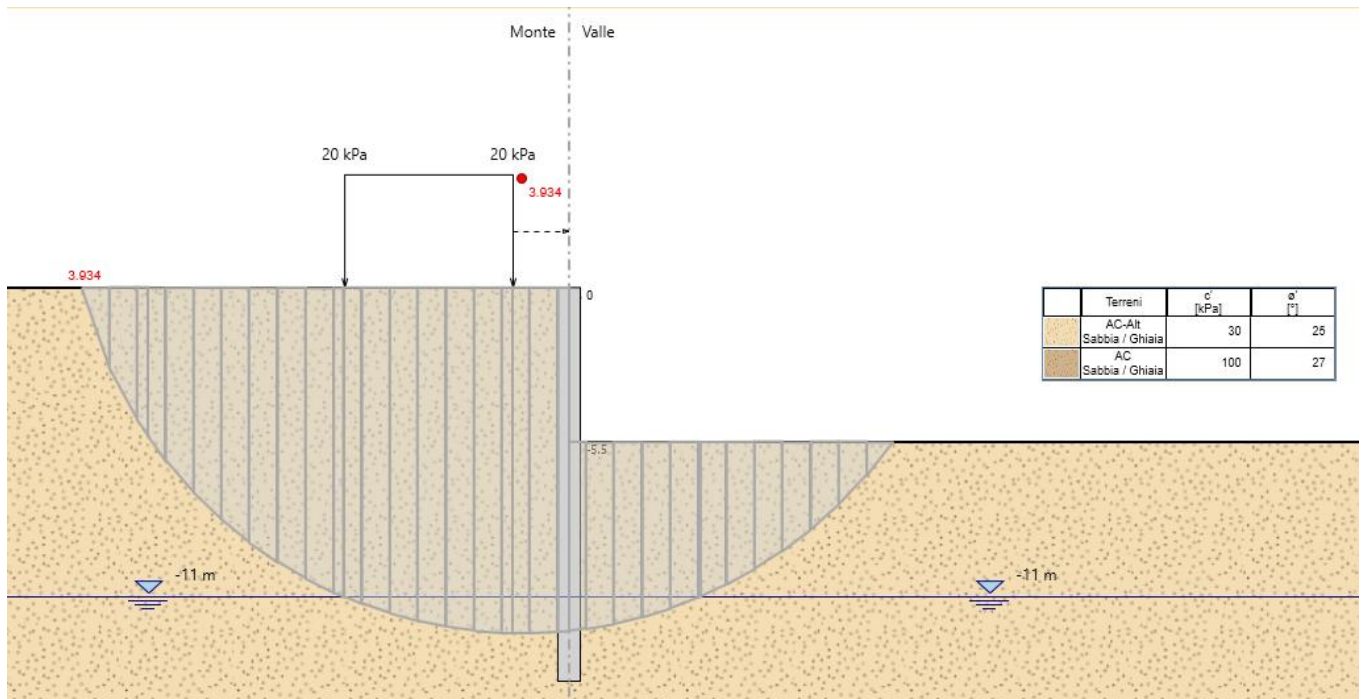
Fig. 15 – Analisi di stabilità STATICA per il caso A2+M2+R2
