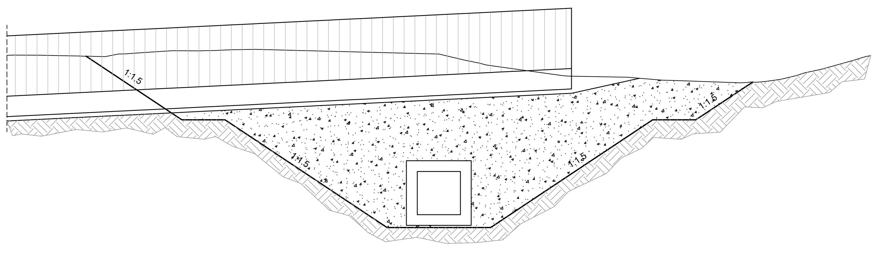
TOMBINO TM11 SEZIONE TRASVERSALE B-B SCALA 1:100
