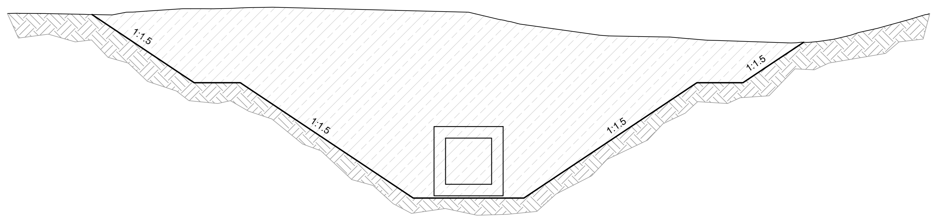
TOMBINO TM11 SEZIONE TRASVERSALE B-B SCALA 1:100
