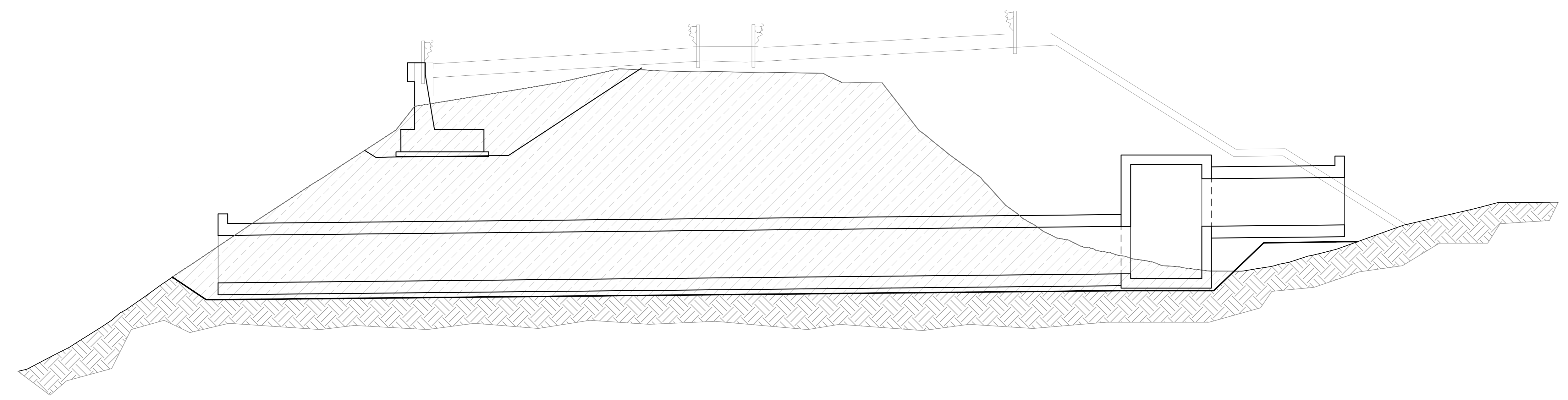
TOMBINO TM11 SEZIONE LONGITUDINALE A-A SCALA 1:100
