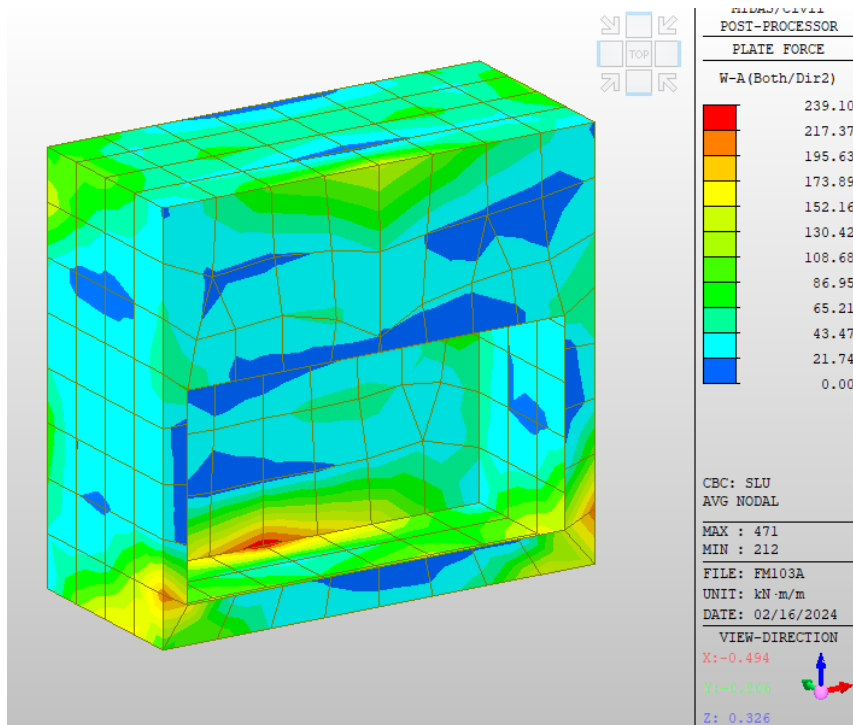
Figura 14 Wood e Armer dir 2 SLU
