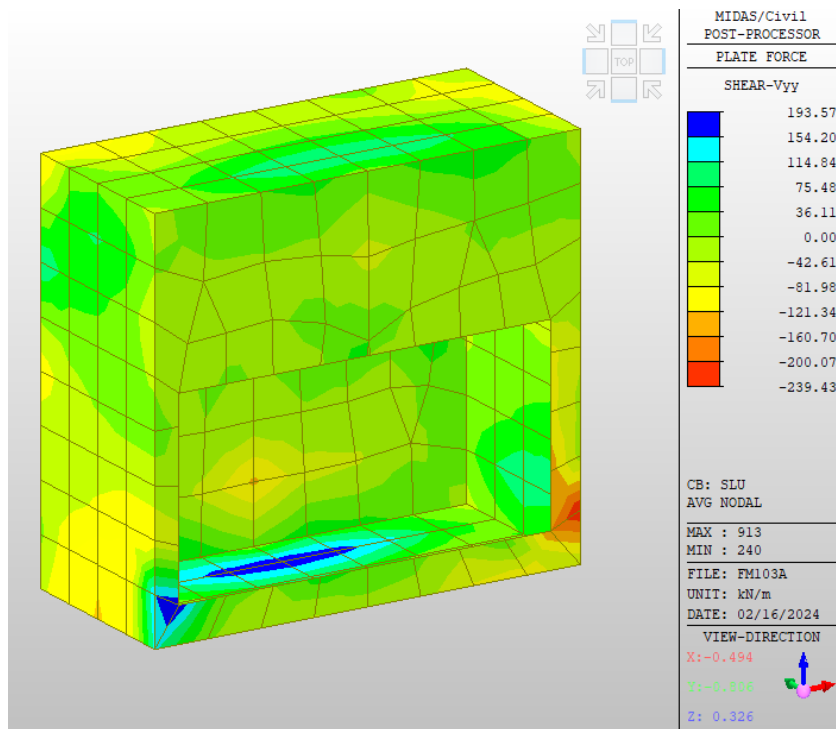
Figura 18 Taglio Vyy SLU
