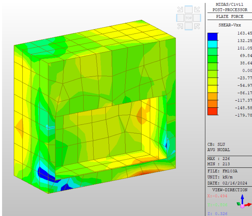
Figura 17 Taglio Vxx SLU
