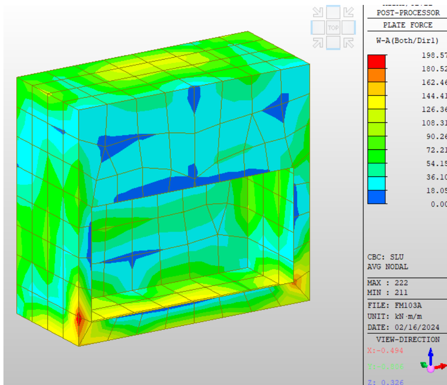
Figura 13 Wood e Armer dir 1 SLU
