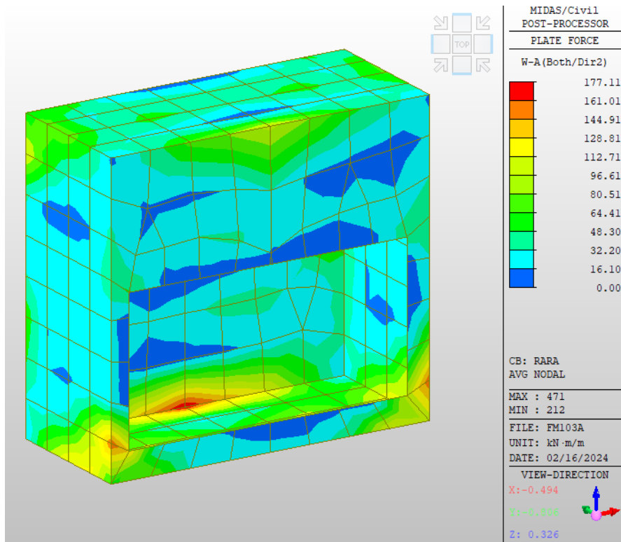
Figura 16 Wood e Armer dir 2 SLE
