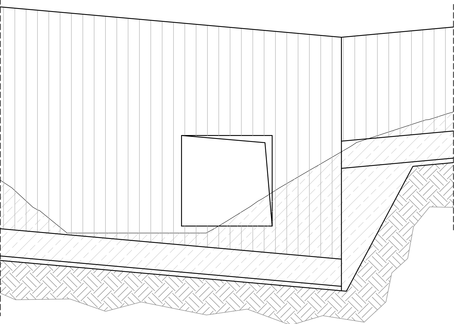
TOMBINO TM21 SEZIONE TRASVERSALE B-B SCALA 1:100
