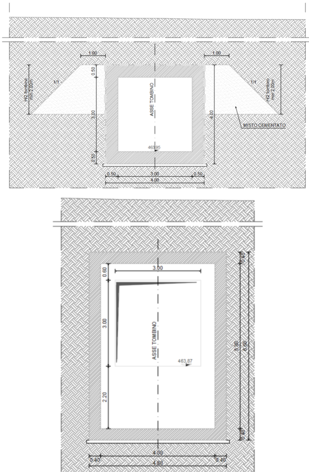
Figura 1 – Sezione trasversale corrente e in corrispondenza dei pozzi
