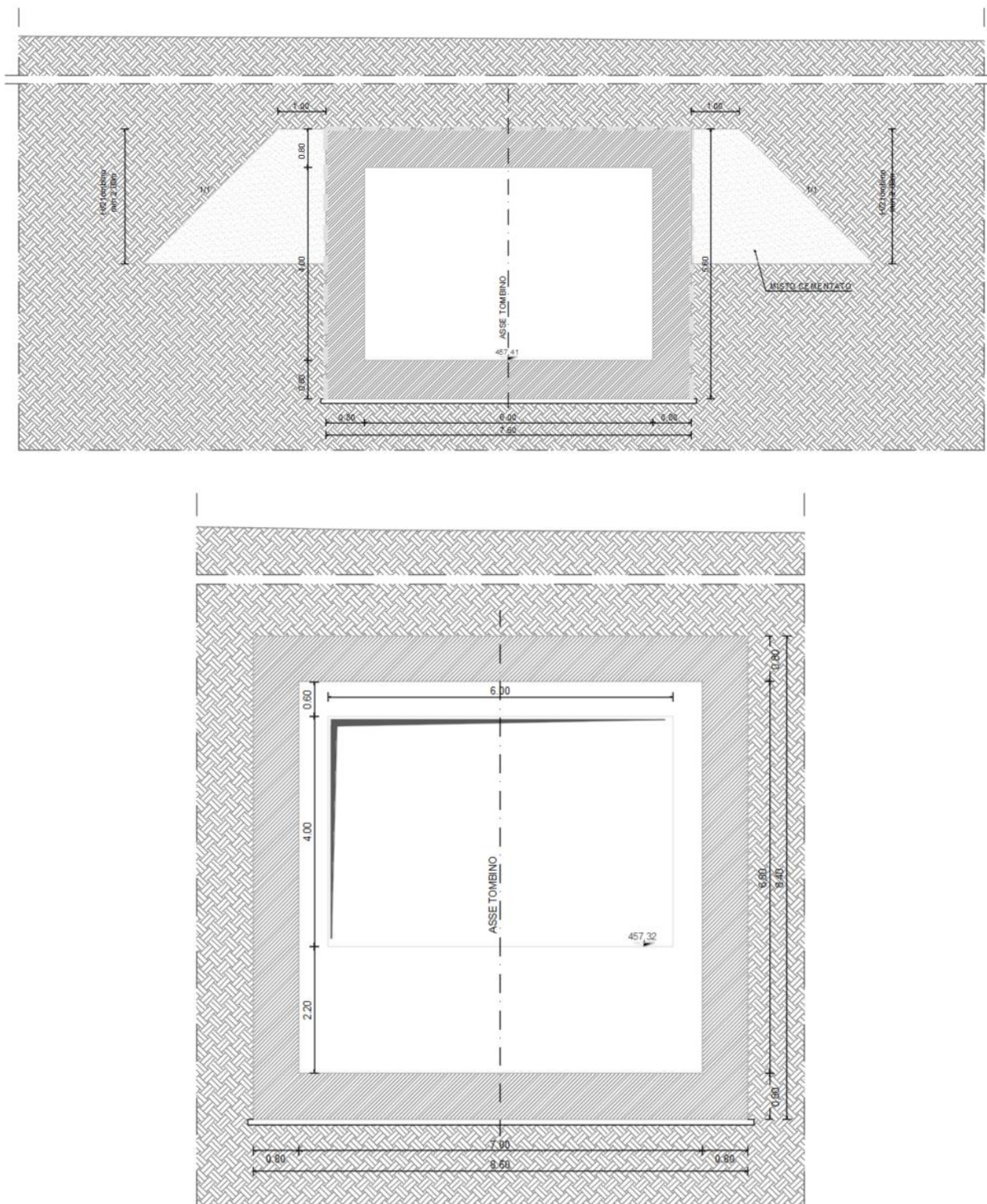
Figura 1 – Sezione trasversale corrente e in corrispondenza dei pozzi
