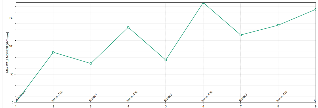
Figura 24: involuppo del momento flettente per la combinazione A1+M1+R1 per gli step da 1 a 10 (scavo completato + extrascavo)
