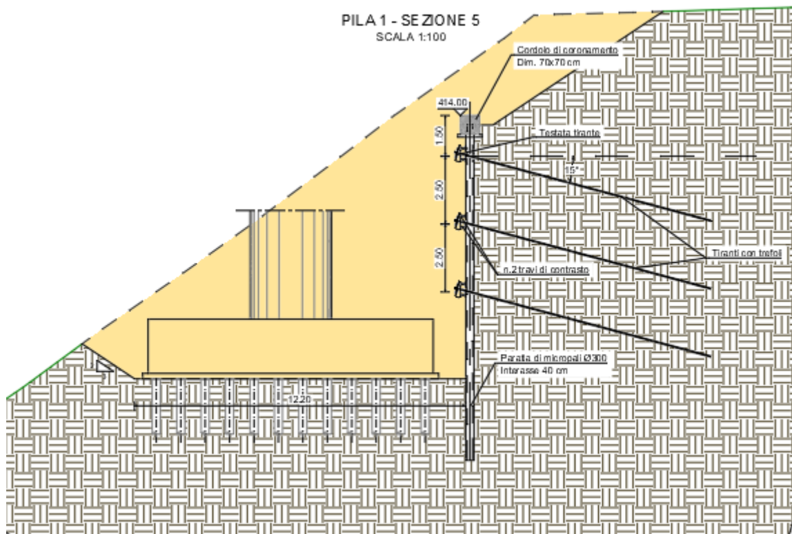
Figura 1 : sezione trasversale dell'opera
