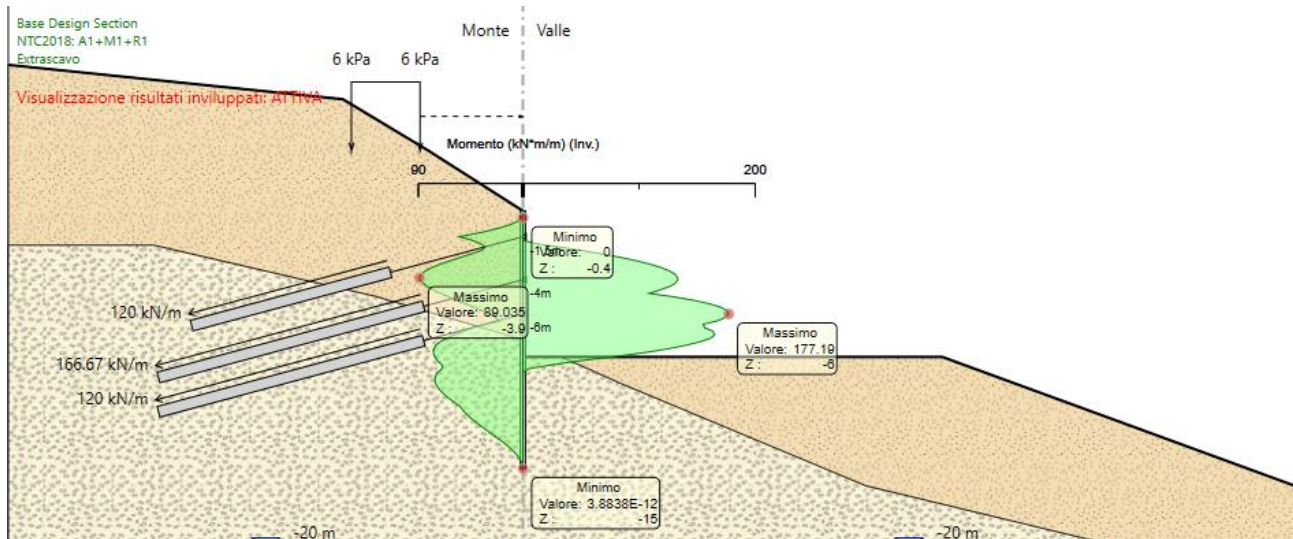
Momenti massimi (assoluti) elementi parete
