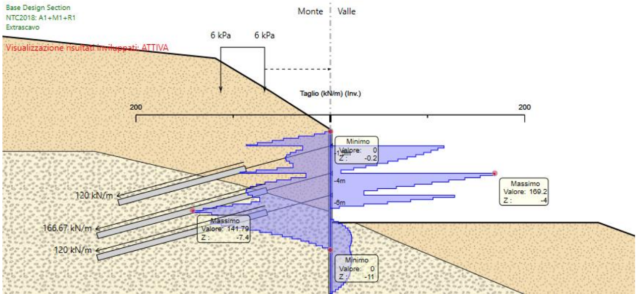
Tagli massimi (assoluti) elementi parete D.A. <NTC2018: A1+M1+R1>
