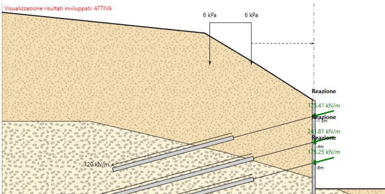
Figura 27: massimo tiro agente nei tiranti per la combinazione A1+M1+R1 e A2+M2+R1 (involuppo dei valori)
