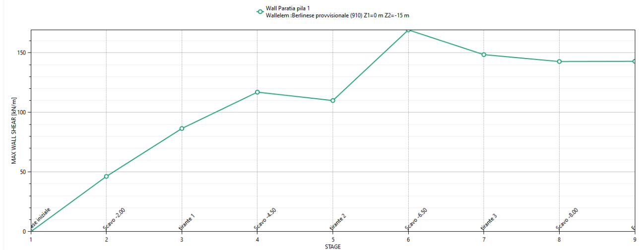
Figura 25: inviluppo dello sforzo di taglio per la combinazione A1+M1+R1 per gli step da 1 a 10 (scavo completato + extrascavo)
