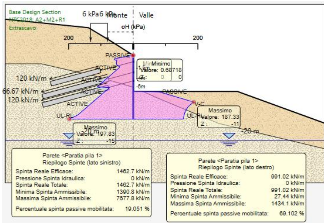
Figura 29 : \sigma'_h nel diaframma [kN/m] – comb. SLU – A2+M2+R1 – fase 9
