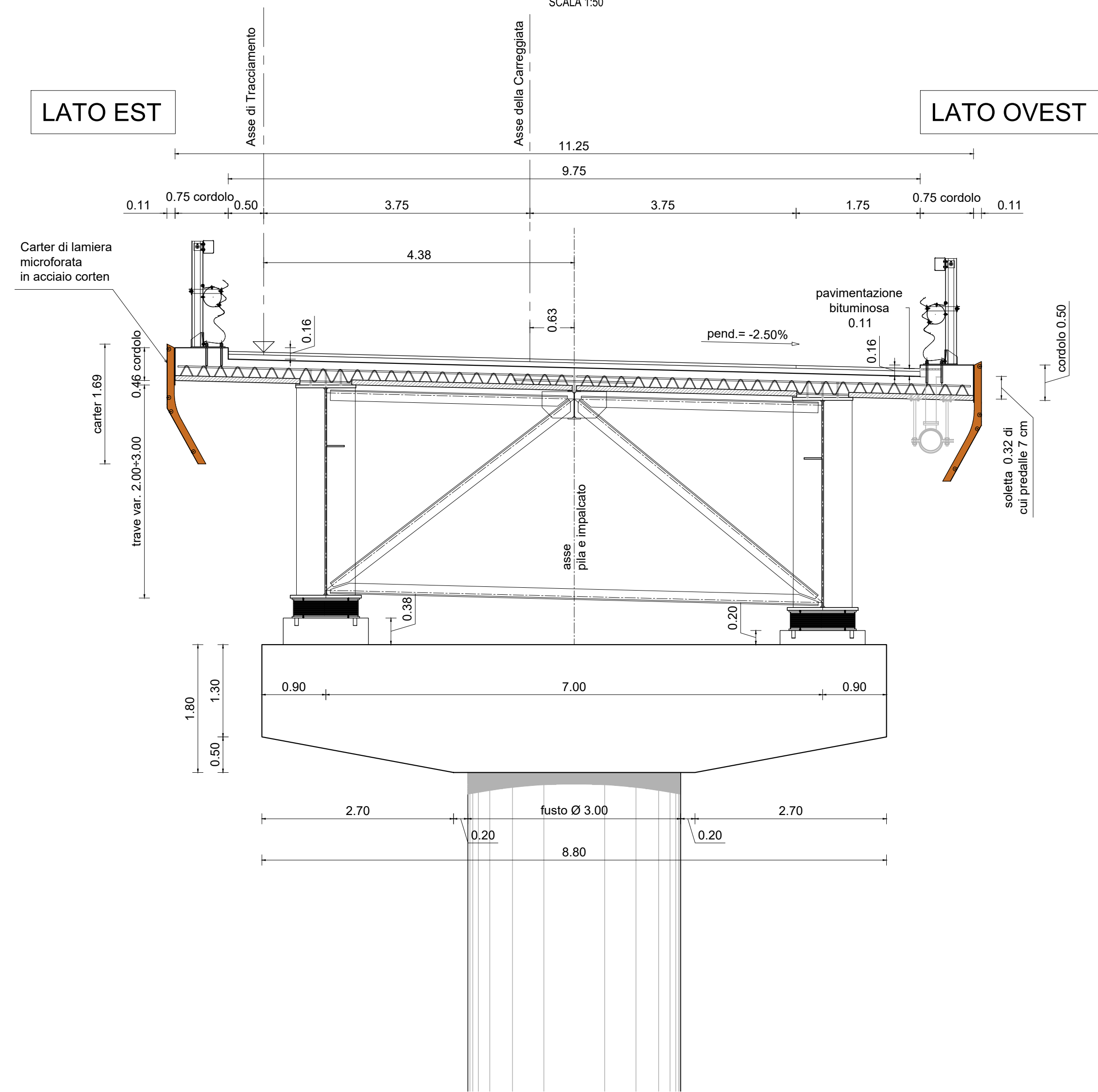
SEZIONE IMPALCATO SCALA 1:50
