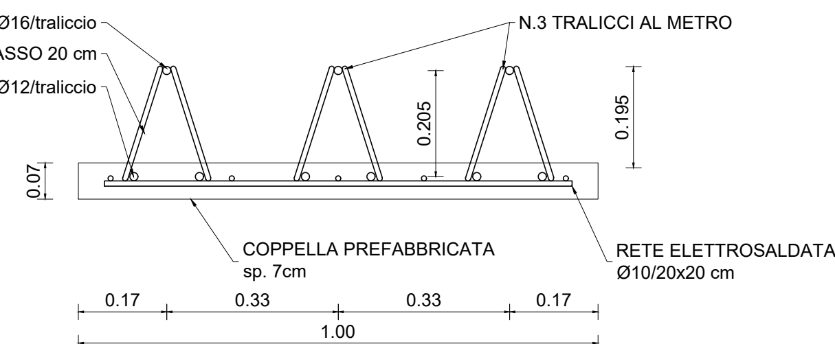
IMPALCATO IN ACCIAIO SEZIONE PEDALLES PREFABBRICATE SCALA 1:10
