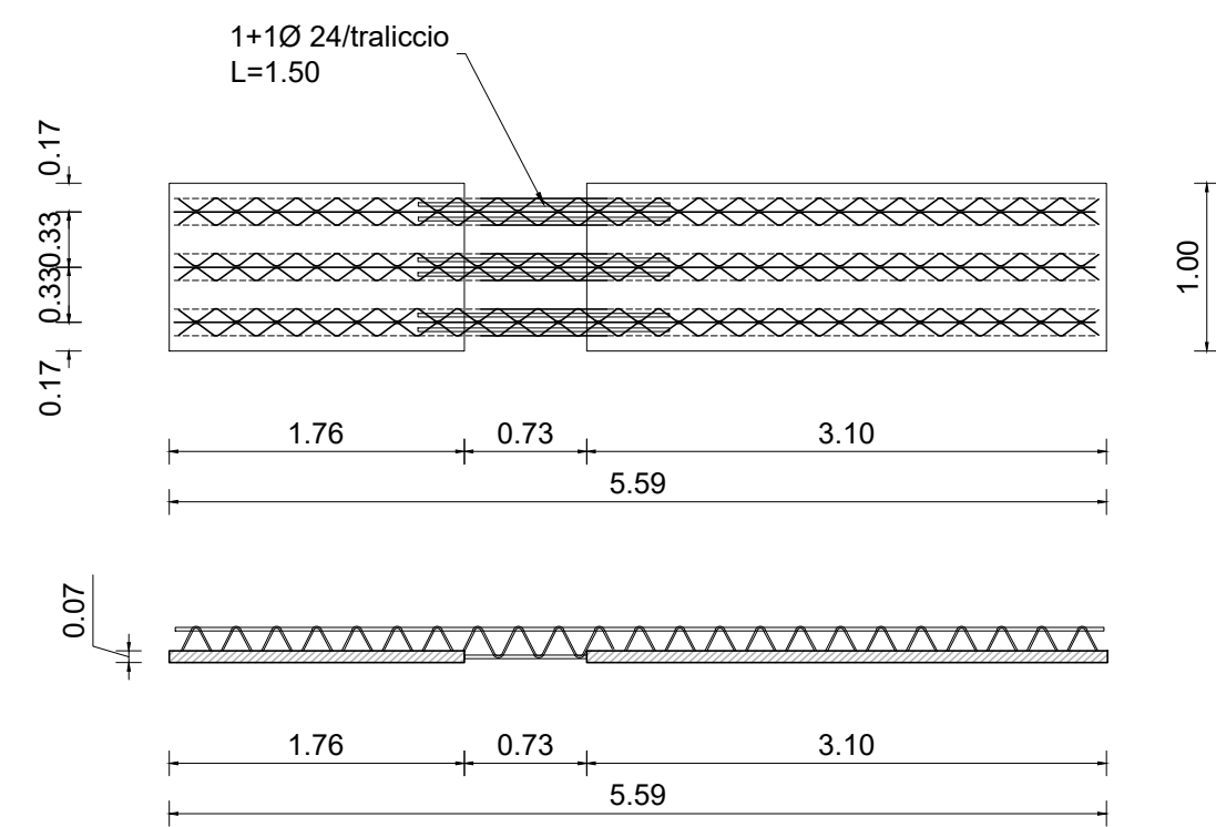
IMPALCATO IN ACCIAIO PIANTA PEDALLES PREFABBRICATE SCALA 1:50
