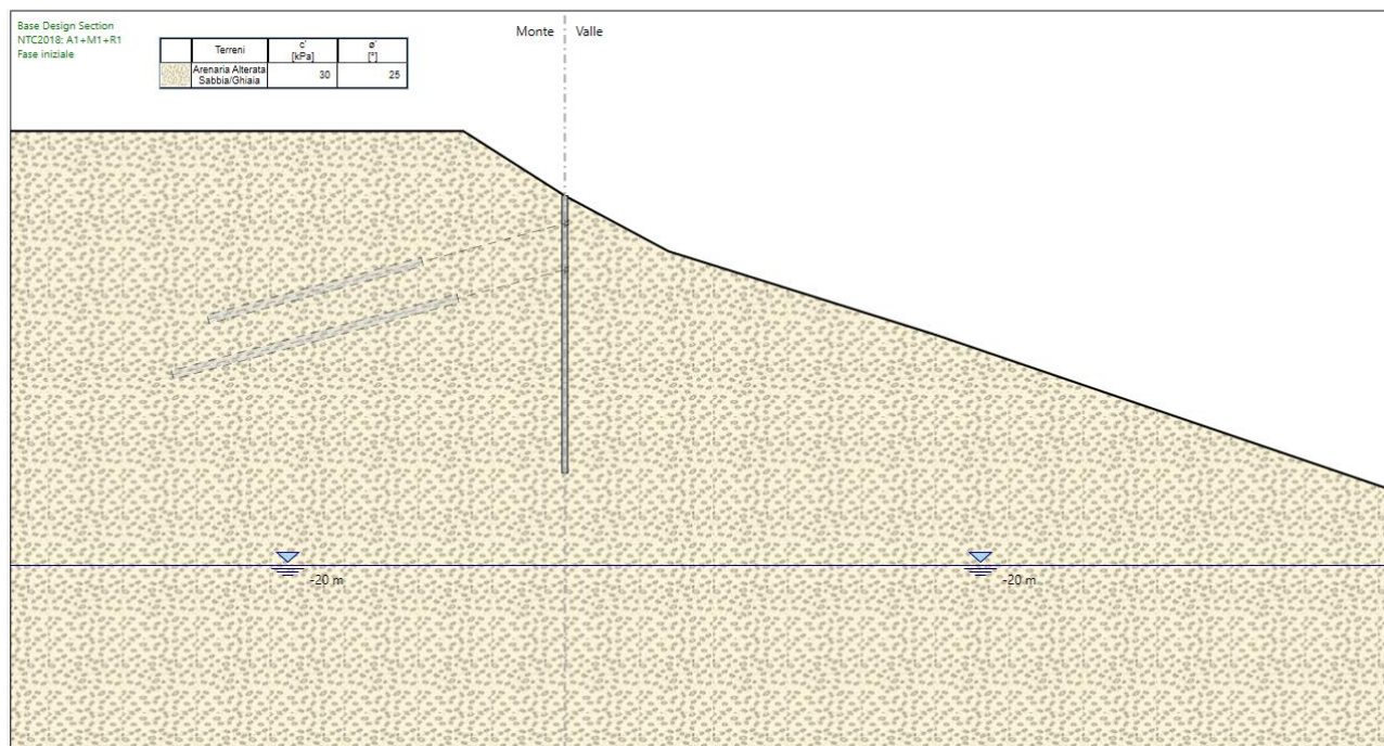
Figura 8 : fase di calcolo nr. 1
