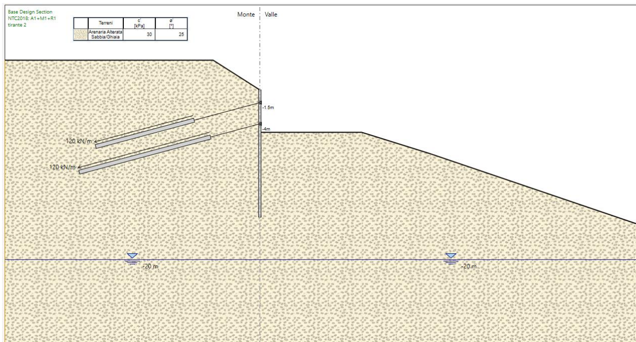
Figura 12 : fase di calcolo nr. 5
