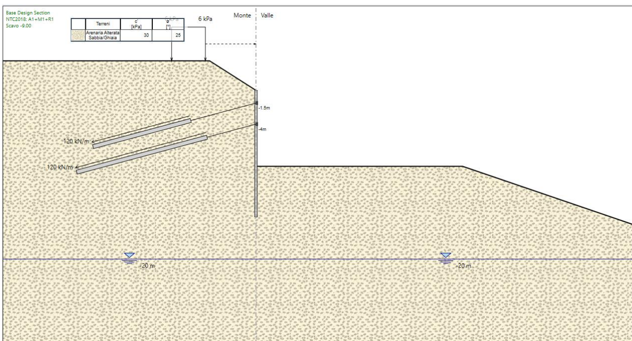
Figura 13 : fase di calcolo nr. 6
