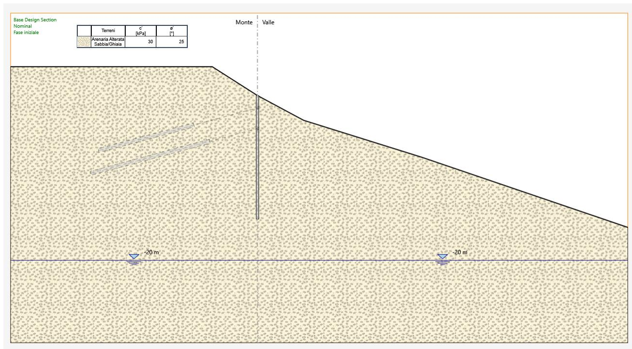
Figura 3 : schema del modello di calcolo adottato
