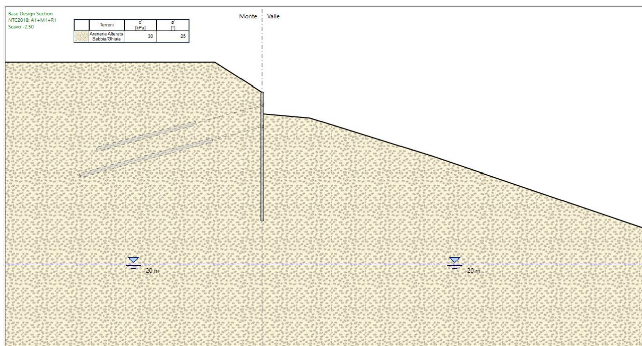
Figura 9 : fase di calcolo nr. 2
