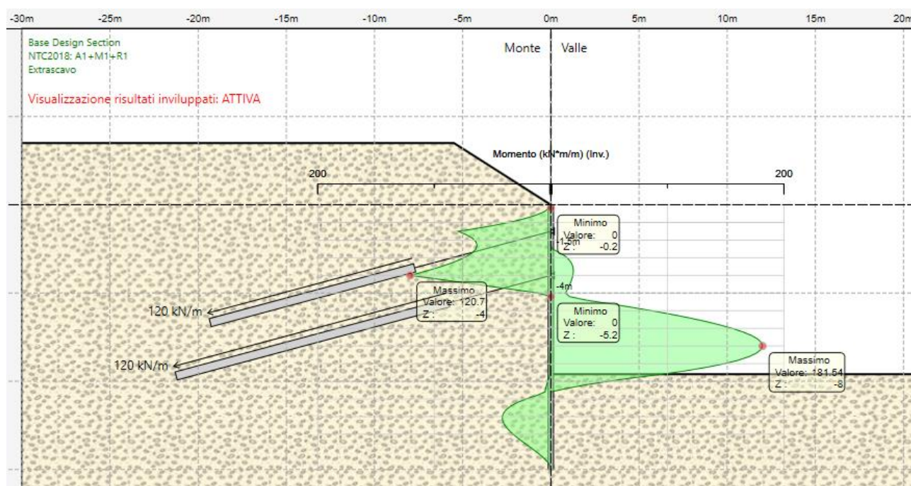
Figura 15: involuppo del momento flettente per la combinazione A1+M1+R1 per gli step da 1 a 7 (scavo completato + extrascavo)
