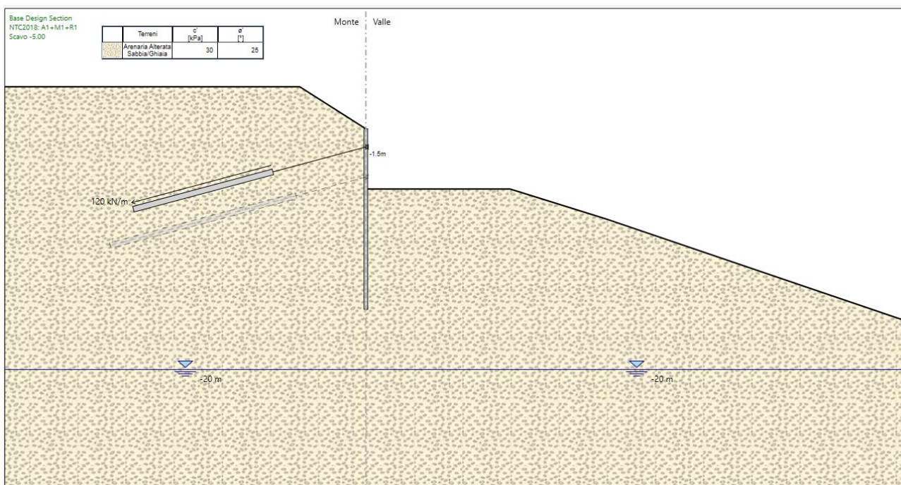
Figura 11 : fase di calcolo nr. 4
