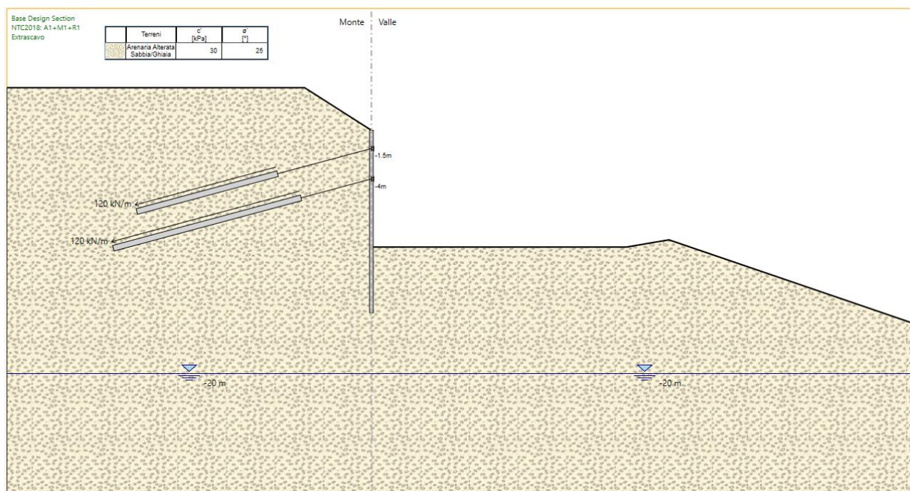
Figura 14 : fase di calcolo nr. 7
