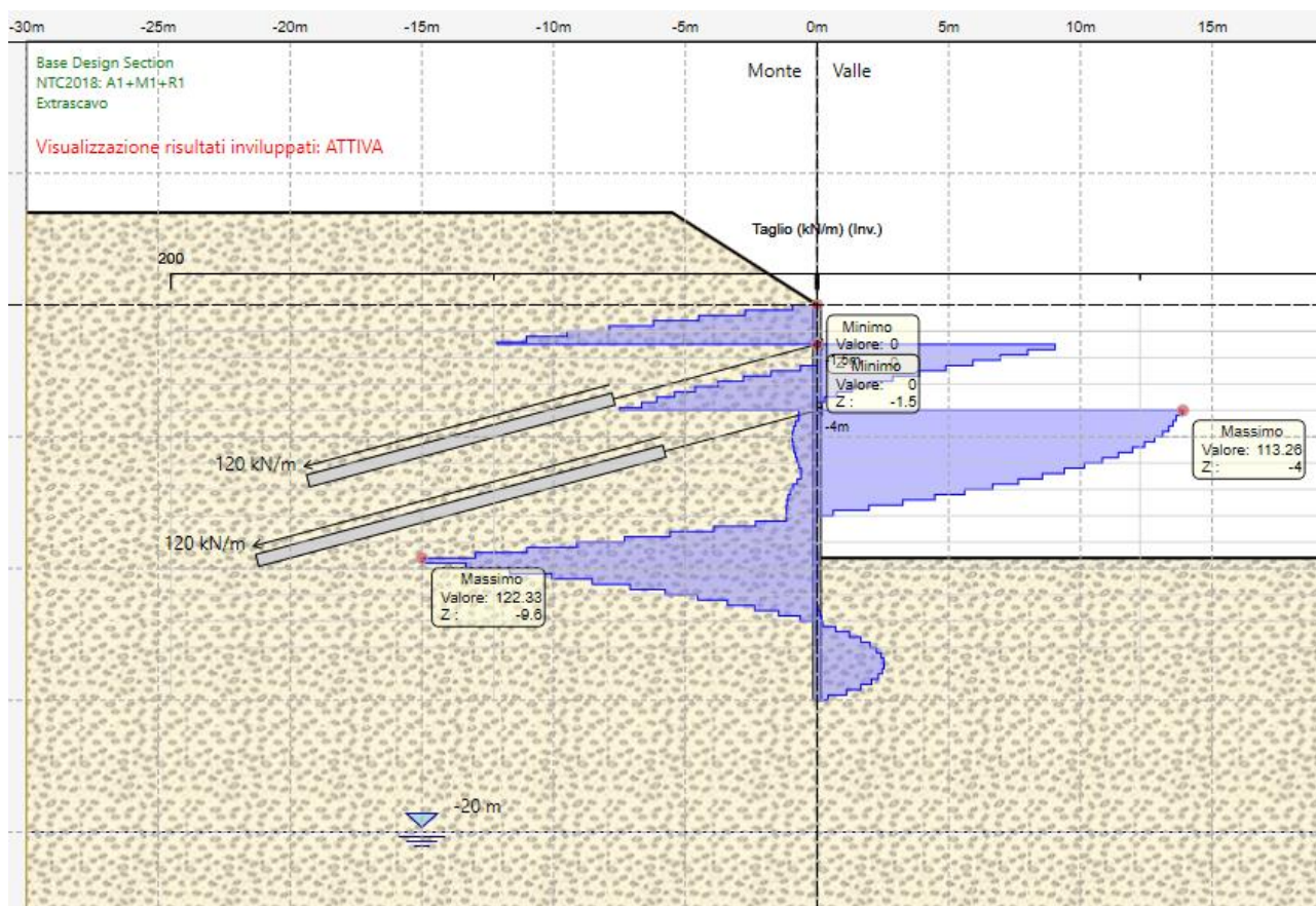
Figura 16: involuppo dello sforzo di taglio per la combinazione A1+M1+R1 per gli step da 1 a 7 (scavo completato + extrascavo)
