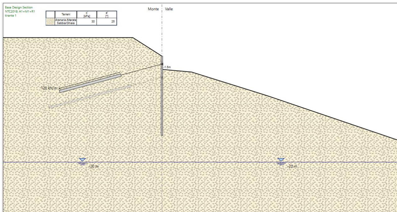
Figura 10 : fase di calcolo nr. 3
