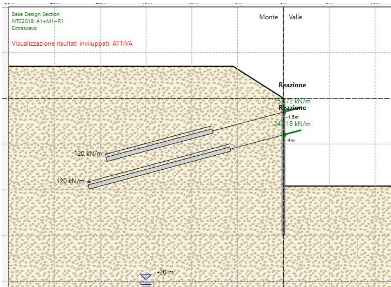
Figura 18: massimo tiro agente nei tiranti del livello fila 1 e della fila 2, per la combinazione A1+M1+R1 nello step 4 (fila 1) e A2+M2+R1 nello step 7 per la fila 2
