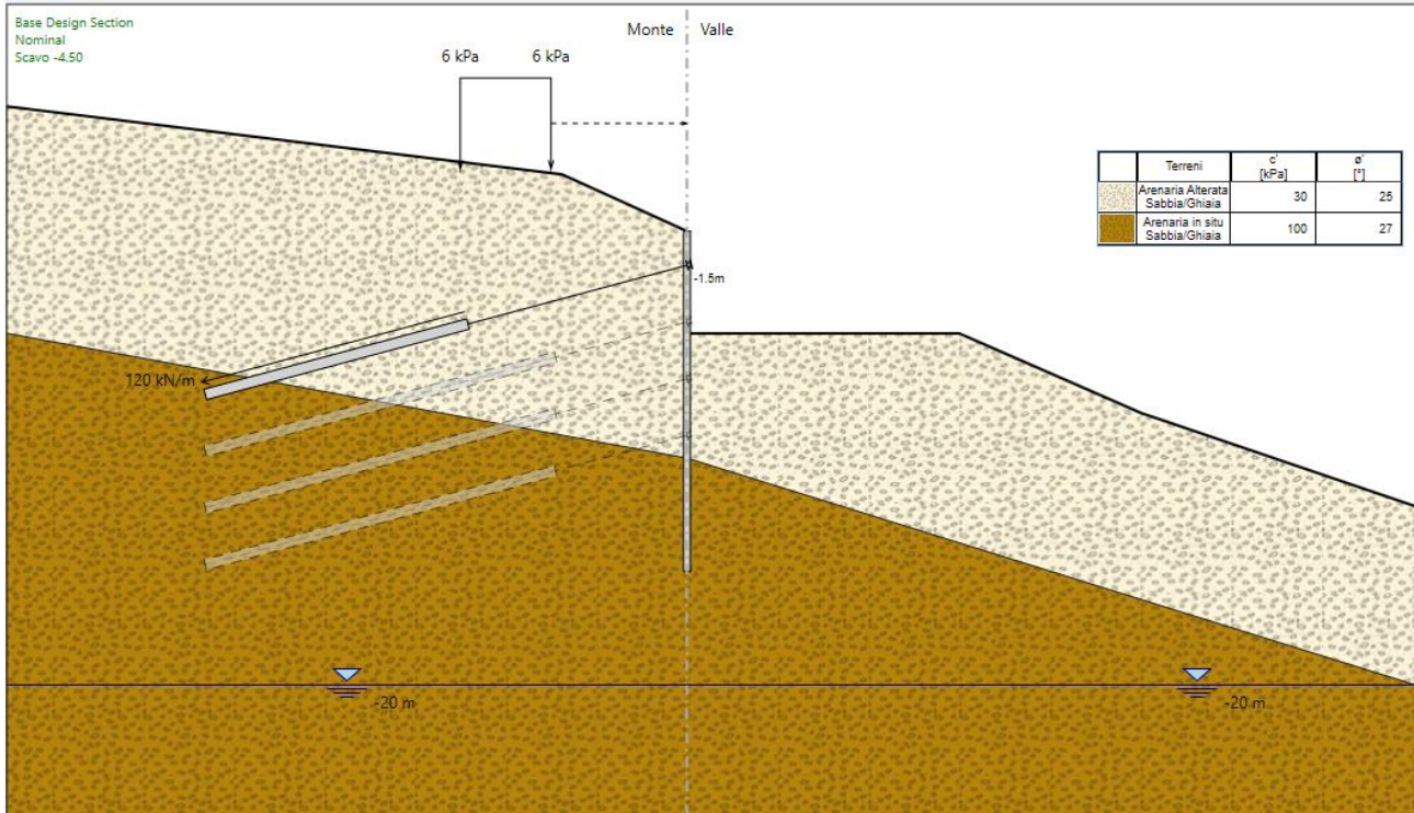
Figura 12 : fase di calcolo nr. 4
