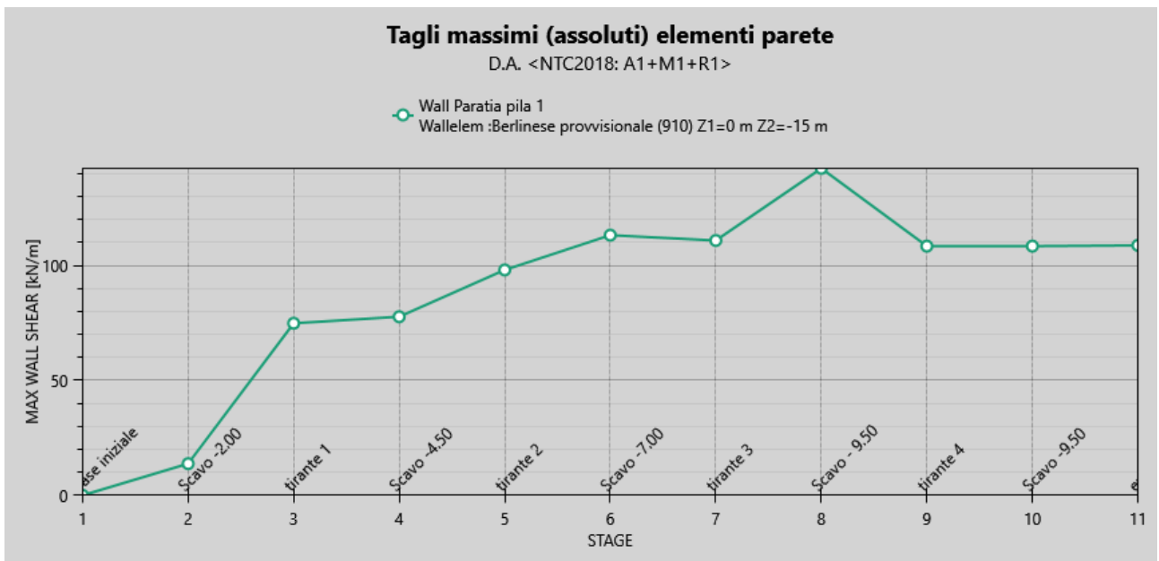
Figura 21: inviluppo dello sforzo di taglio per la combinazione A1+M1+R1 per gli step da 1 a 10 (scavo completato + extrascavo)
