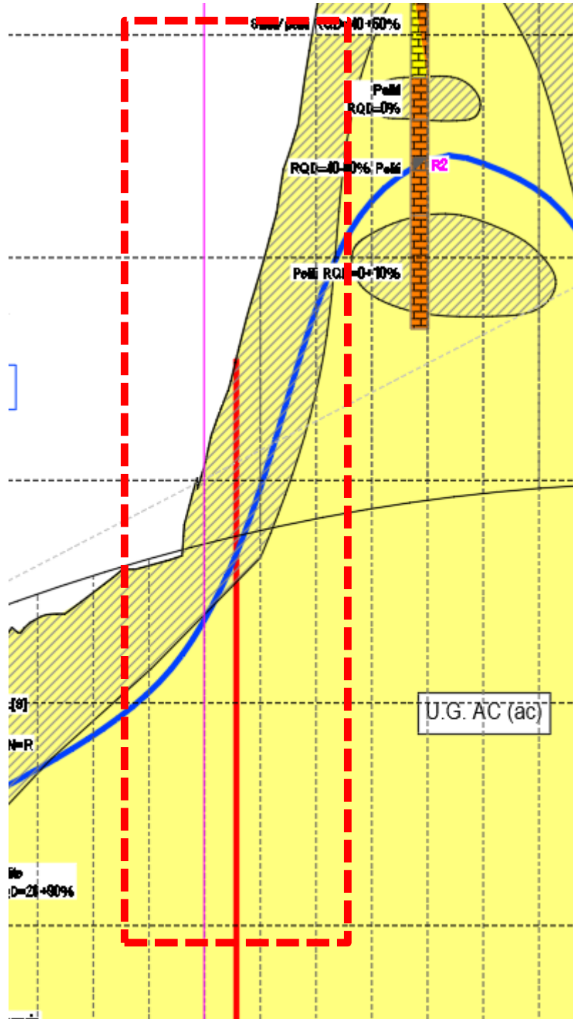
Figura 2: estratto dal profilo geologico di progetto
