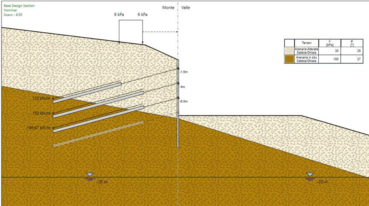
Figura 16 : fase di calcolo nr. 8
