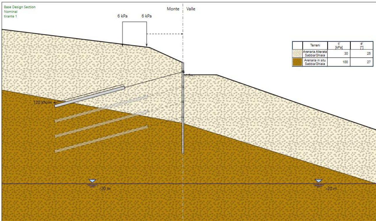
Figura 11 : fase di calcolo nr. 3
