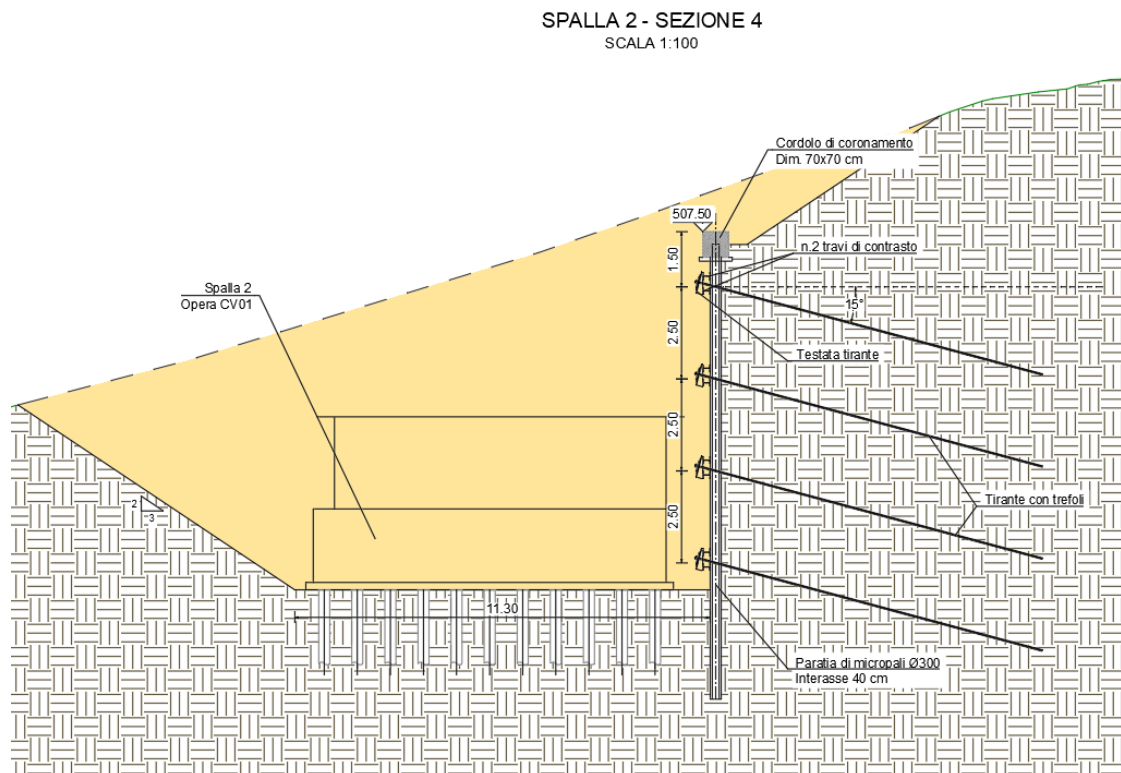
Figura 1: sezione tipologica di verifica
