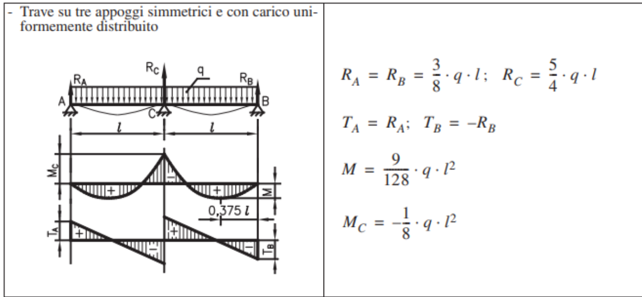
Figura 24: schema statico considerato per lo studio delle travi di ripartizione
