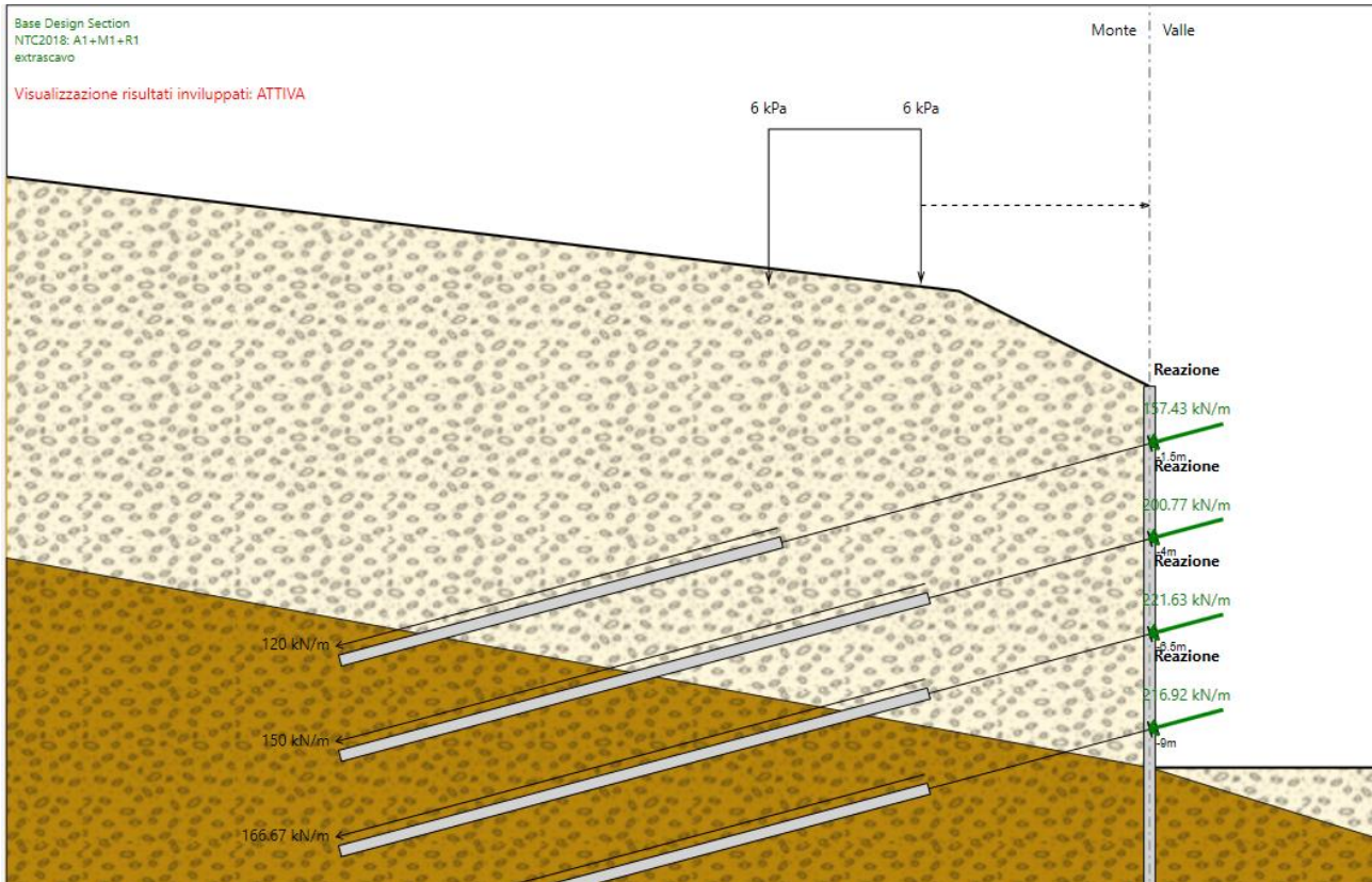
Figura 23: involuppo del tiro agente nei tiranti per le combinazioni A1+M1+R1, A1+M1+R3 e A2+M2+R1
