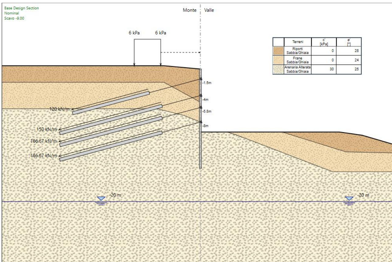
Figura 4 : schema del modello di calcolo adottato
