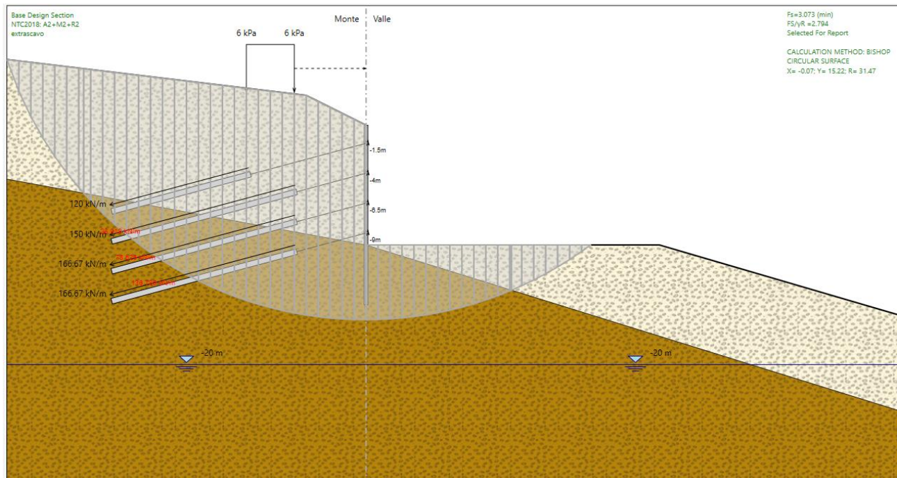
Figura 27 : superfici di scorrimento critica – comb. SLU - A2 + M2 + R2
