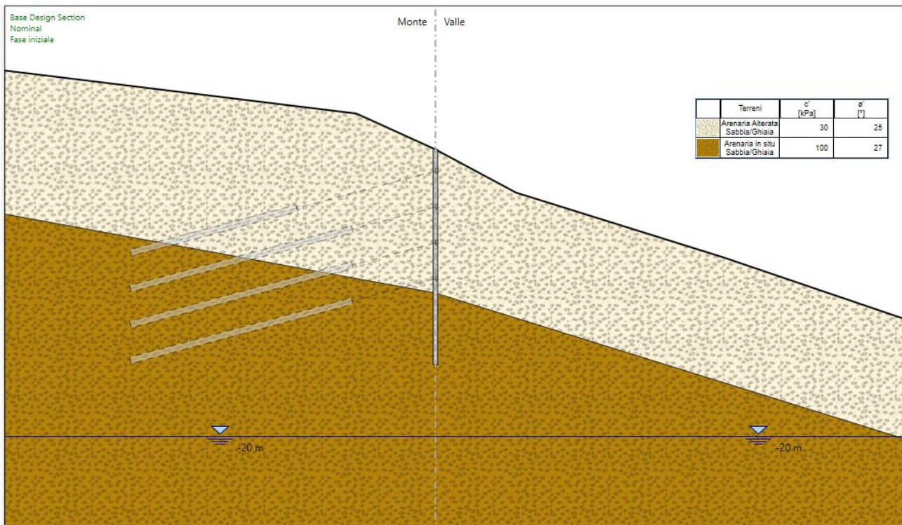
Figura 9 : fase di calcolo nr. 1
