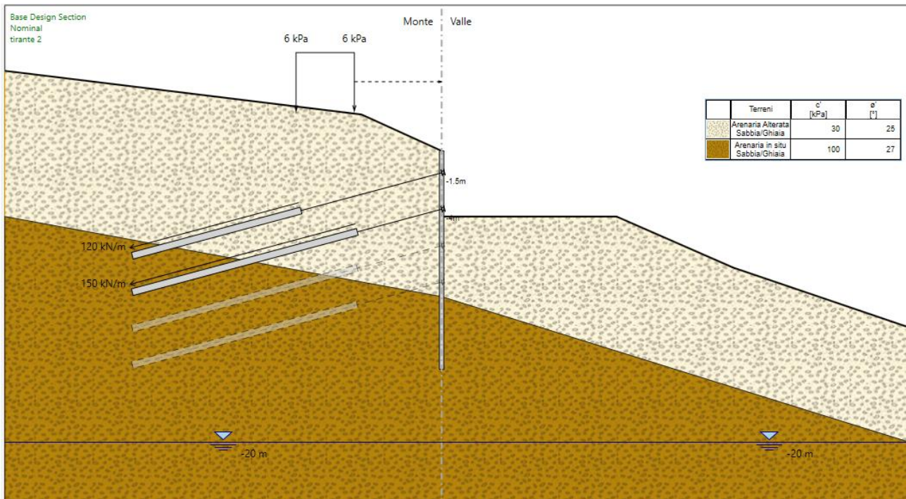
Figura 13 : fase di calcolo nr. 5
