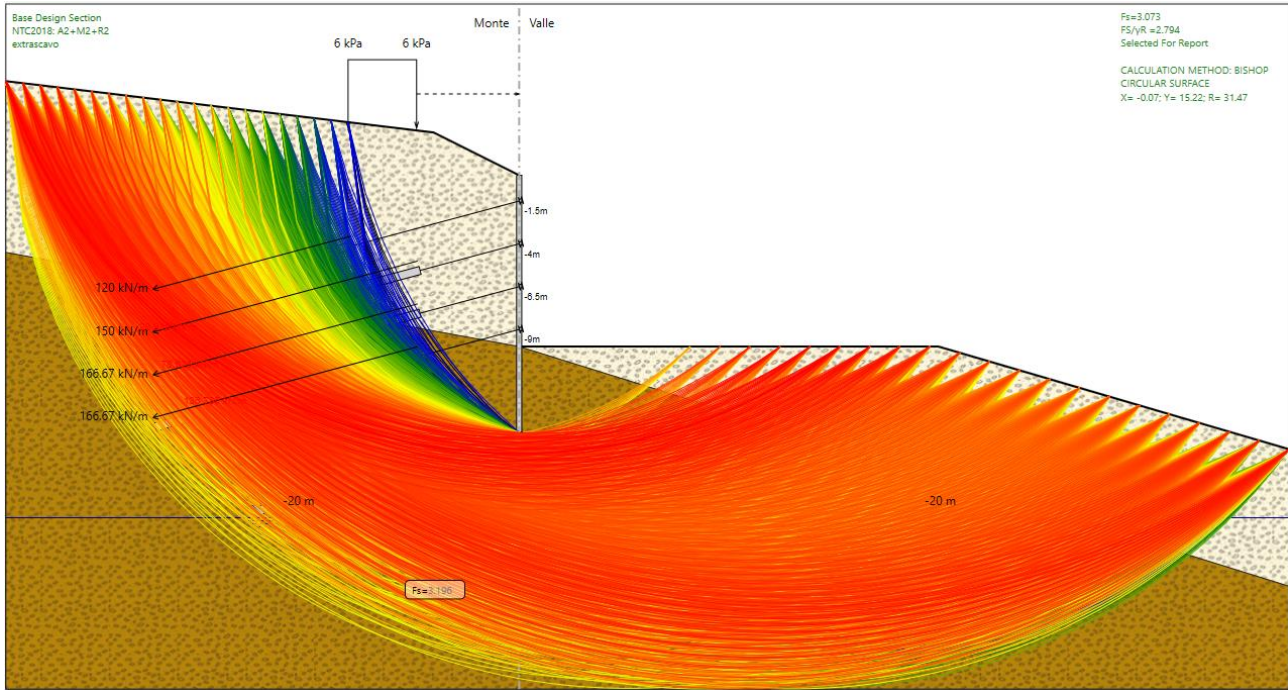
Figura 26 : superfici di scorrimento analizzate – comb. SLU - A2 + M2 + R2
