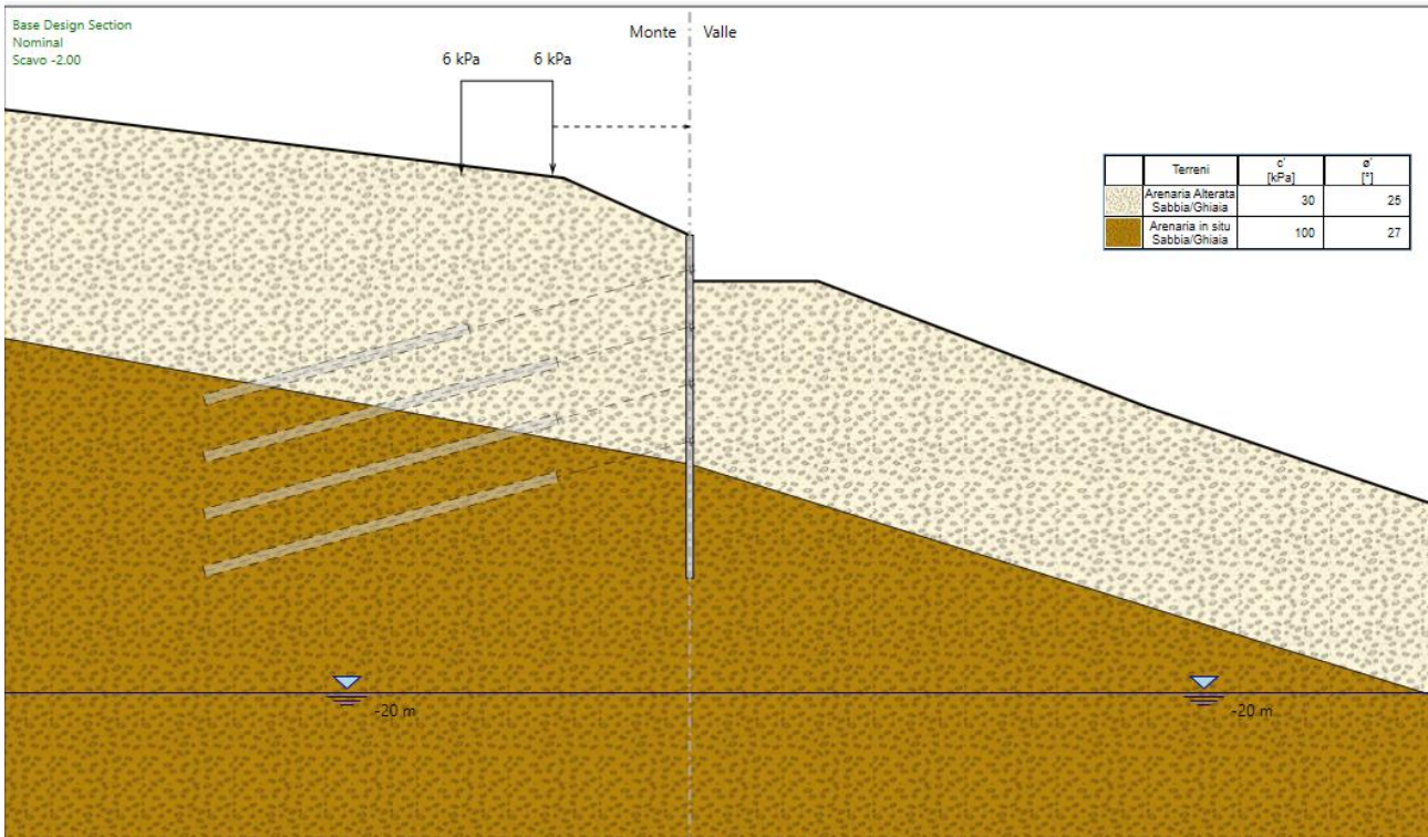
Figura 10 : fase di calcolo nr. 2
