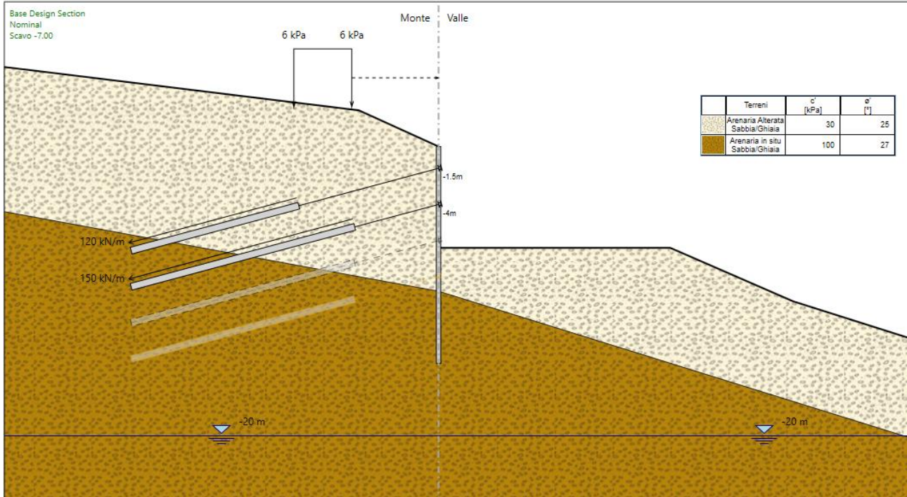
Figura 14 : fase di calcolo nr. 6
