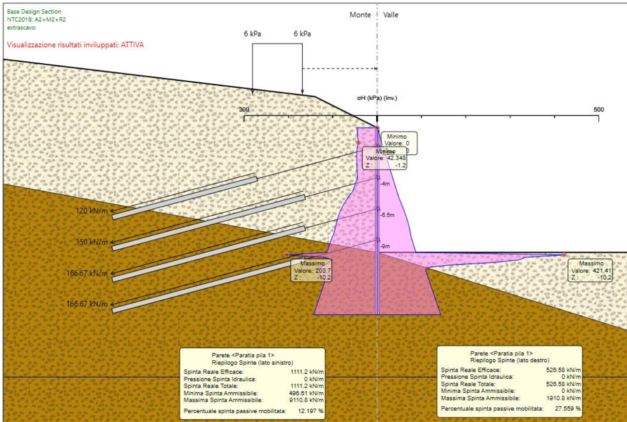
Figura 25 : \sigma'_h nel diaframma [kN/m] – comb. SLU – A2+M2+R1 – involuppo
