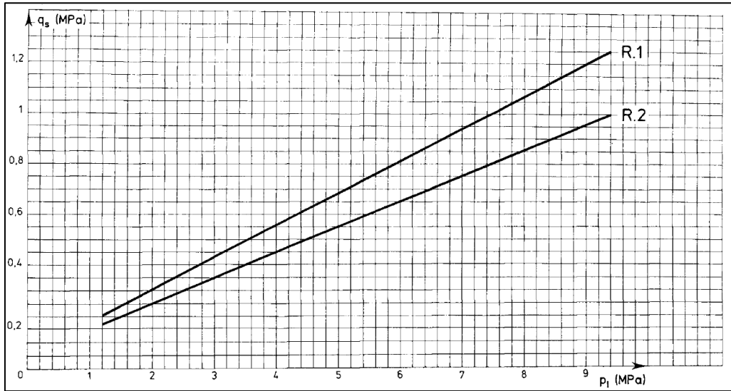
Figura 3-5 Grafici per il calcolo di q_s per rocce alterate e fratturate
