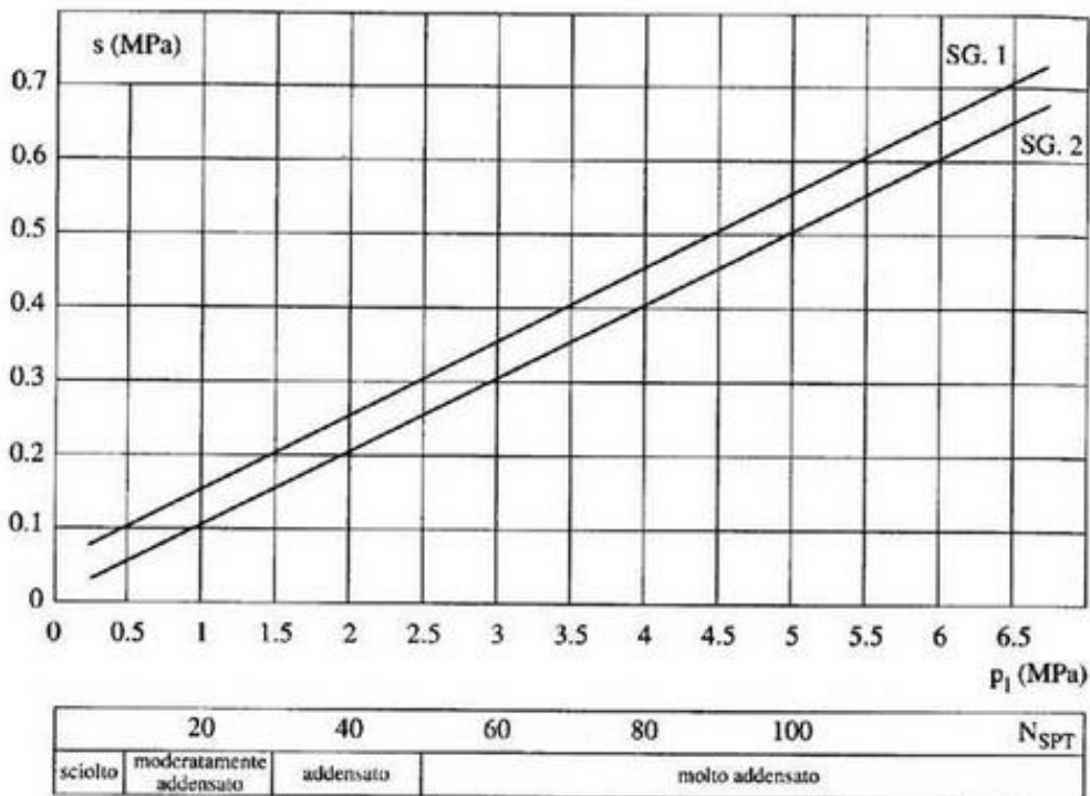
Figura 3-6 Grafici per il calcolo di q_s per sabbie e ghiaie
