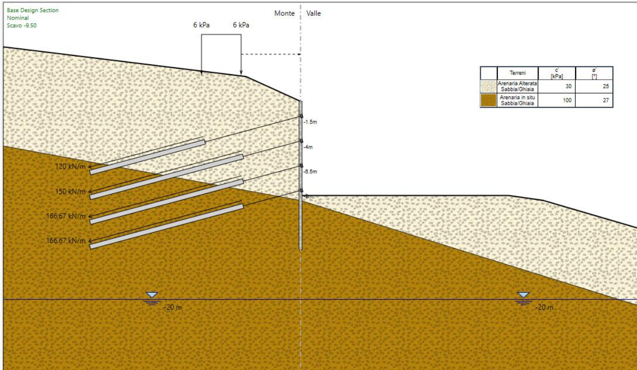
Figura 18 : fase di calcolo nr. 10
