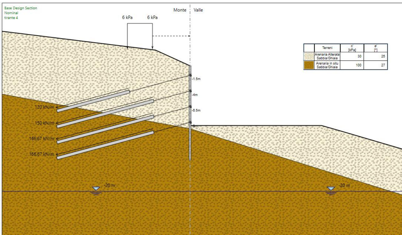
Figura 17 : fase di calcolo nr. 9
