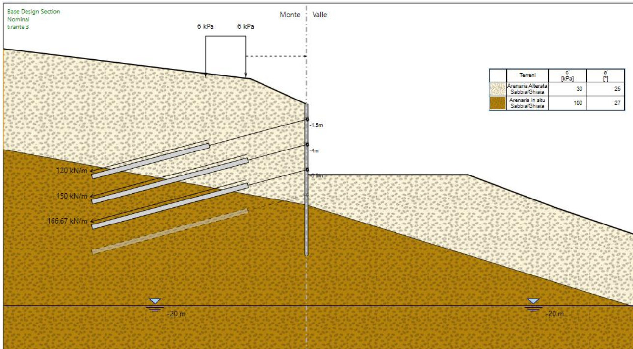
Figura 15 : fase di calcolo nr. 7
