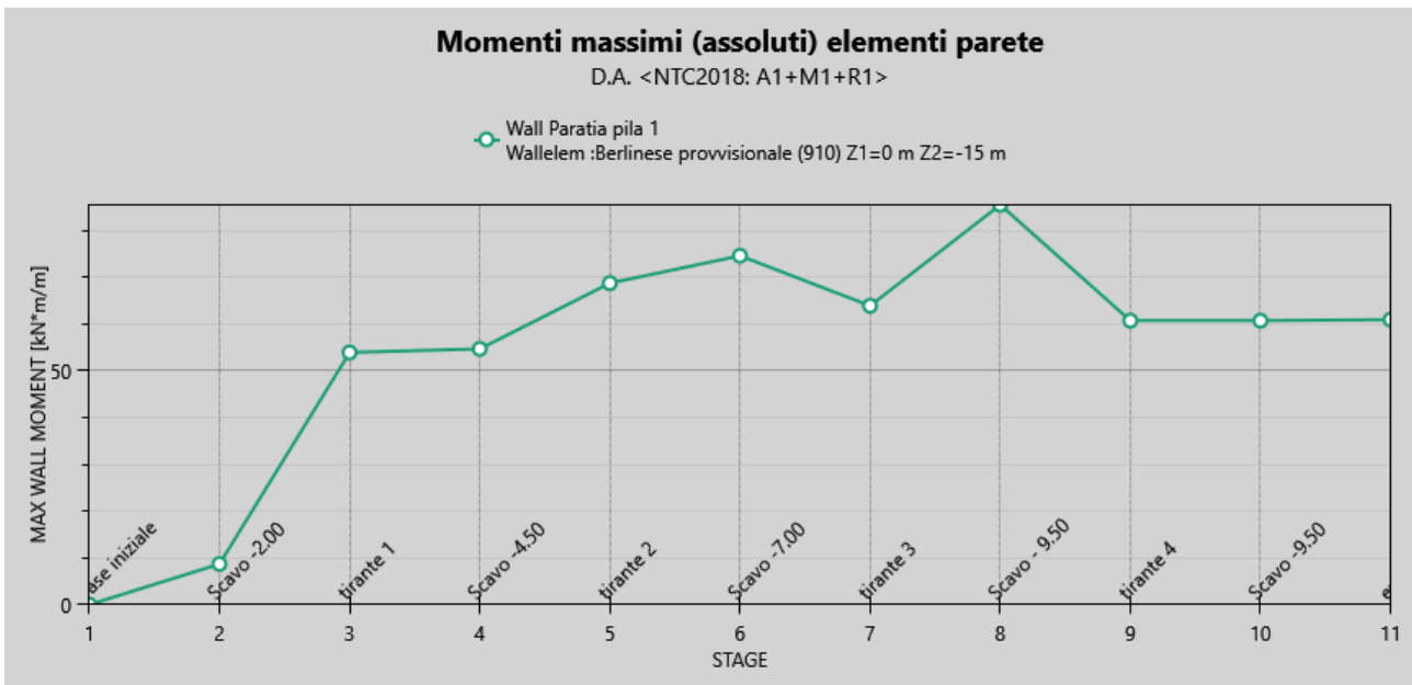
Figura 20: inviluppo del momento flettente per la combinazione A1+M1+R1 per gli step da 1 a 11 (scavo completato + extrascavo)
