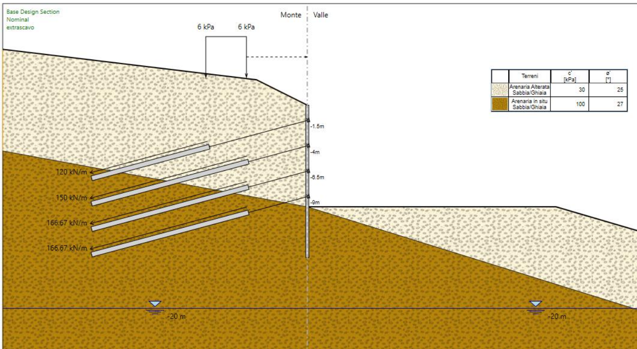
Figura 19 : fase di calcolo nr. 11
