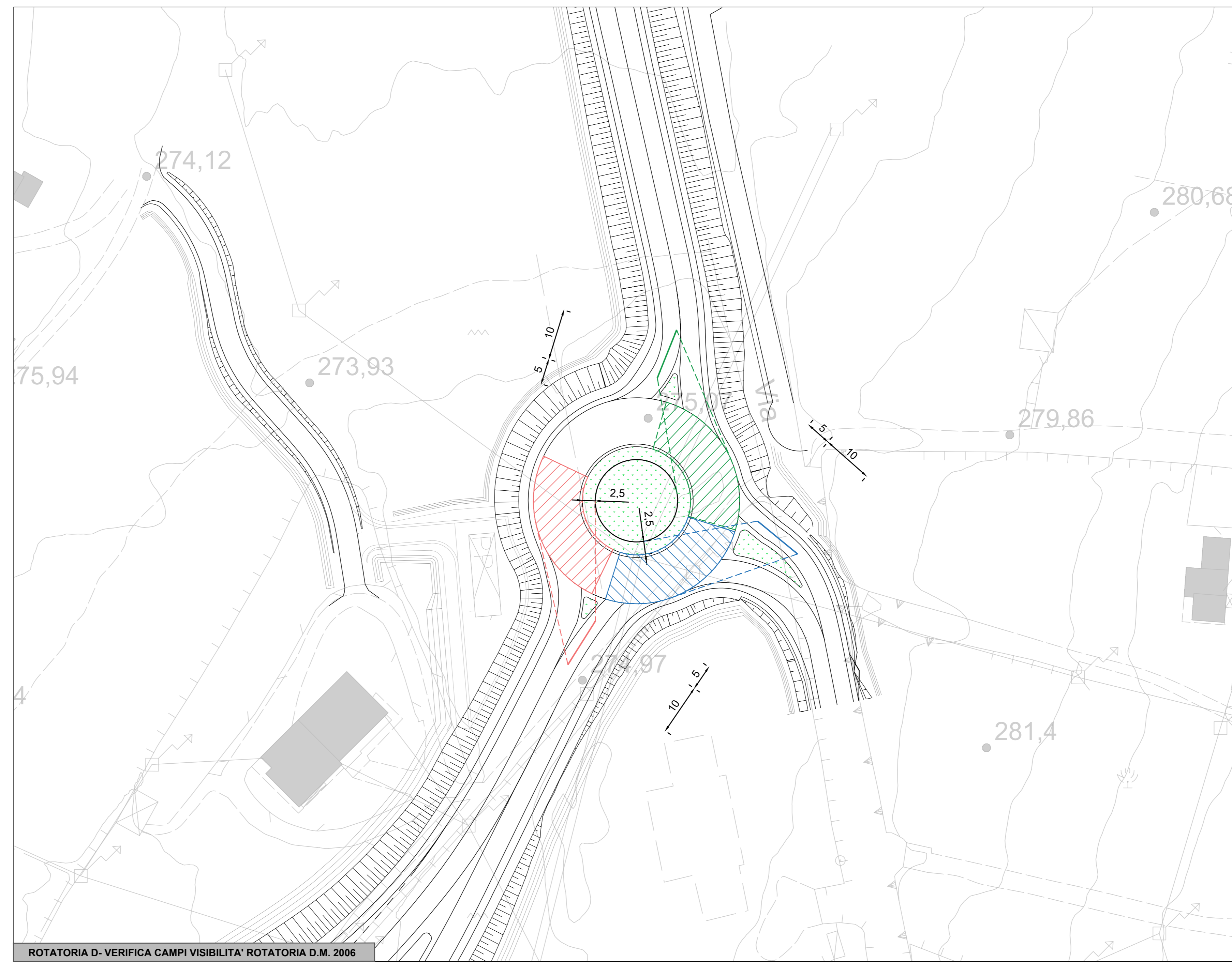
ROTATORIA D - VERIFICA CAMPI VISIBILITA' ROTATORIA D.M. 2006
