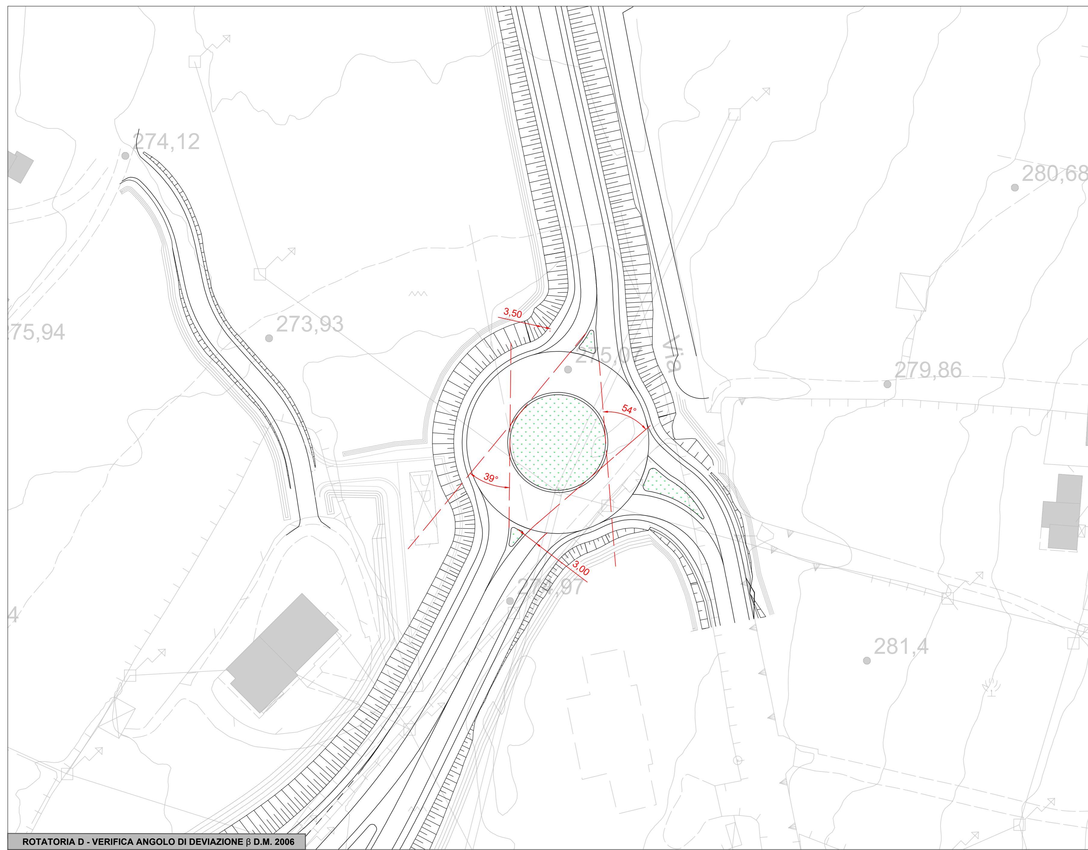
ROTATORIA D - VERIFICA ANGOLO DI DEVIAZIONE P D.M. 2006
