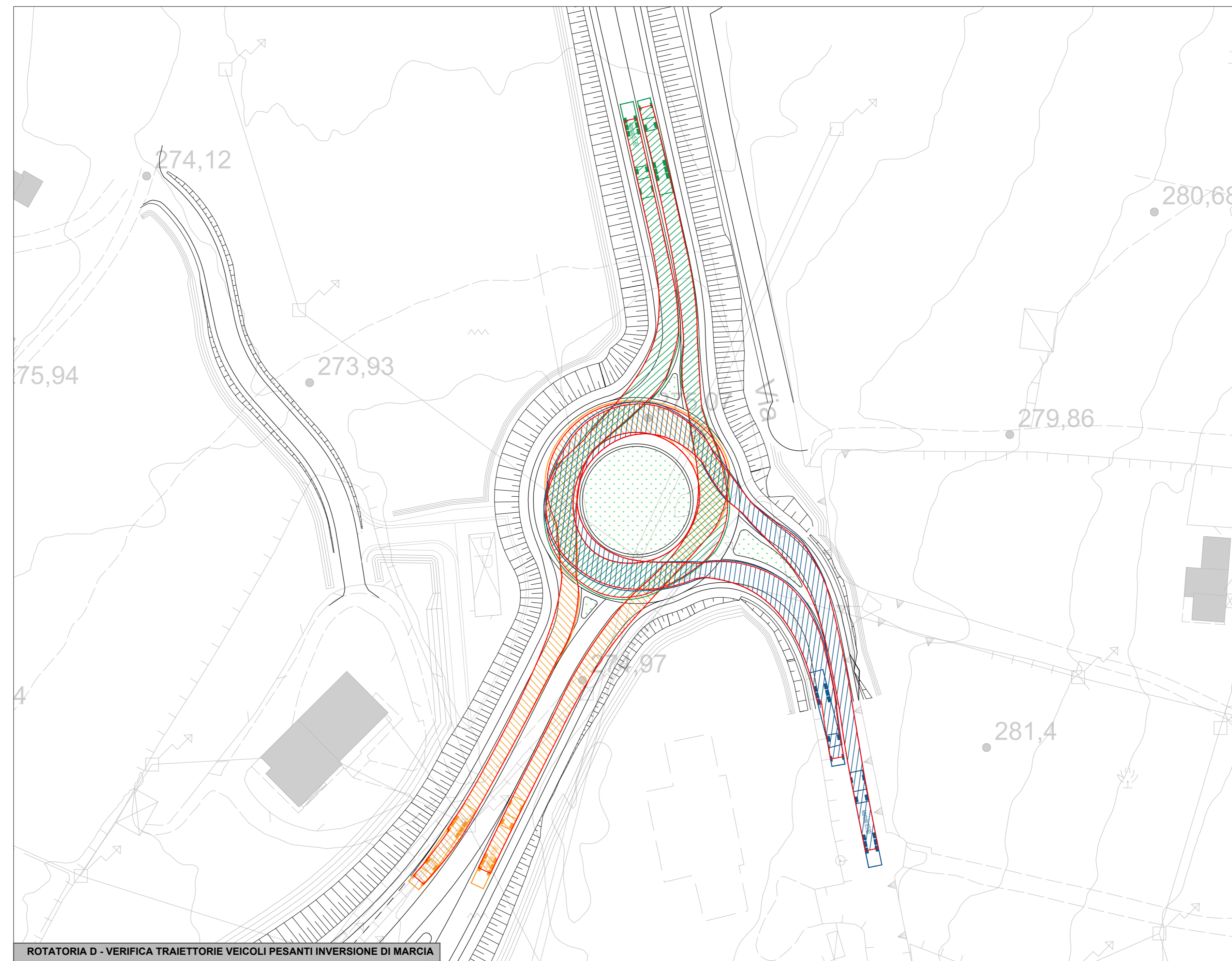
ROTATORIA D - VERIFICA TRAIETTORIE VEICOLI PESANTI INVERSIONE DI MARCIA
