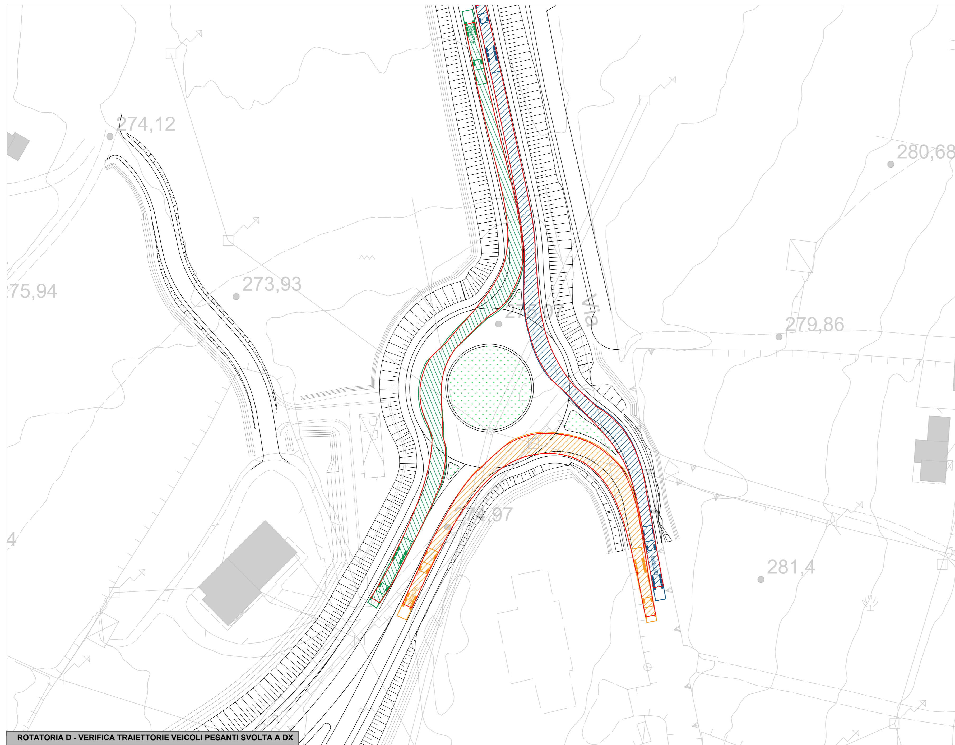
ROTATORIA D - VERIFICA TRAIETTORIE VEICOLI PESANTI SVOLTA A DX
